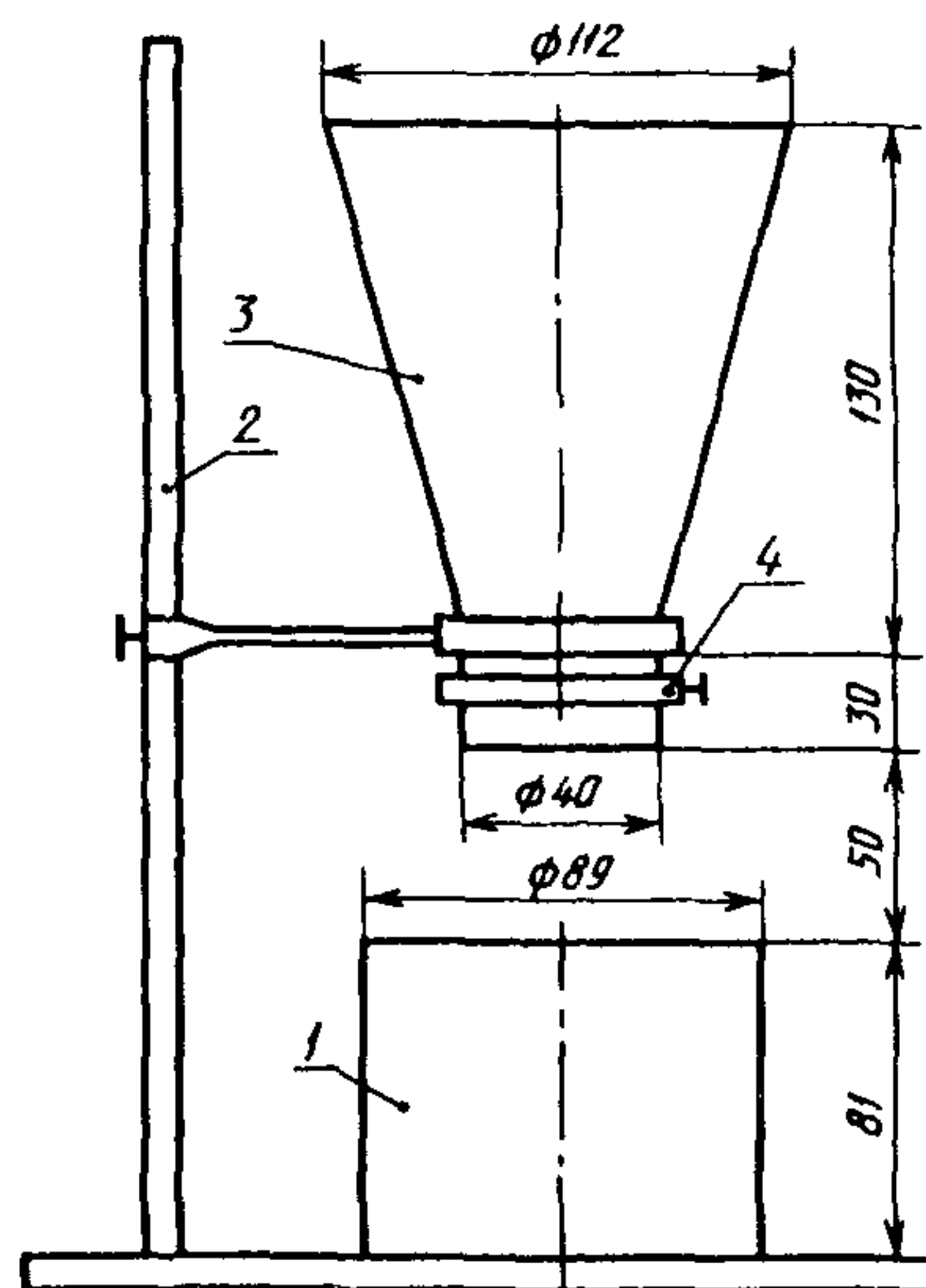
1 — измерительный цилиндр, 2 — штатив, 3 — воронка, 4 — задвижка
