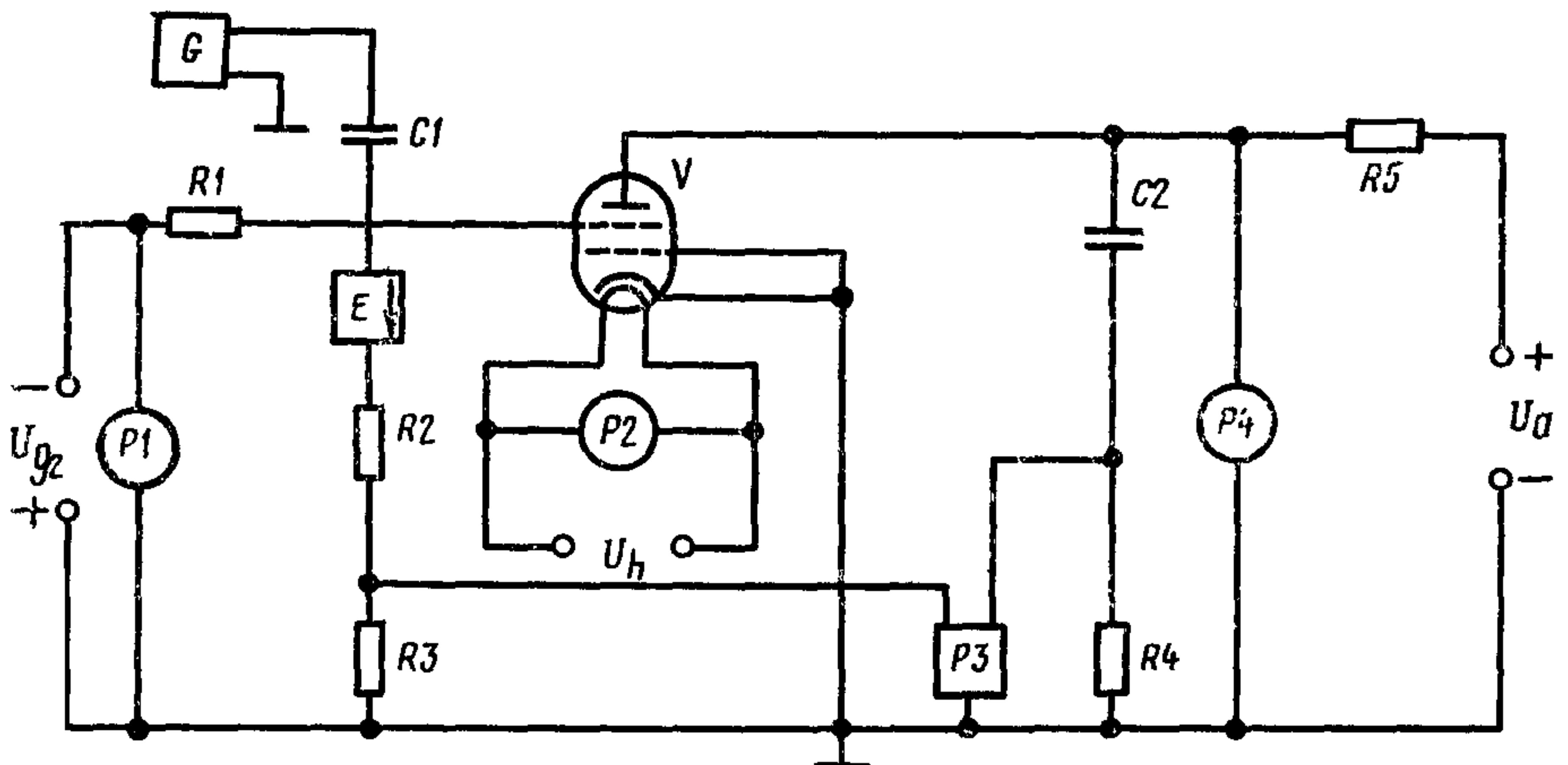
C1 —разделительный конденсатор; C2 —накопительный конденсатор; G —генератор импульсов; P1, P2, P4 —приборы для измерения постоянного (переменного) напряжения; P3 —электронный осциллограф; R1 —ограничительный резистор; R2, R3 —делитель напряжения; R4 —измерительный резистор; R5 —зарядный резистор; V —испытываемая лампа; E —электровакуумный или полупроводниковый диод
