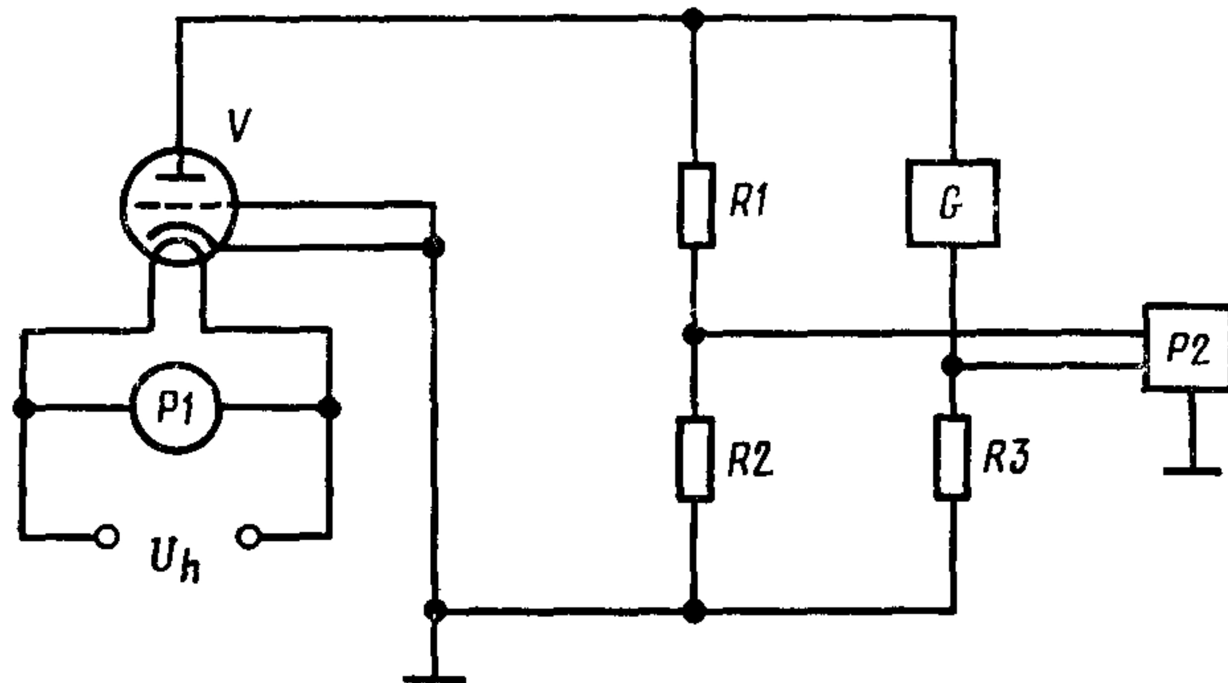
G —генератор импульсов; P1 —прибор для измерения постоянного (переменного) напряжения; P2 —электронный осциллограф; R1R2 —делитель напряжения; R3 —измерительный резистор; V —испытываемая лампа
