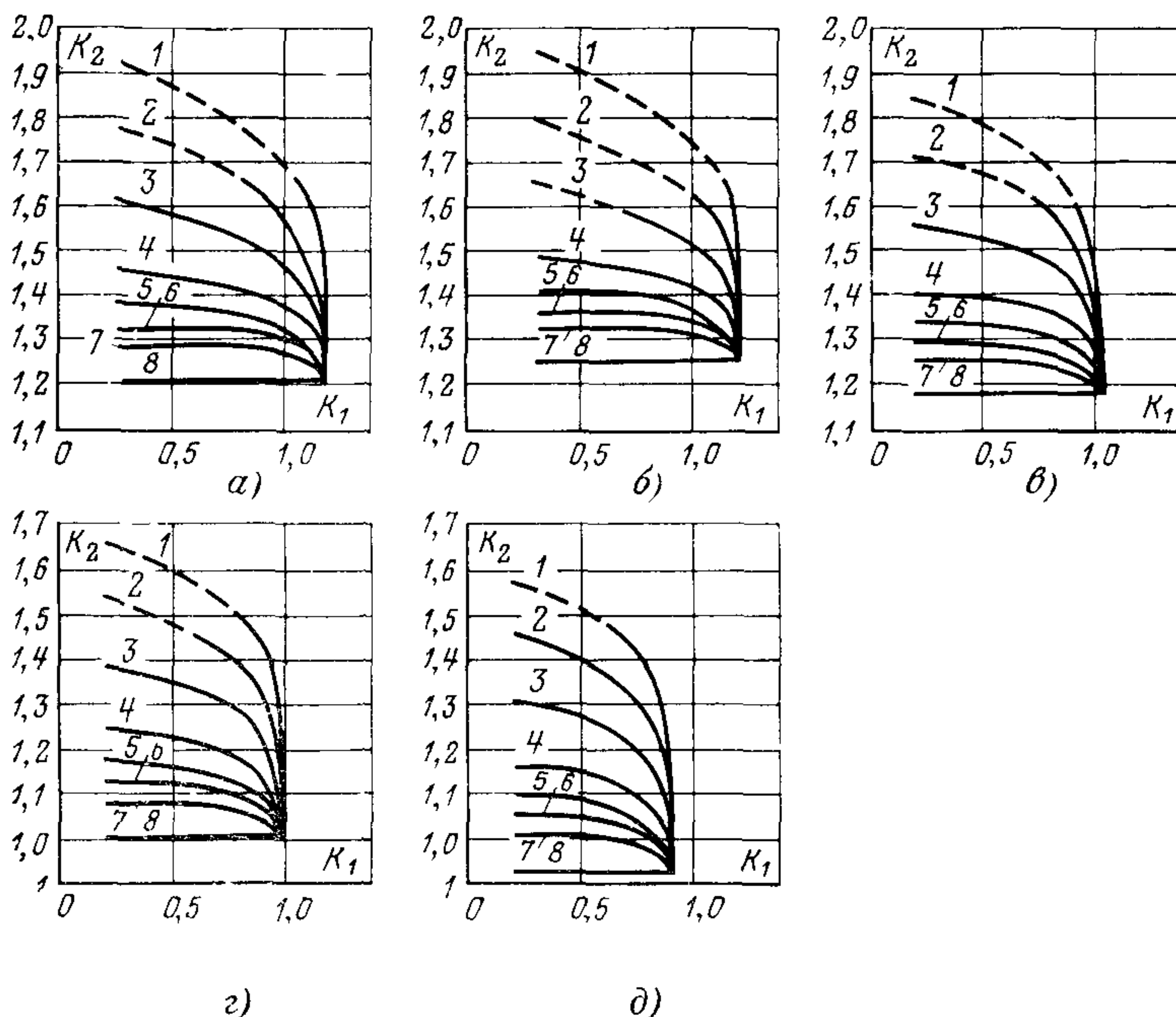
Рис. 2.3. Графики нагрузочной способности масляных трансформаторов с охлаждением ДЦ и Ц при эквивалентной температуре, °С. а — \vartheta_{\text{ср}} = -10 ; б — при \vartheta_{\text{ср}} = 0 , в — при \vartheta_{\text{ср}} = 10 ; г — при \vartheta_{\text{ср}} = 20 , д — при \vartheta_{\text{ср}} = 30 . Остальные обозначения см на рис 2.
