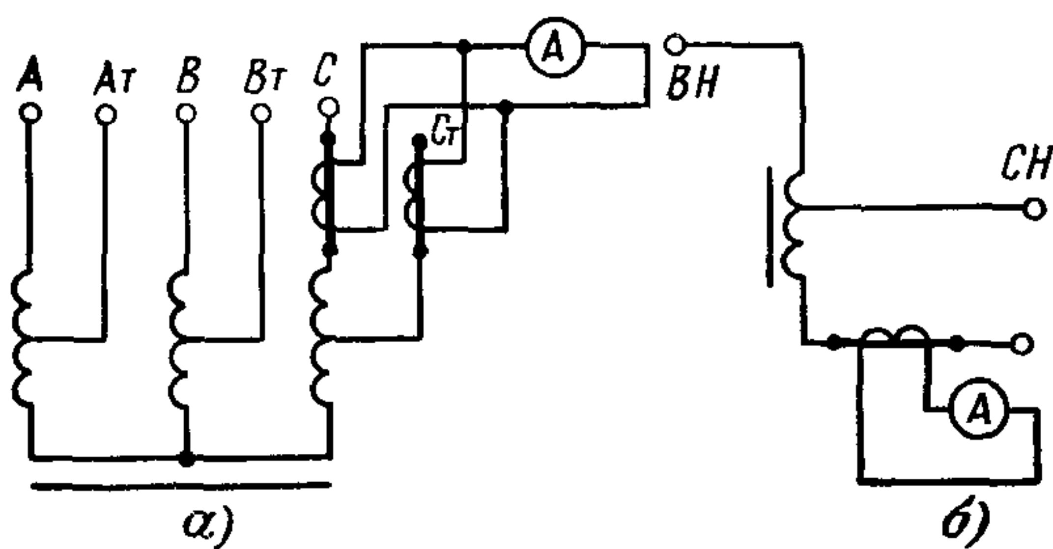
Рис. ПЗ.1. Схема включения амперметра для измерения тока в общей части обмотки автотрансформатора. а — трехфазного; б — однофазного.
