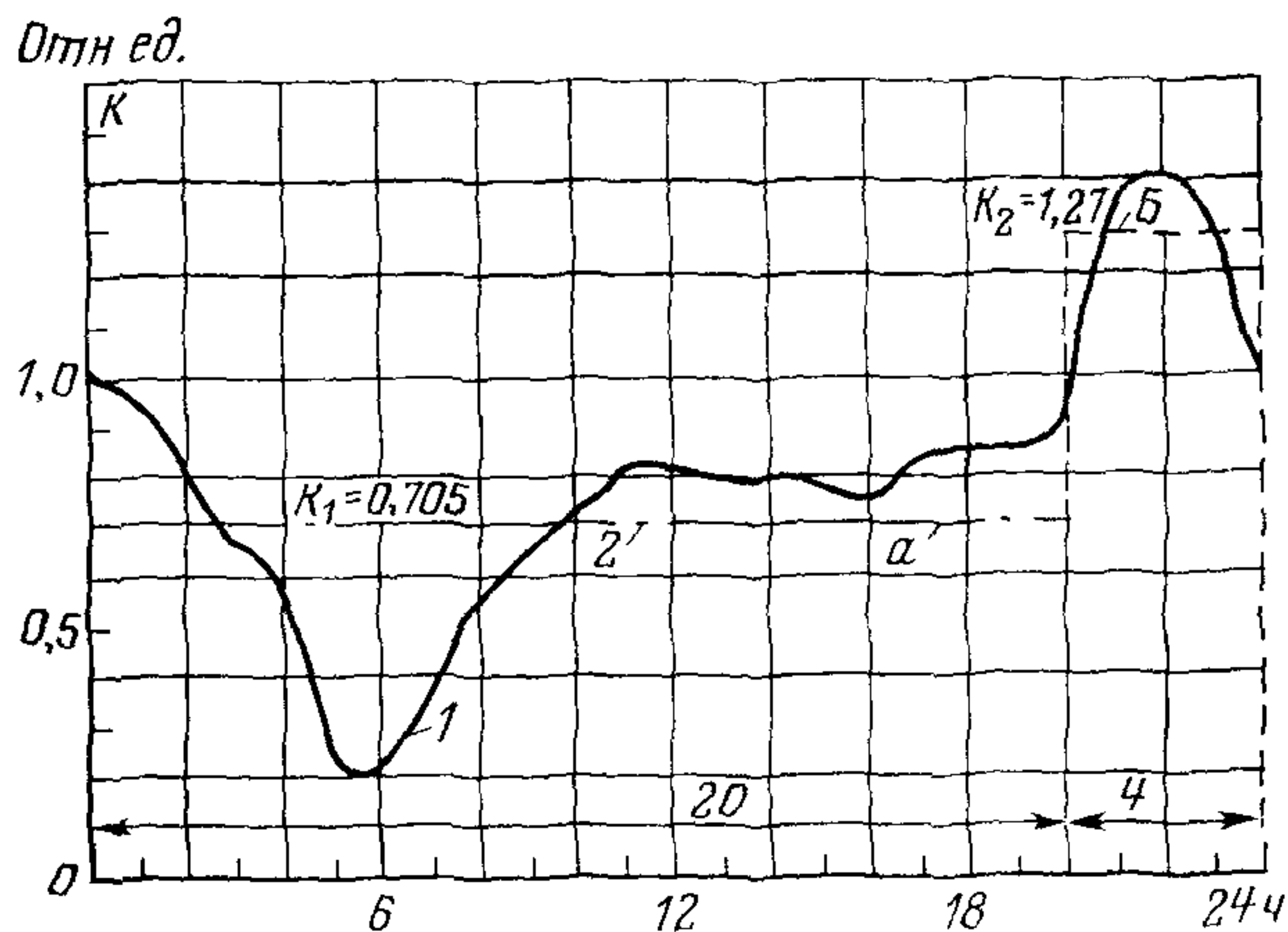
Рис. 2.1. Графики нагрузки
