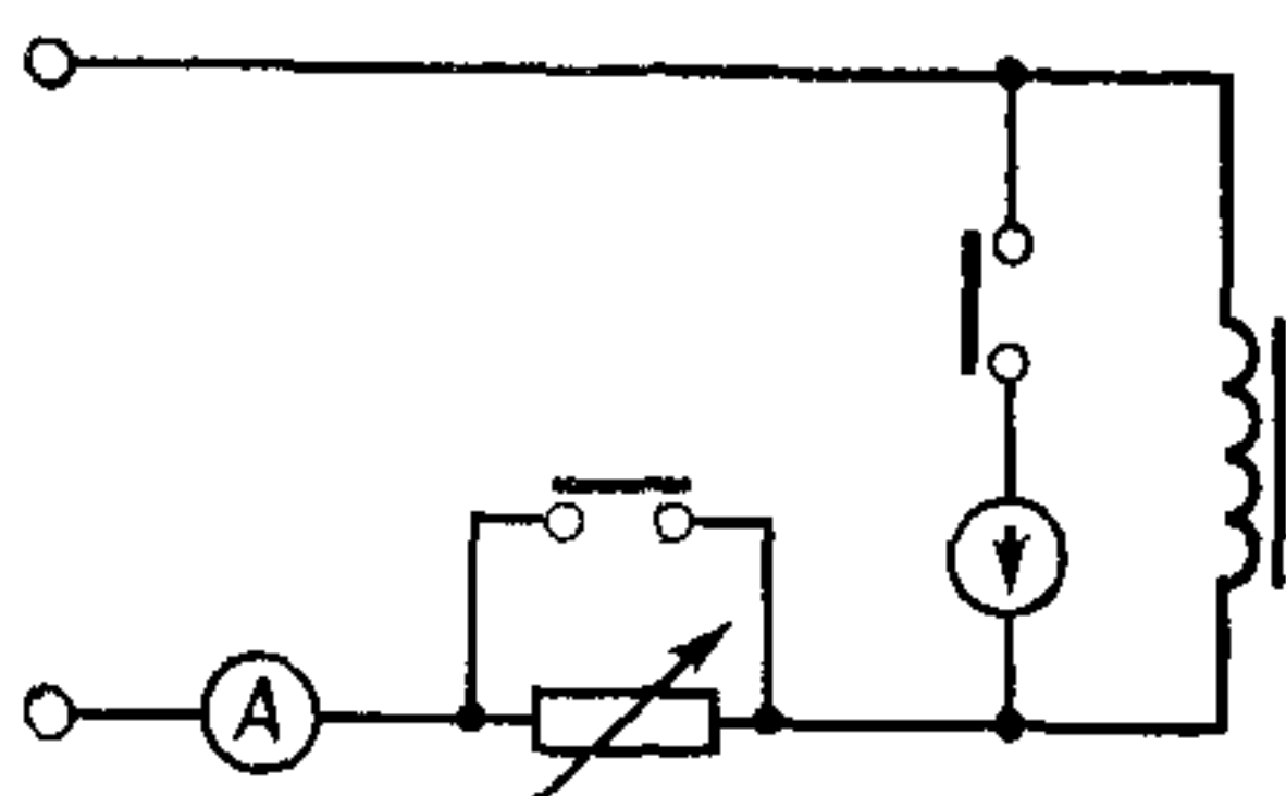
Рис. П6.1. Схема для измерения сопротивления обмотки трансформатора по методу падения напряжения.
