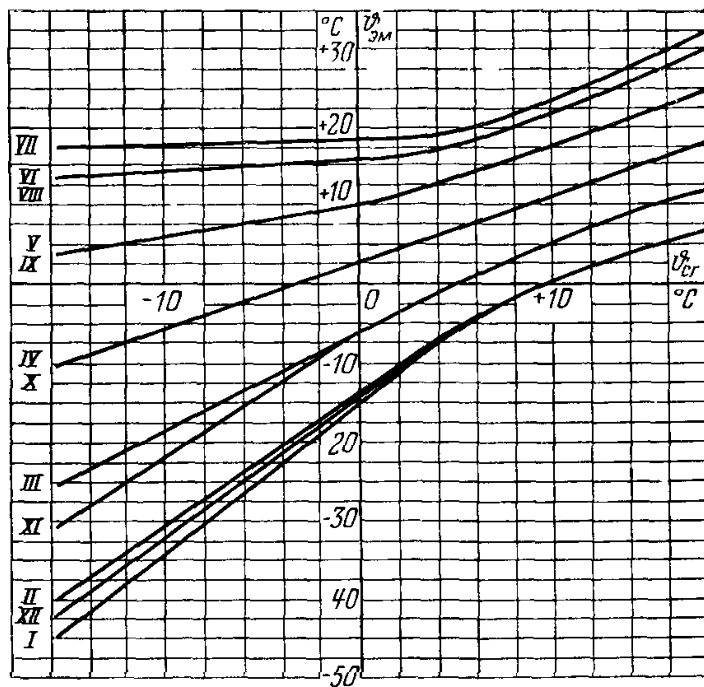
Рис. 2.5 Кривые зависимости эквивалентных месячных температур t_{э.м.} от среднегодовой температуры t_{ср.} . I—XII — месяцы года.
