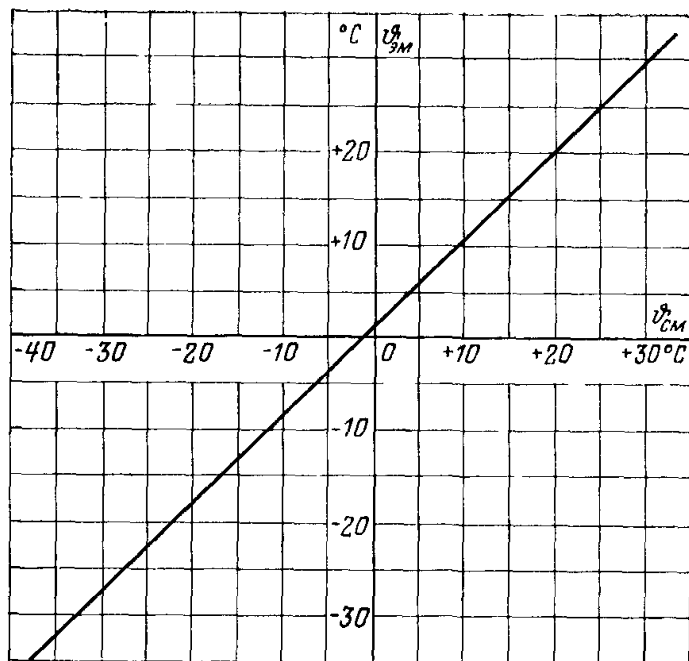
Рис. 2.6 Зависимость эквивалентных месячных температур t_{э.м.} от среднемесячных.
