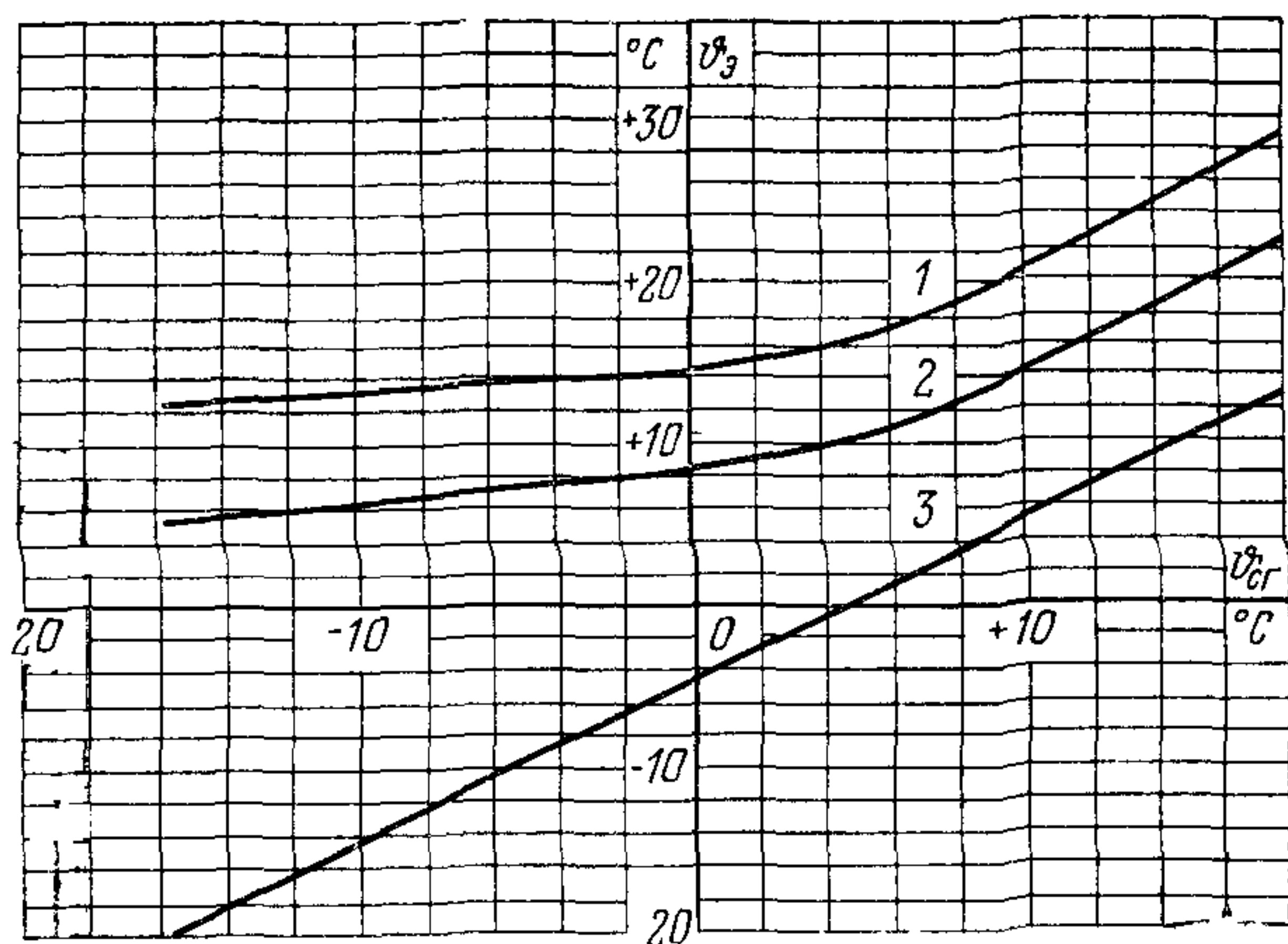
Рис 24 Кривые зависимости эквивалентных температур \theta_{э} от среднегодовой температуры \theta_{сг} .
