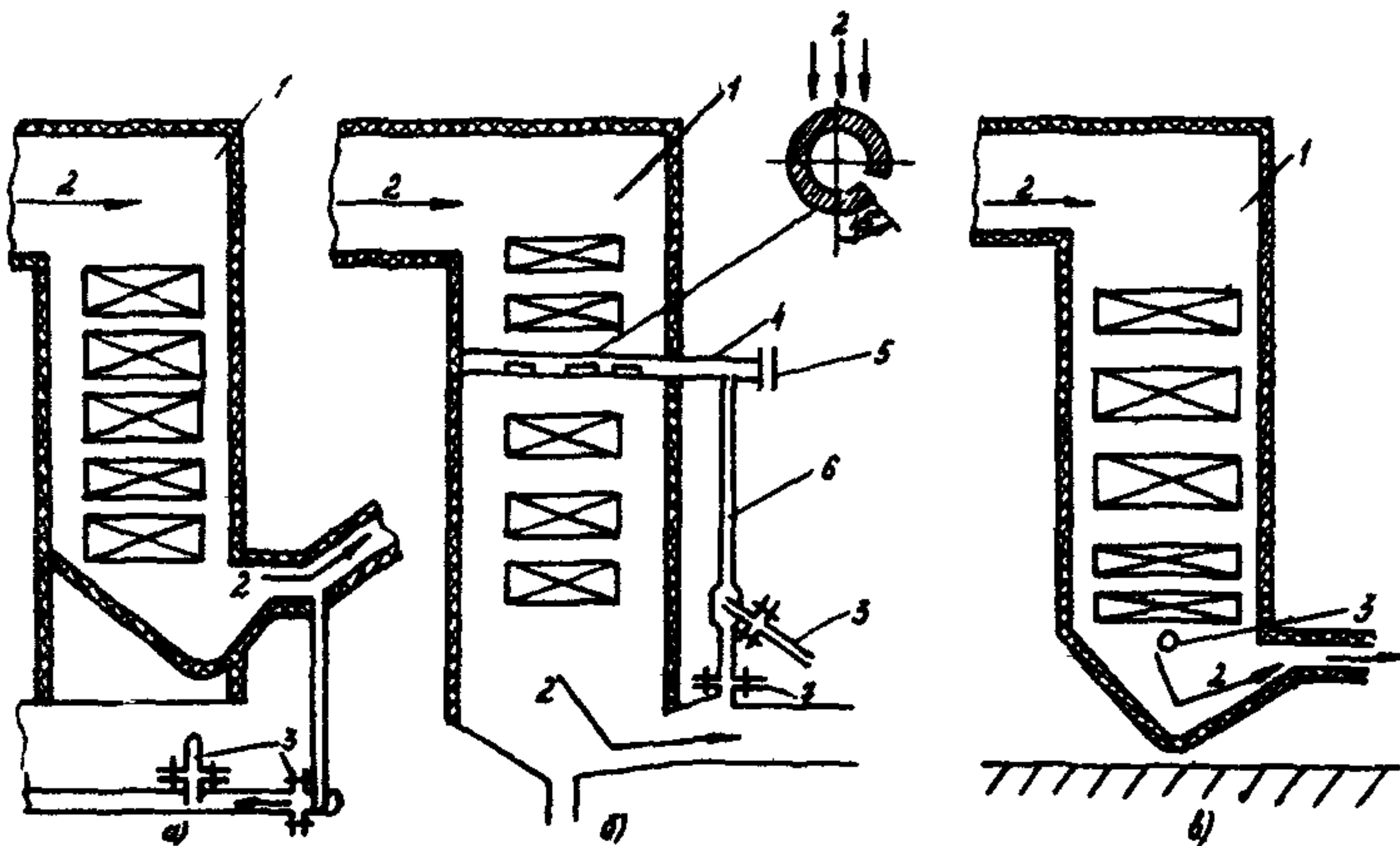
Отбор пробы дымовых газов
