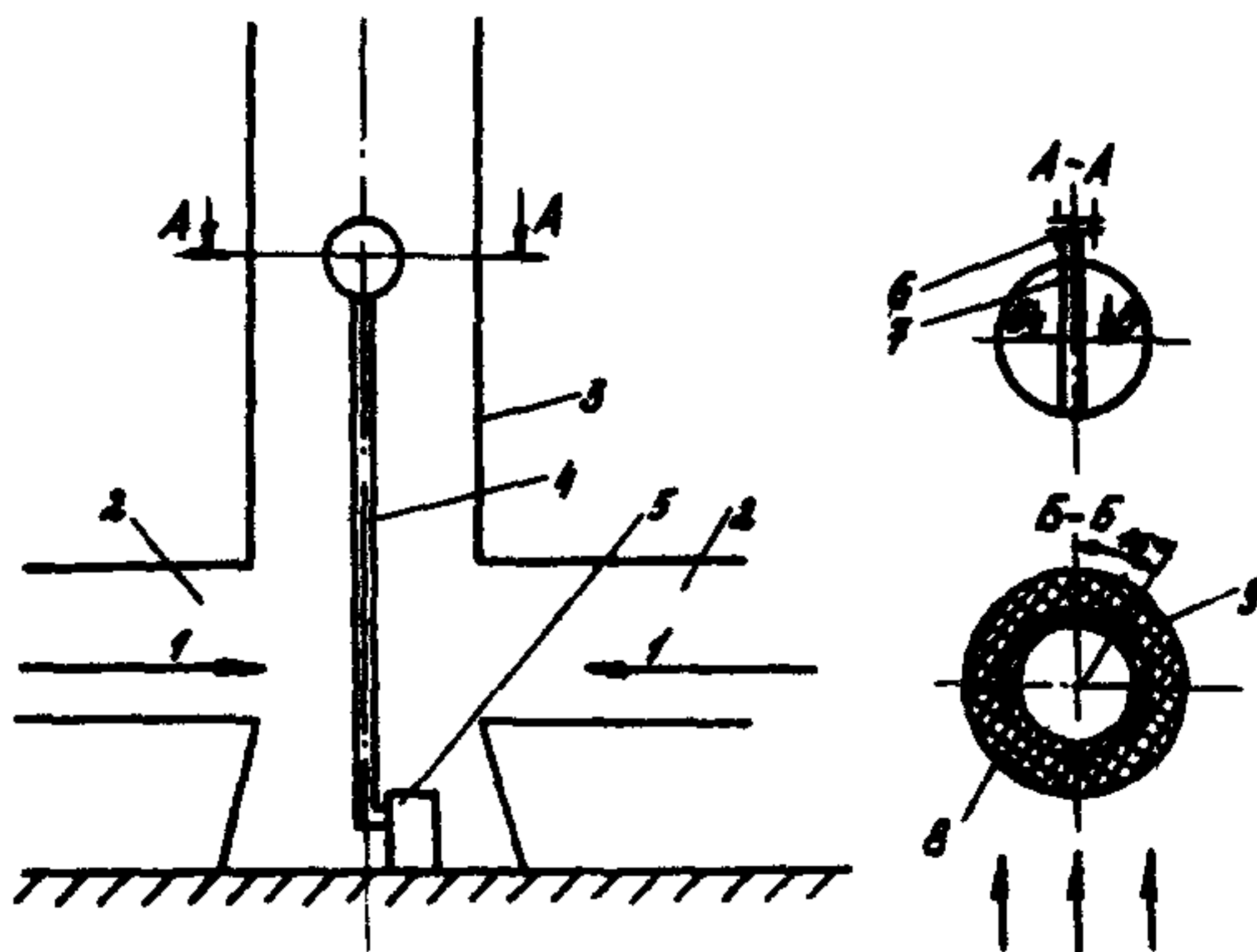
Отбор пробы из дымовой трубы
