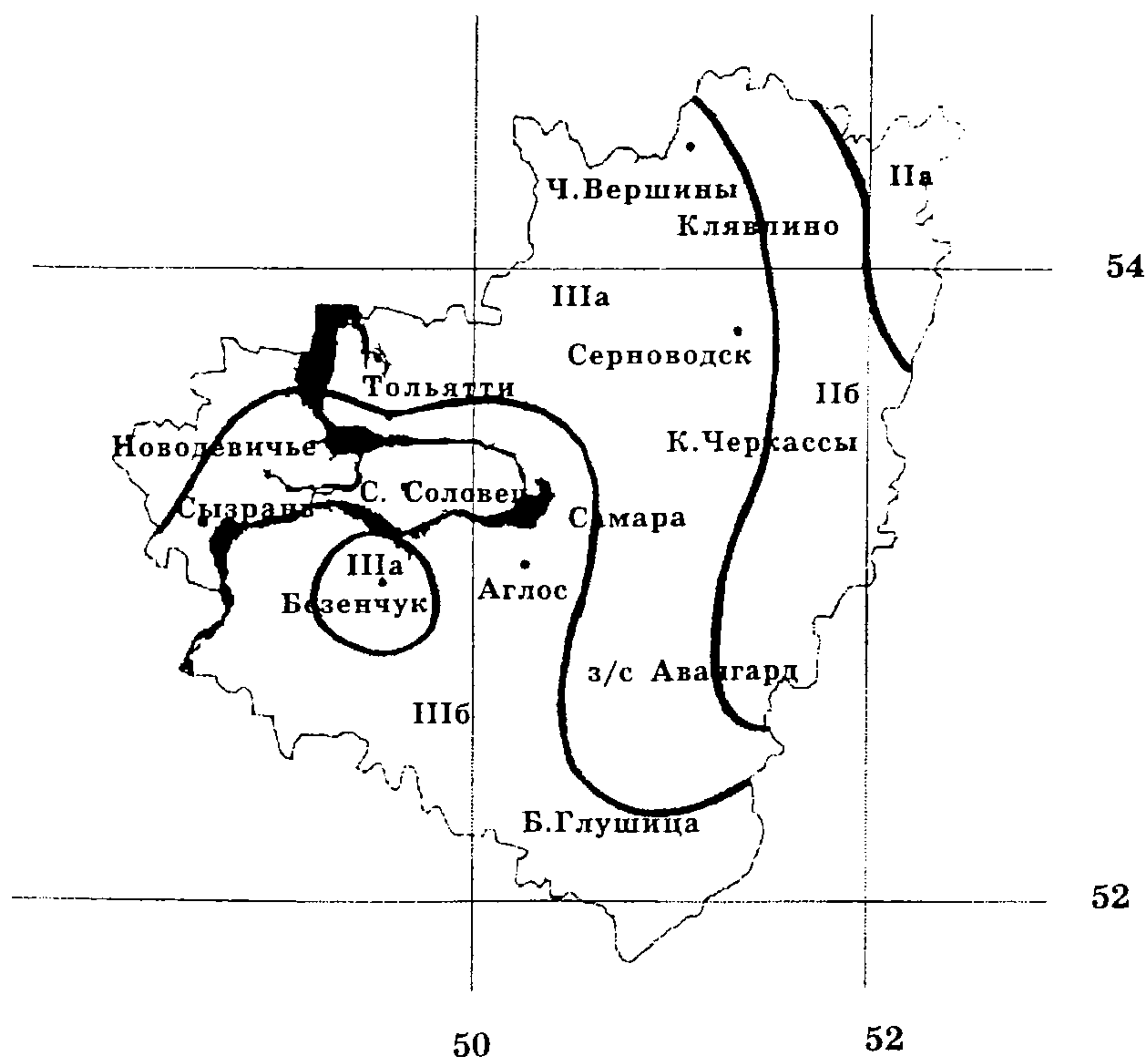
Рис. 5. Схематическая карта дорожно-климатического районирования (рекомендуемая).
