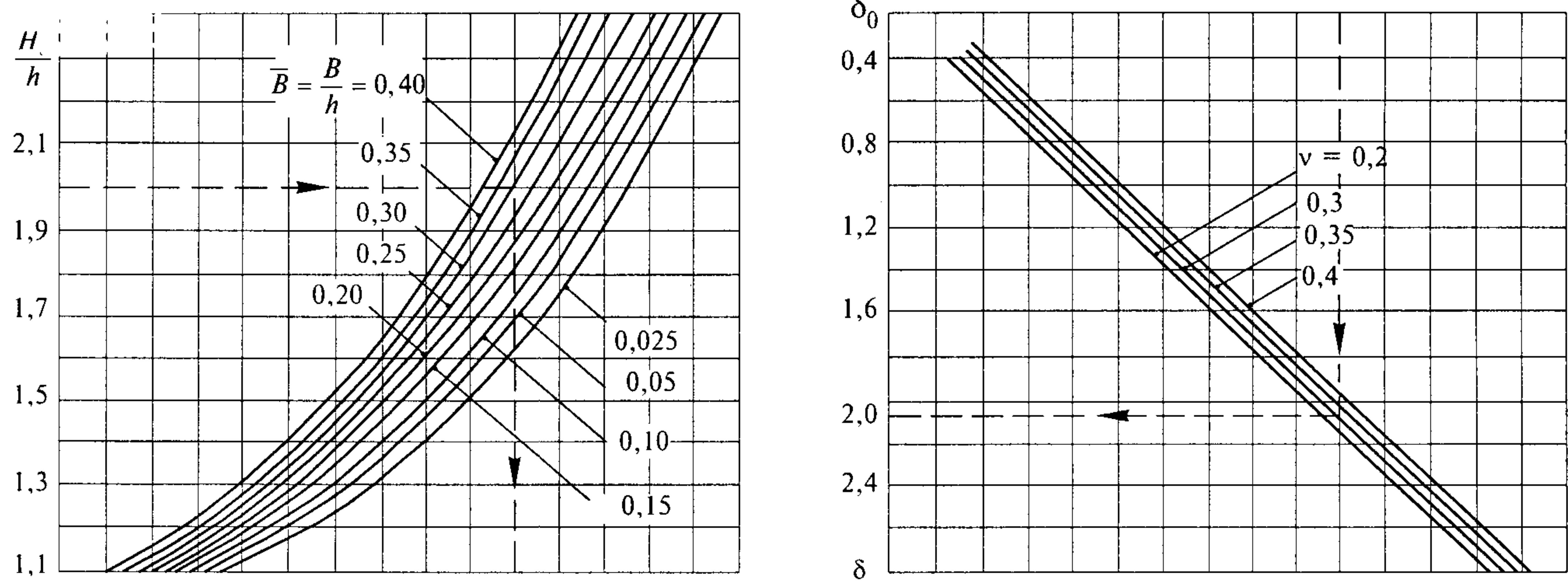
Рисунок Ж.1 — Номограмма для определения значений \delta_0
