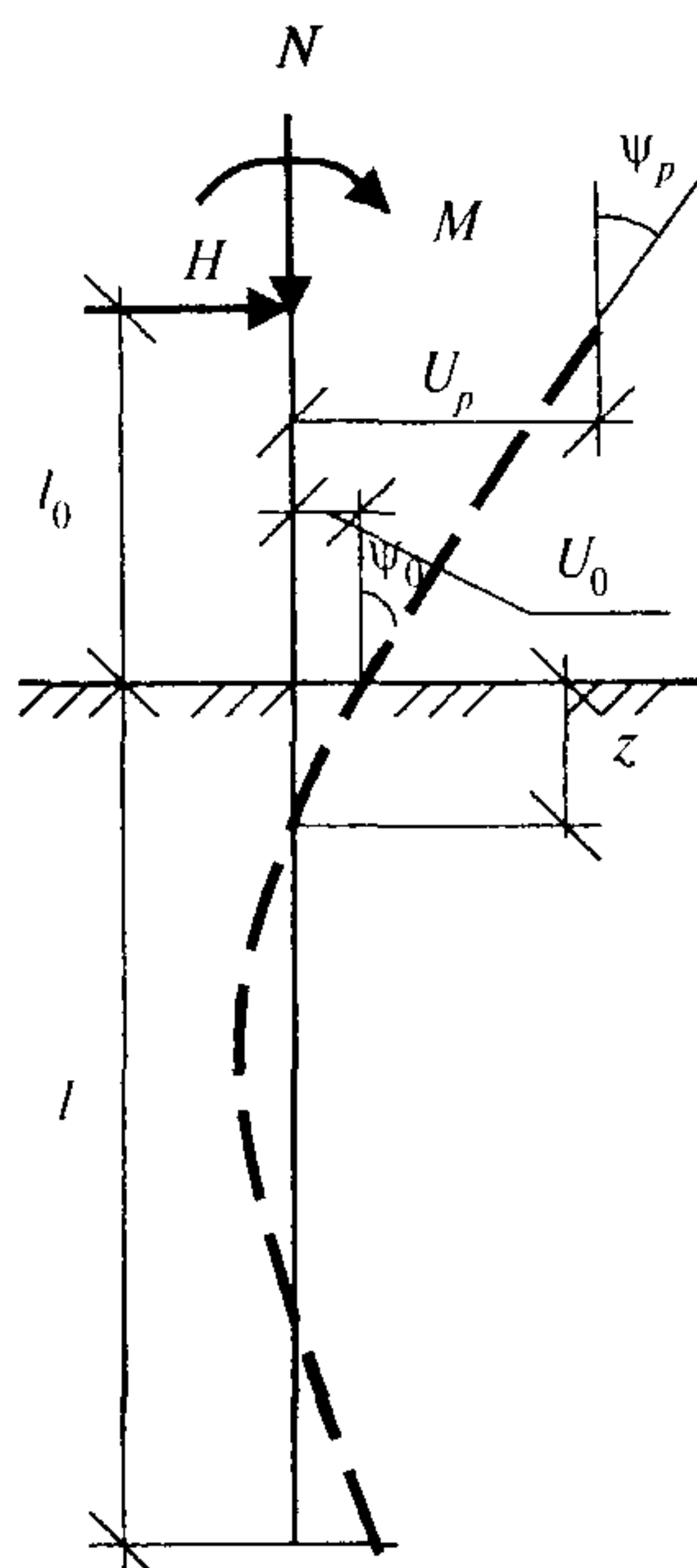
Рисунок Д.1 — Схема нагрузок на сваю
