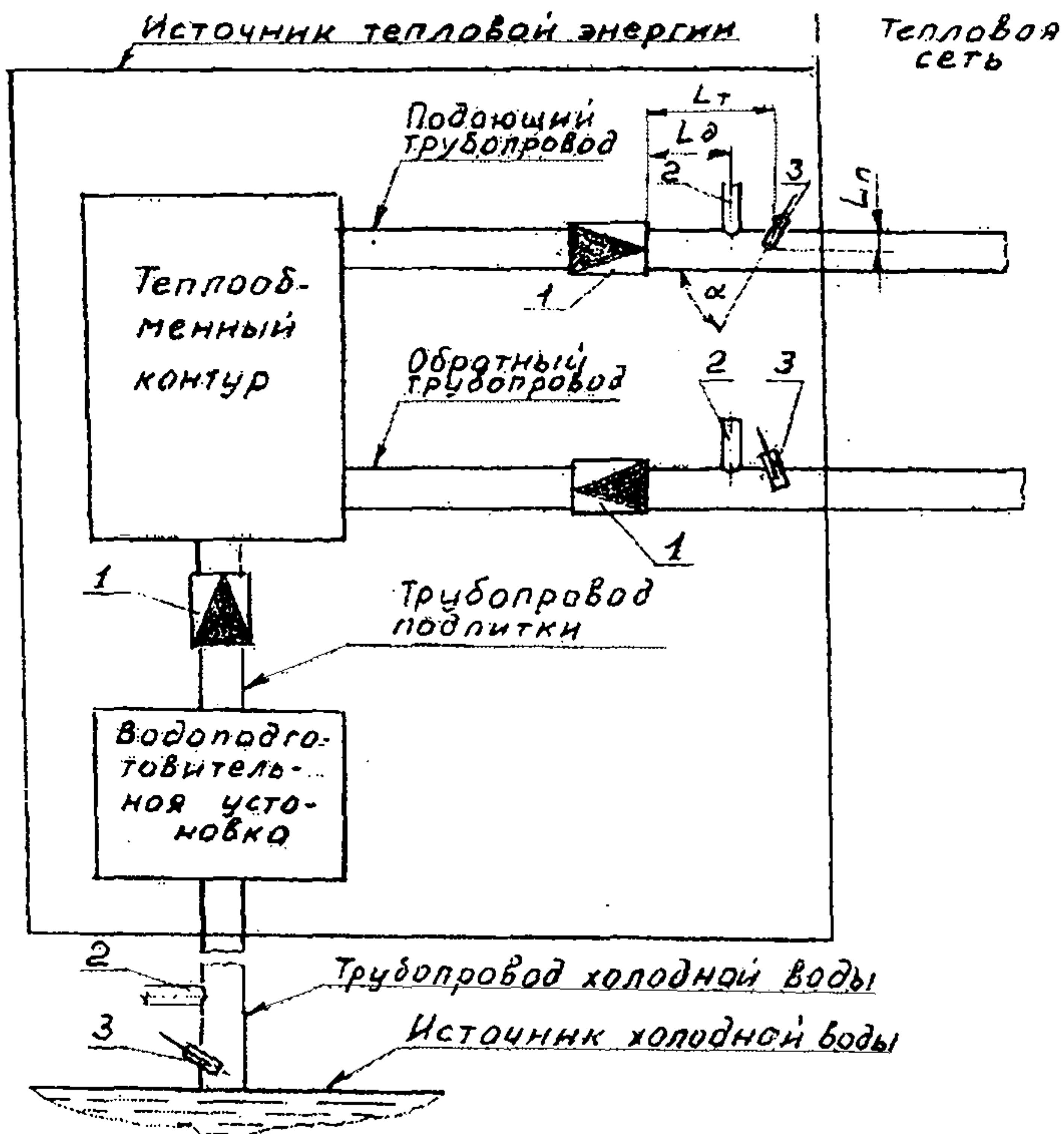
Б.1 Схема расположения первичных преобразователей на источнике тепловой энергии
