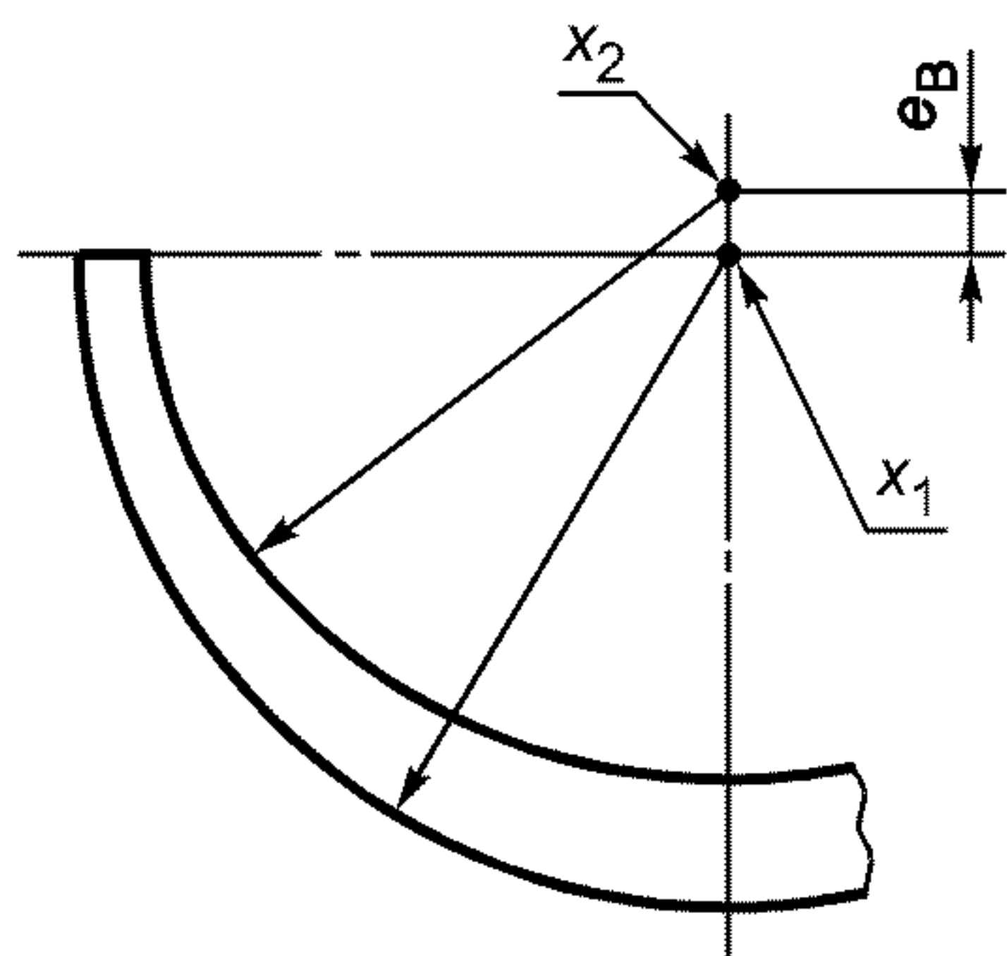
Рисунок 3 — Эксцентрическое отверстие тонкостенного гладкого или буртового вкладыша
