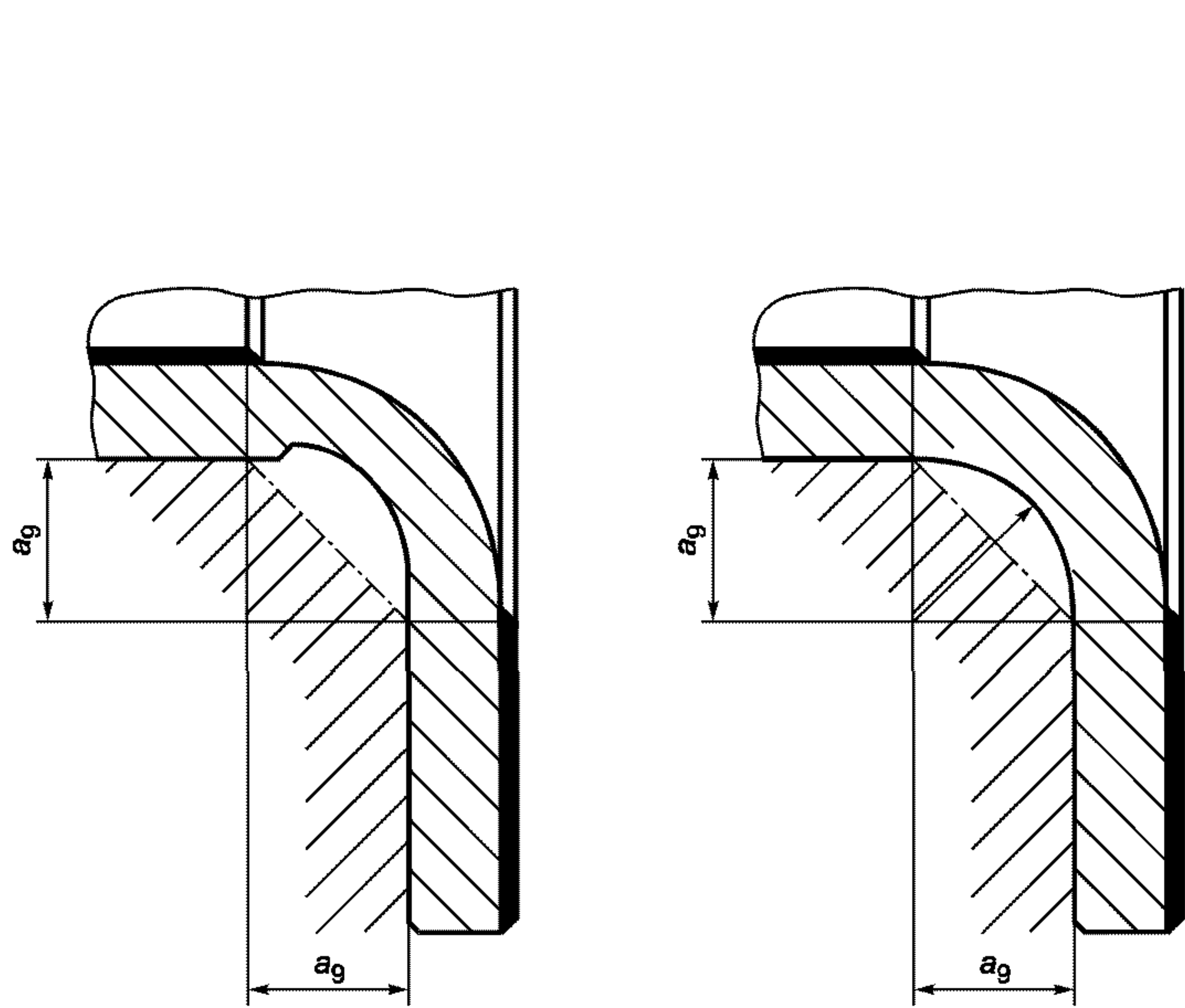
Рисунок 11 — Типы зоны перехода между радиальными частями
