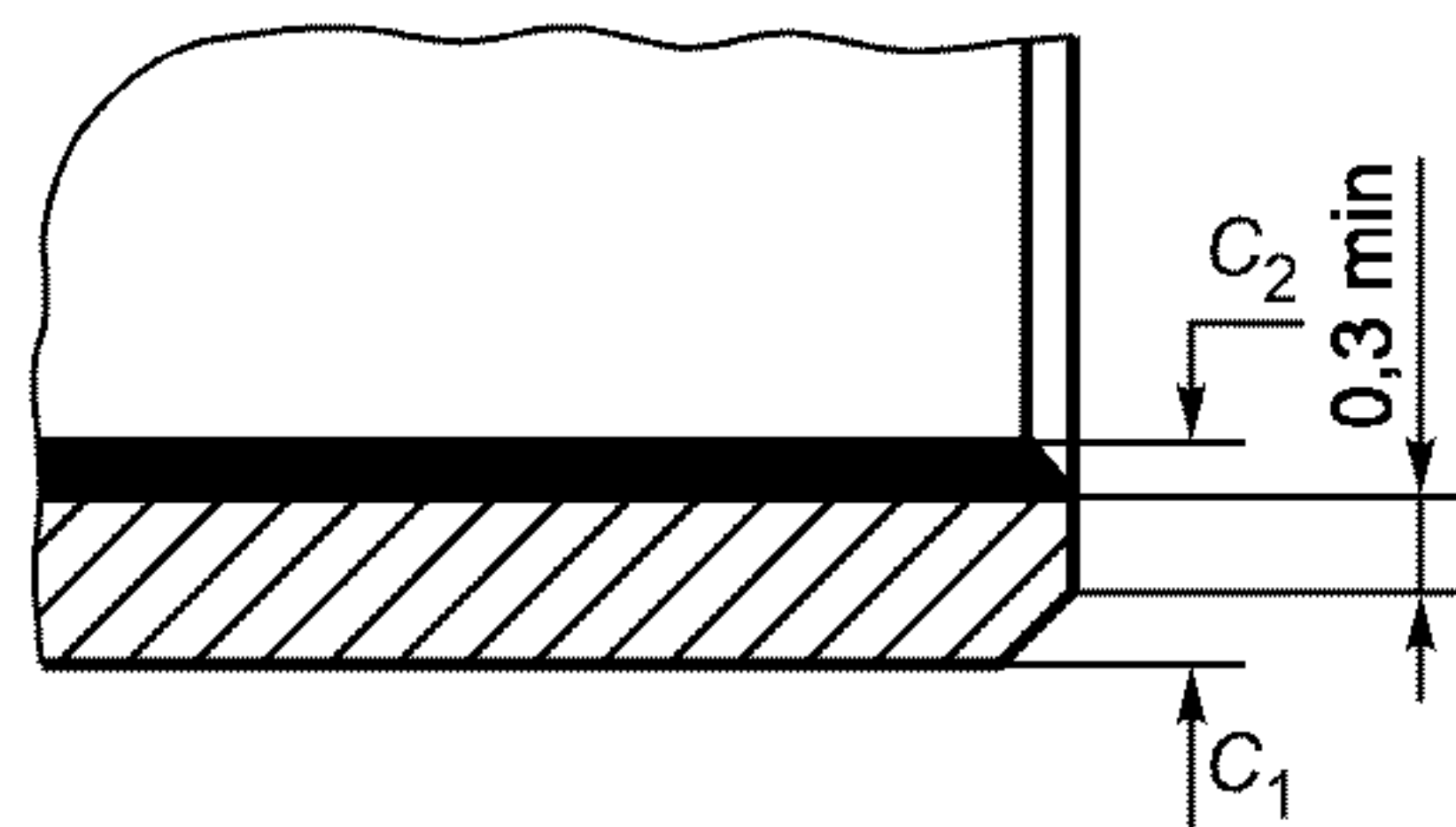
Рисунок 9 — Фаски
