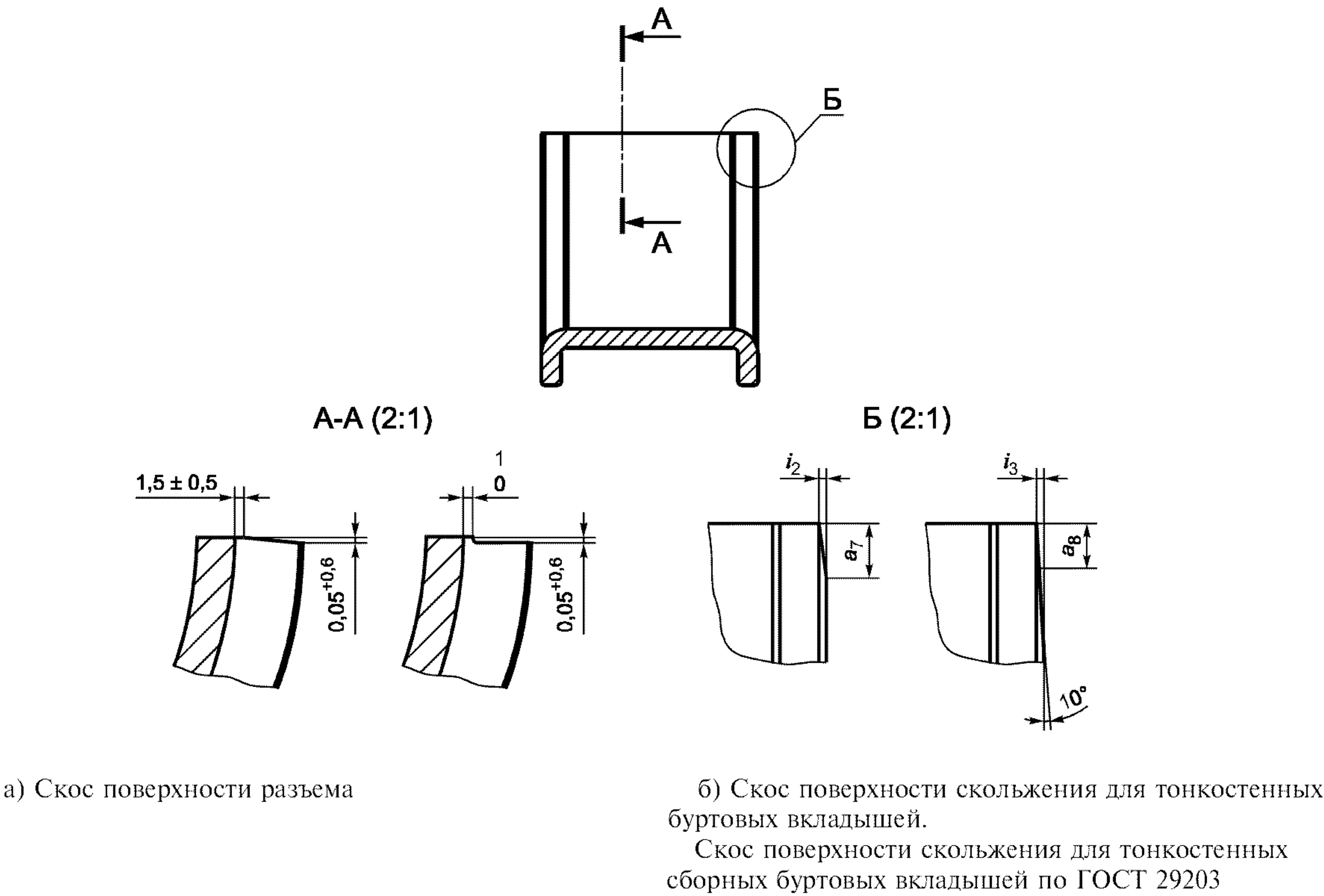
Рисунок 10 — Скосы бурта (конструкция по выбору изготовителя)
