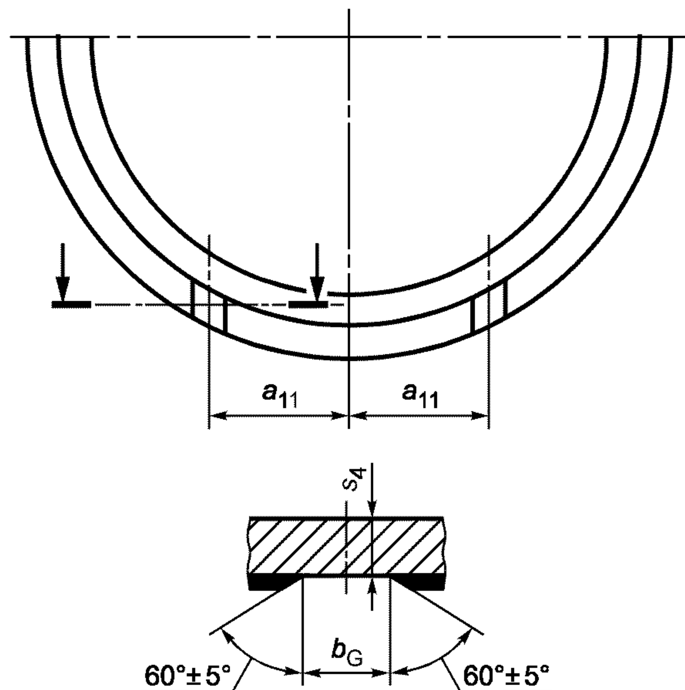
Рисунок 16 — Форма канавки на поверхности бурта
