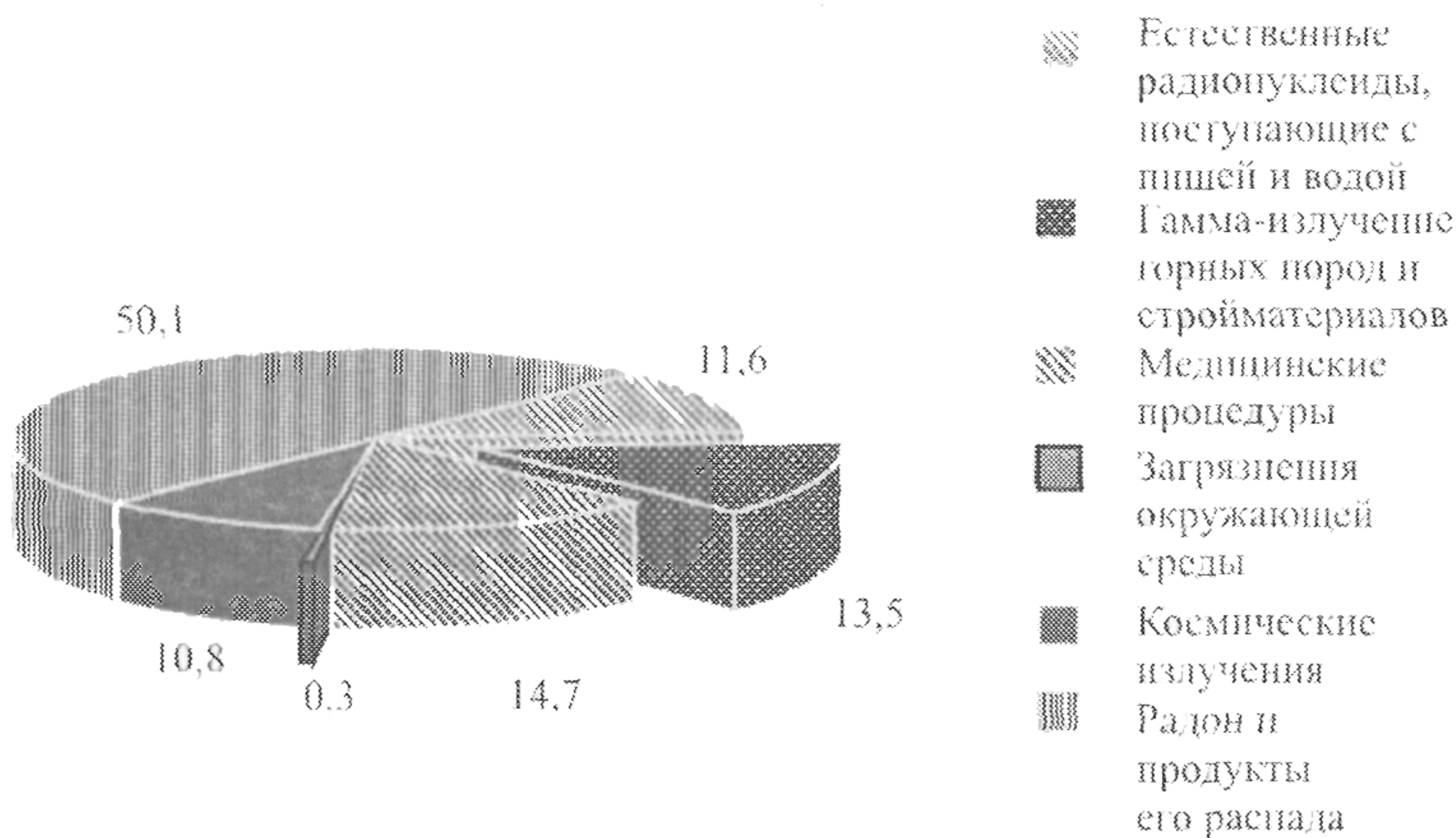
Рис. 3. Структура формирования эффективной дозы облучения
