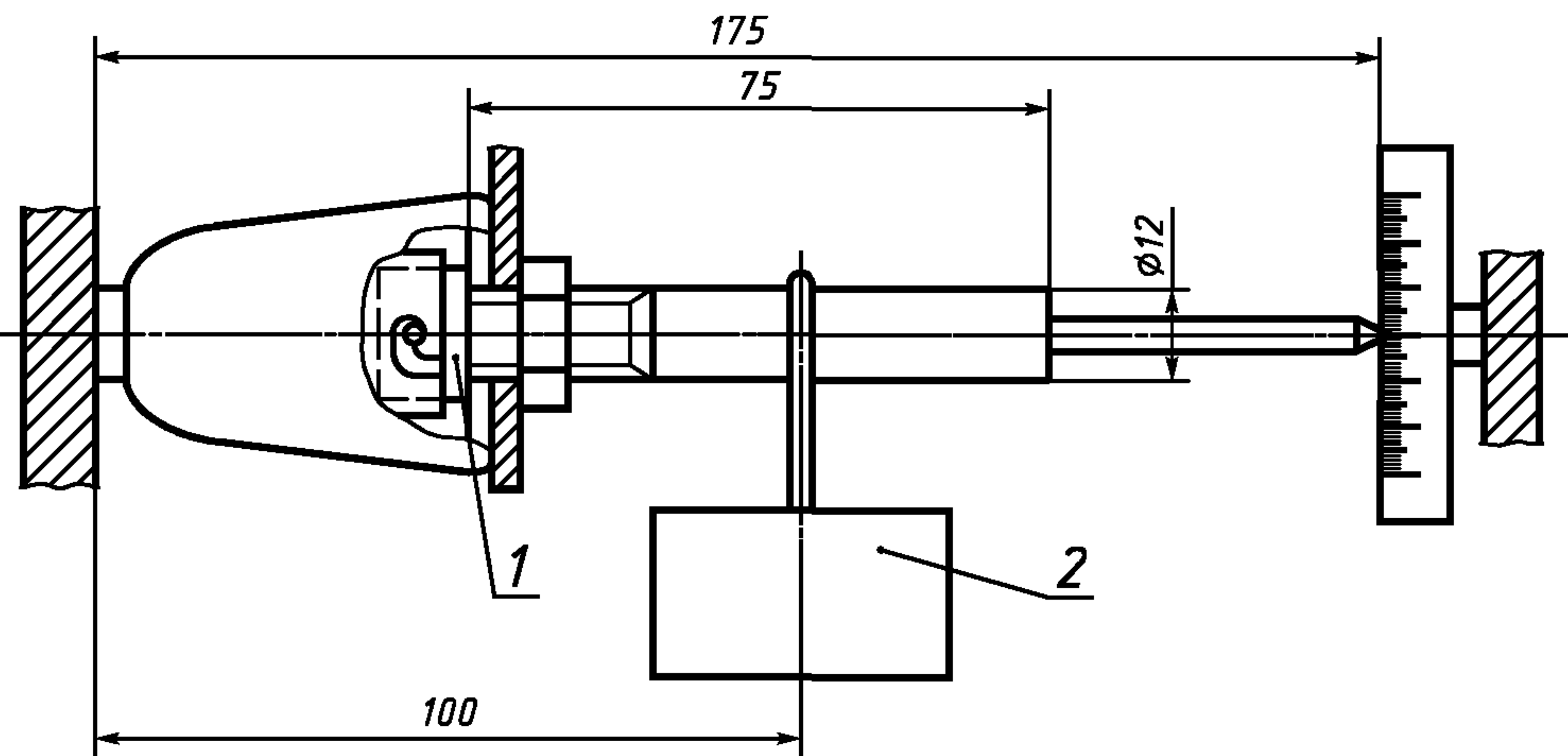
1 — испытательный цокль; 2 — груз G
