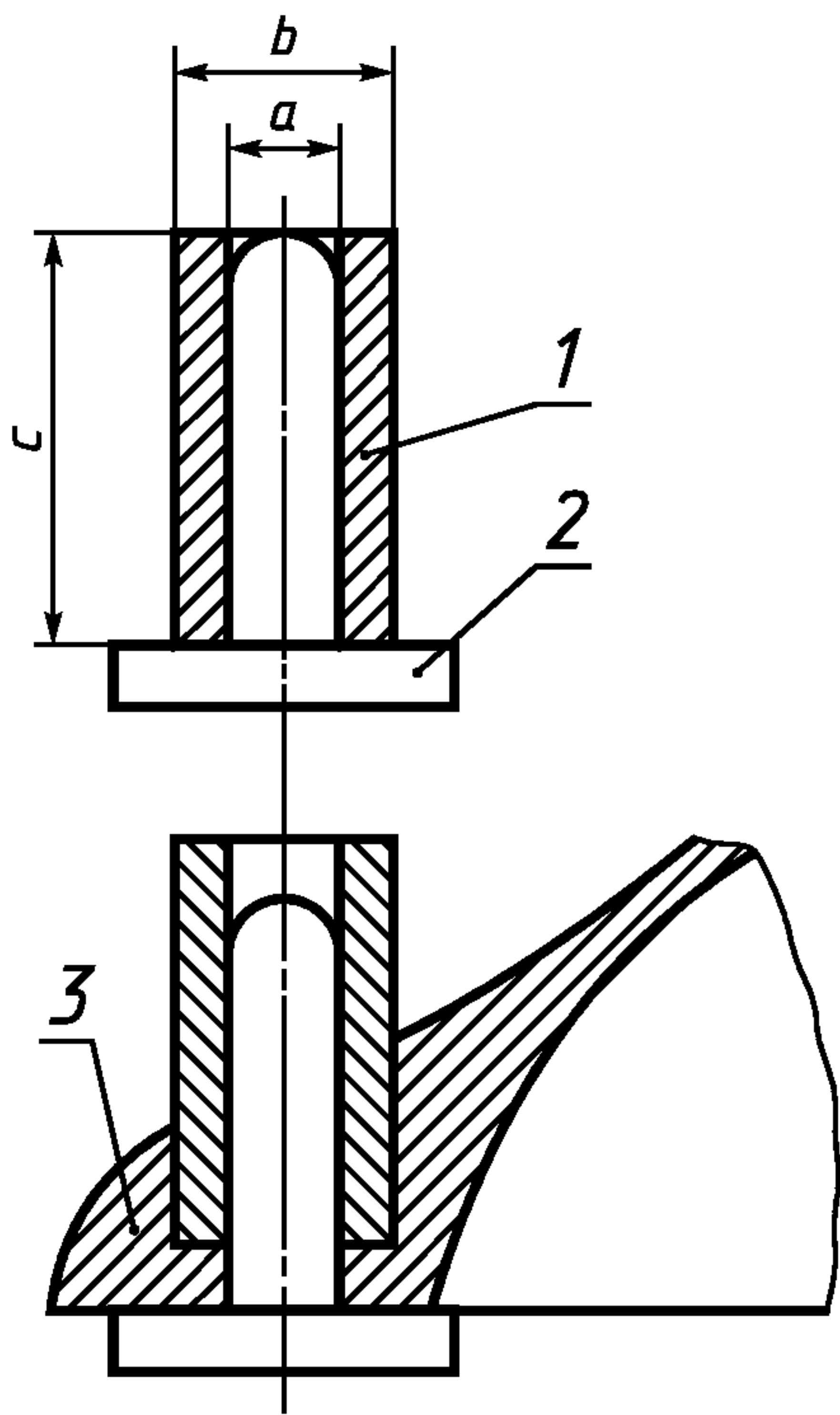
1 — втулка; 2 — вилка; 3 — основание
