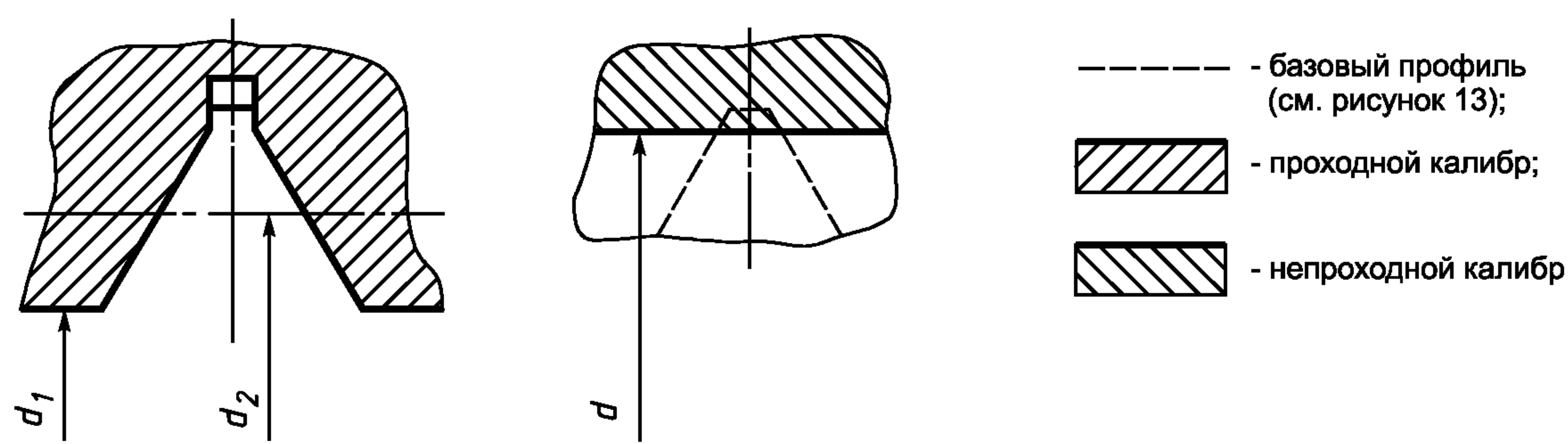
Калибры для винта
