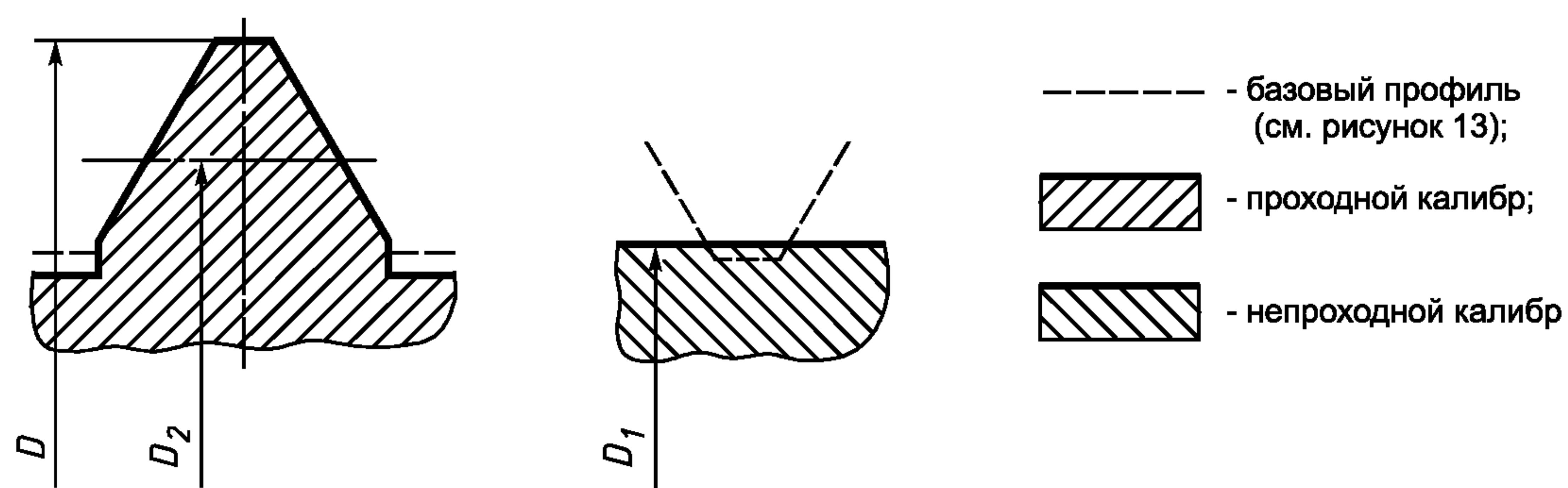
Калибры для гайки
