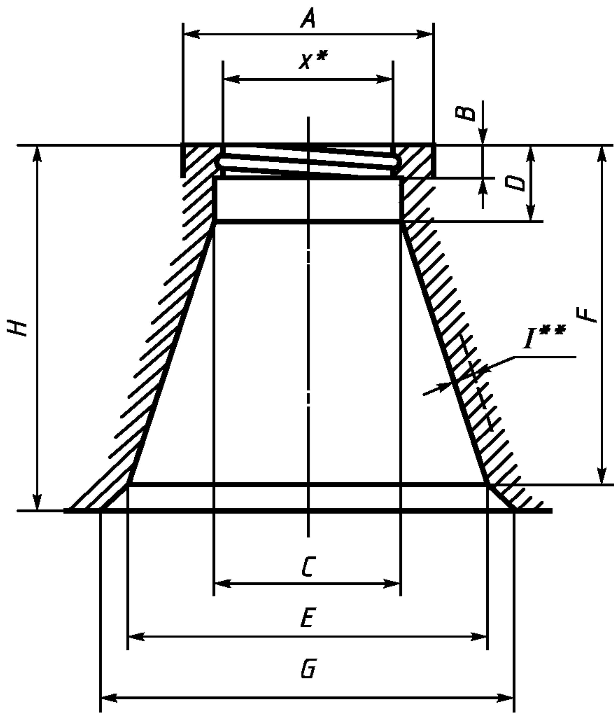
Рисунок 8 — Размеры устройства для крепления абажура (см. 8.1)
