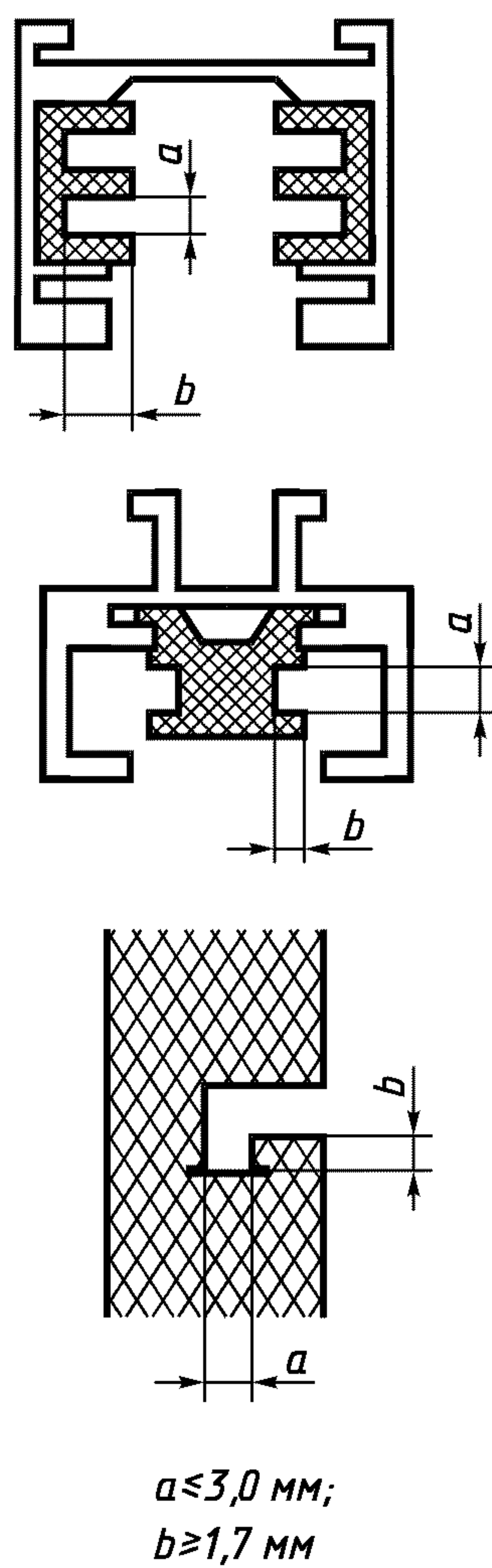
Рисунок 4 — Измеряемые места типичных секций шинопроводов класса I
