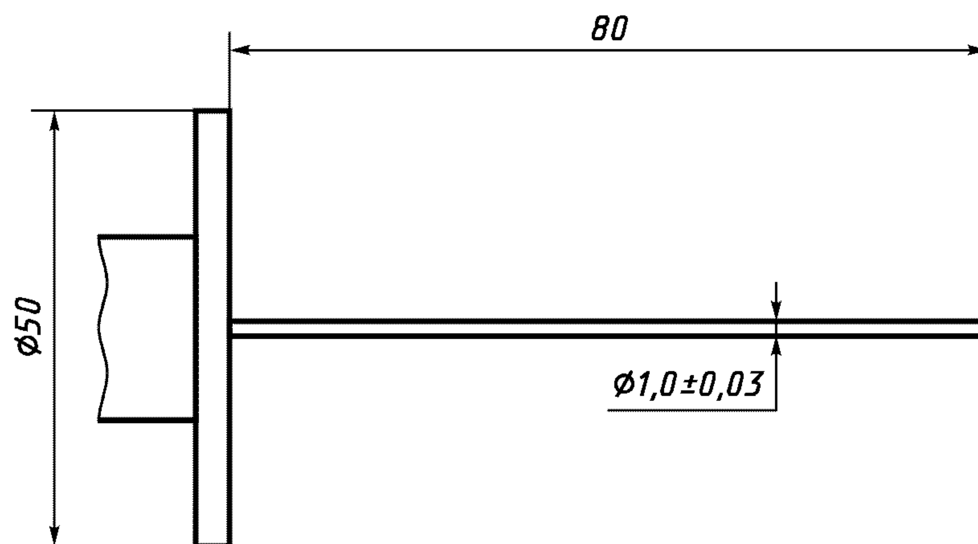
Рисунок 2 — Испытательный щуп
