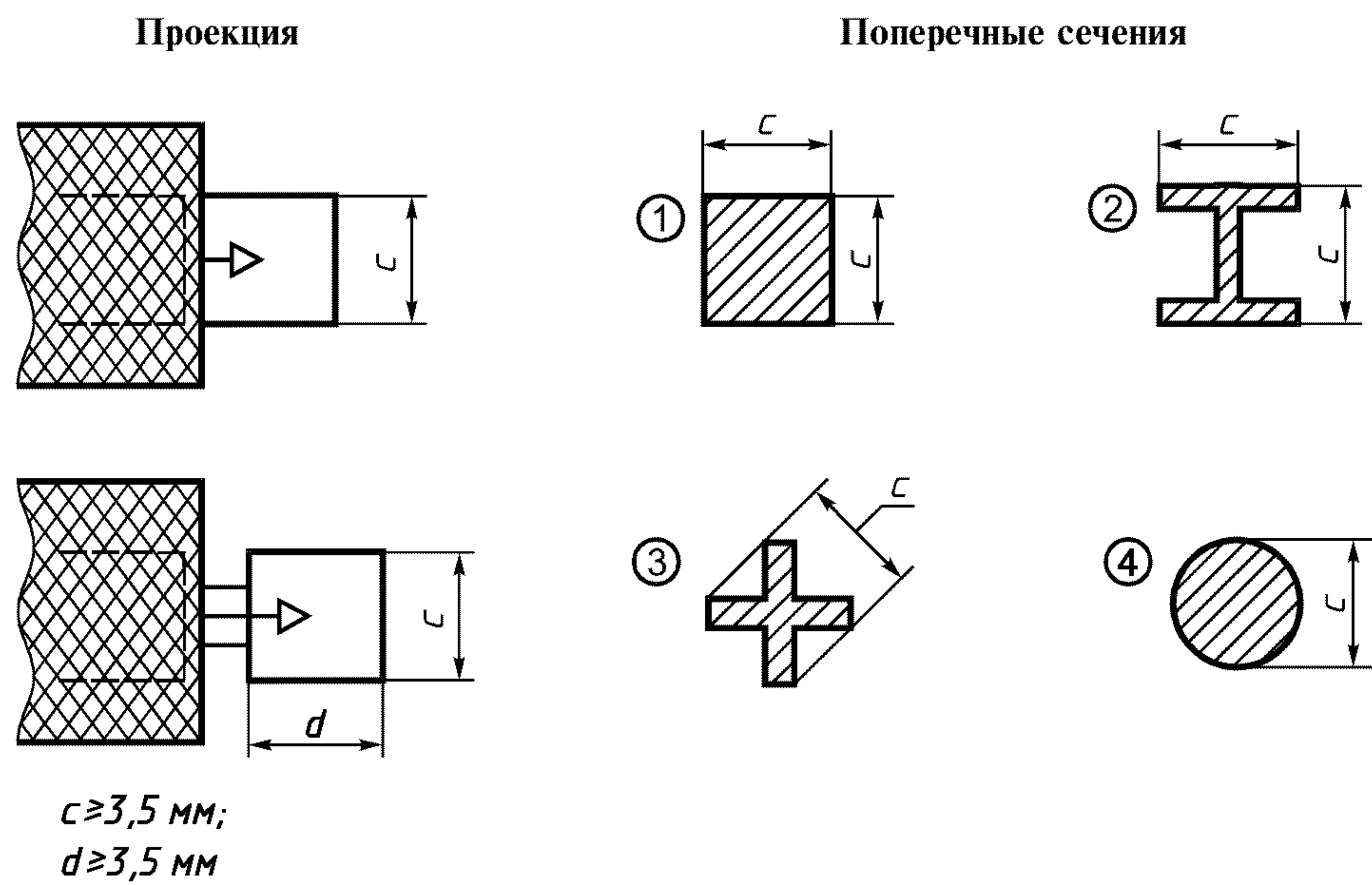
Рисунок 3 — Измеряемые места типичных контактов адаптеров класса III
