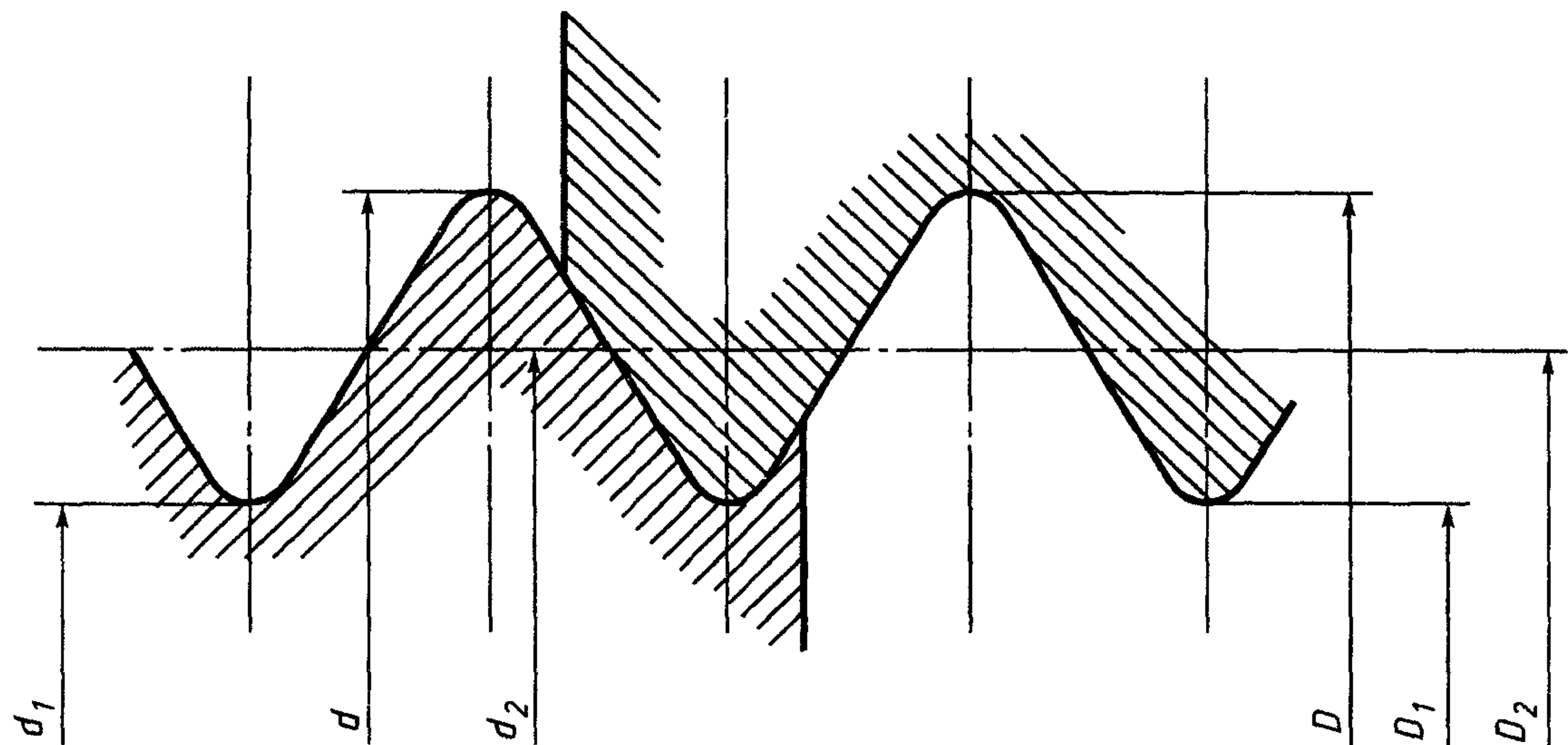
Предельный профиль винта
