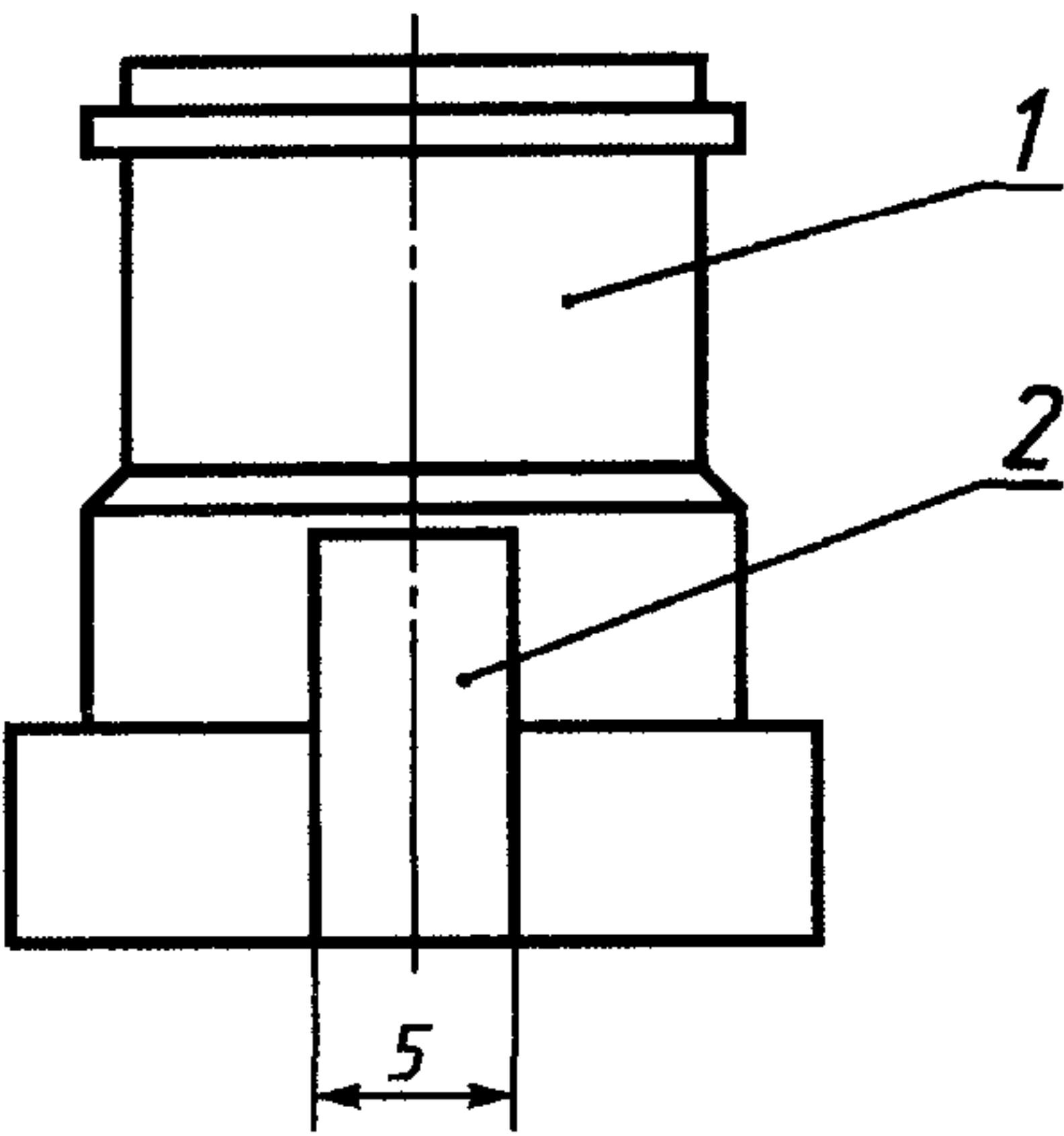
1 — образец; 2 — паз (щель)
