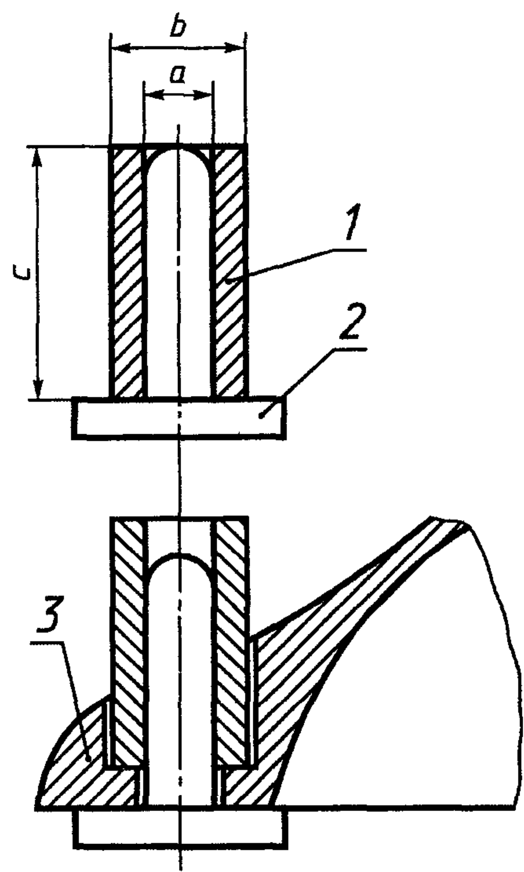
1 — втулка; 2 — штырь; 3 — фланец
