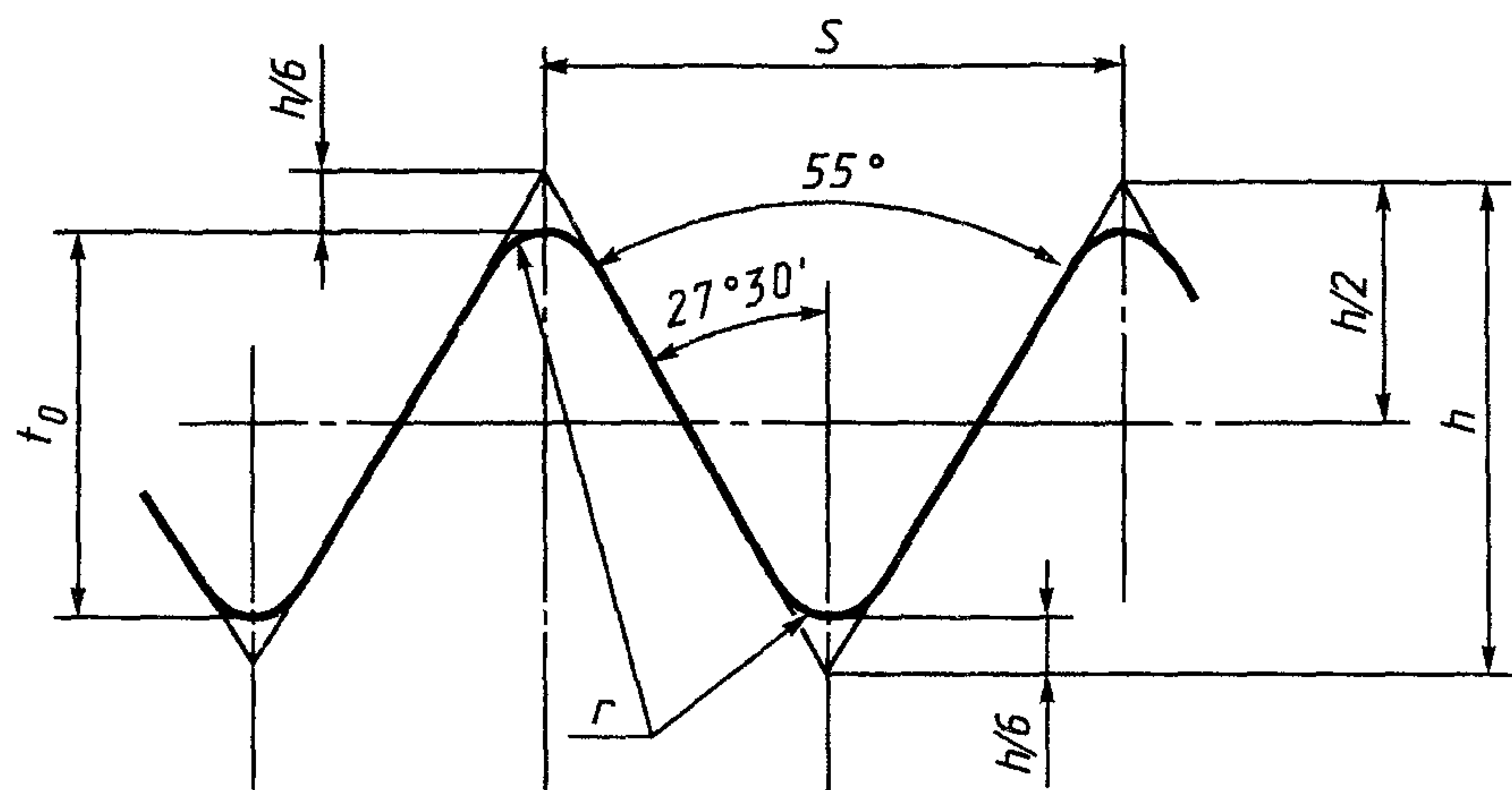
Трубная резьба ИСО
