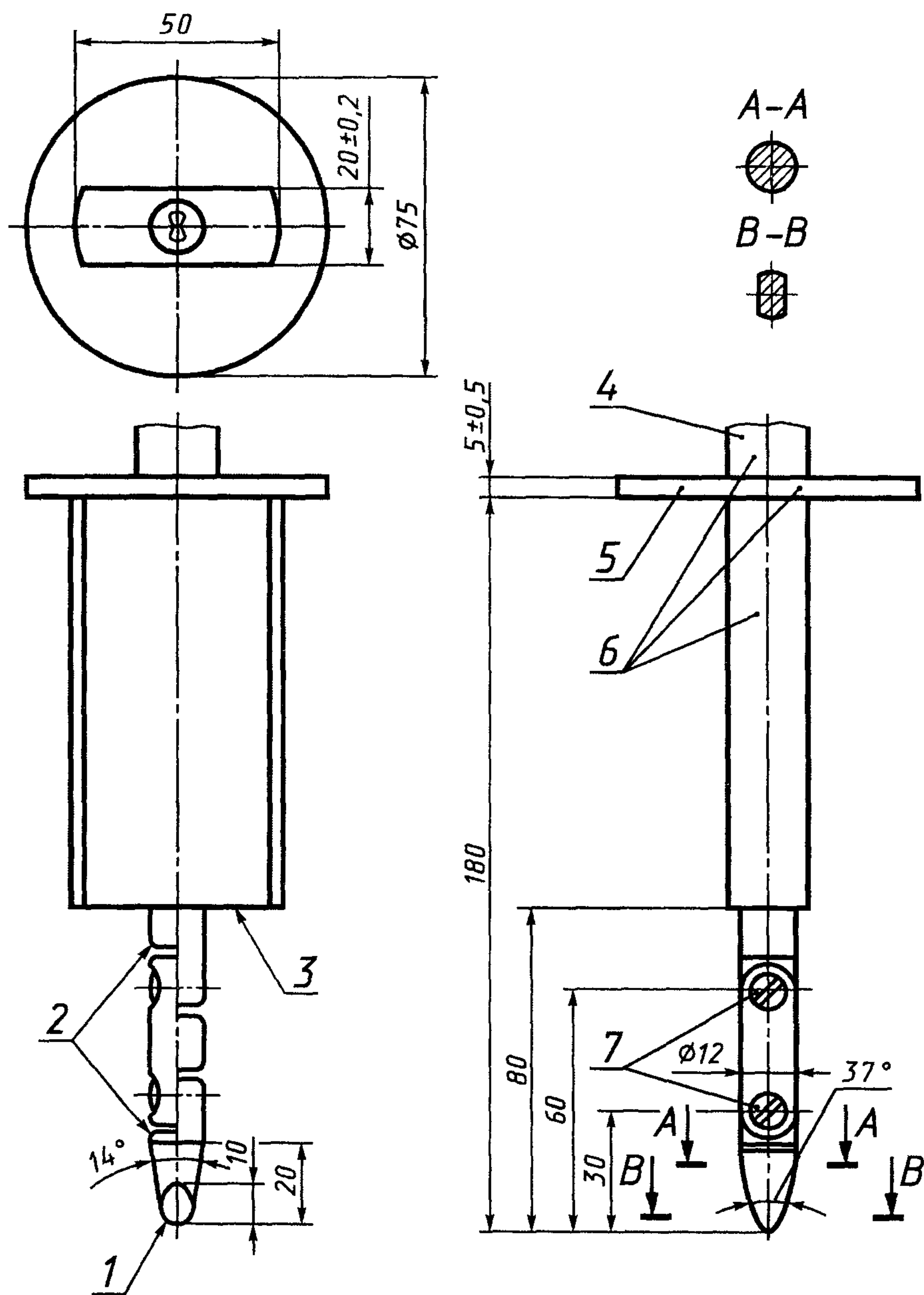
1 — сферическая поверхность R4 \pm 0,05 ; 2 — скруглить все края; 3 — ограничивающая поверхность; 4 — рукоятка; 5 — предохранитель; 6 — изолирующий материал; 7 — шарниры; 8 — цилиндрическая поверхность R2 \pm 0,05
