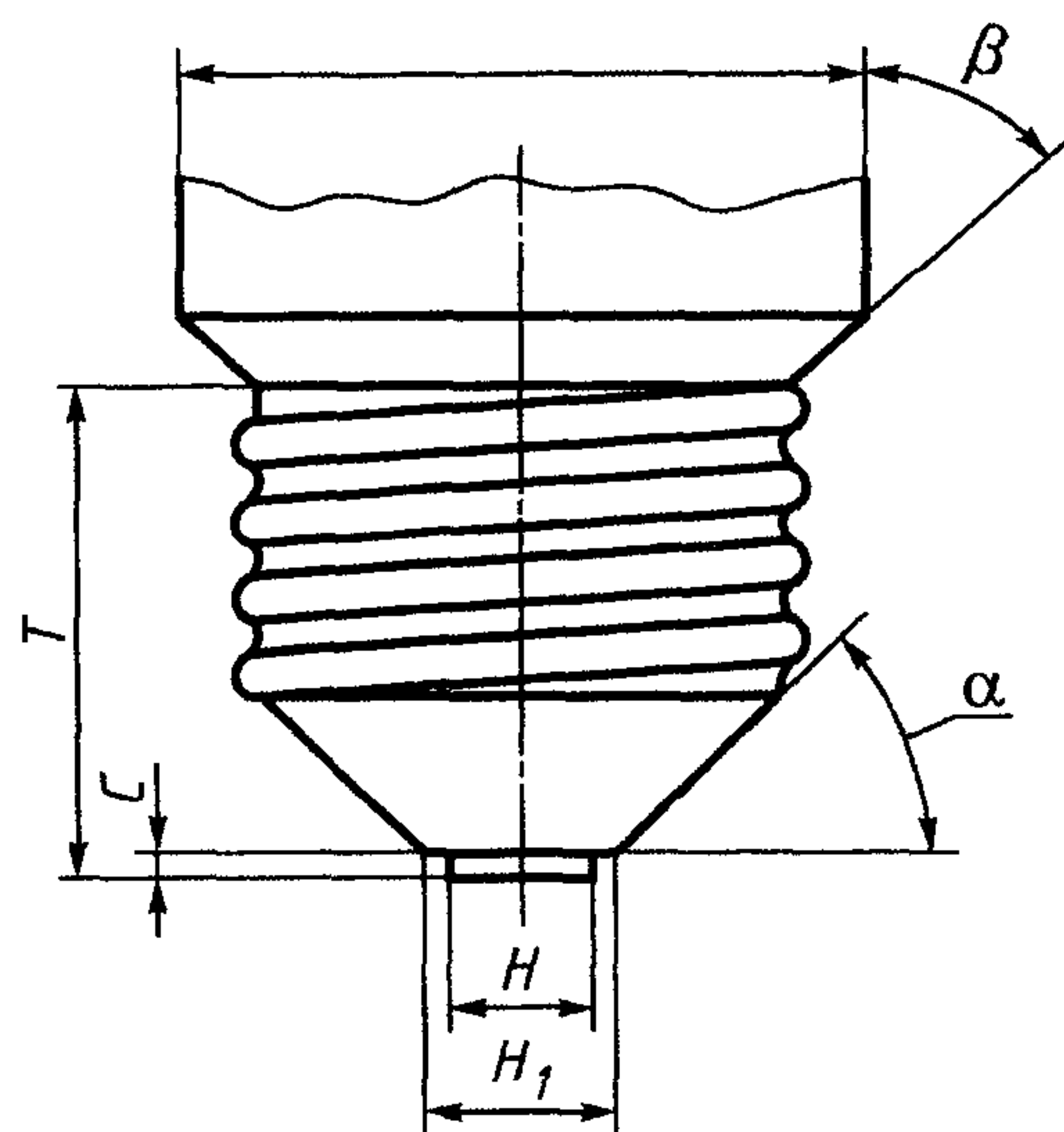
Испытательный цоколь E40
