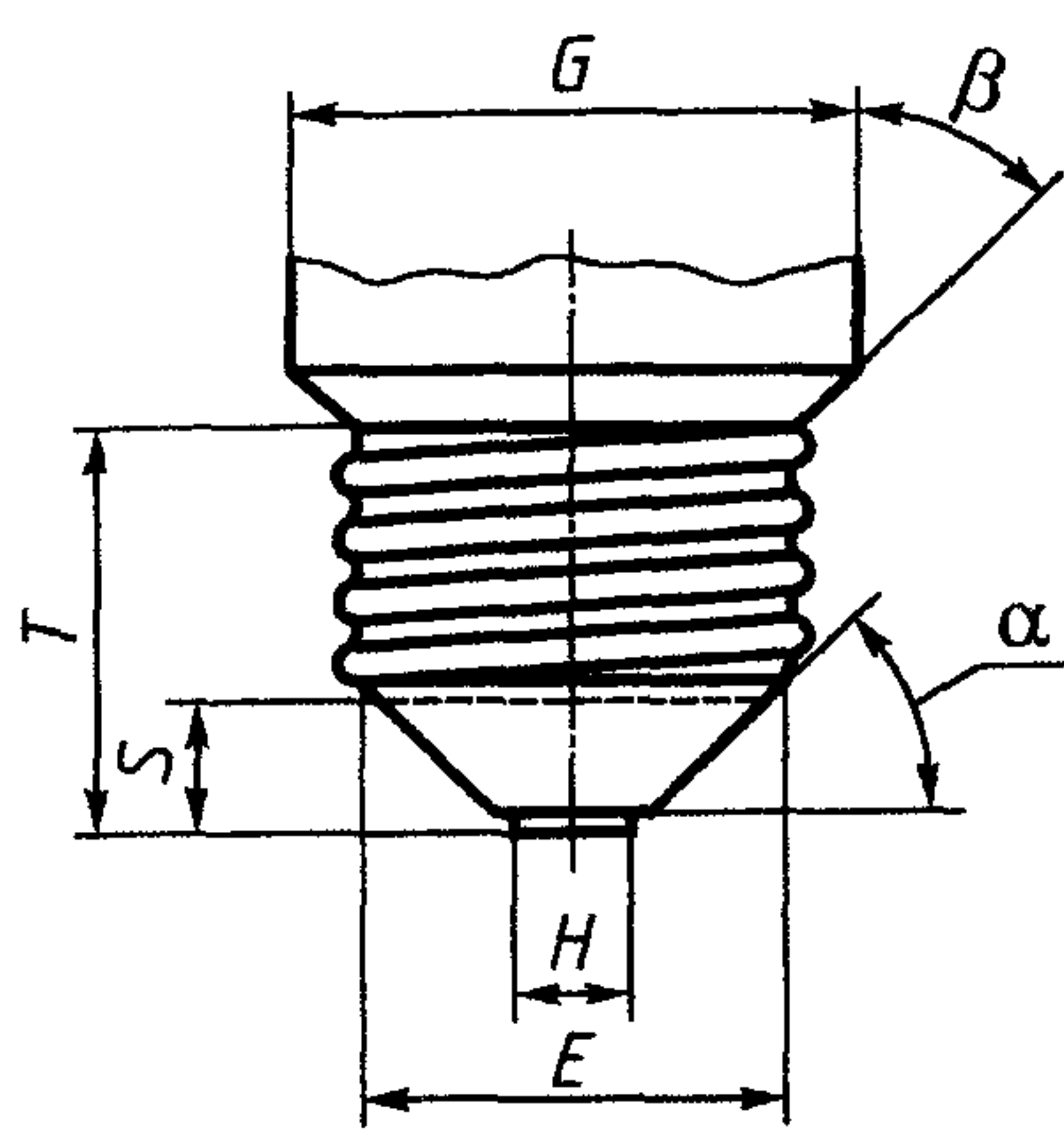
Испытательные цоколи E14 и E27
