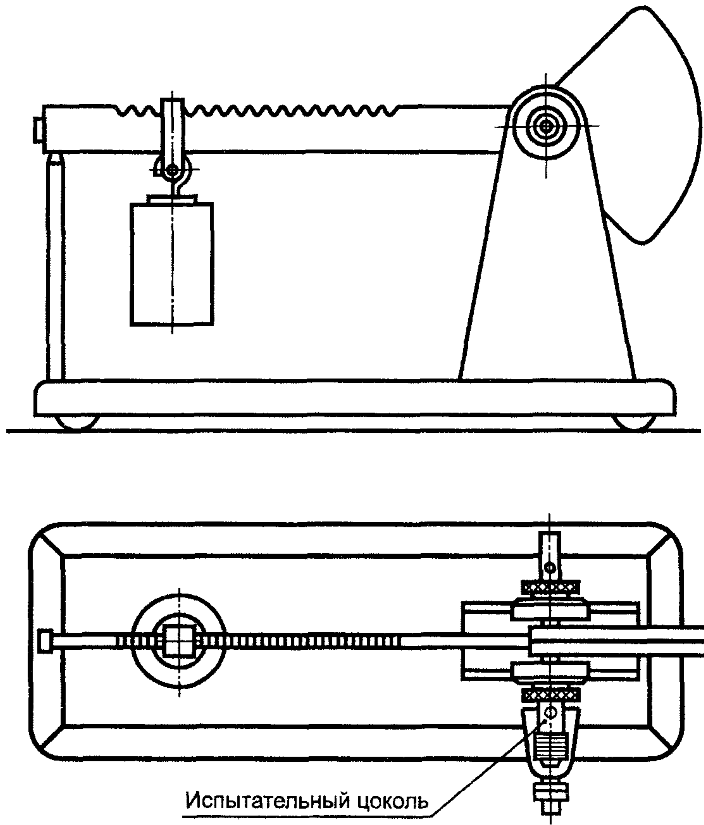
Рисунок 6 — Установка для проверки на скручивание
