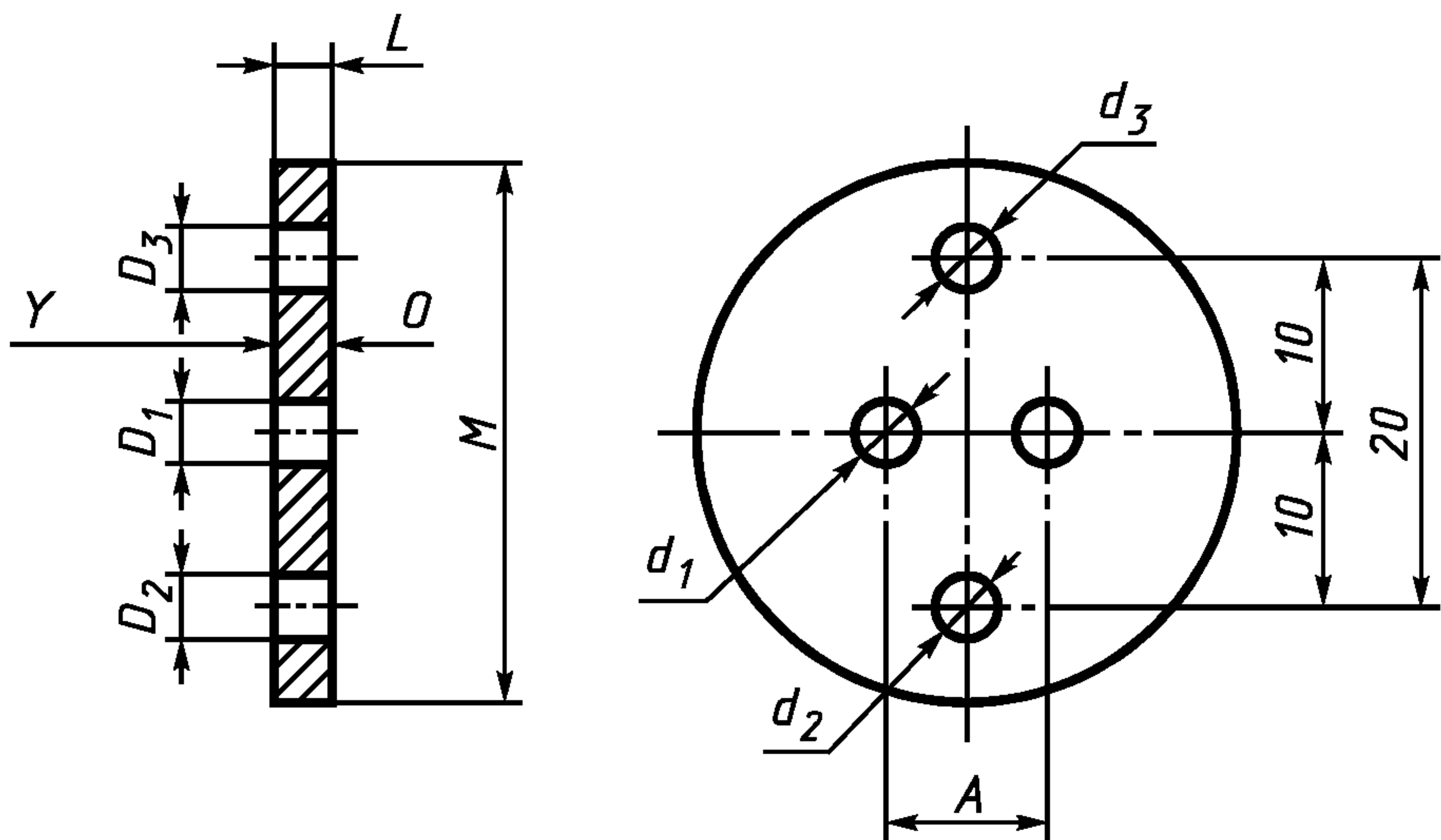
Указаны только контролируемые размеры Рисунок 1 — Размеры стартеров
