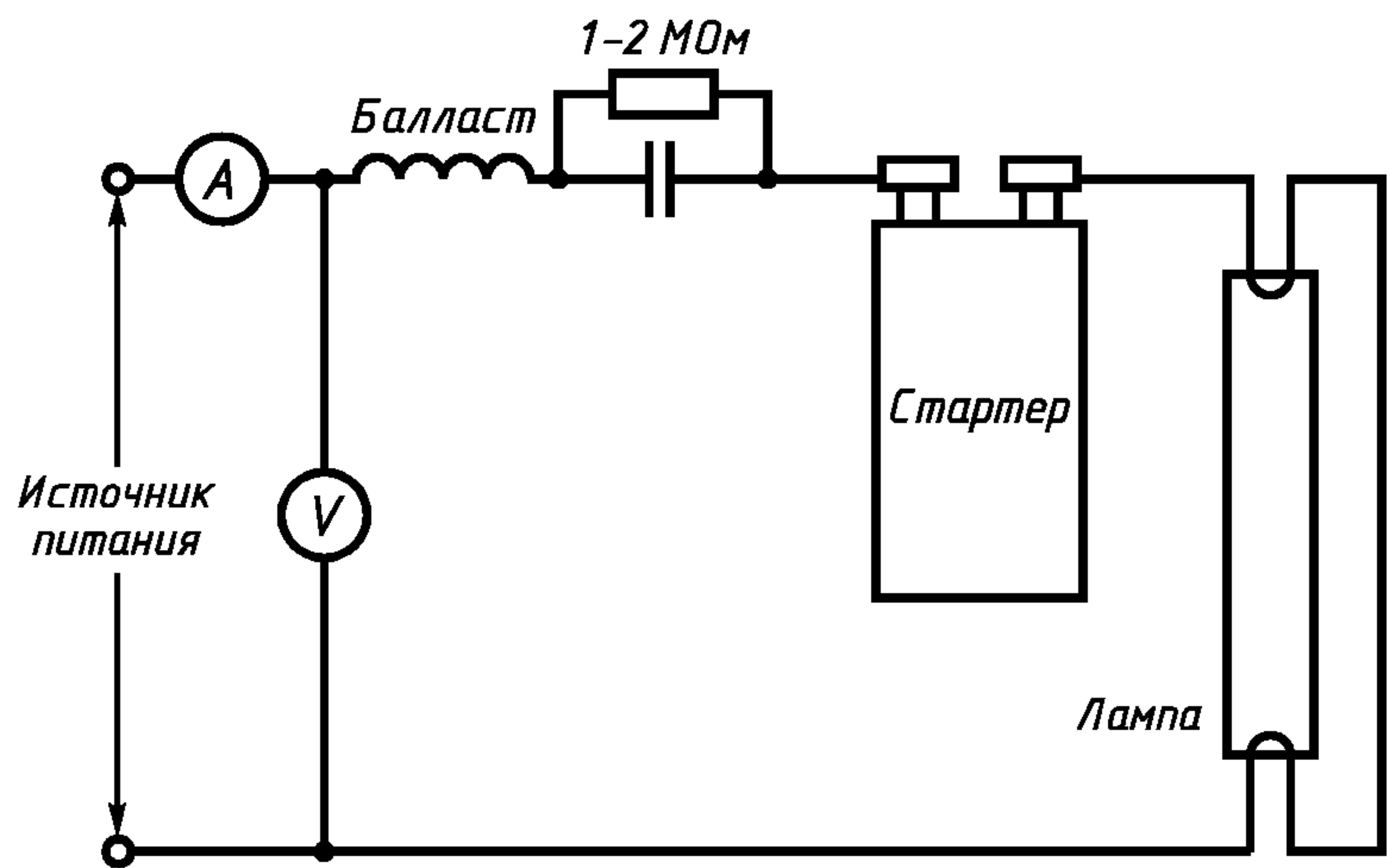
Рисунок 7 — Схема испытания стартеров на зажигание
