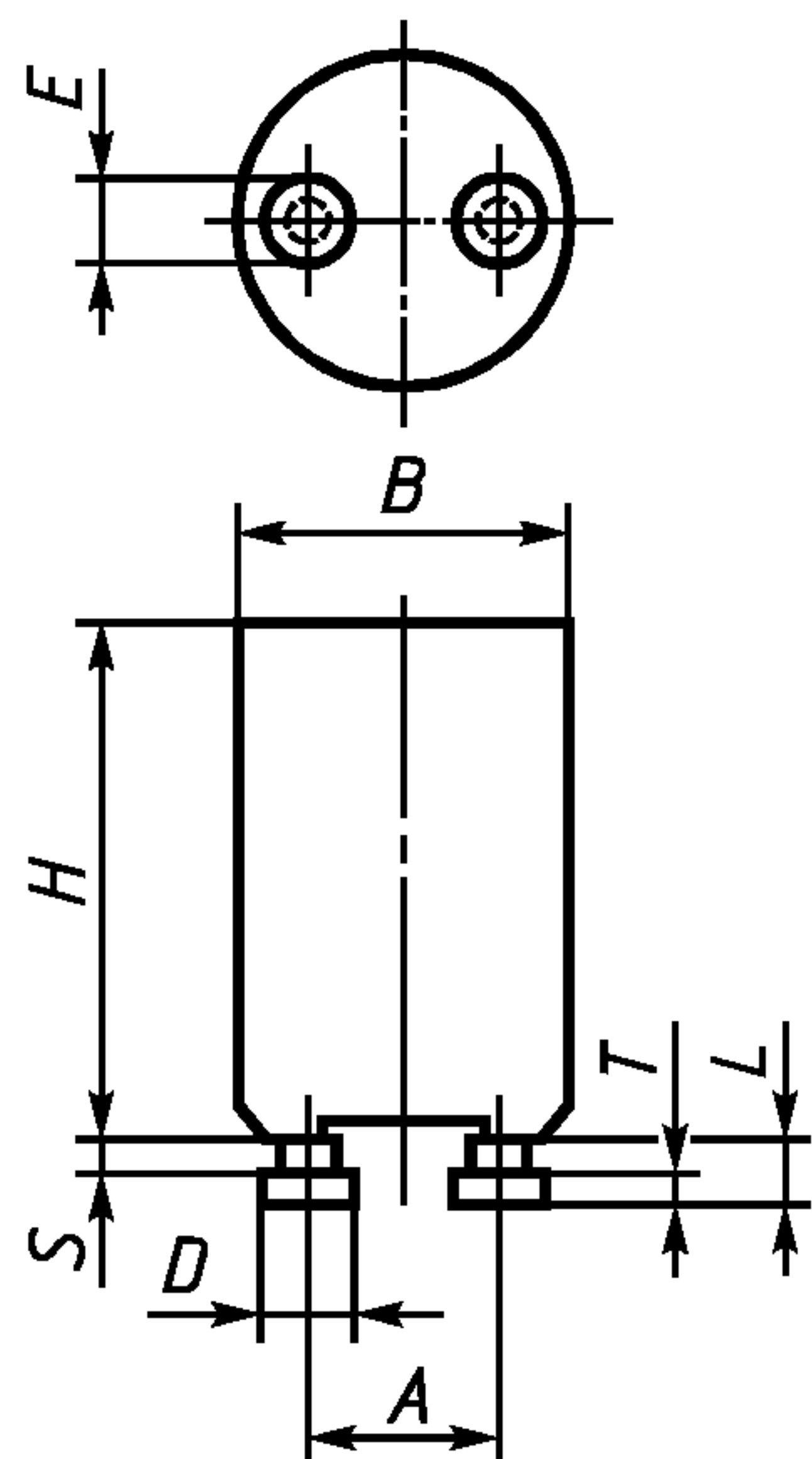
Указаны только контролируемые размеры Рисунок 1 — Размеры стартеров
