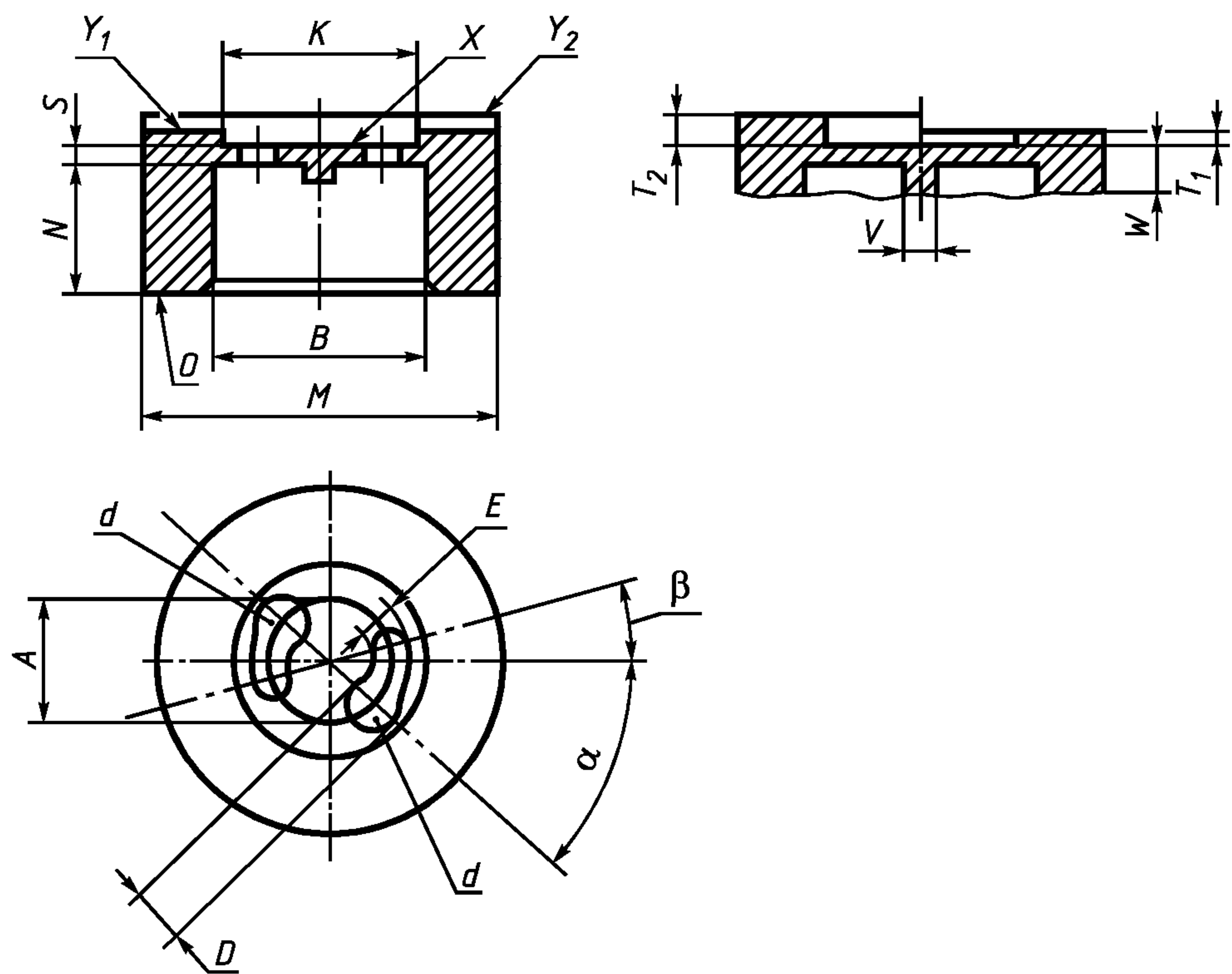
Указаны только основные размеры калибра
