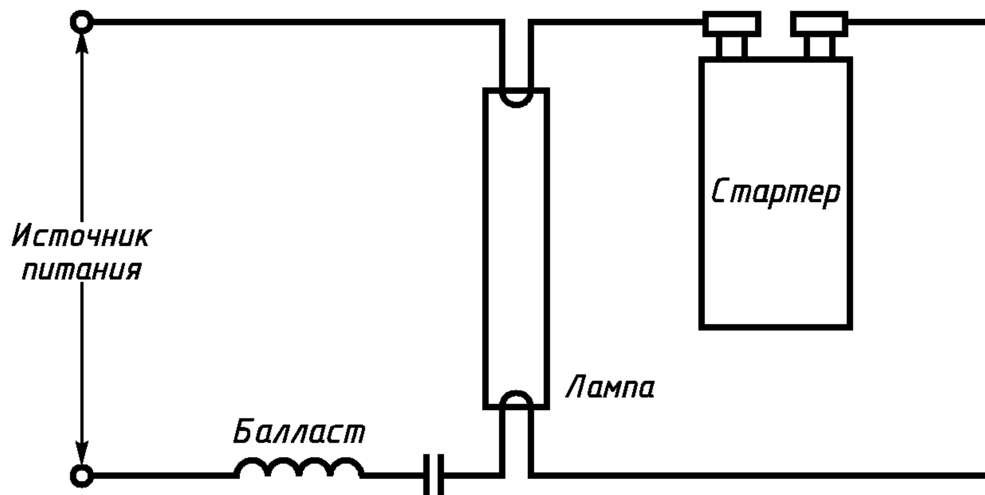
Рисунок 10 — Схема испытания стартеров на долговечность
