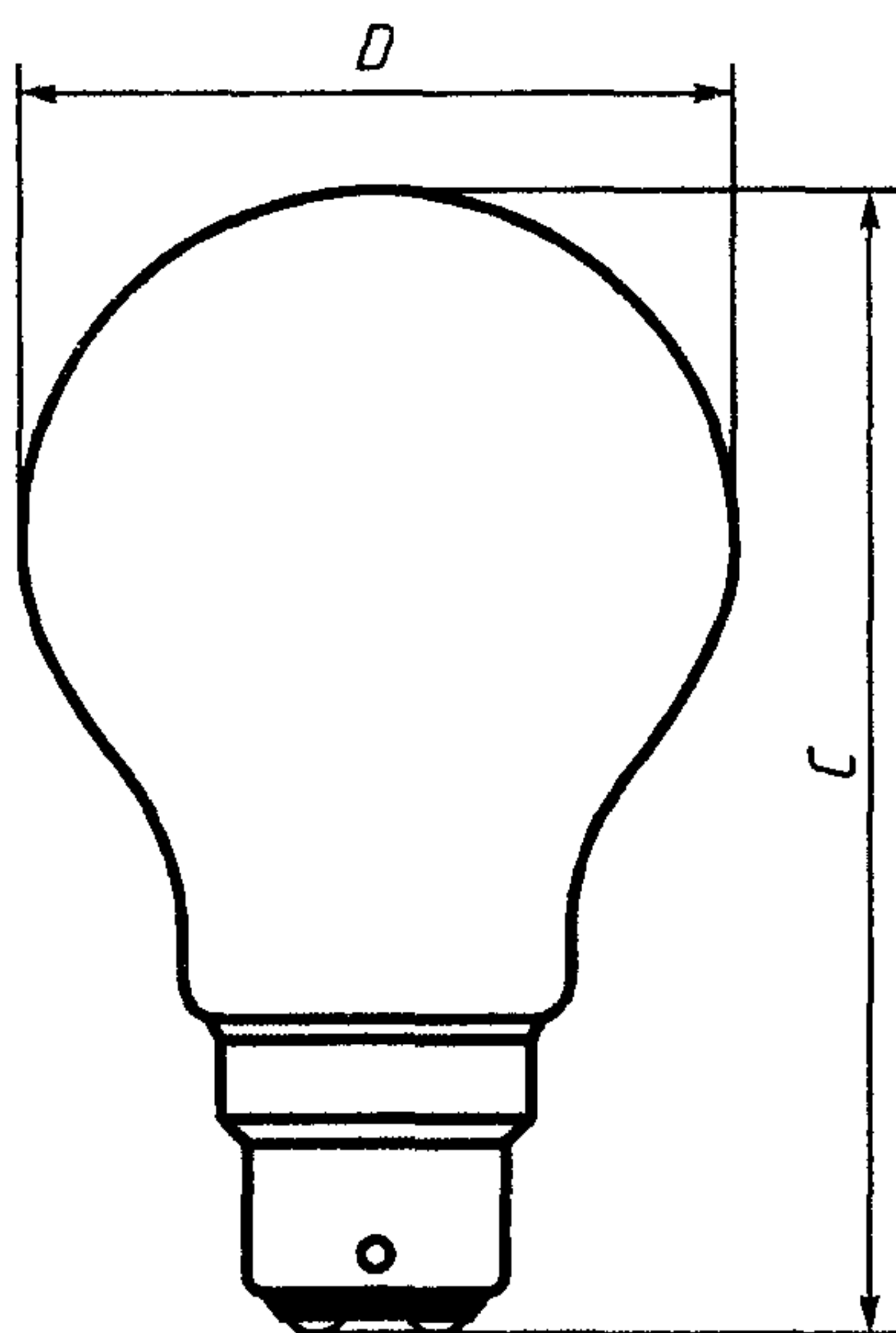
Рисунок 1 — Лампа с цоколем B22d
