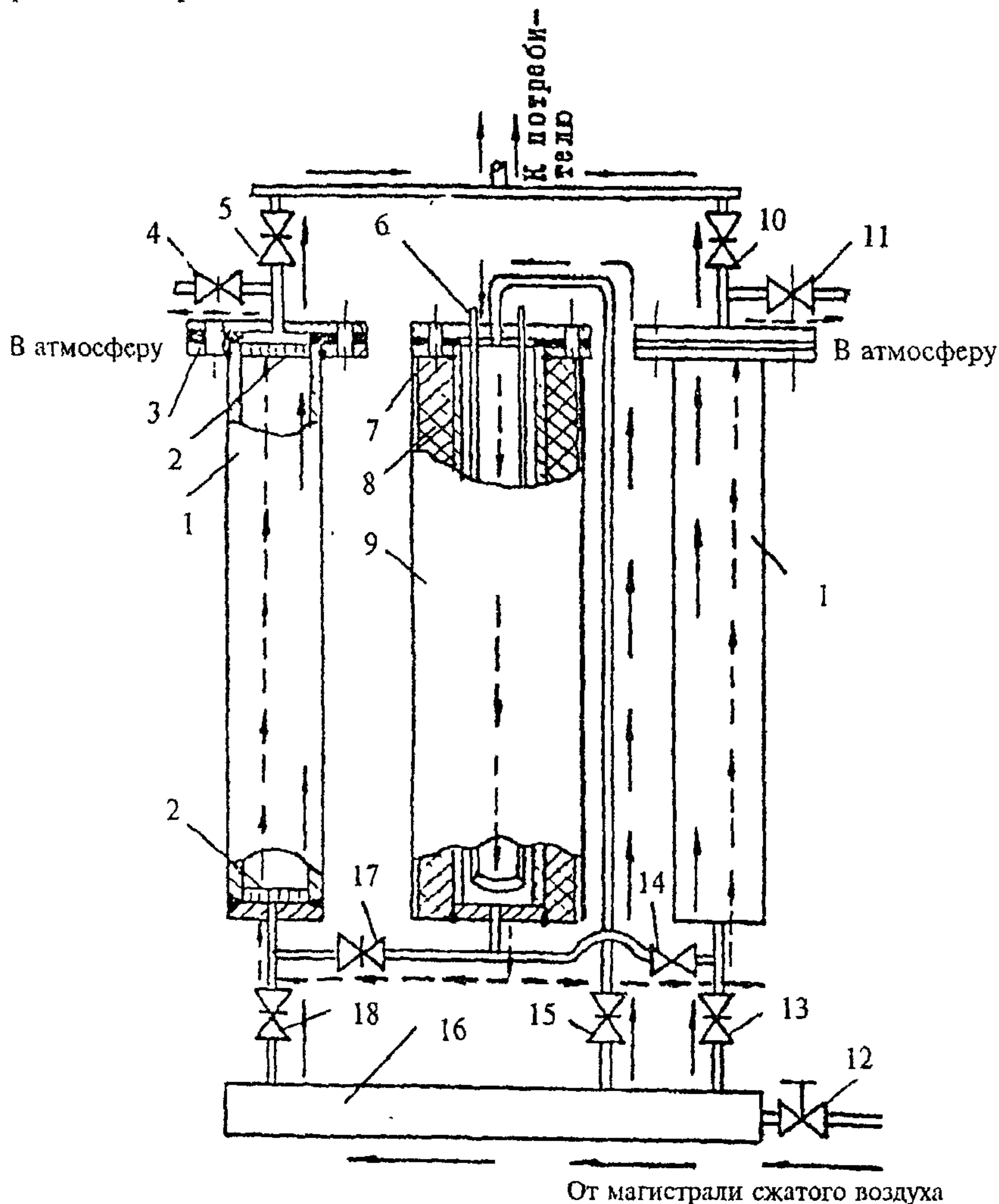
Рис. В.2. Схема переносного масловлагоотделителя:
