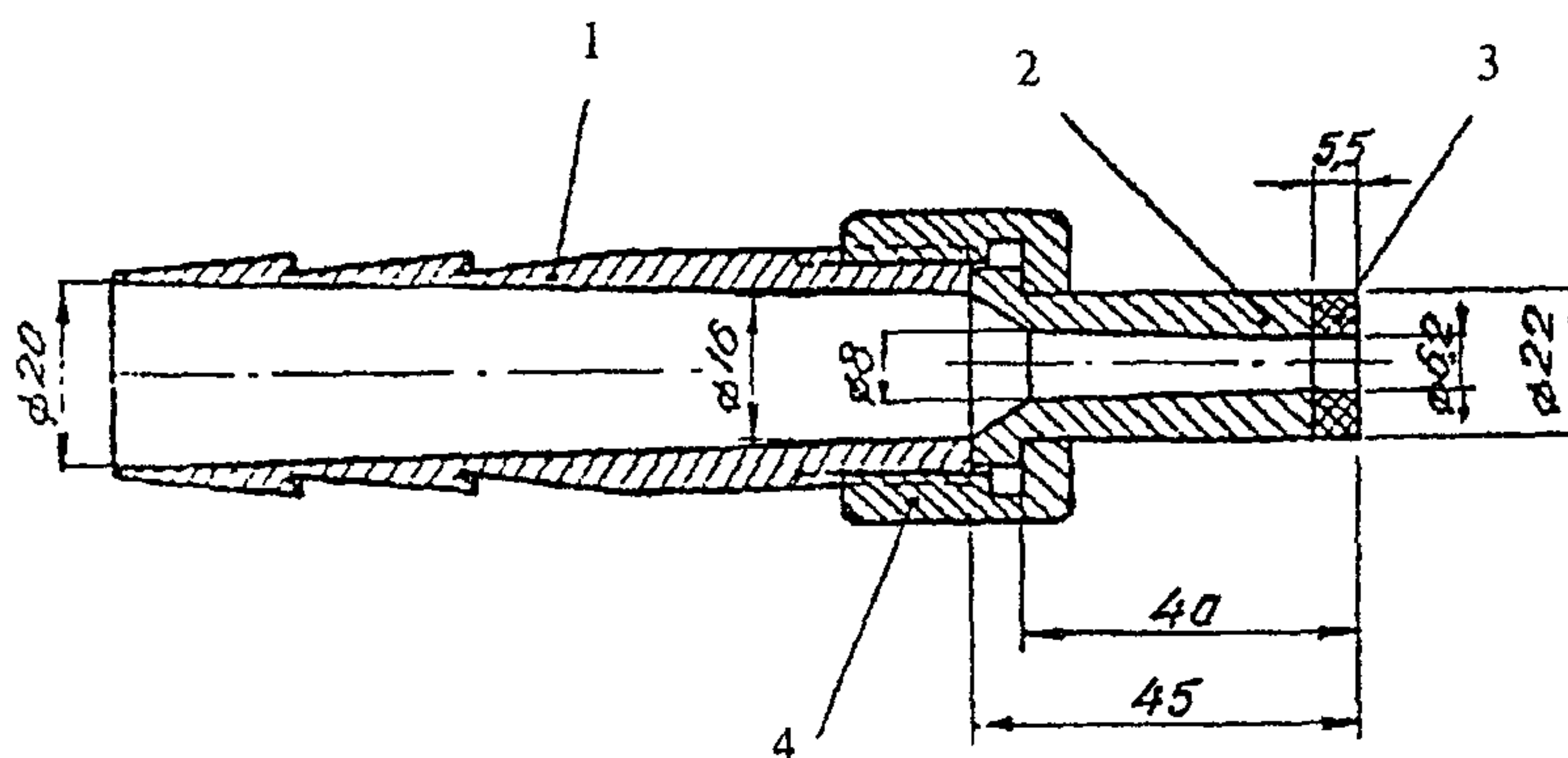
Рис. Б.1. Металлическое сопло:
