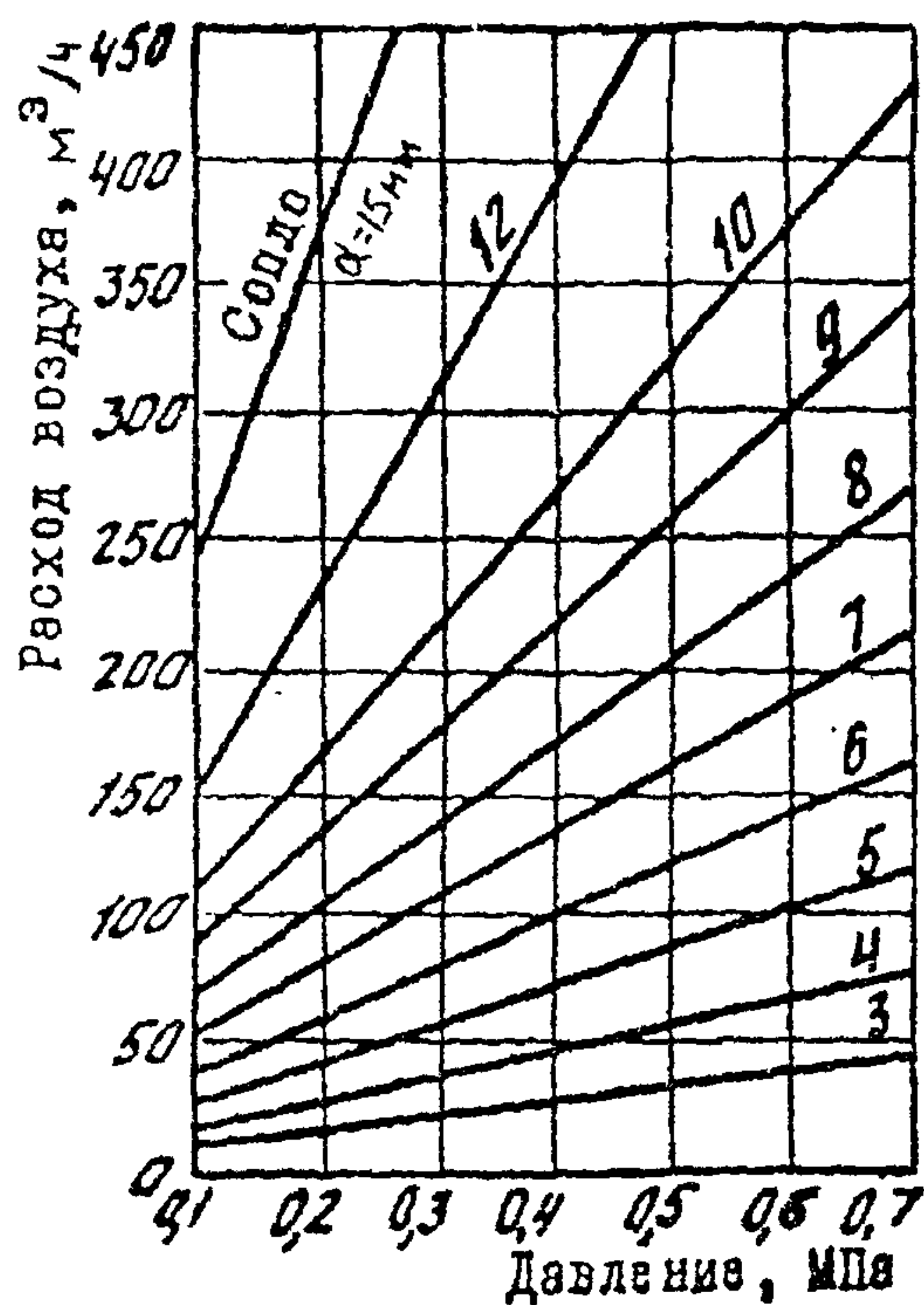
Рис 2 Номограмма расхода жидкого топлива
