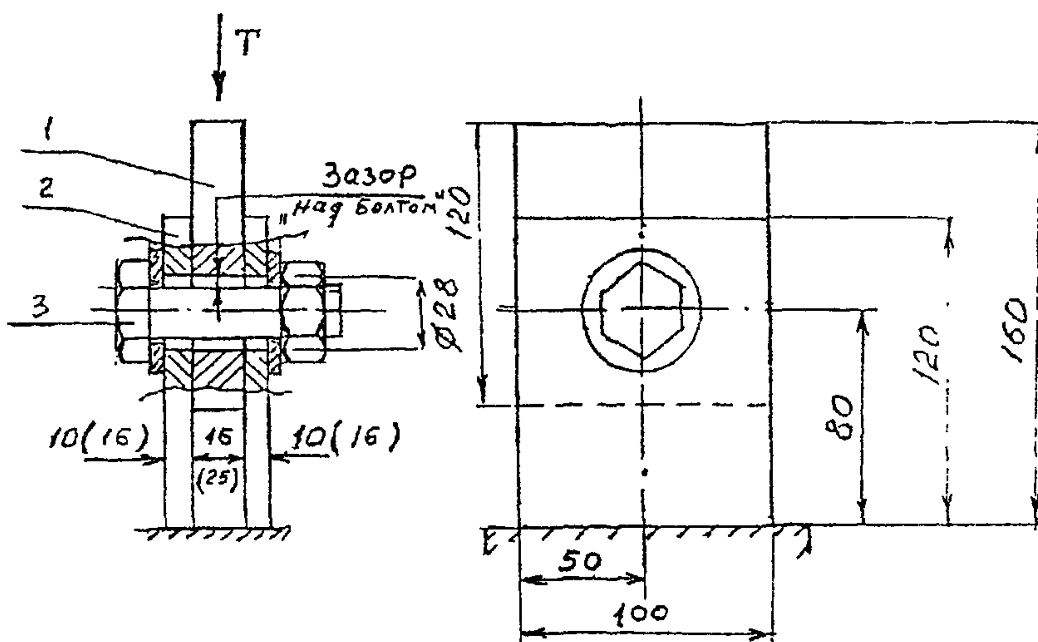
Рис. Л.1. Образец для испытания на сдвиг при сжатии:
