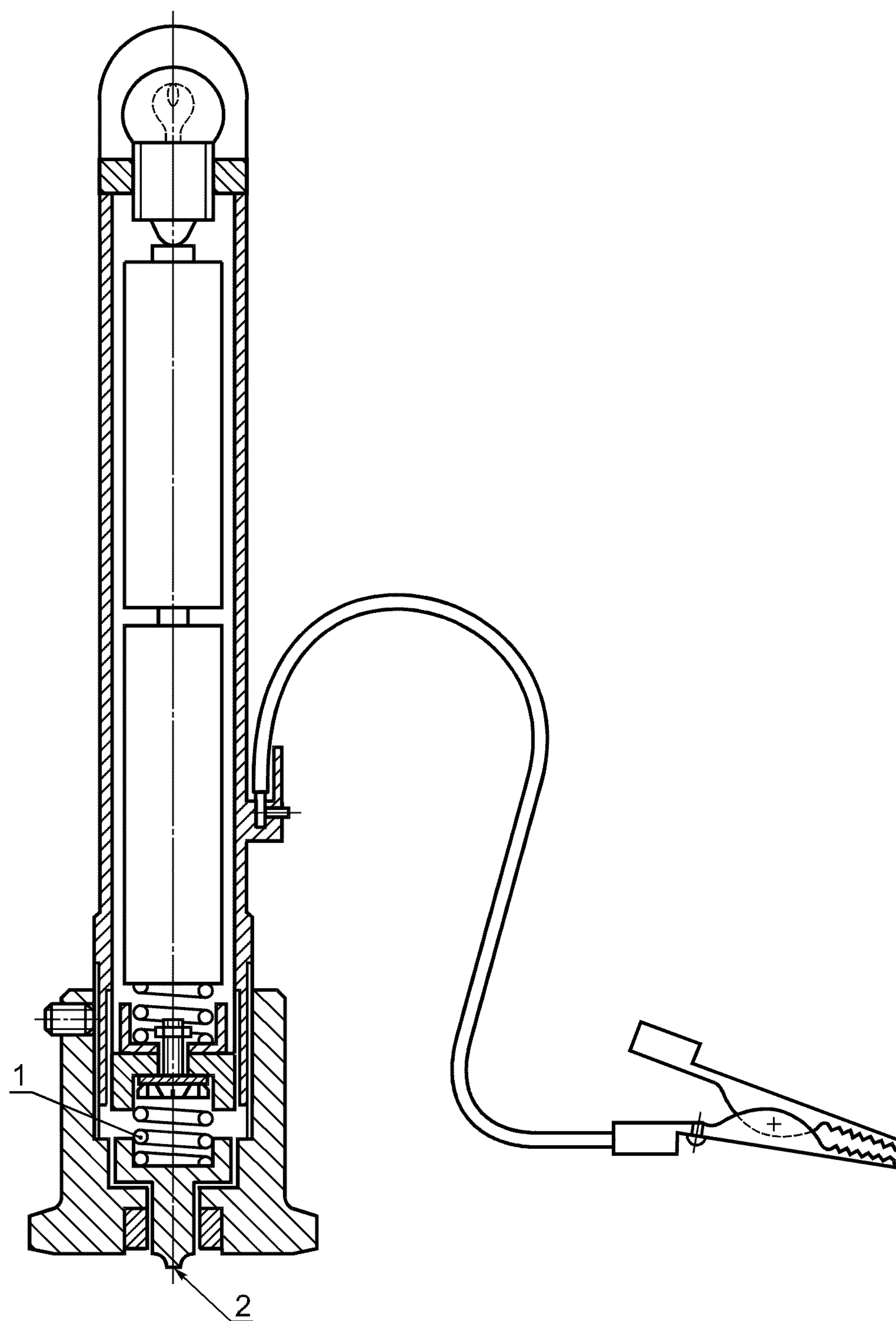
1 — пружина; 2 — рабочая точка (стальной шарик диаметром 1 мм)
