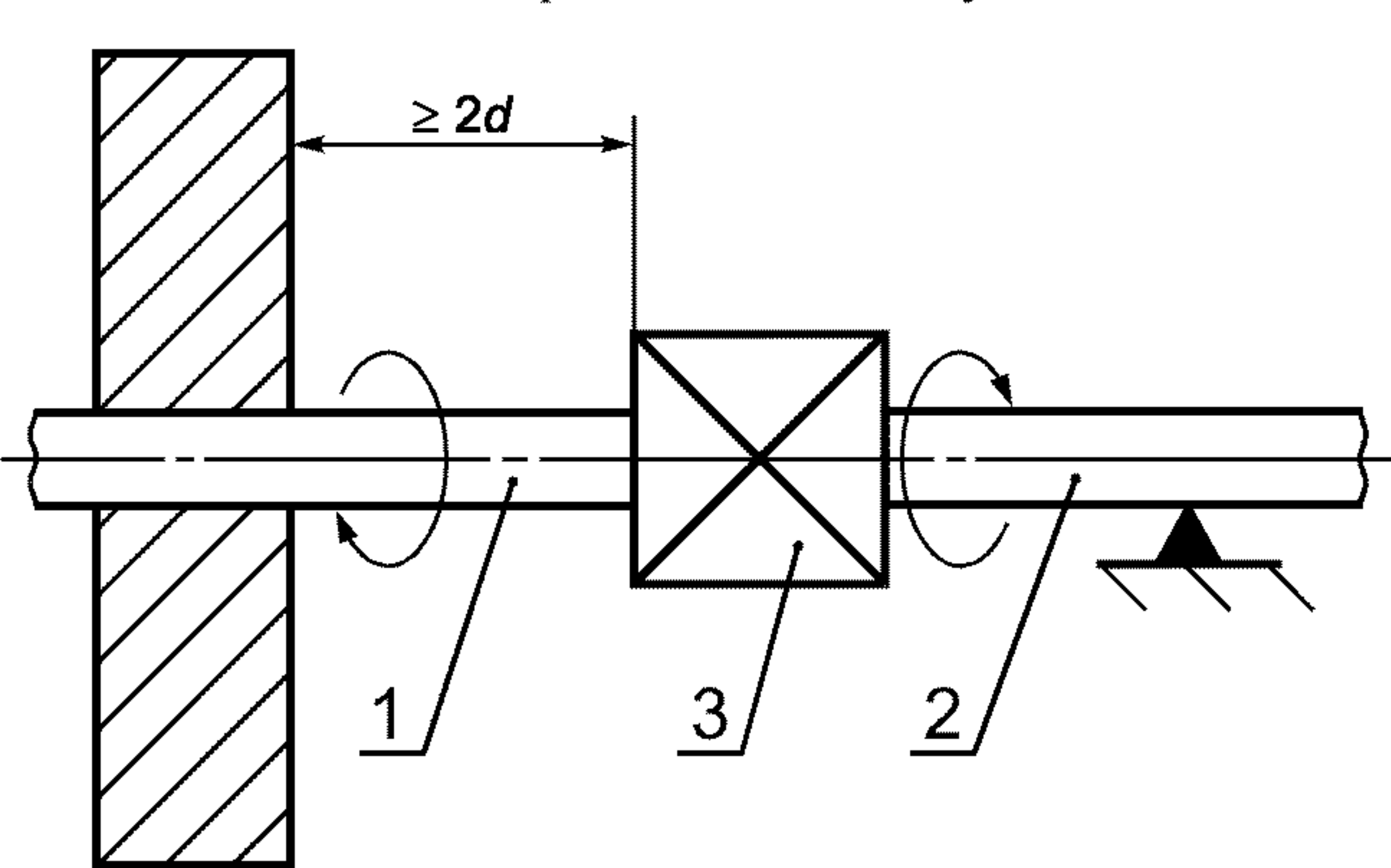
d — наружный диаметр 1, 2 — труба; 3 — испытуемый образец
