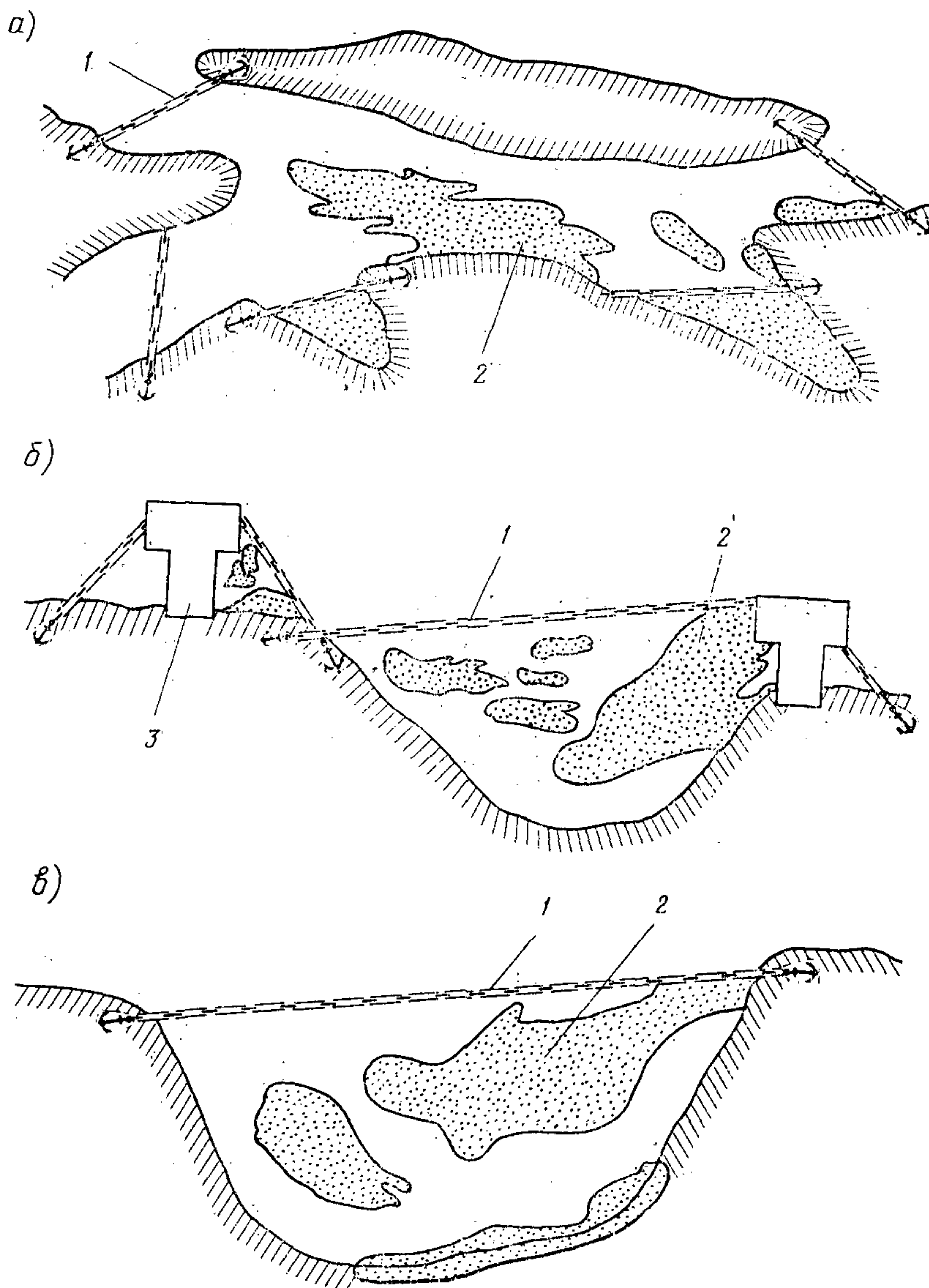
Рис. 20. Схема локализации нефтяного загрязнения: а — в протоке или озере, сообщающихся с рекой; б — в районе причалов; в — у заводи; 1 — боновое заграждение; 2 — нефтяное пятно; 3 — причал
