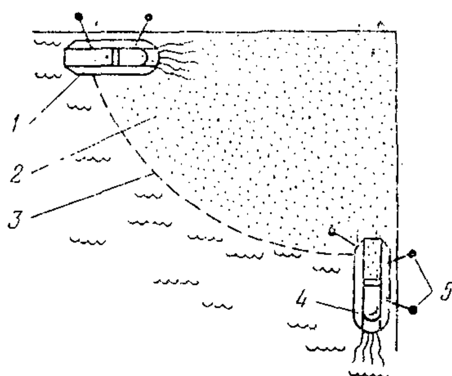
Рис. 10 Сбор загрязняющих веществ в углах причалов с использованием вспомогательного нефтемусоросборщика и боновых заграждений 1 — вспомогательный нефтемусоросборщик или катер, 2 — загрязняющие вещества, 3 — оперативные боновые заграждения, 4 — рабочий нефтемусоросборщик, 5 — швартовы
