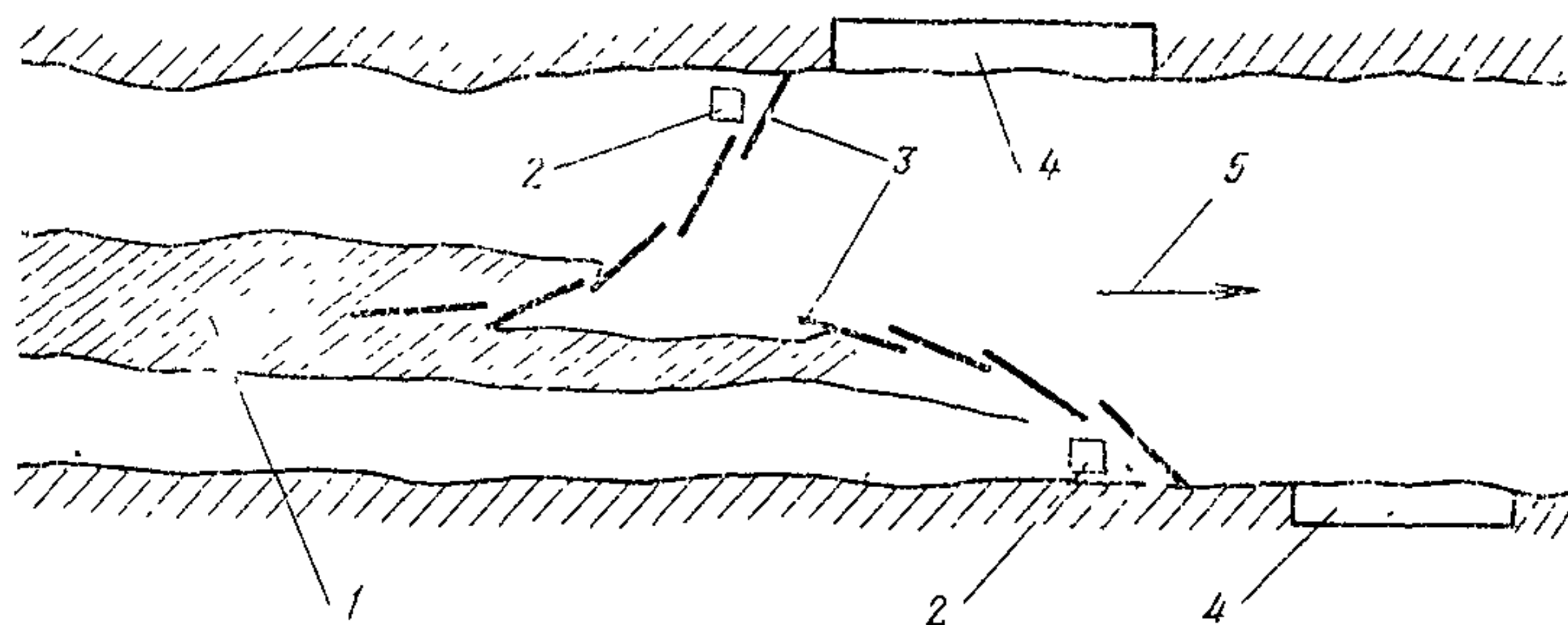
Рис. 14. Шевронное расположение бонов: 1 — нефтяное пятно; 2 — нефтеприемник; 3 — боны; 4 — защищаемый объект; 5 — направление течения
