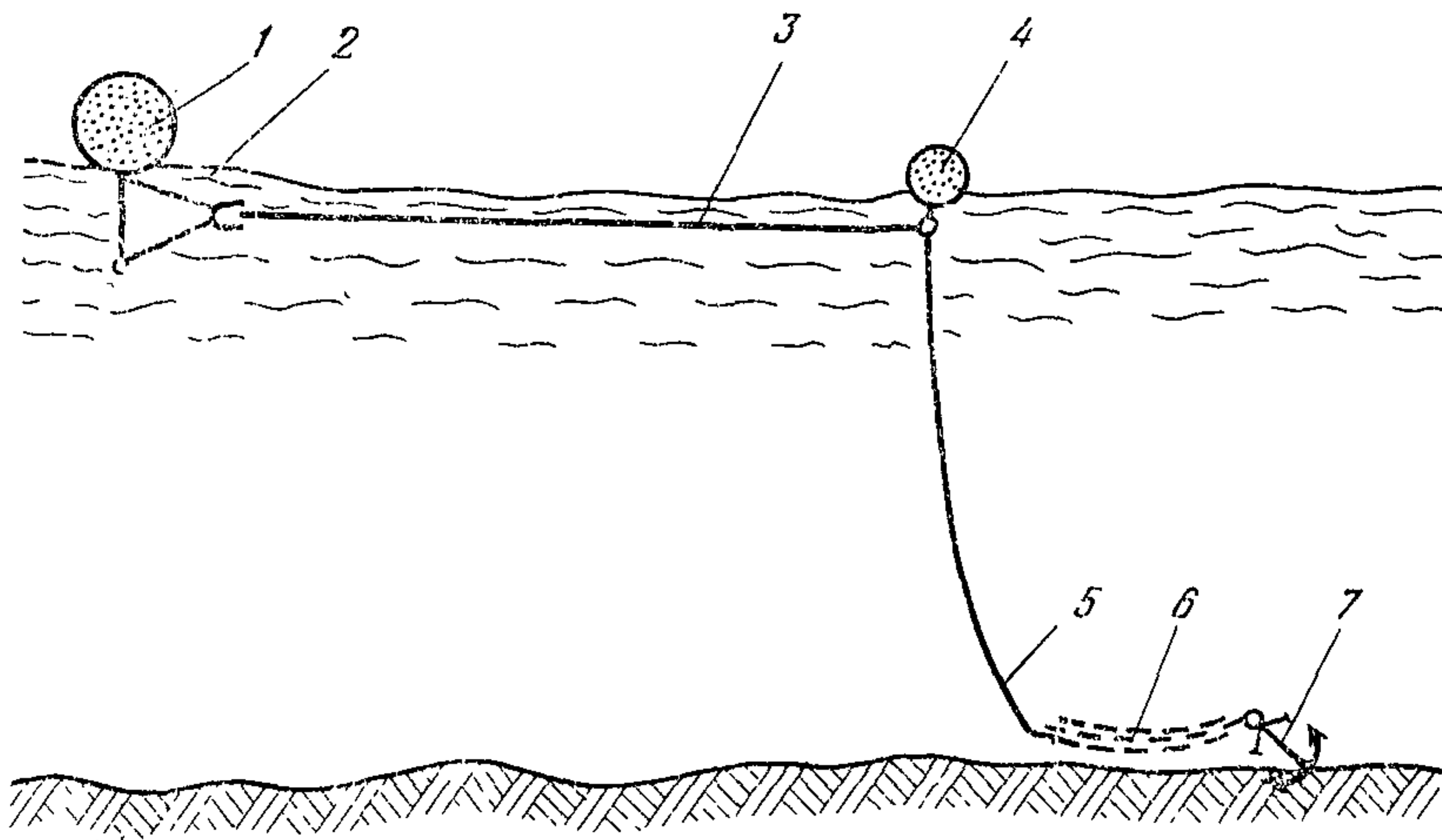
Рис. 21 Установка бонового заграждения на буй 1 — бон; 2 — оттяжка бона, 3 — синтетический канат, 4 — буй; 5 — канат буя, 6 — якорь-цепь, 7 — якорь
