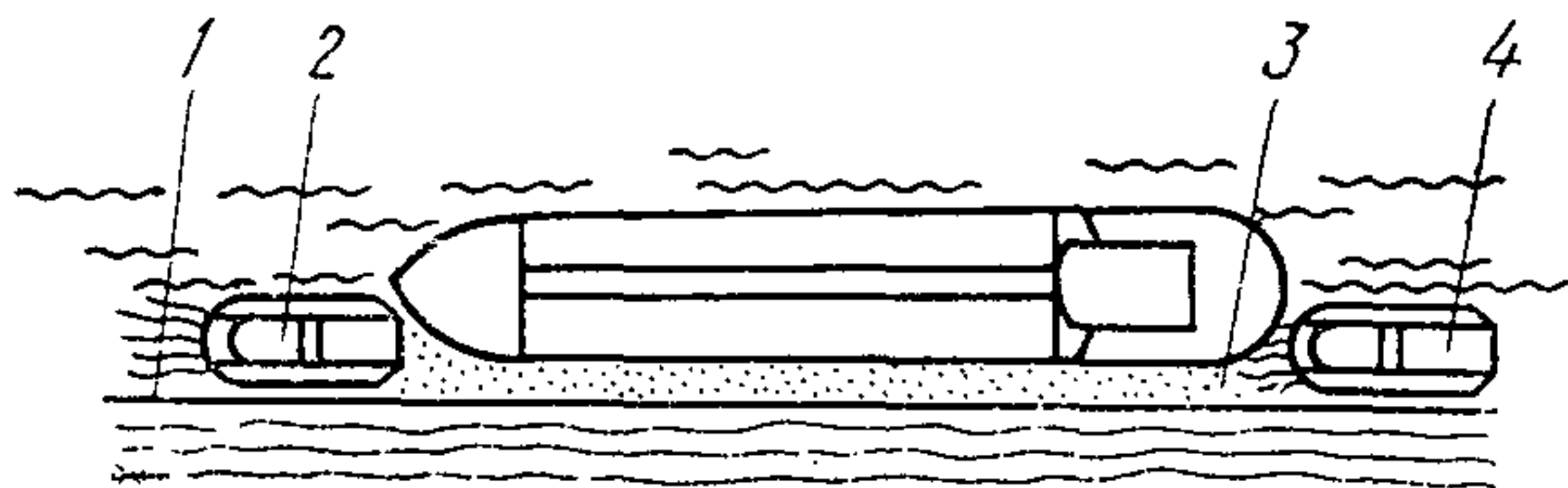
Рис 6 Сбор загрязняющих веществ между судном и причалом 1 — причал, 2 — рабочий нефтемусоросборщик, 3 — загрязняющие вещества, 4 — вспомогательный нефтемусоросборщик или катер
