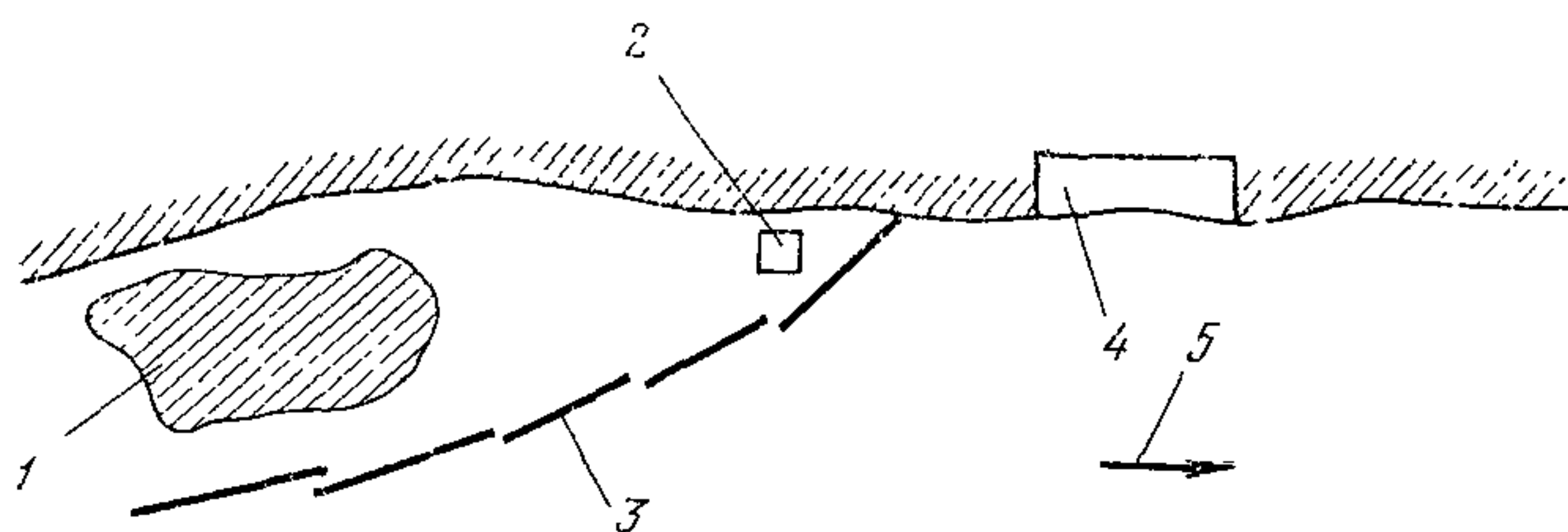
Рис. 15. Каскадное расположение бонов: 1 — нефтяное пятно; 2 — нефтеприемник; 3 — бон; 4 — защищаемый объект; 5 — направление течения
