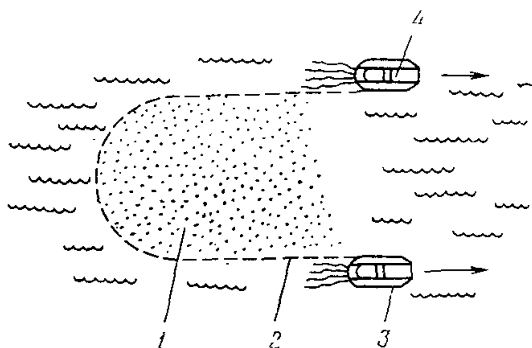
Рис. 1. Движение нефтемусоросборщиков при очистке открытой акватории:
