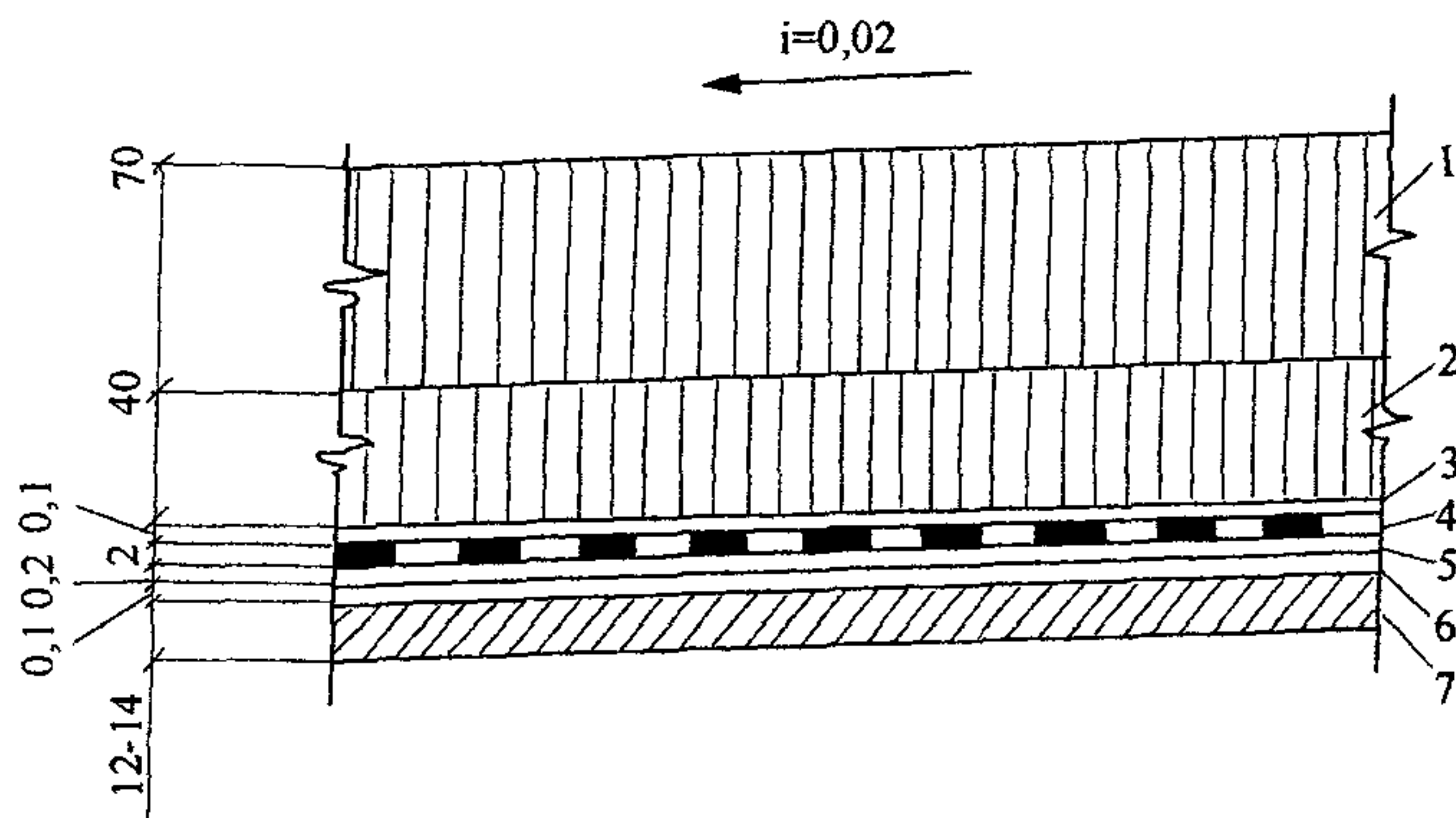
Рис. 1. Одежда ездового полотна по сварной ортотропной плите:
