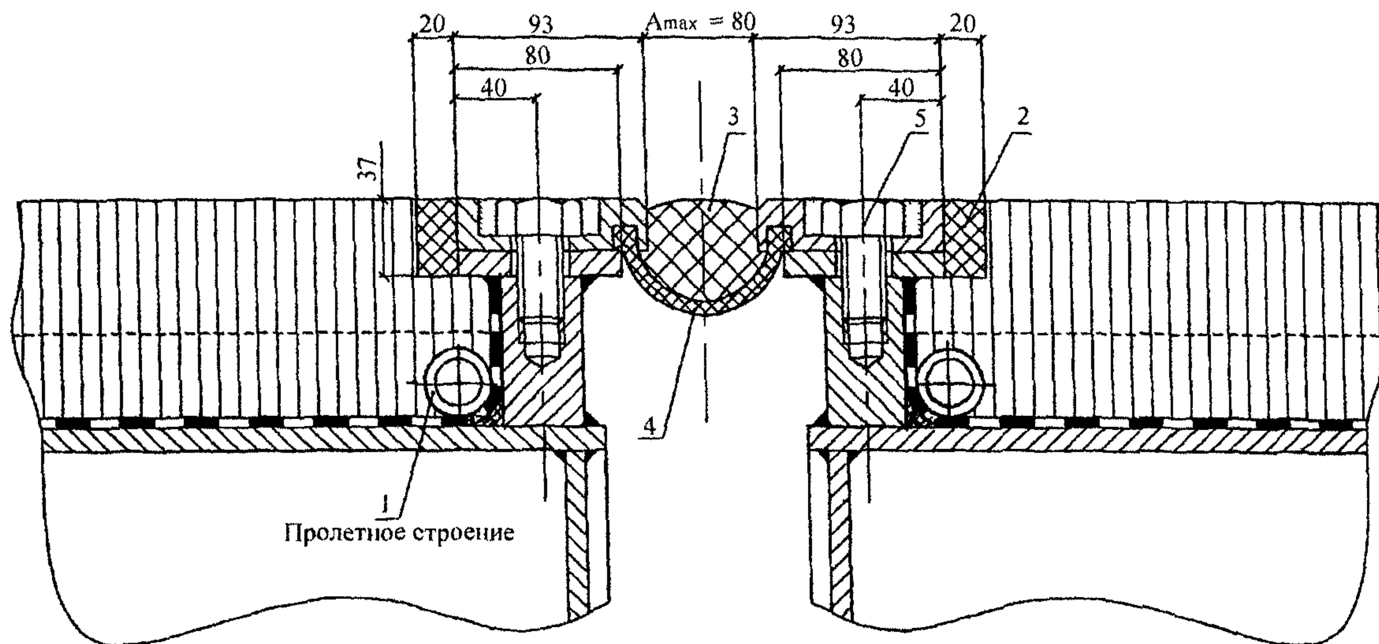
Рис. 5. Гидроизоляция в примыкании к деформационному шву: 1 – дренажная перфорированная трубка; 2 – штрабы, заполненные эластичной мастикой; 3 – упругий пористый заполнитель; 4 – резиновый компенсатор К-8; 5 – высокопрочный болт
