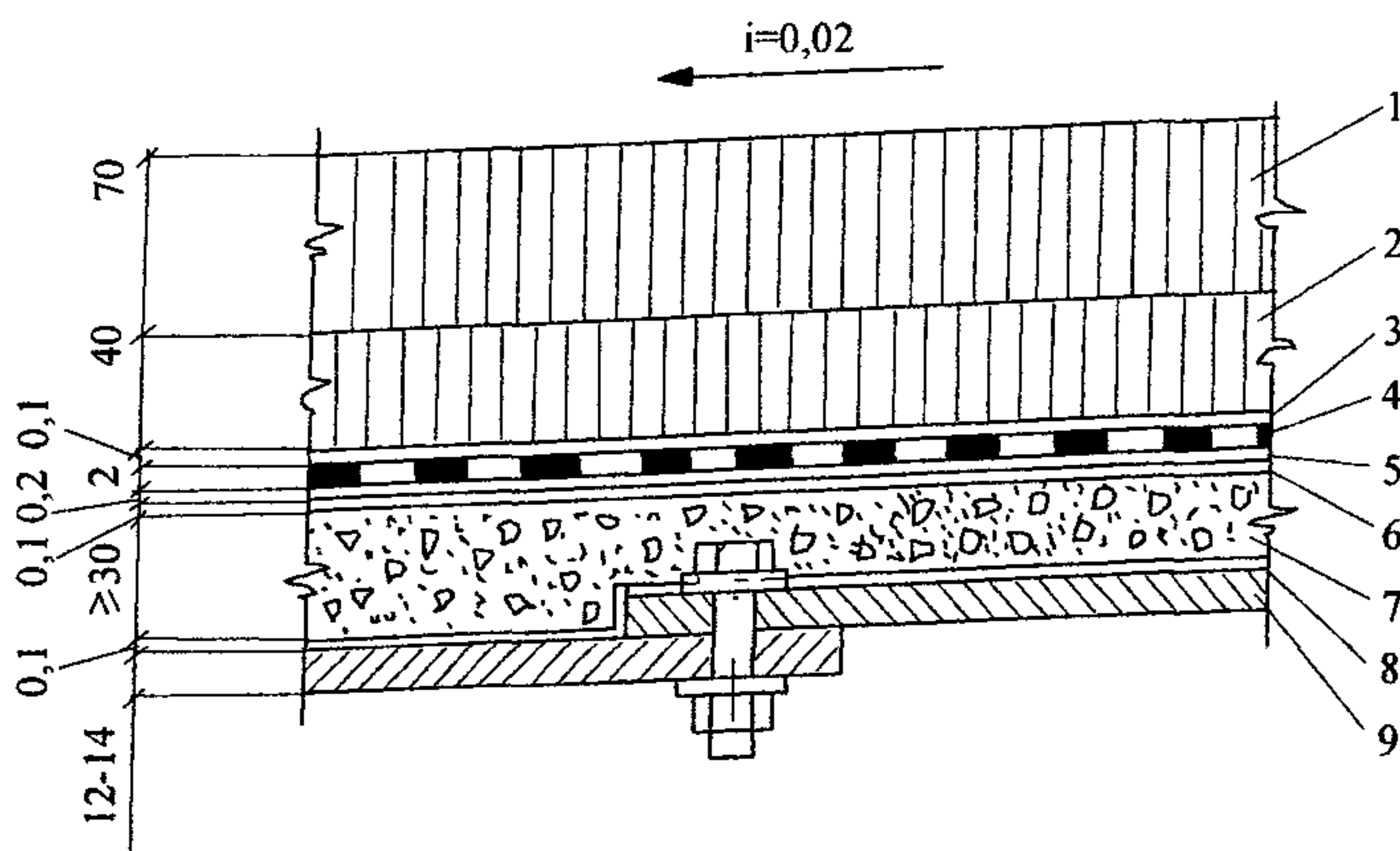
Рис. 2. Одежда ездового полотна по стальной ортотропной плите с соединениями на высокопрочных болтах:
