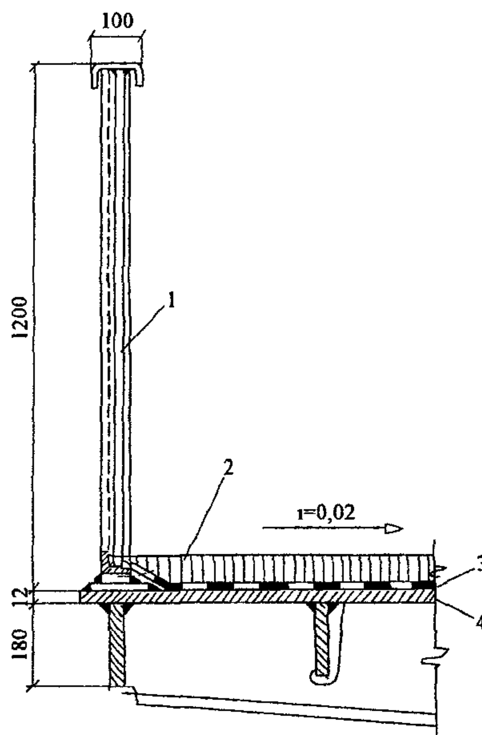
Рис. 7. Гидроизоляция у стоек перил:
