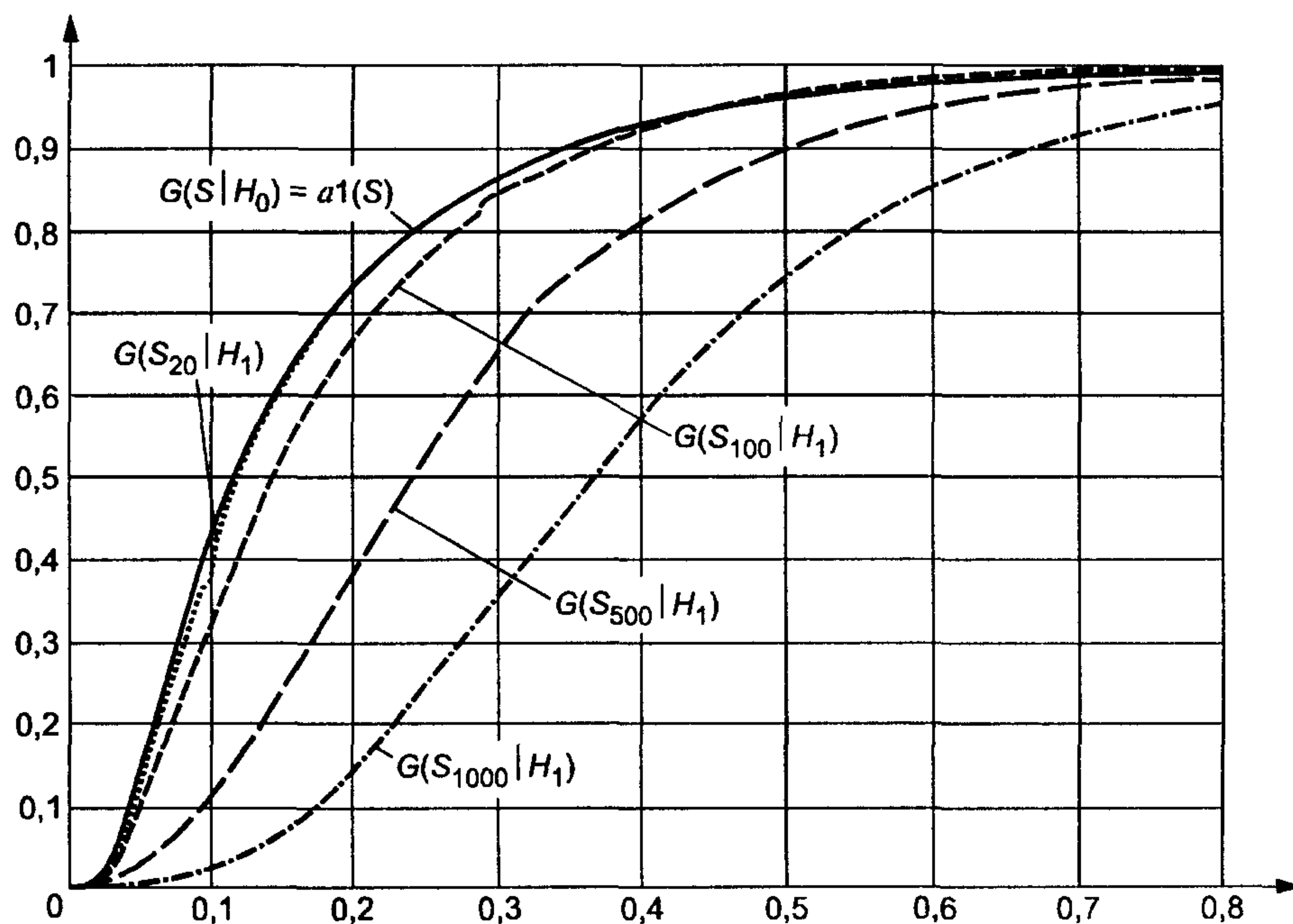
Рисунок 7 — Зависимость от n распределений G(S_n | H_1) статистики S_\omega Крамера — Мизеса — Смирнова при простой гипотезе ( H_0 — нормальное распределение, H_1 — логистическое): n = 20, 100, 500, 1000
