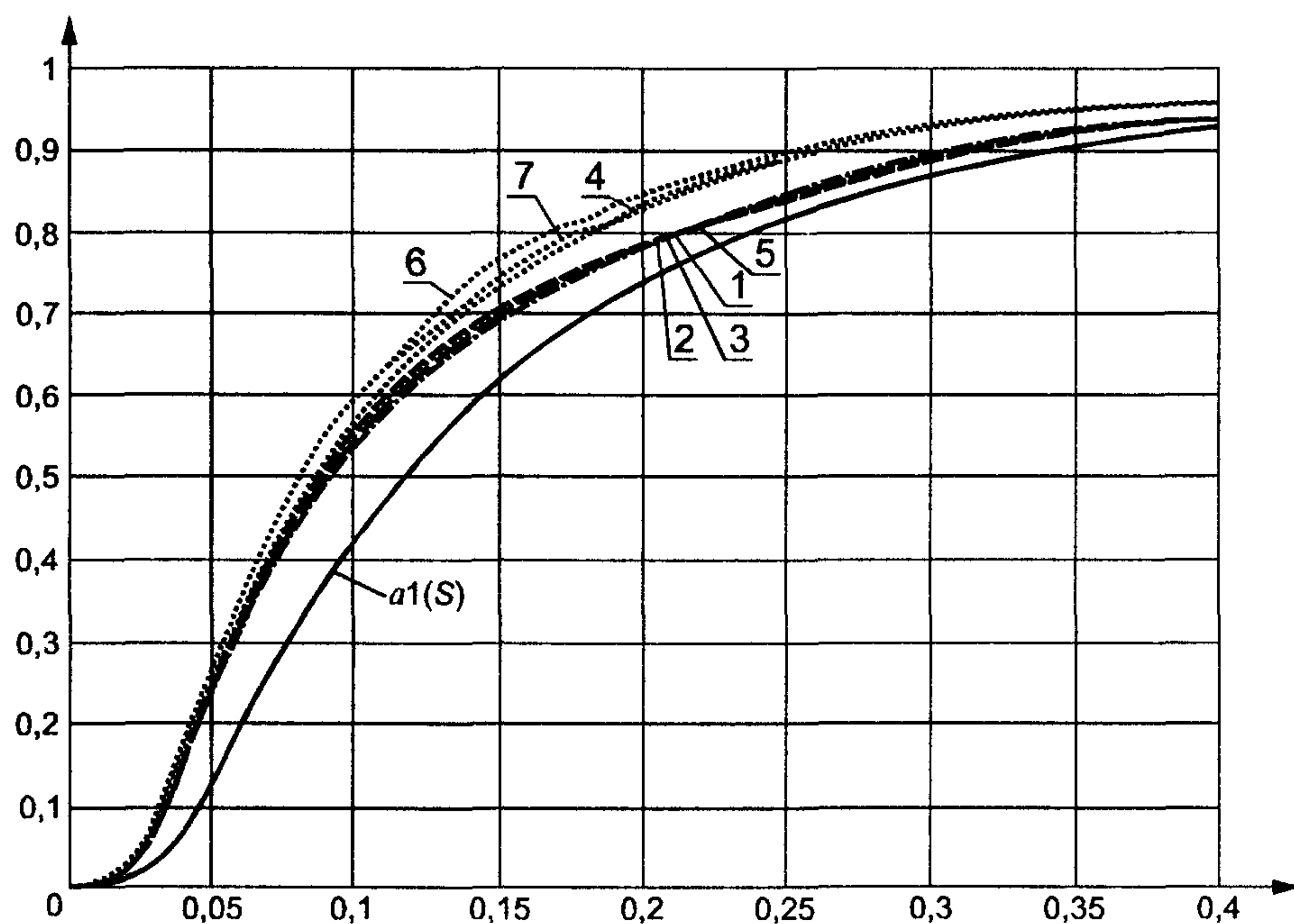
Рисунок 14 — Распределения G(S_n | H_0) статистики S_\omega Крамера — Мизеса — Смирнова при оценивании масштабного параметра закона, соответствующего гипотезе H_0 , ( \delta — максимального значения; 7 — Вейбулла, параметр формы), при использовании MD -оценок S_\omega
