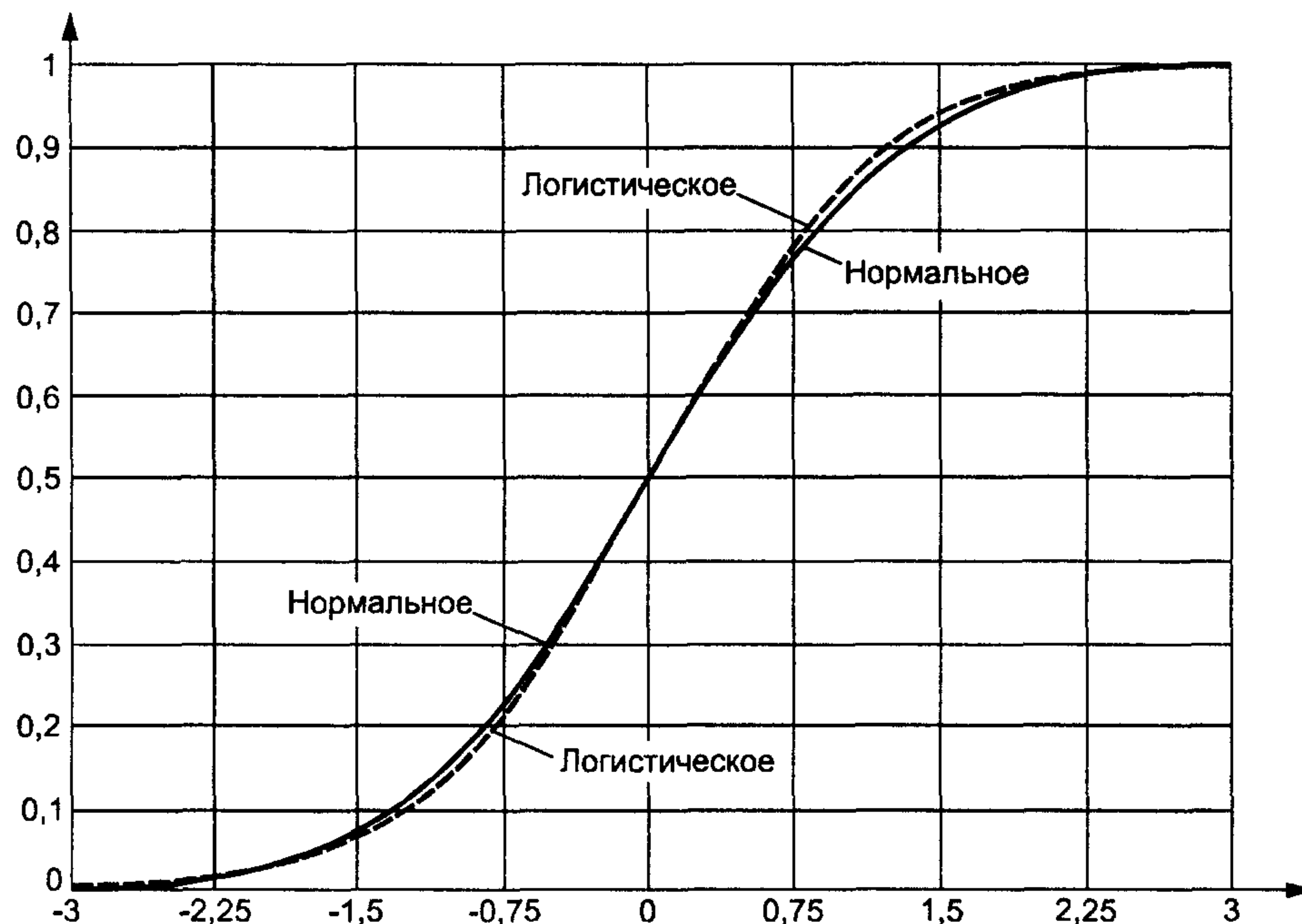
Рисунок 4 — Функции распределения нормального и логистического законов
