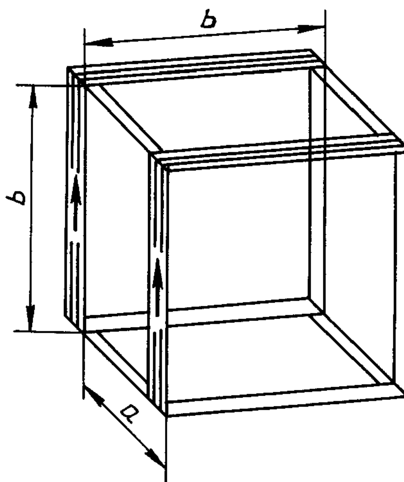
Рисунок 7 — Схема катушки Гельмгольца
