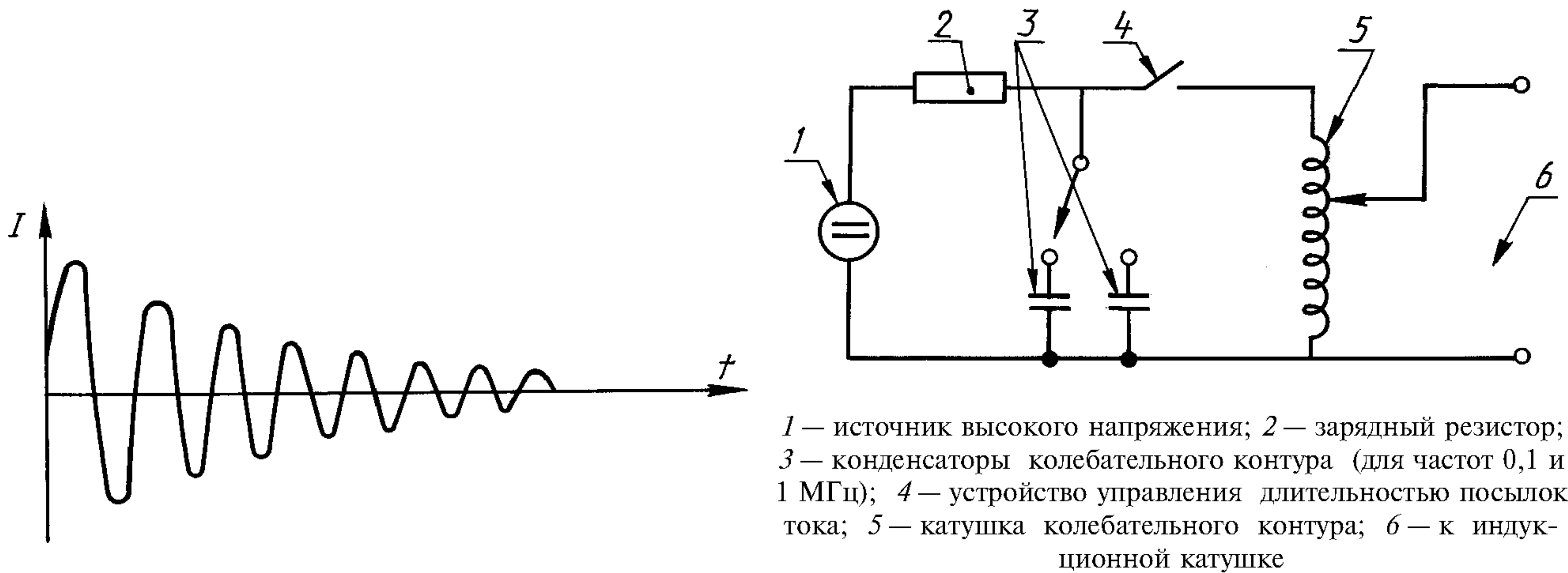
Рисунок 2 — Форма выходного тока ИГ
