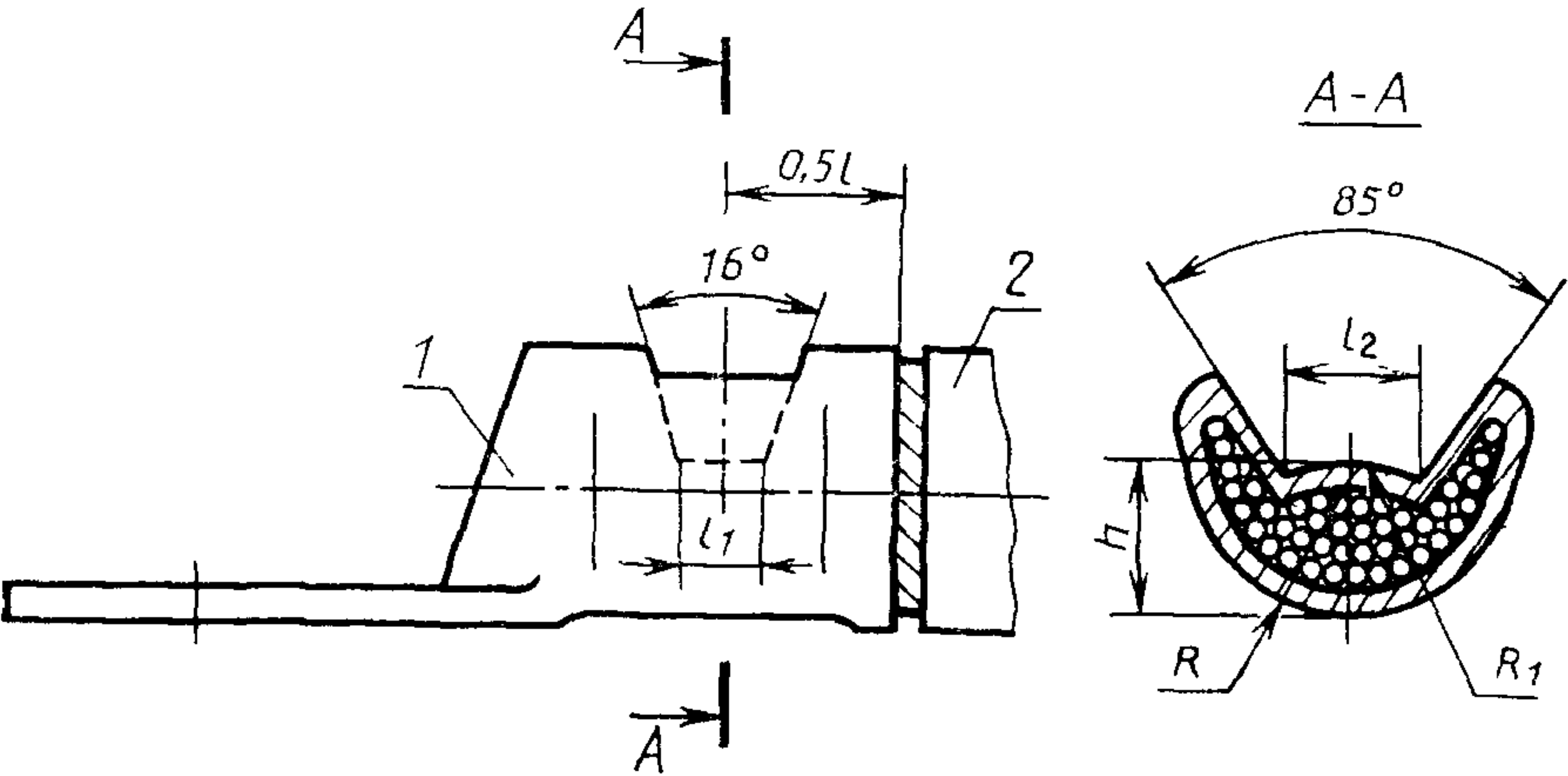
1—наконечник; 2—кабель.
