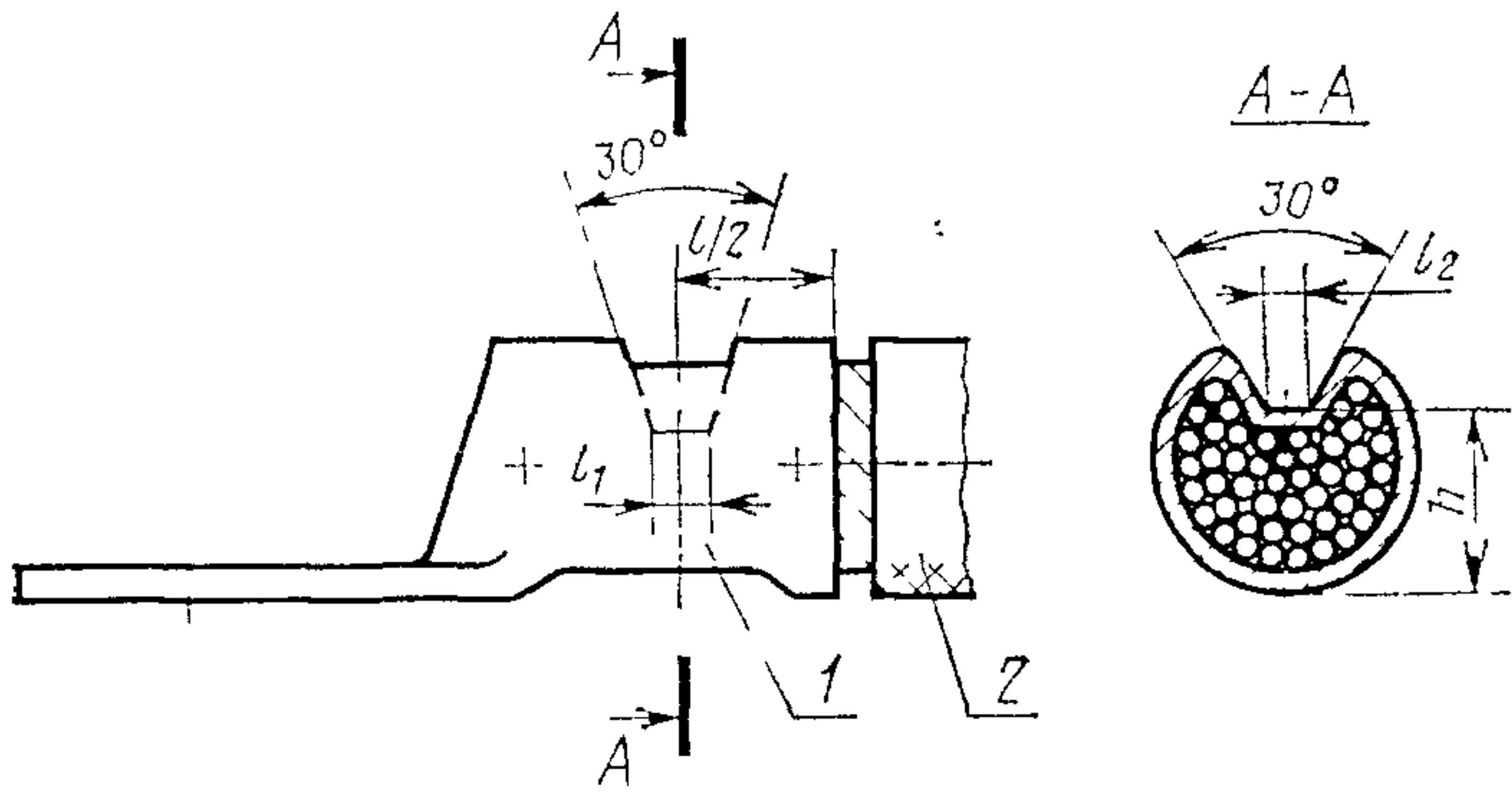
1—наконечник; 2—кабель. Черт. 1
