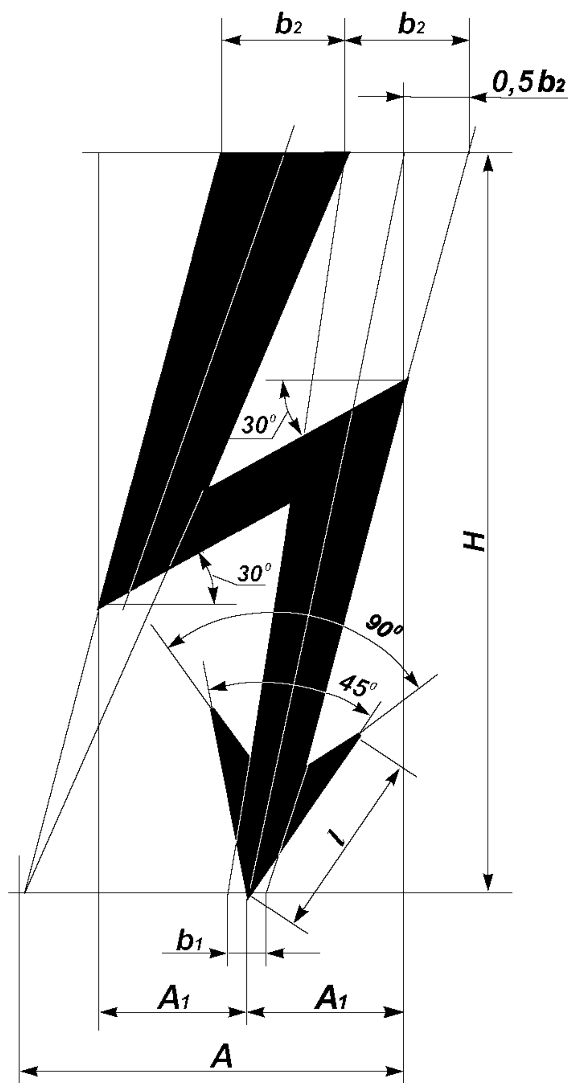
Рисунок Л.1 — Графический символ электрического напряжения
