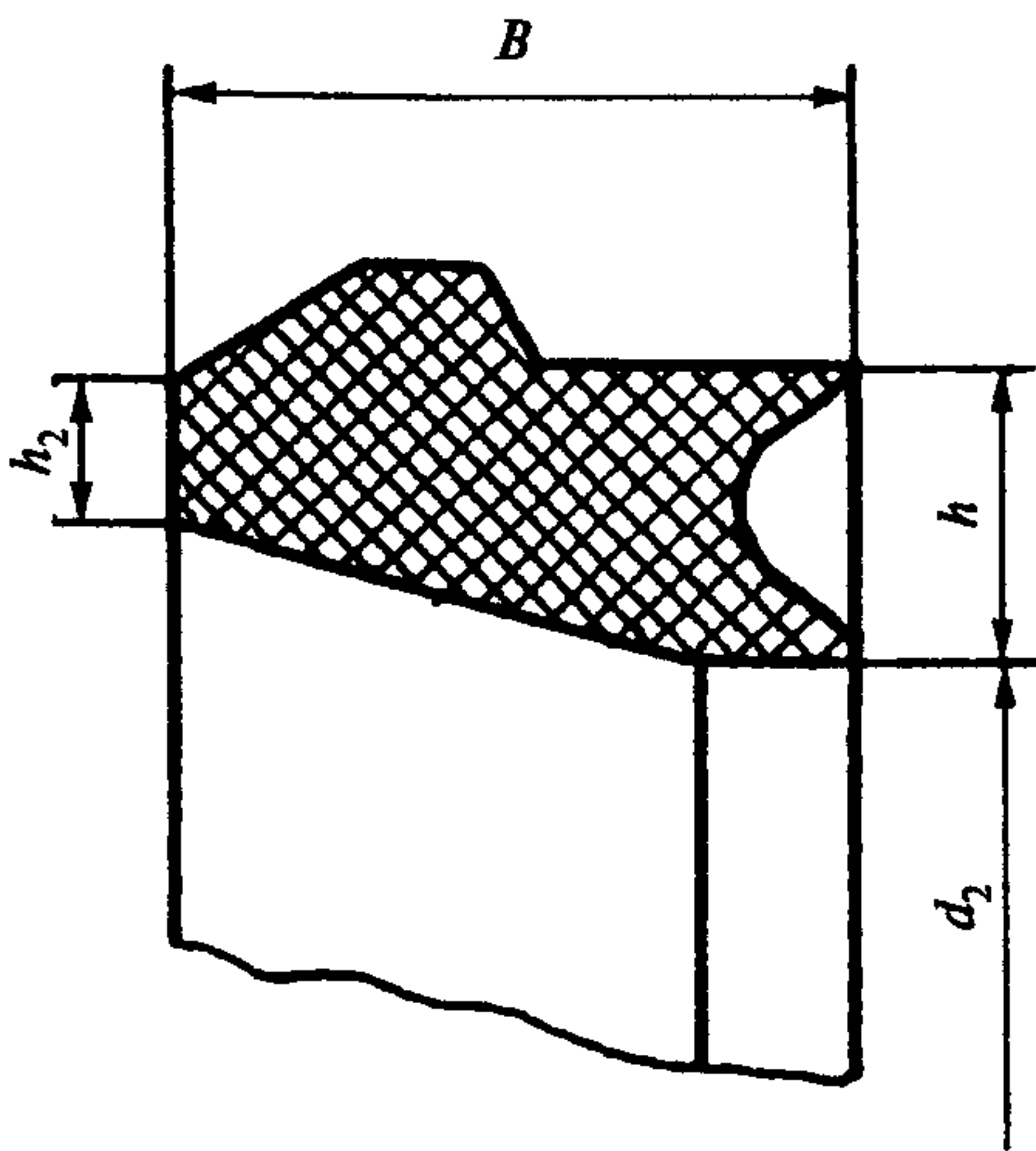
Рисунок 7 — Резиновое кольцо (размеры по таблице 10)
