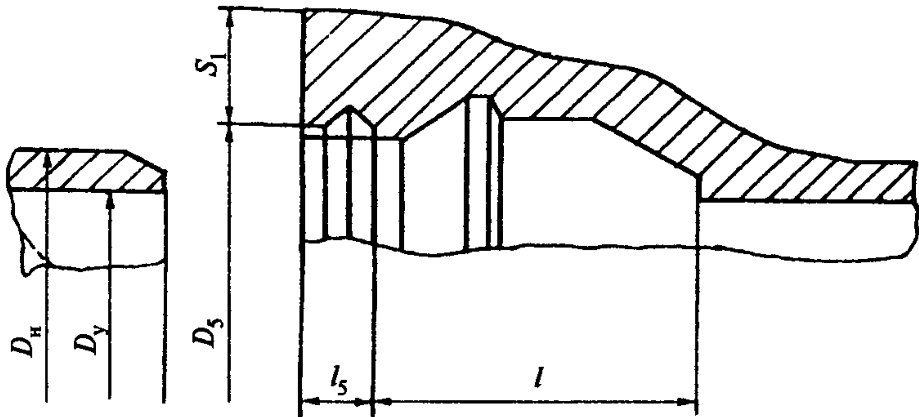
Рисунок 6 — Раструбное соединение труб диаметром 400 мм (размеры по таблице 9)
