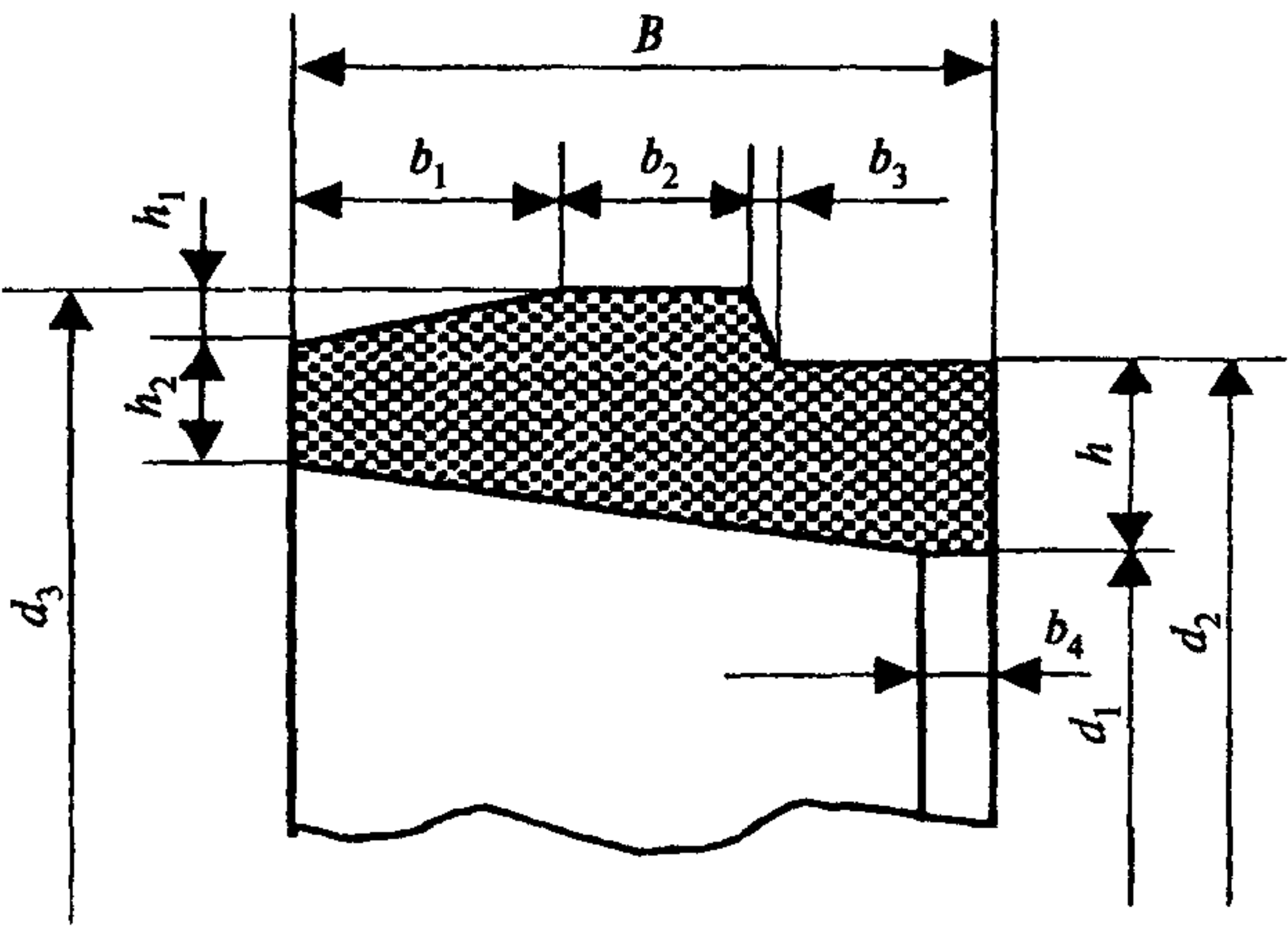
Рисунок 2 — Универсальное резиновое кольцо к раструбным соединениям (рисунок 1а, размеры по таблице 5)
