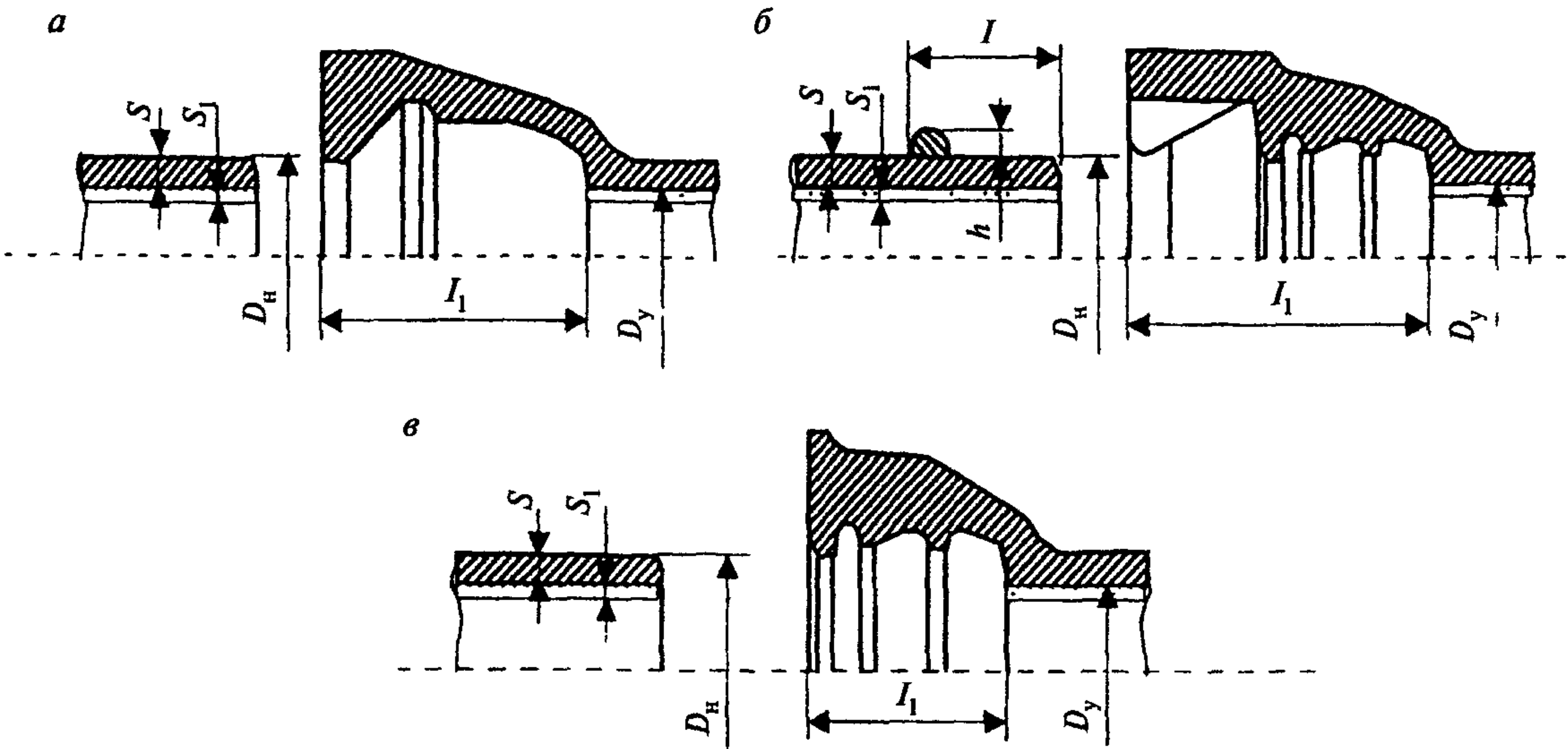
а — соединение под универсальное резиновое кольцо; б — соединение ВРС; в — соединение ВР
