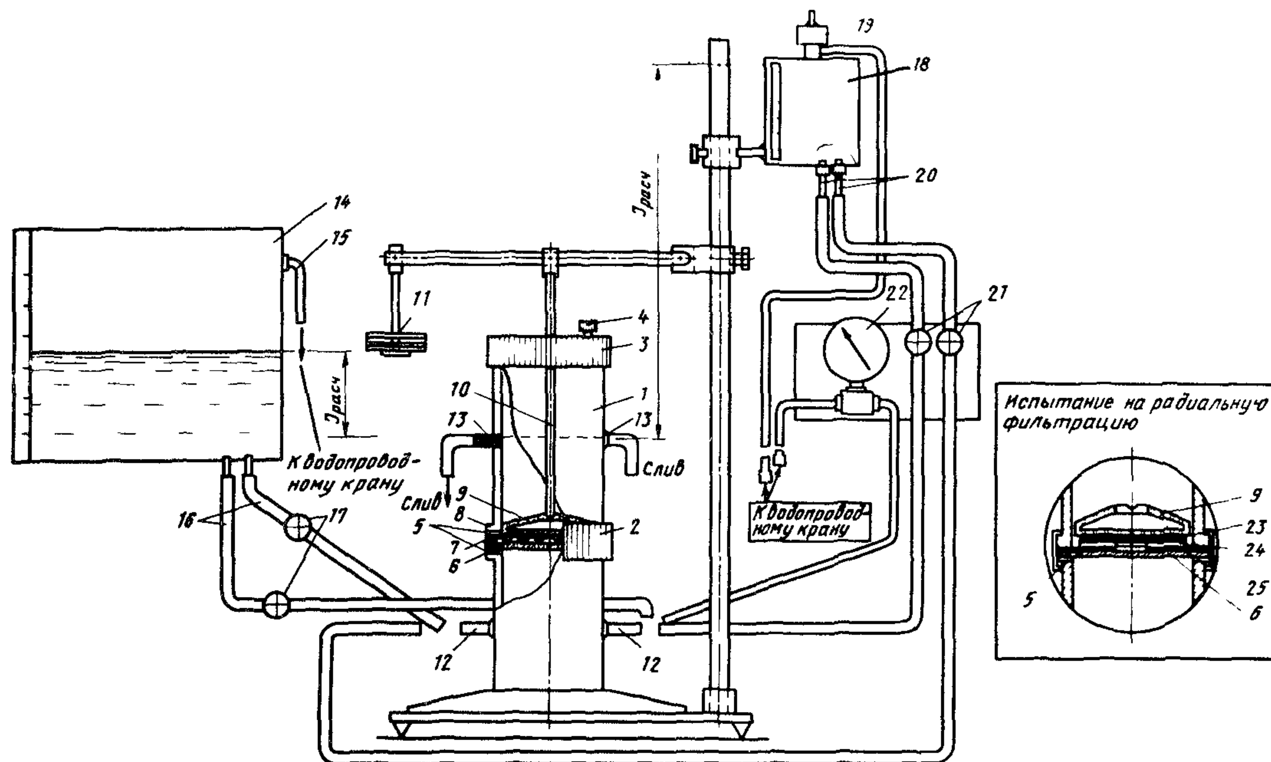
Рис.1. Схема фильтрационного прибора: 1-корпус прибора; 2-среднее кольцо; 3-верхнее кольцо; 4-воздушный клапан; 5-уплотнительное резиновое кольцо; 6-перфорированный диск; 7-образец геотекстиля диаметром 130 мм; 8-сетка; 9-перфорированный штамп; 10-шток; 11-нагрузка; 12-нижние штуцера; 13-верхние штуцера; 14-водомерный бак; 15-наливной штуцер; 16-сливные штуцера; 17-кран; 18-малый водомерный бак; 19-запорный клапан; 20-сливные штуцера; 21-кран; 22-манометр; 23-резиновый диск диаметром 90 мм; 24-образец геотекстиля диаметром 90 мм с отверстием в центре диаметром 30 мм; 25-резиновый диск диаметром 130 мм с отверстием в центре диаметром 30 мм
