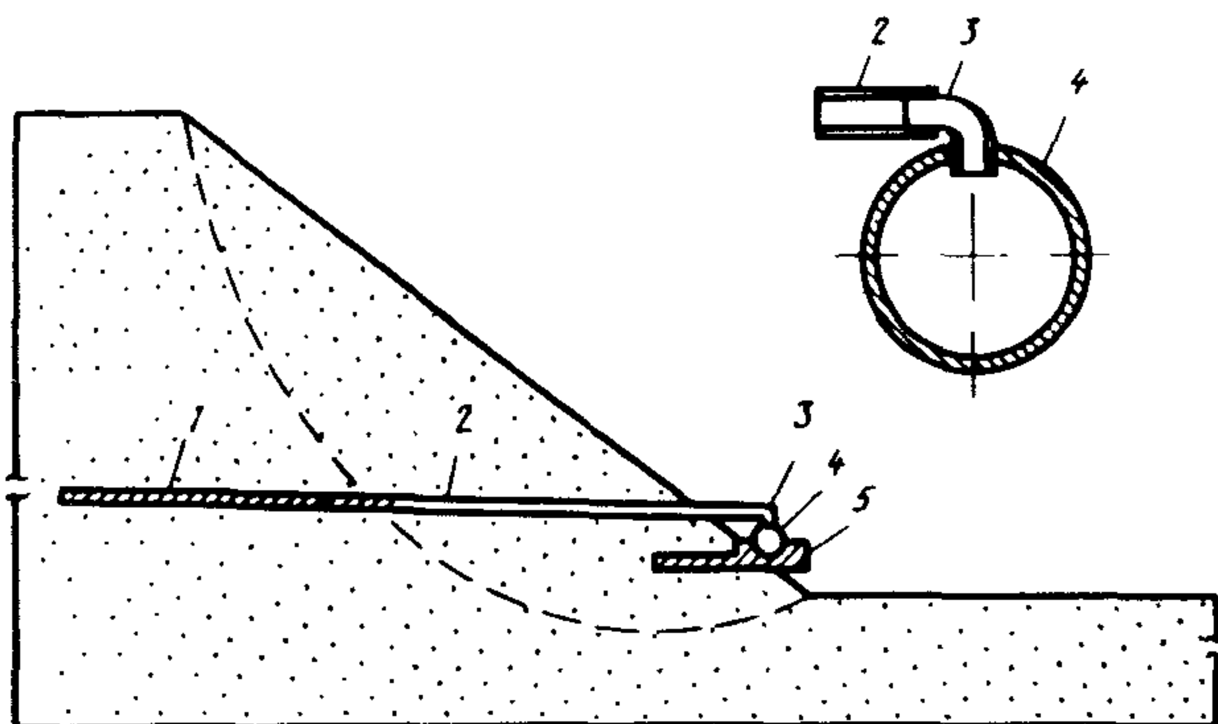
Рис.9. Сброс грунтовых вод по коллектору: 1-водоприемная часть дрены; 2-водоотводная часть дрены; 3-переходник; 4-коллектор; 5-опора
