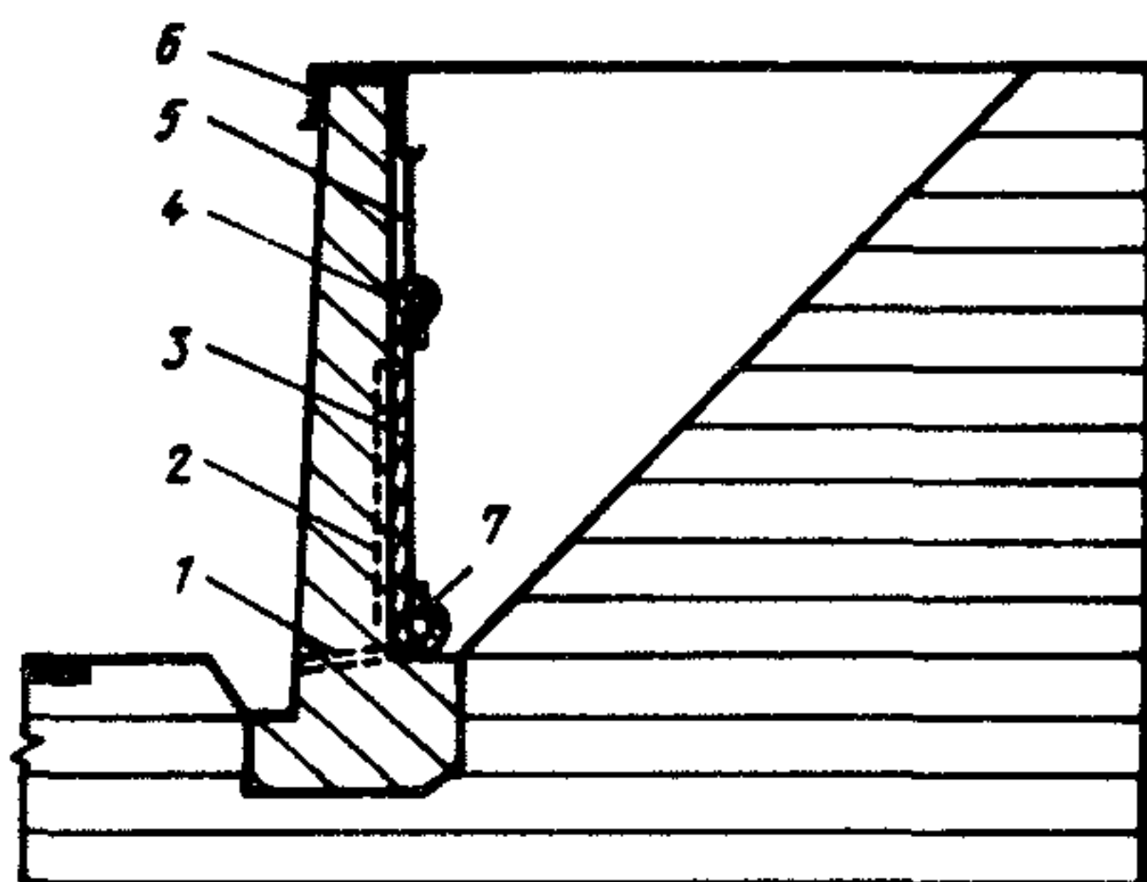
Рис.4. Схема навешивания полотнища из геотекстильного материала: 1-дренажное окно; 2-канал; 3-геотекстиль; 4-стержень, 5-трос; 6-скоба
