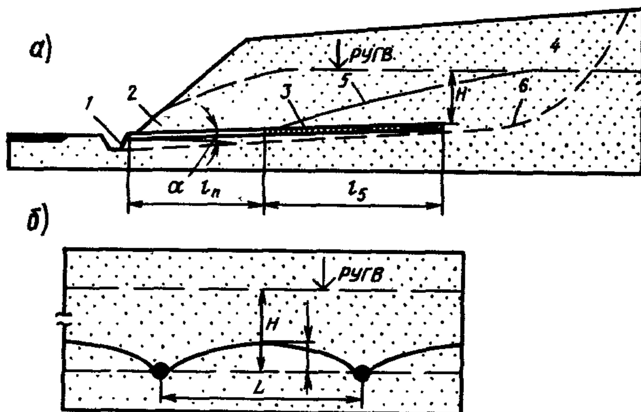
Рис.3. Схема бестраншейного горизонтального дренажа: 1-лоток; 2-водоотводная часть дрены; 3-водоприемная часть дрены; 4-грунт; 5-уровень грунтовых вод после осушения грунтового массива; 6-поверхность скольжения
