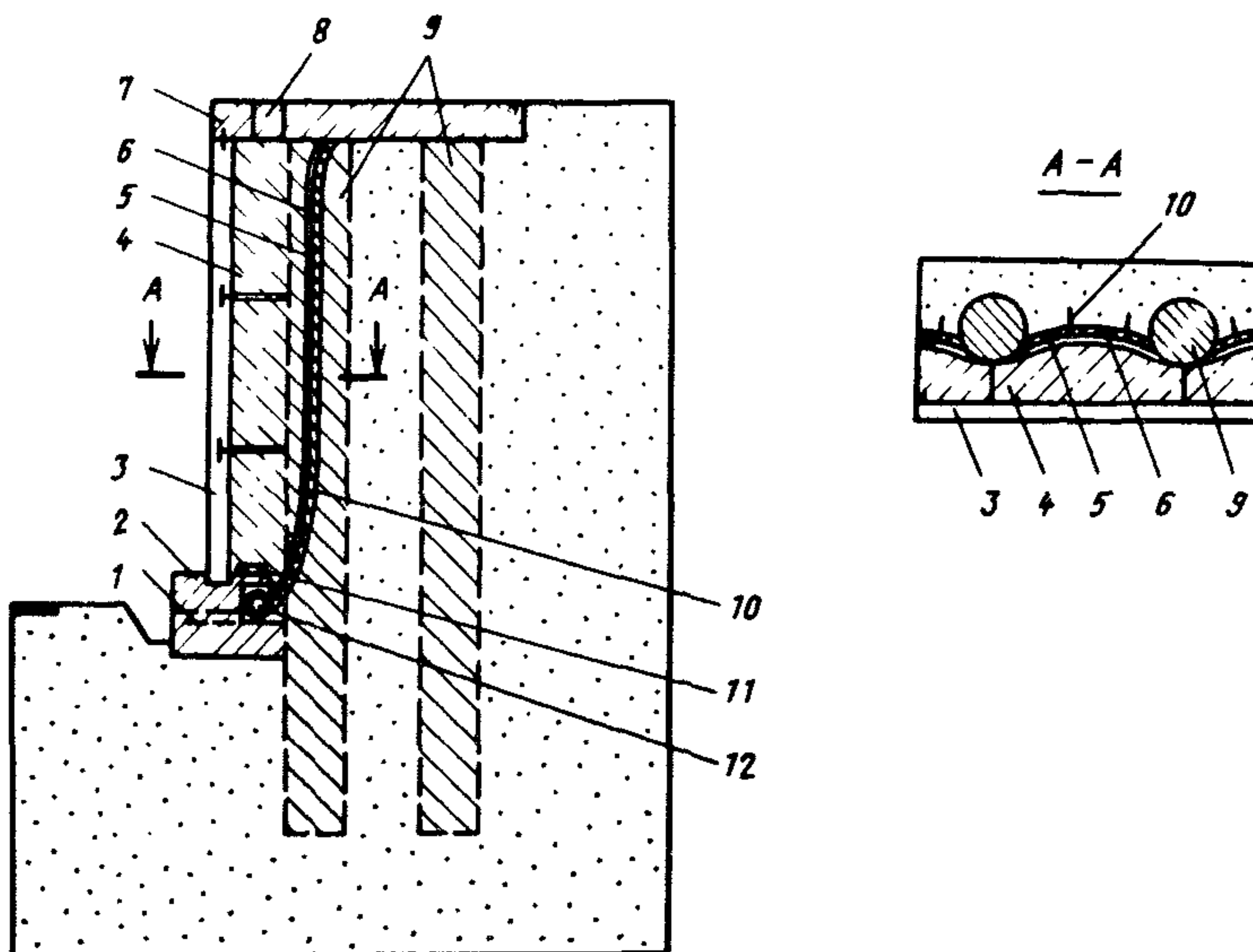
Рис.7. Застенный дренаж в конструкциях из буронабивных свай с монолитной облицовочной стенкой: 1-дренажное окно; 2-брус; 3-опалубка; 4-бетон; 5-пленка; 6-геотекстиль; 7-ростверк; 8-отверстие; 9-сваи; 10-штырь; 11-слой битума; 12-дренажная труба
