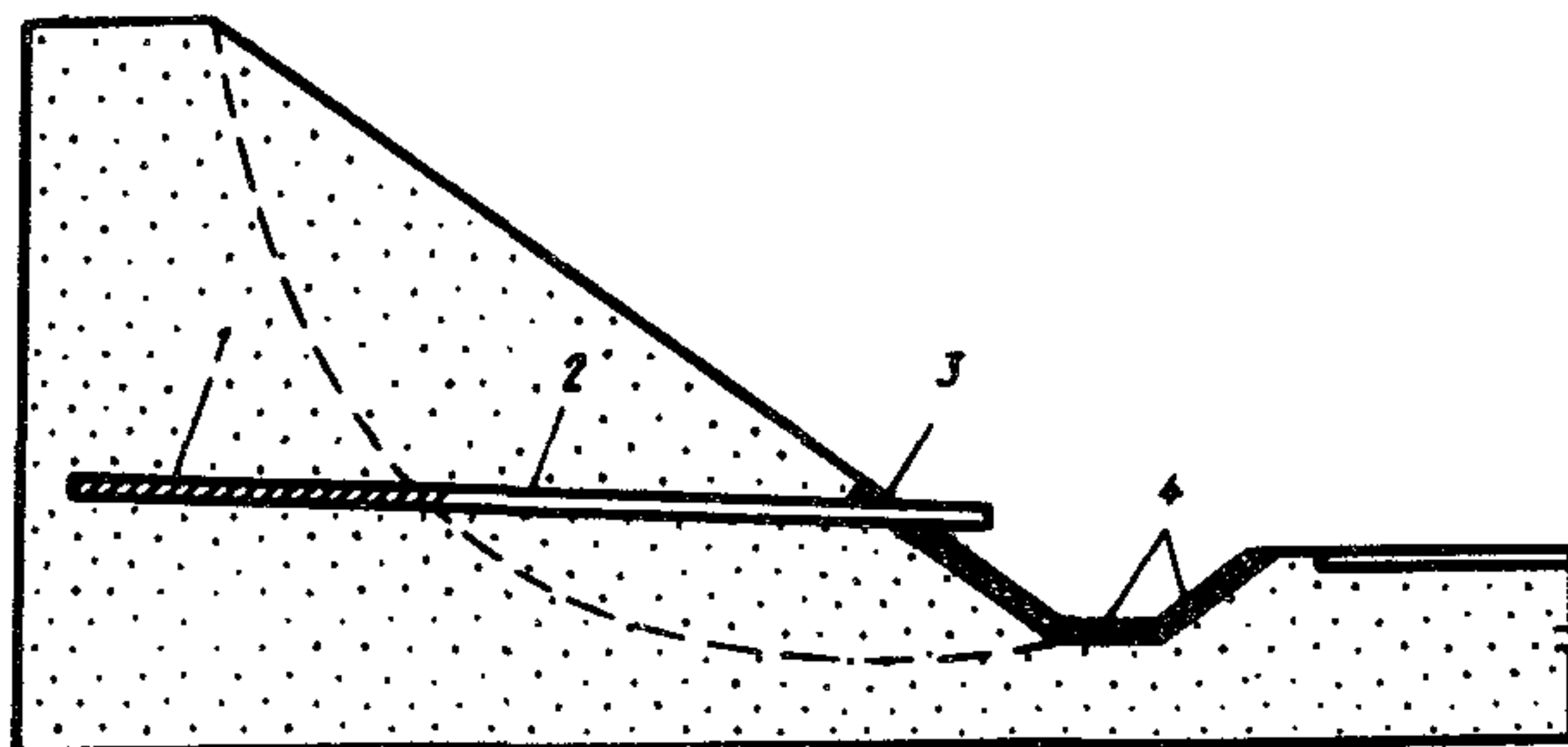
Рис.8. Прямое примыкание дрен к водоотводному лотку: 1-водоприемная часть дрены; 2-водоотводная часть дрены; 3-оголовок; 4-плитки
