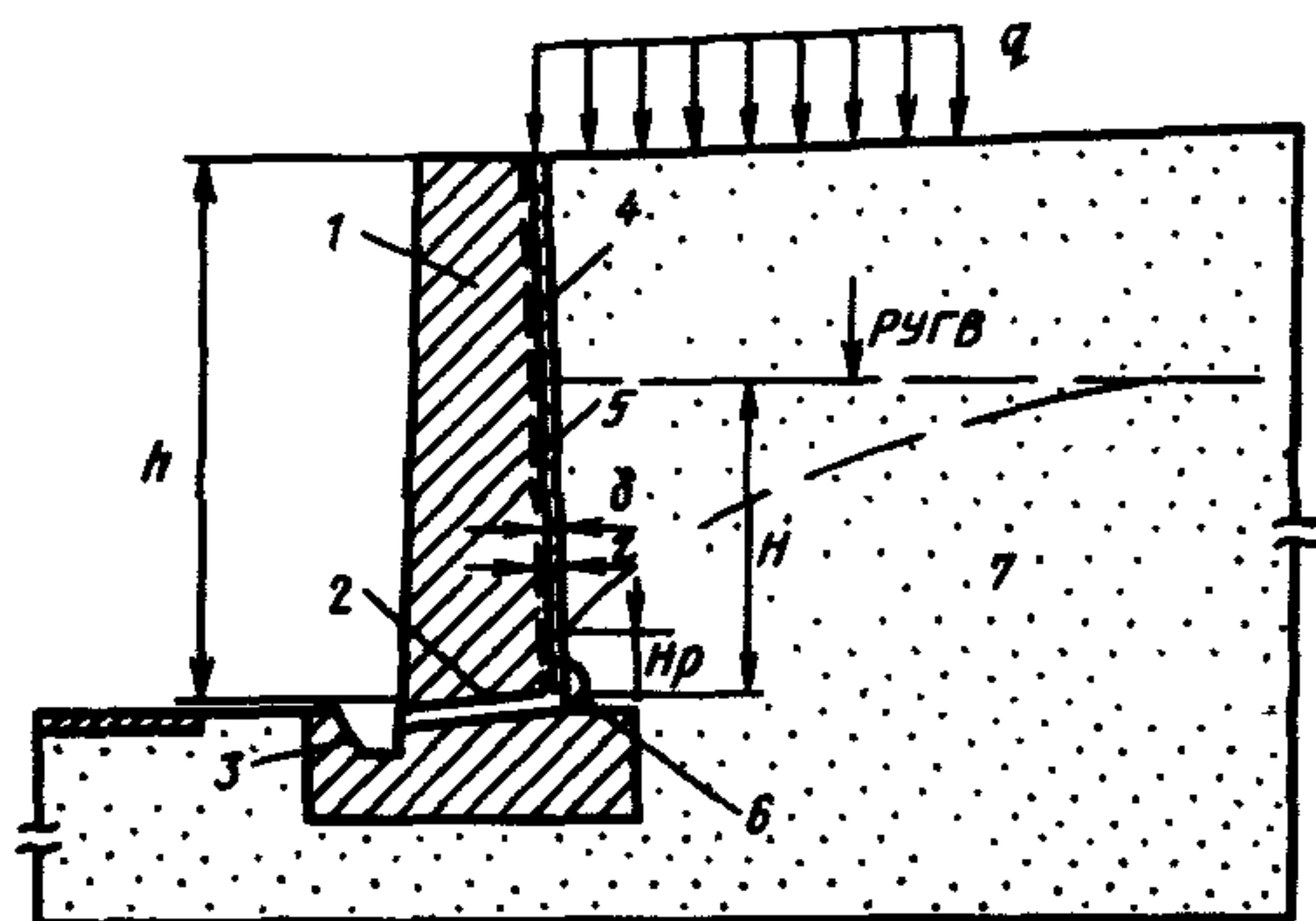
Рис.2. Схема застенного дренажа: 1-подпорная стена; 2-дренажное окно; 3-лоток; 4-канал; 5-геотекстиль; 6-дренажная труба; 7-грунт
