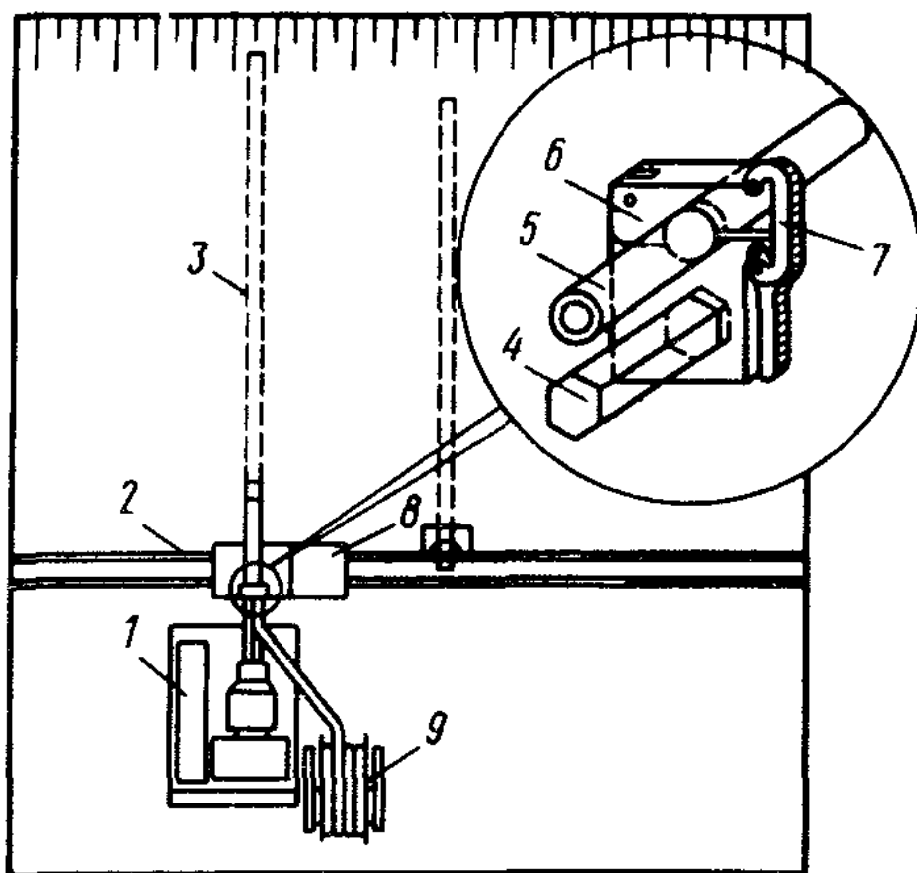
Рис.11. Схема установки дрены в скважину; 1–буровой станок; 2–лоток; 3–скважина; 4–переходник к буровому станку; 5–дрена; 6–зажим; 7–ключ; 8–щит; 9–бухтодержатель
