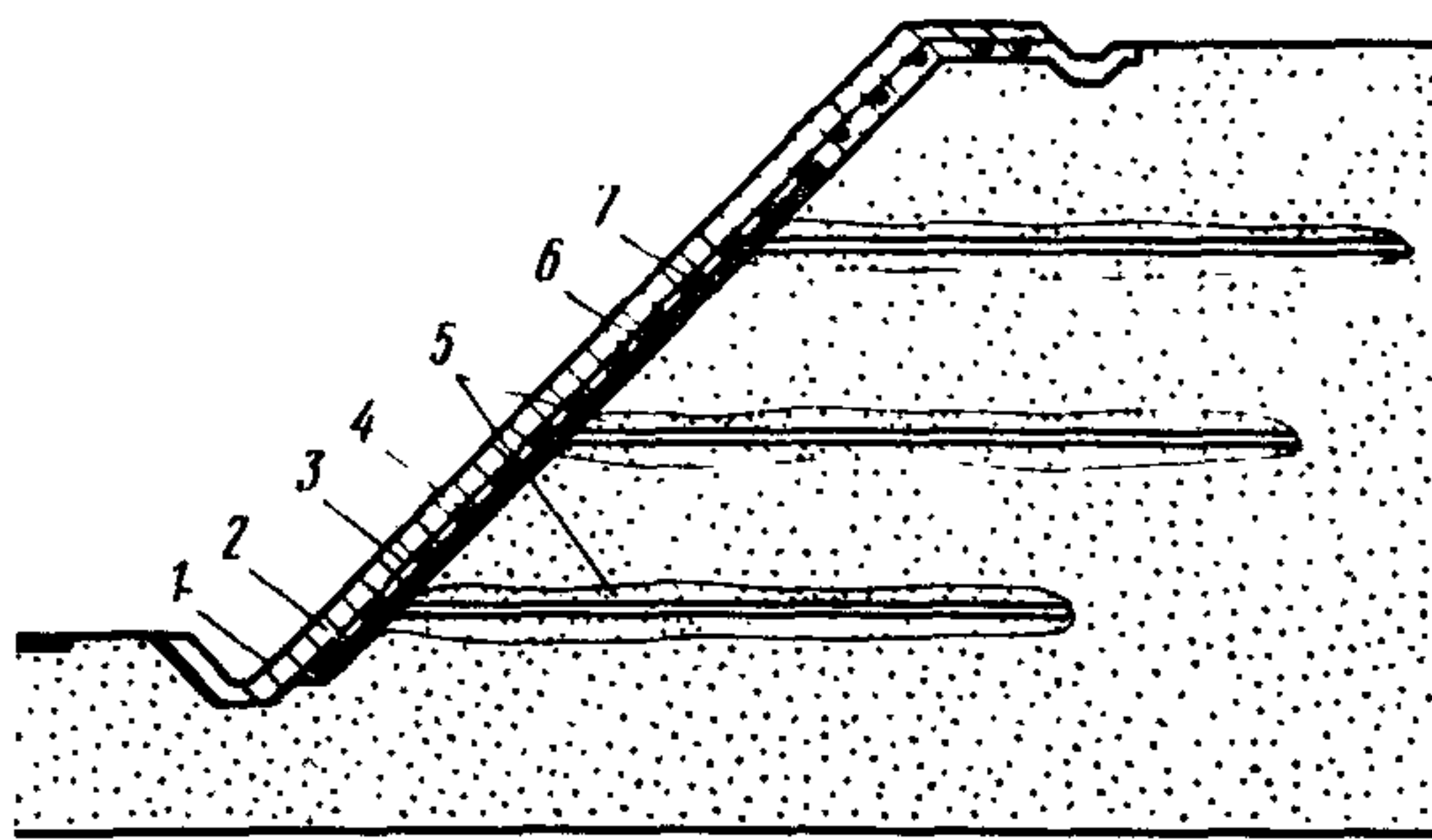
Рис.1. Схема нагельной конструкции: 1-лоток; 2-дренажное окно; 3-покрытие; 4-арматурная сетка; 5-нагели; 6-прослойка из водонепроницаемого материала; 7-геотекстильный материал
