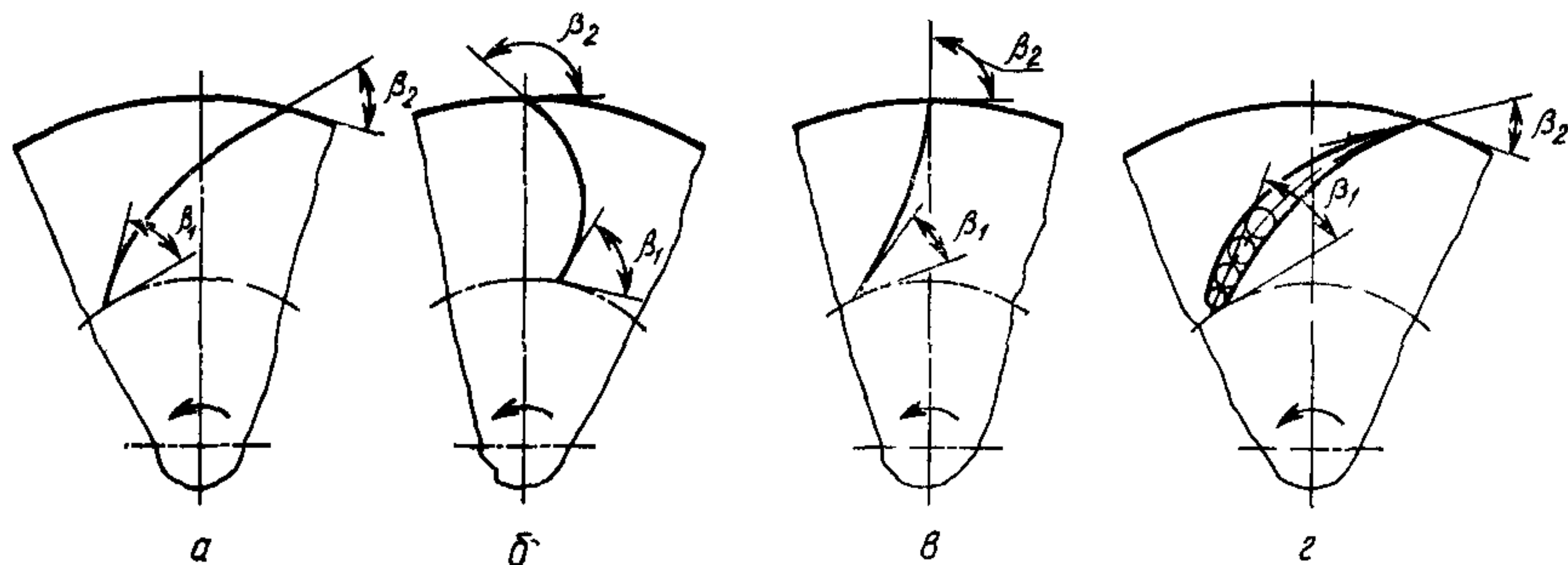
a — лопатки, загнутые назад ( \beta_2 < 90^\circ ), б — лопатки, загнутые вперед ( \beta_2 > 90^\circ ); в — лопатки, радиально оканчивающиеся ( \beta_2 = 90^\circ ), г — профильная лопатка
