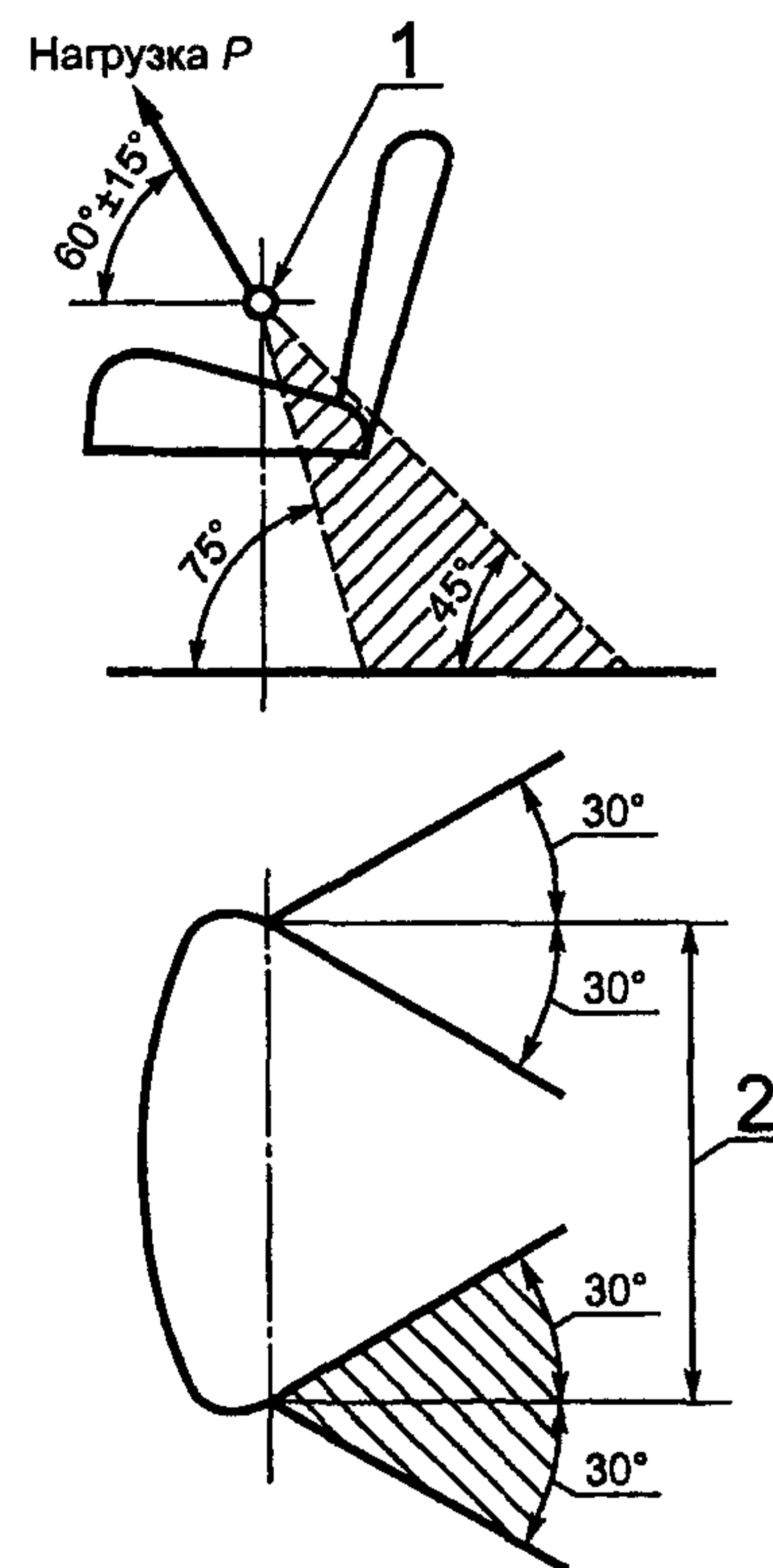
1 — контрольная точка сиденья — по ГОСТ 27715; 2 — ширина подушки
