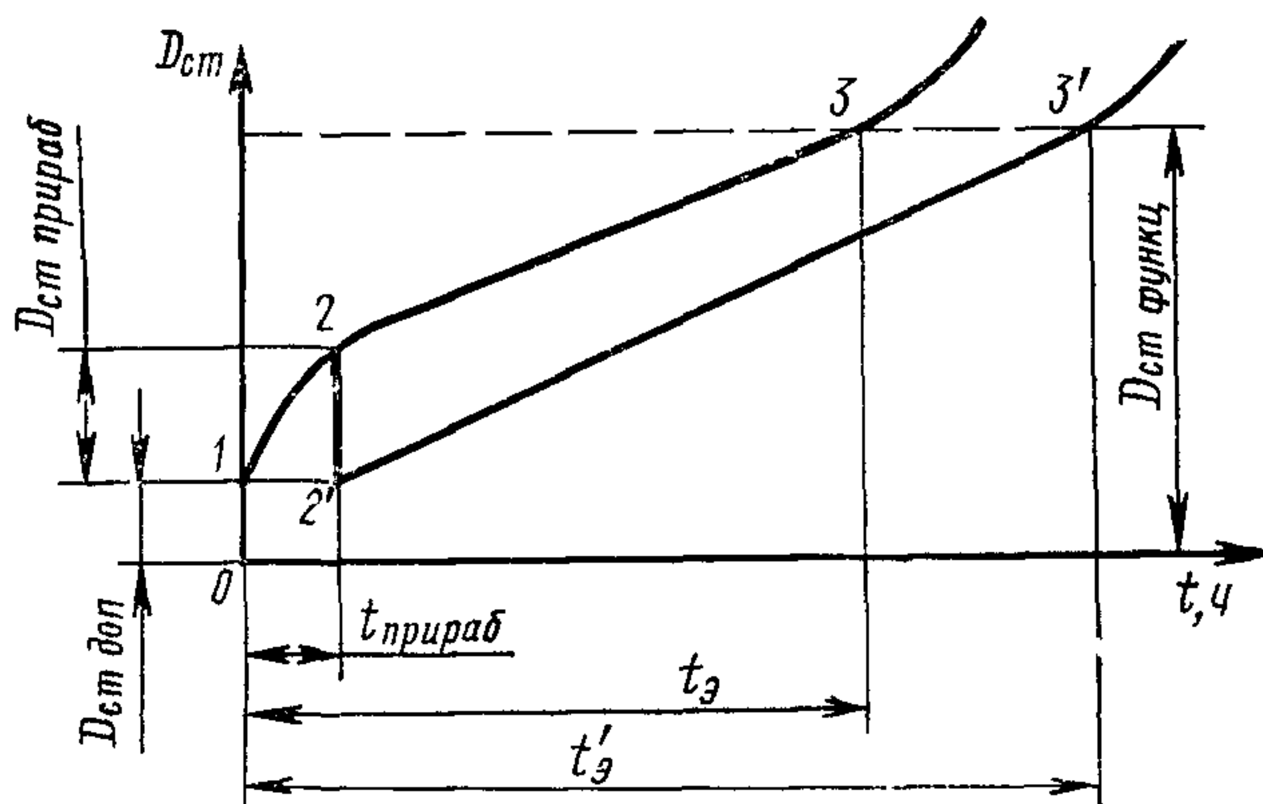
Черт. 48
