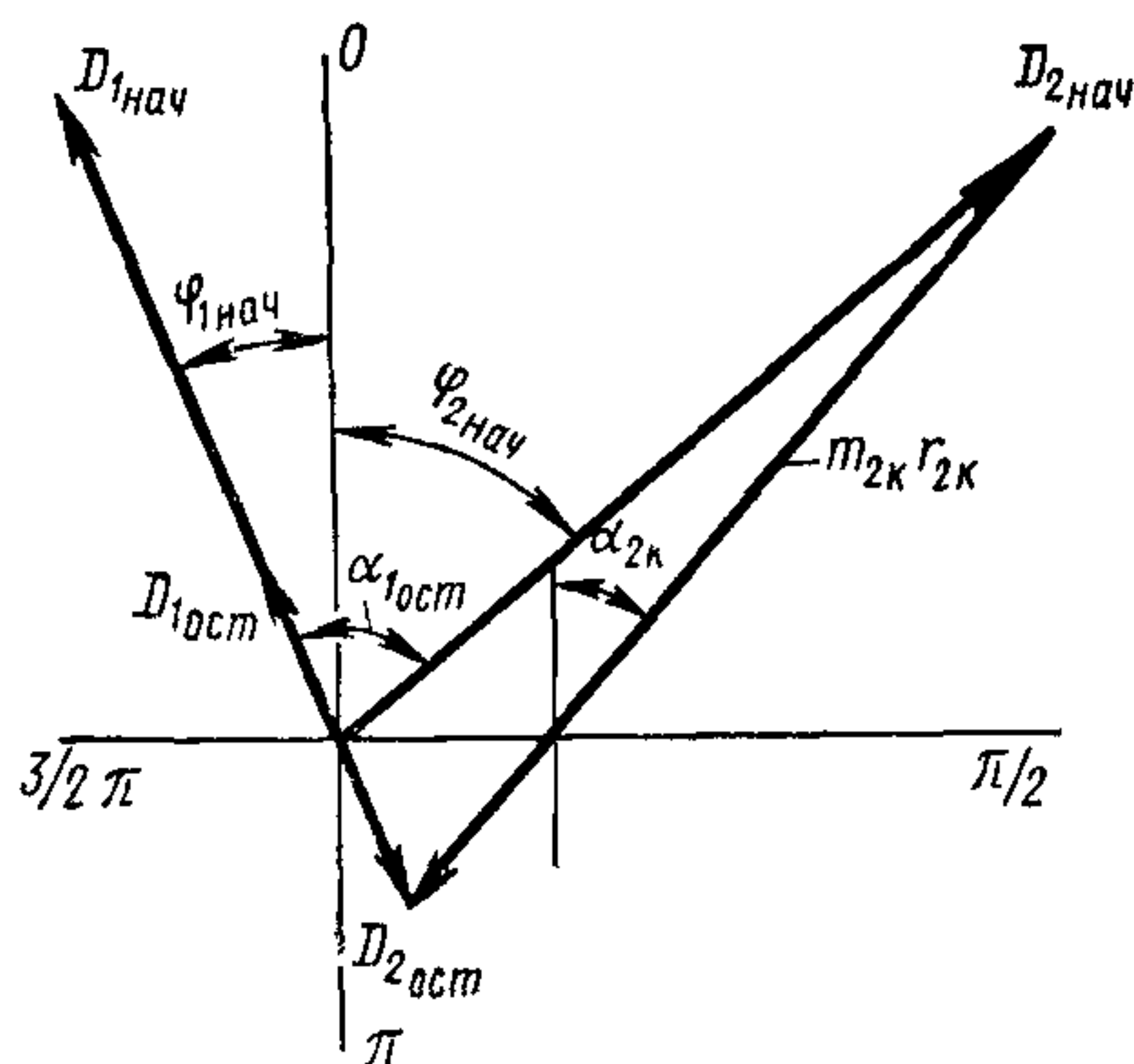
Черт. 52
