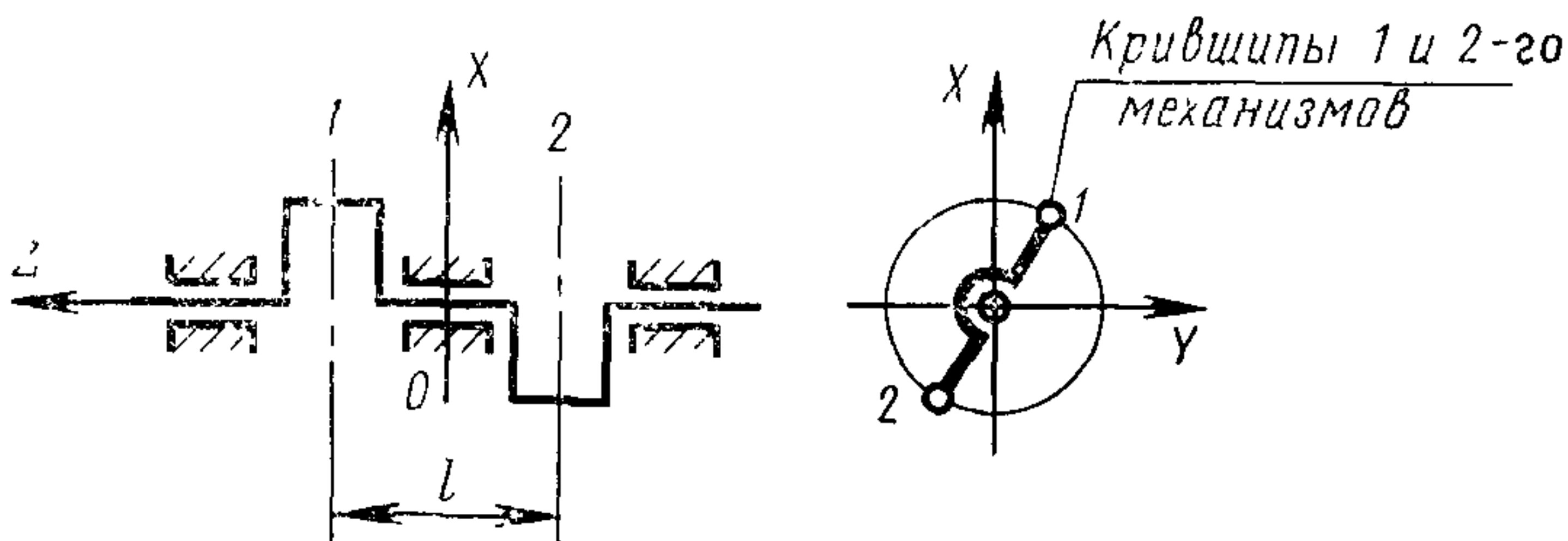
Черт. 17
