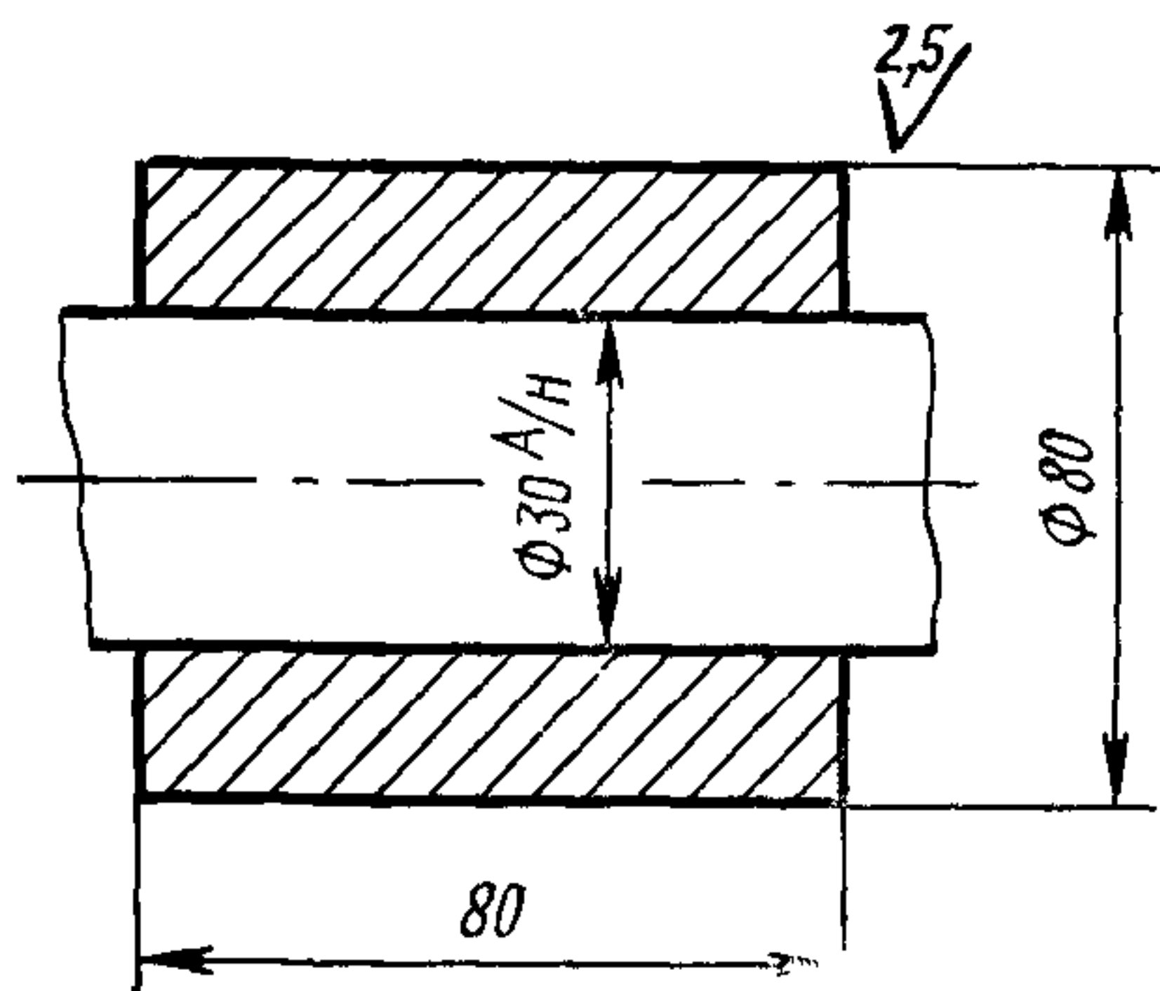
Черт. 44
