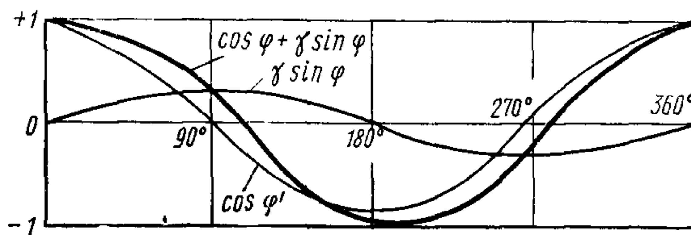
Черт. 24
