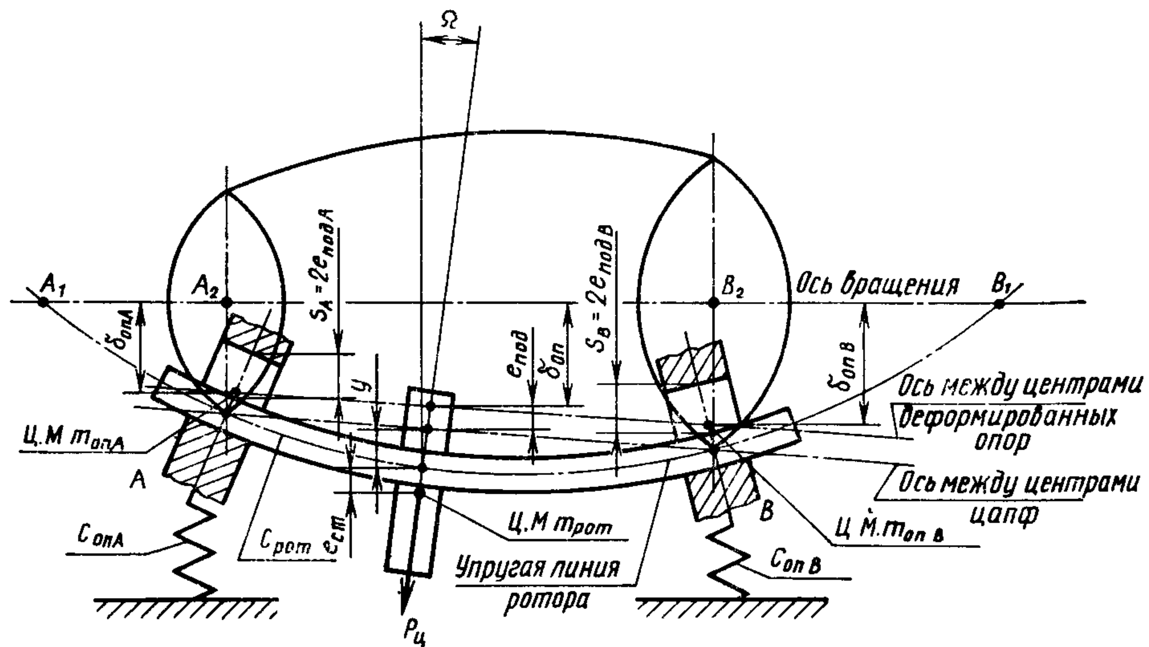
Черт. 28
