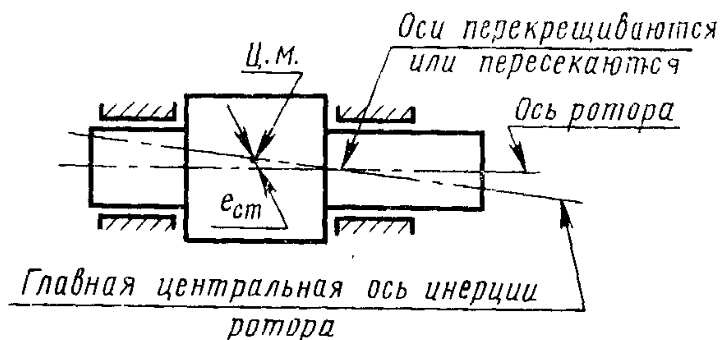
Черт. 1
