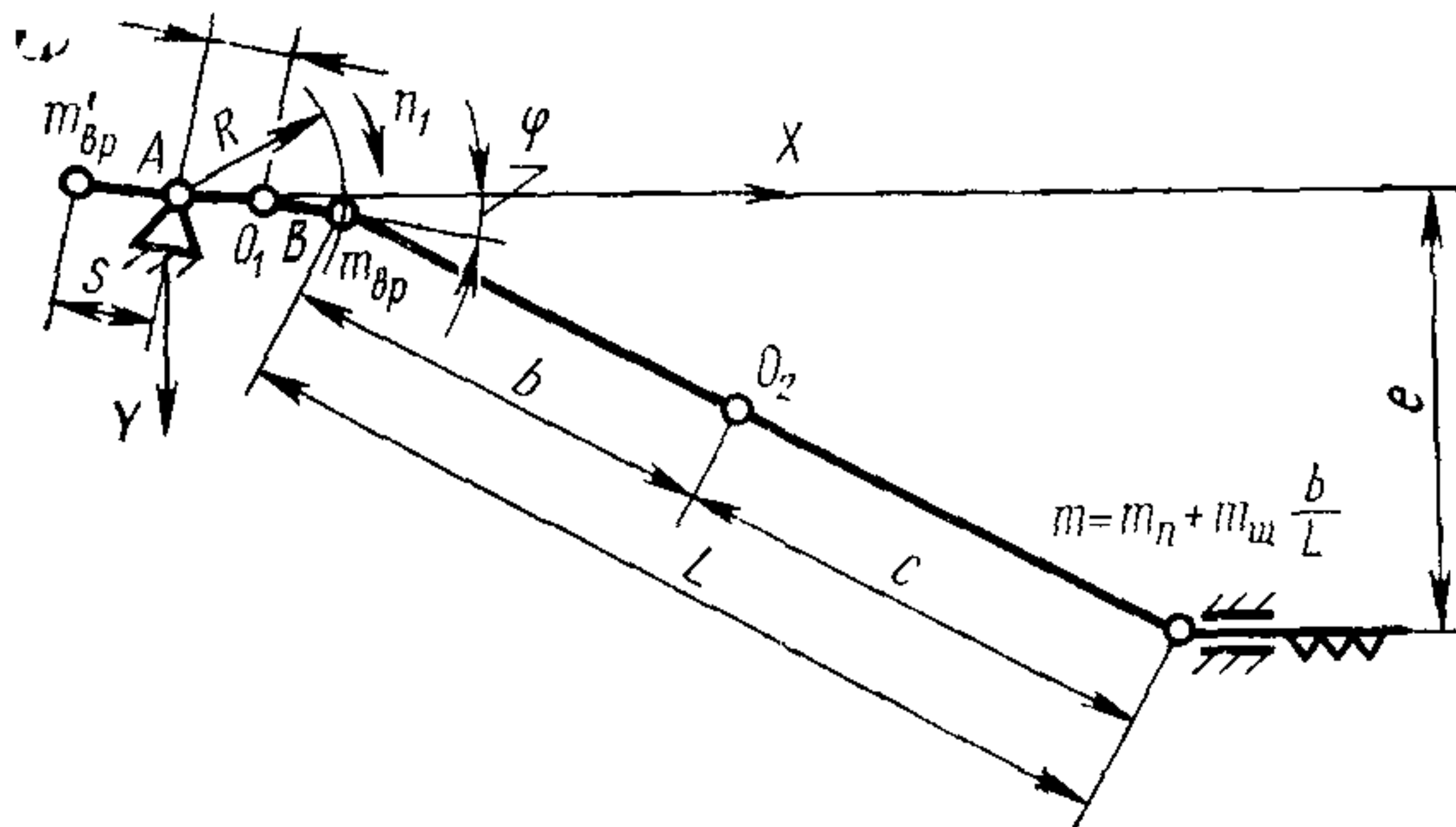
Черт. 23
