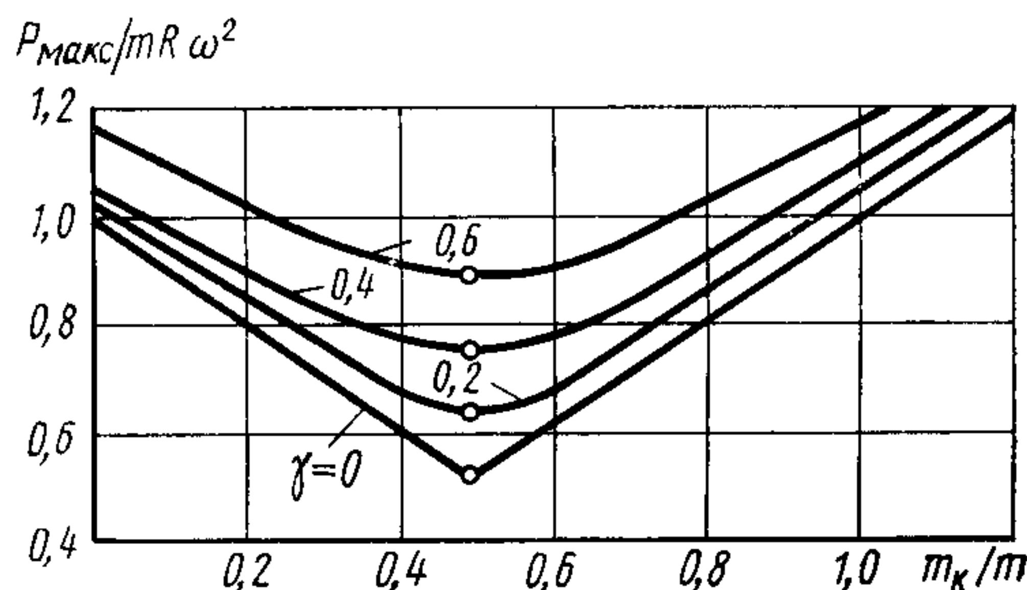
Черт. 26
