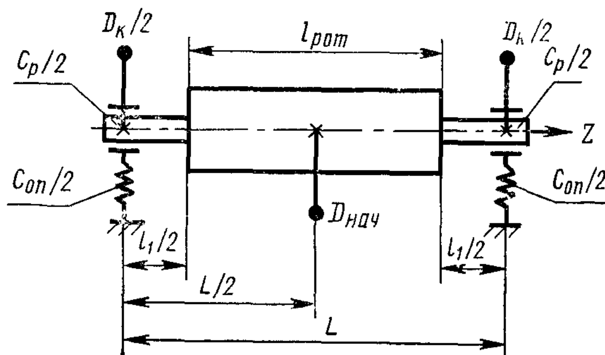
Черт. 32
