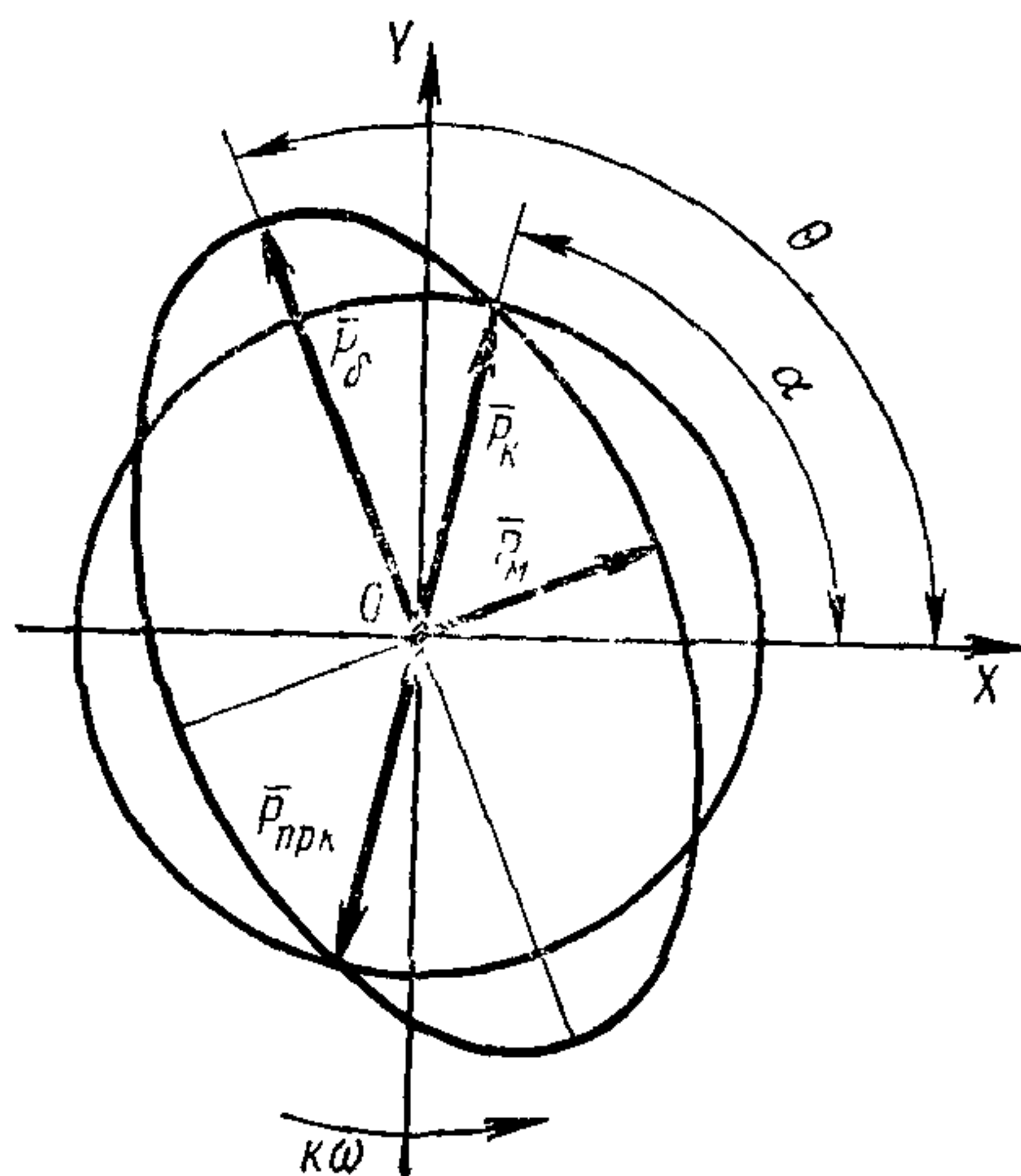
Черт. 22
