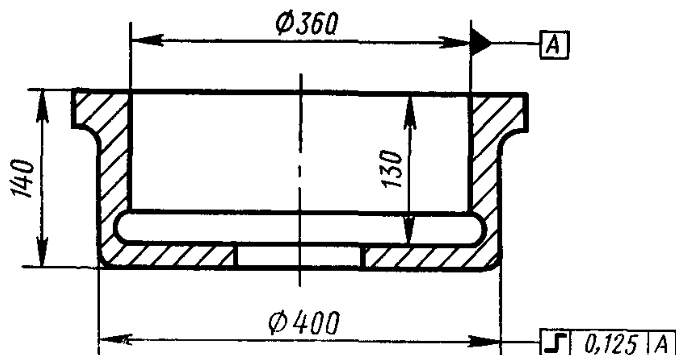
Черт. 49
