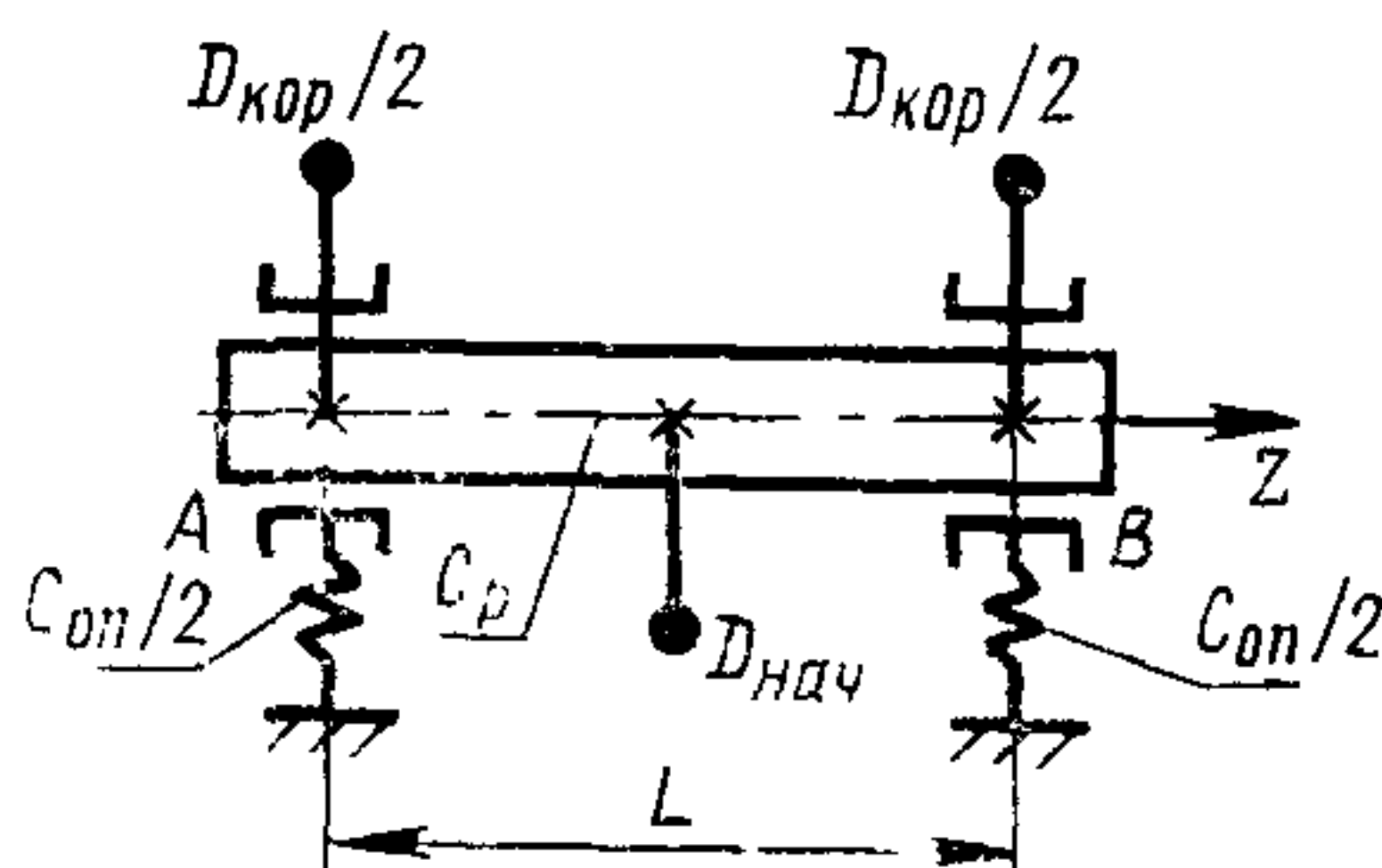
Черт. 33
