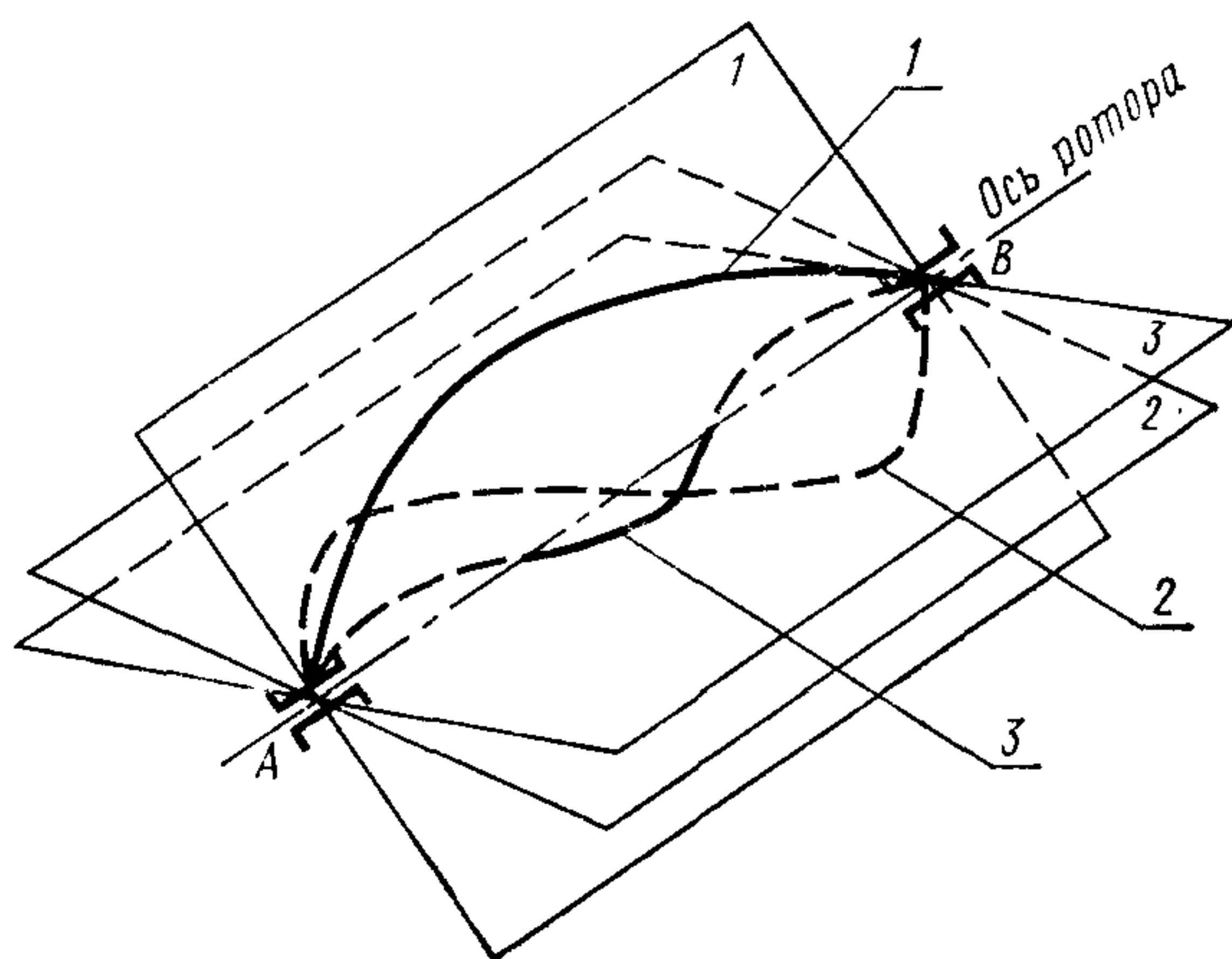
Черт. 30
