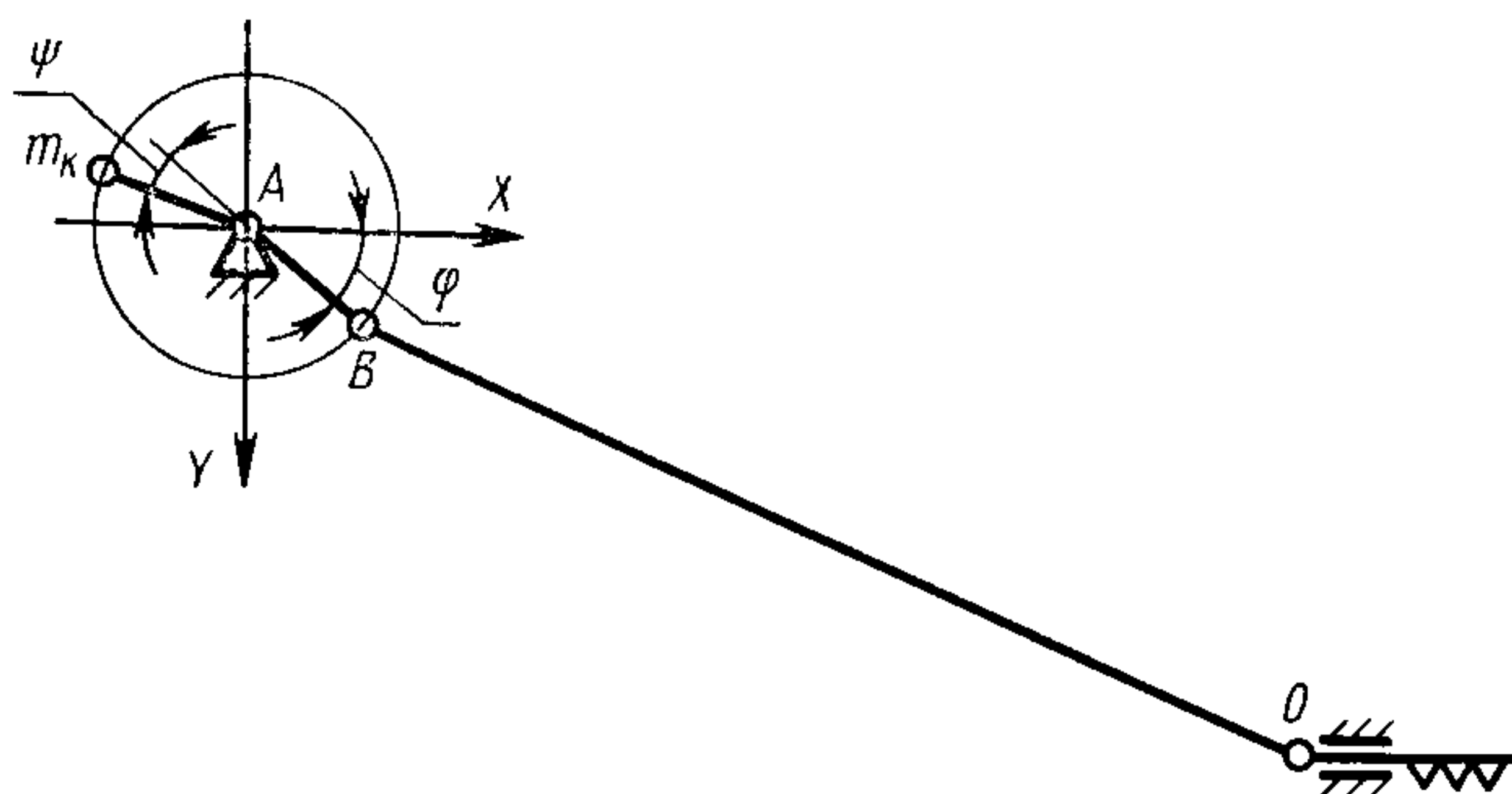
Черт. 27
