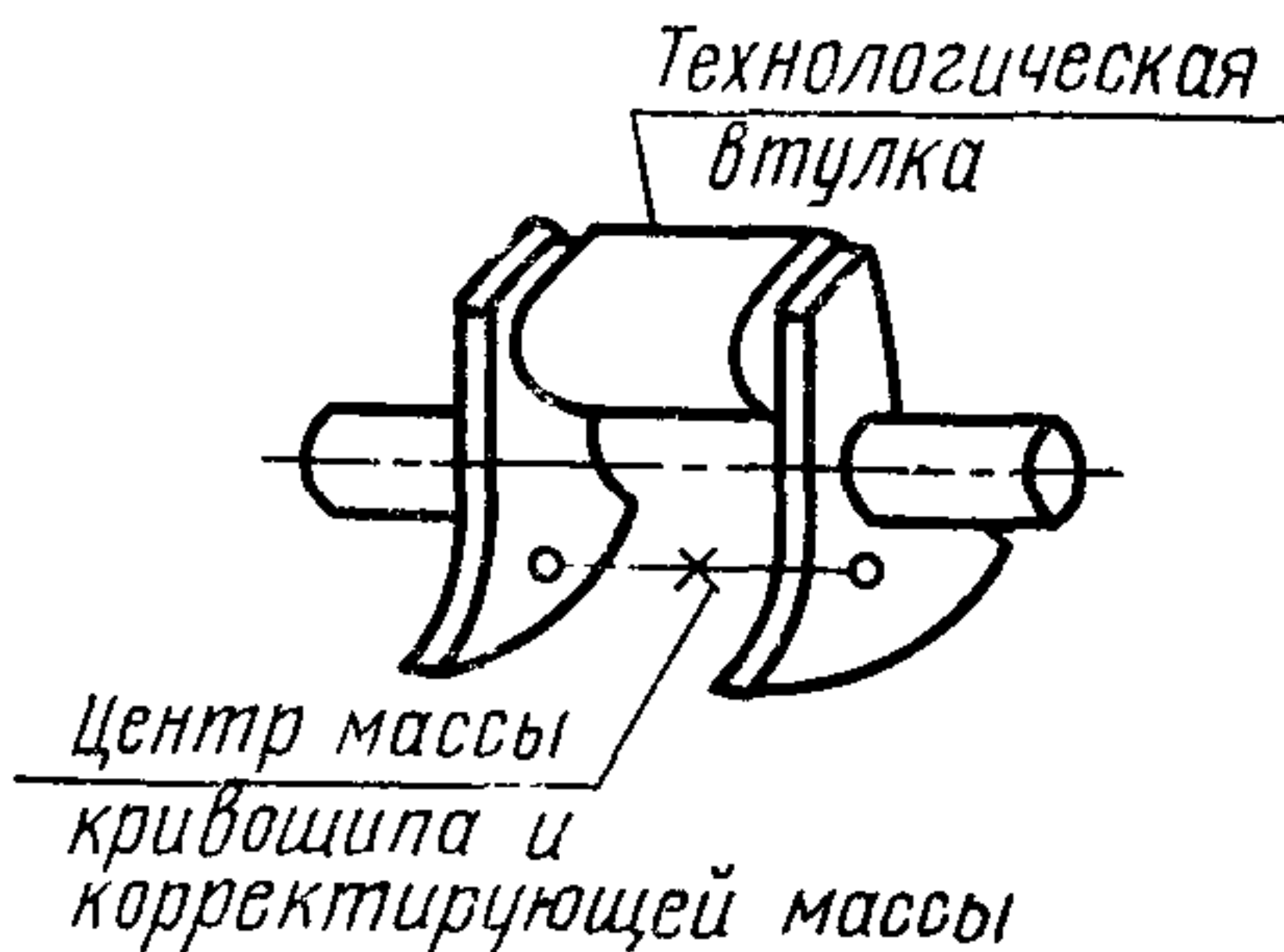
Черт. 18
