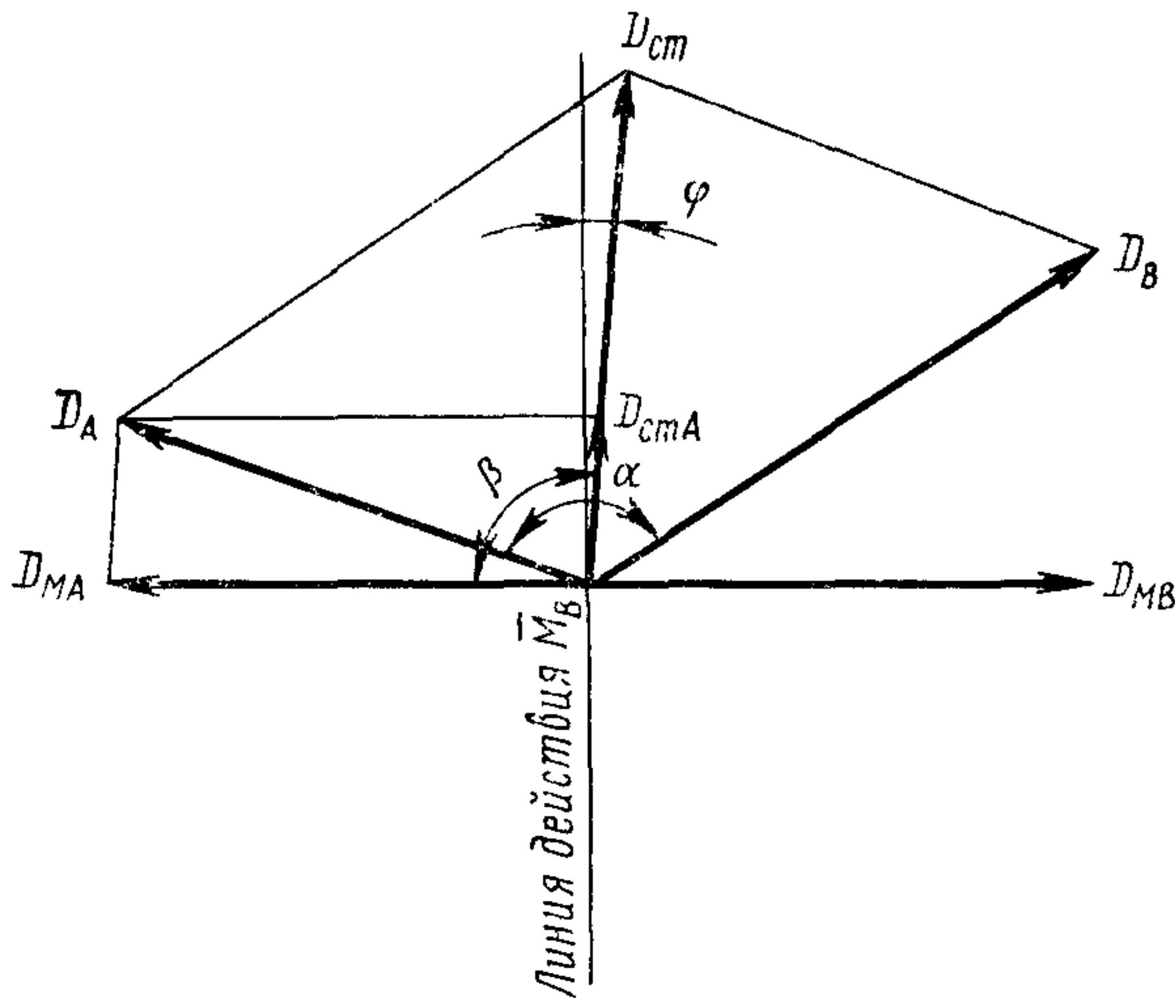
Черт. 6
