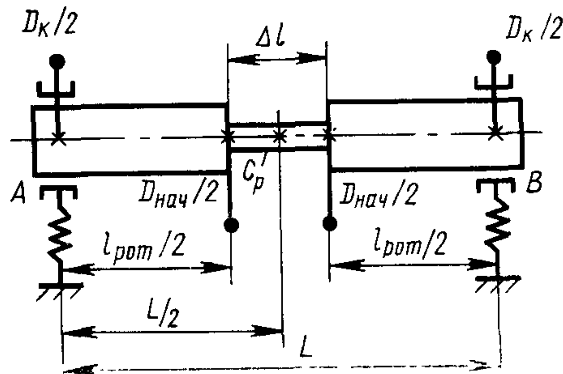
Черт. 34
