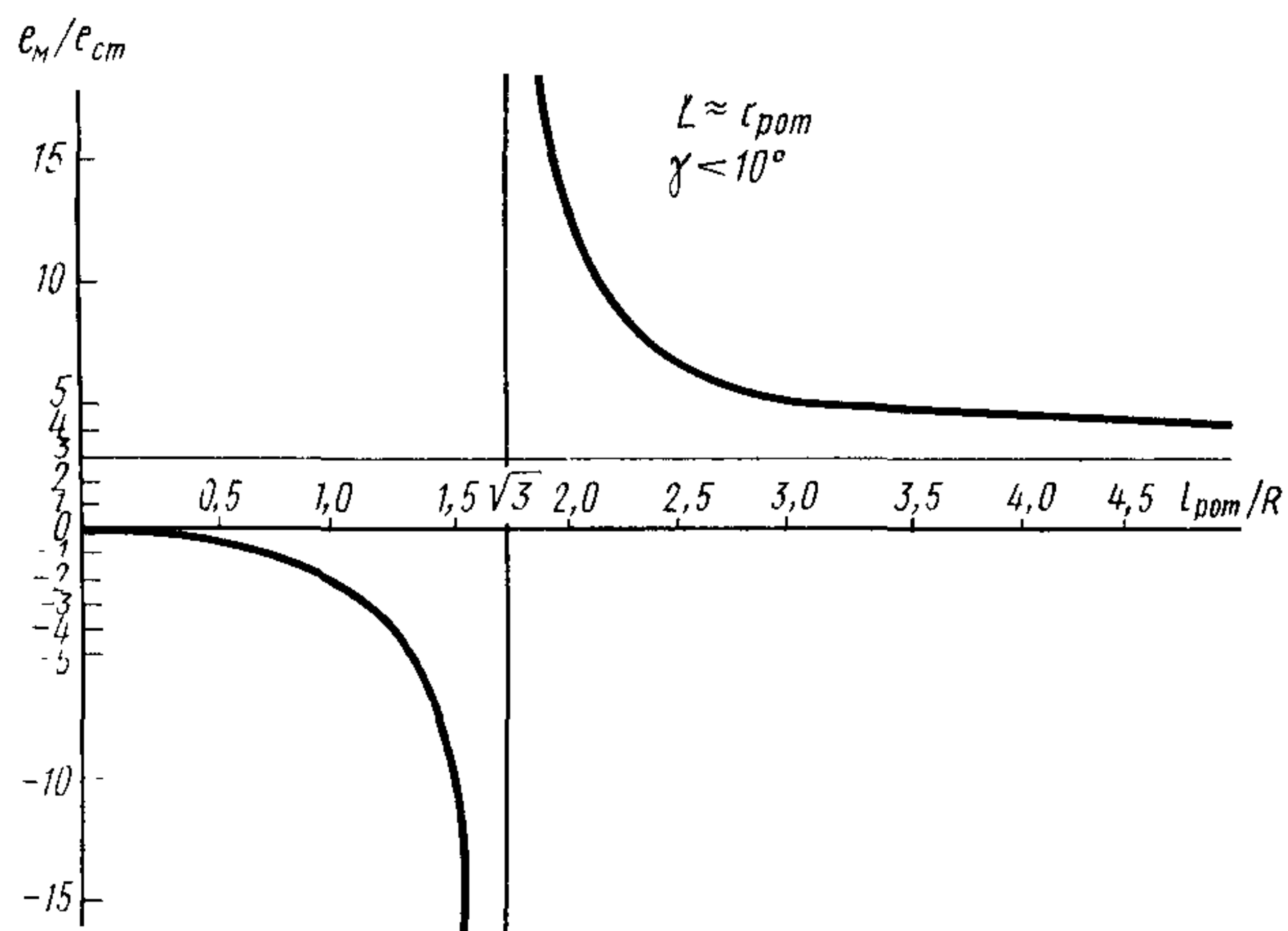
Черт. 8
