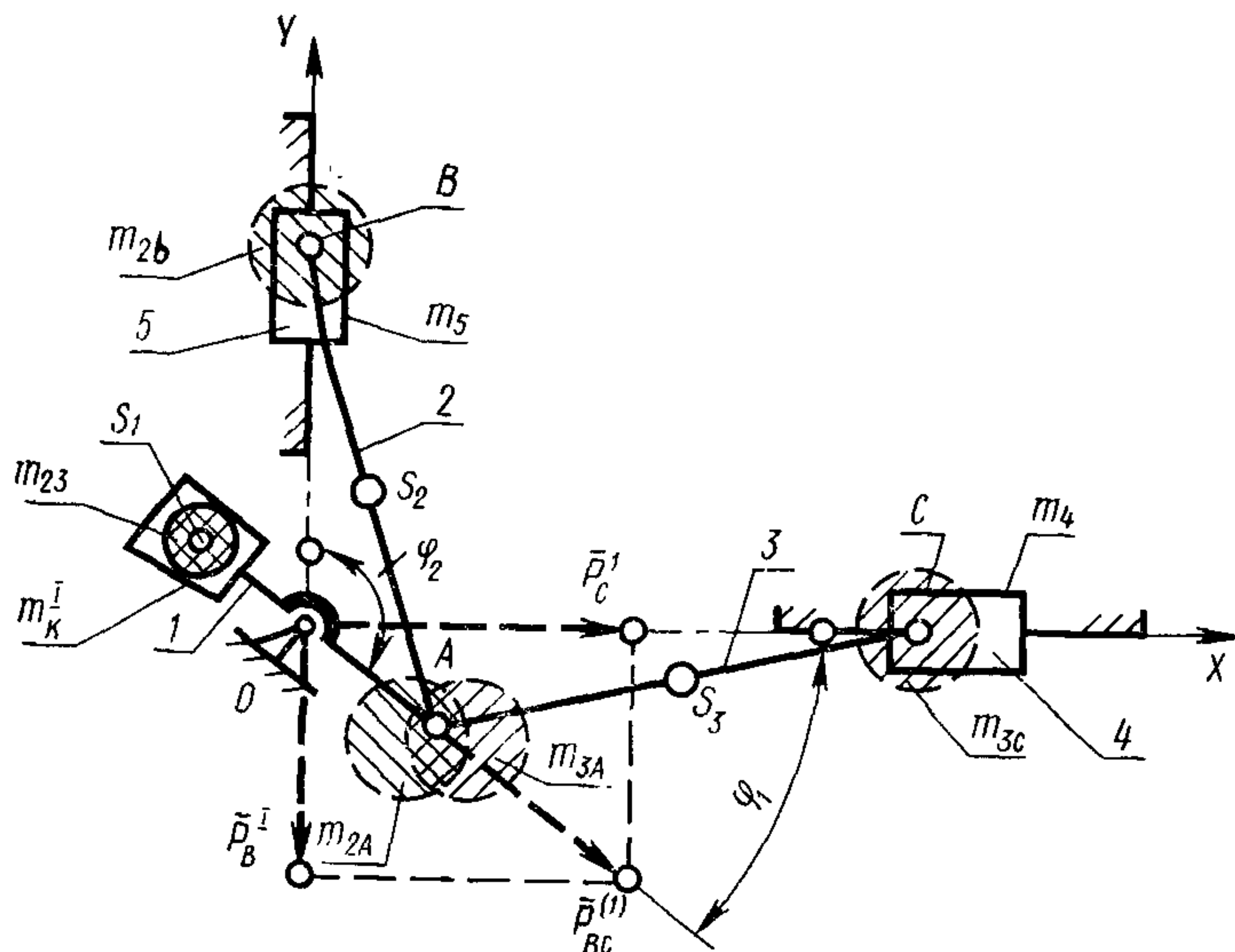
Черт. 19
