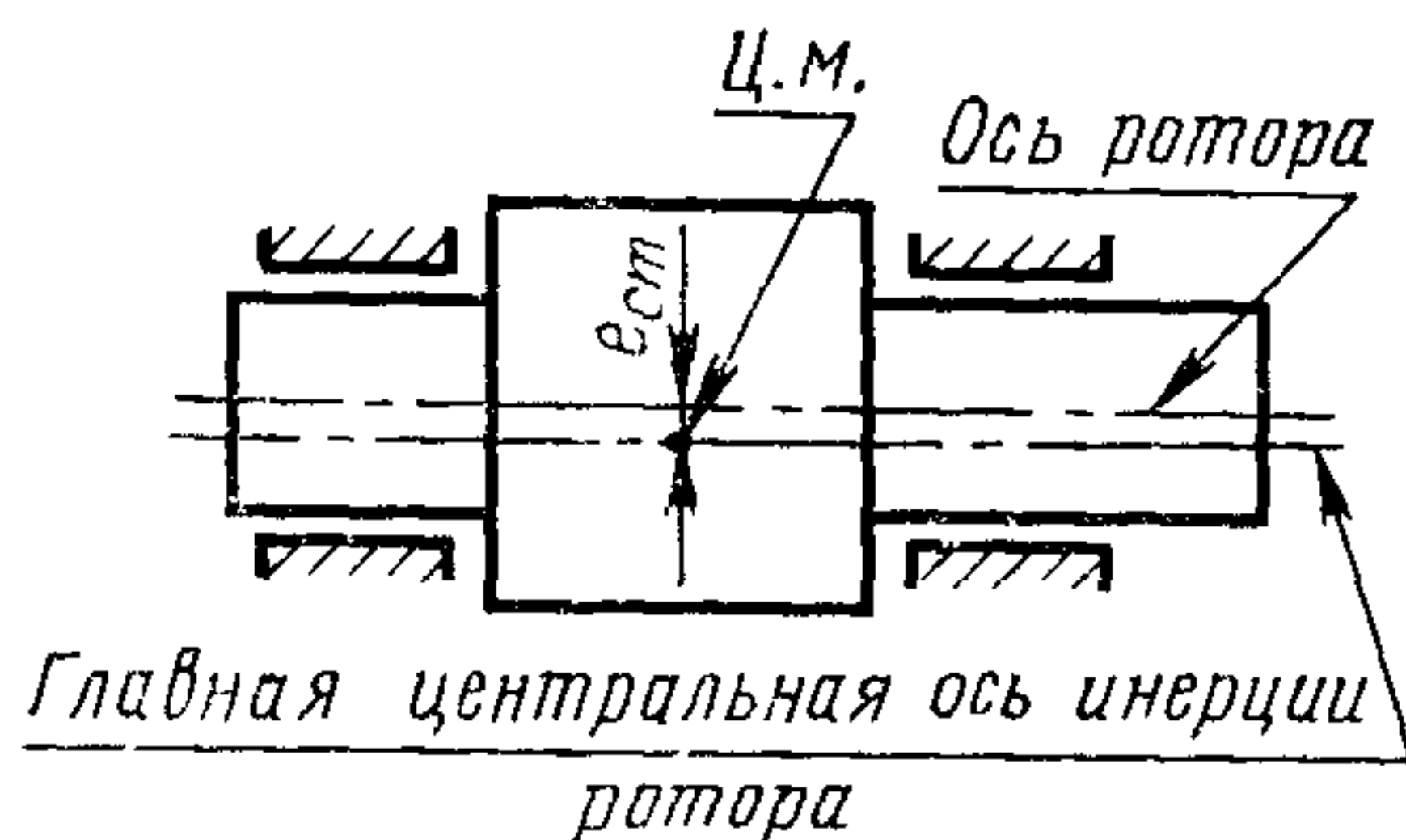
Черт. 2
