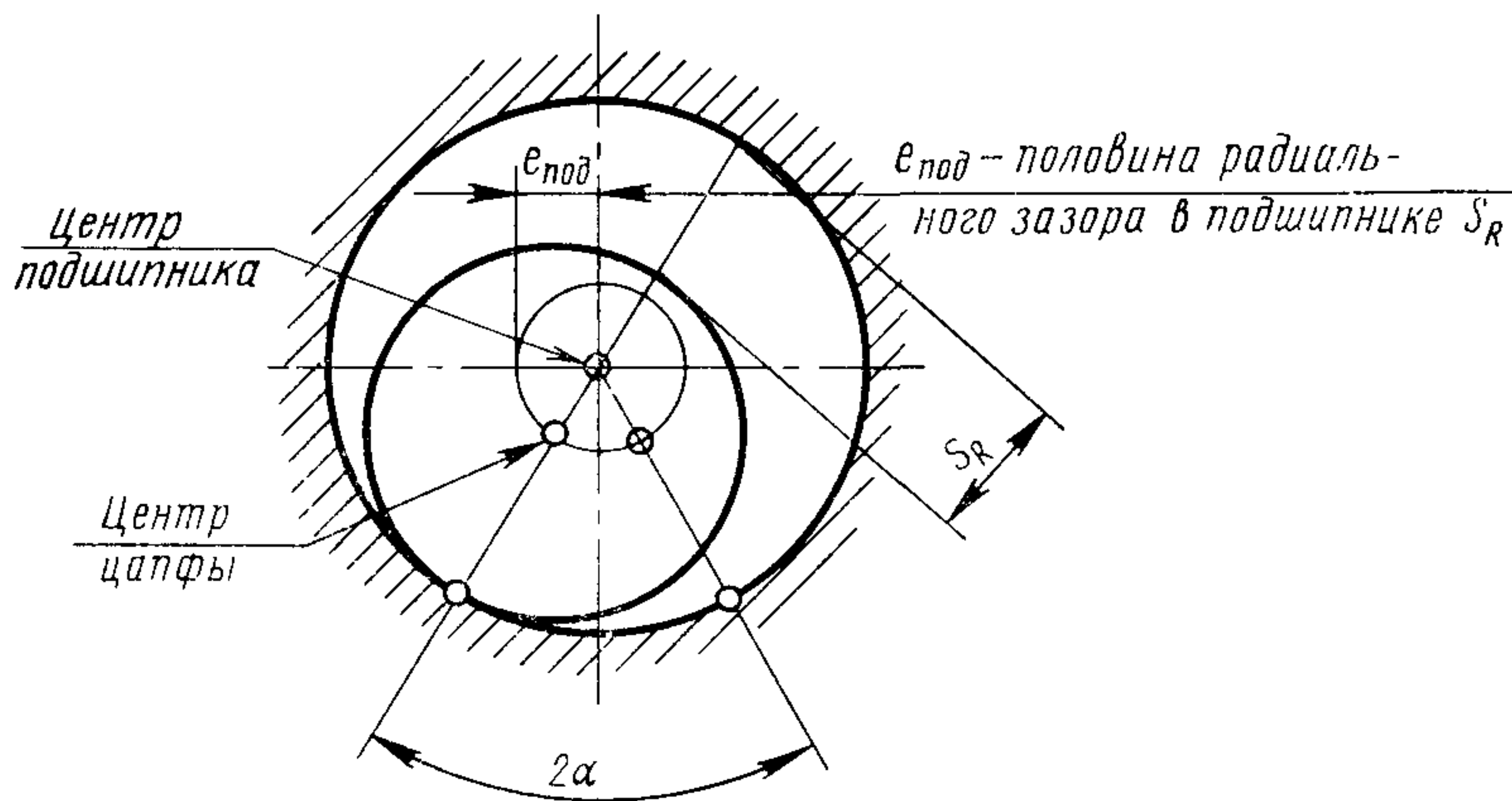
Черт. 12
