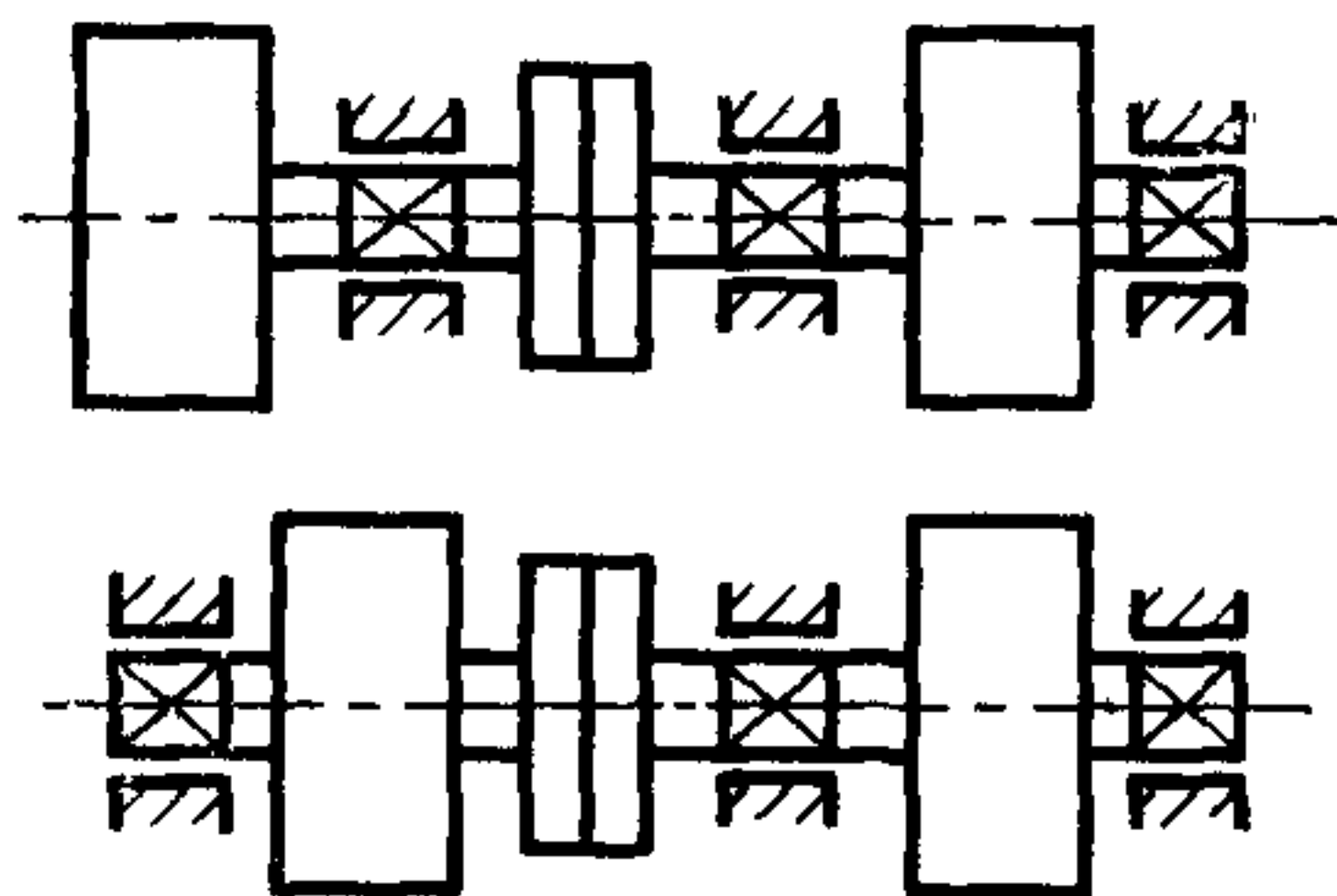
Черт. 43
