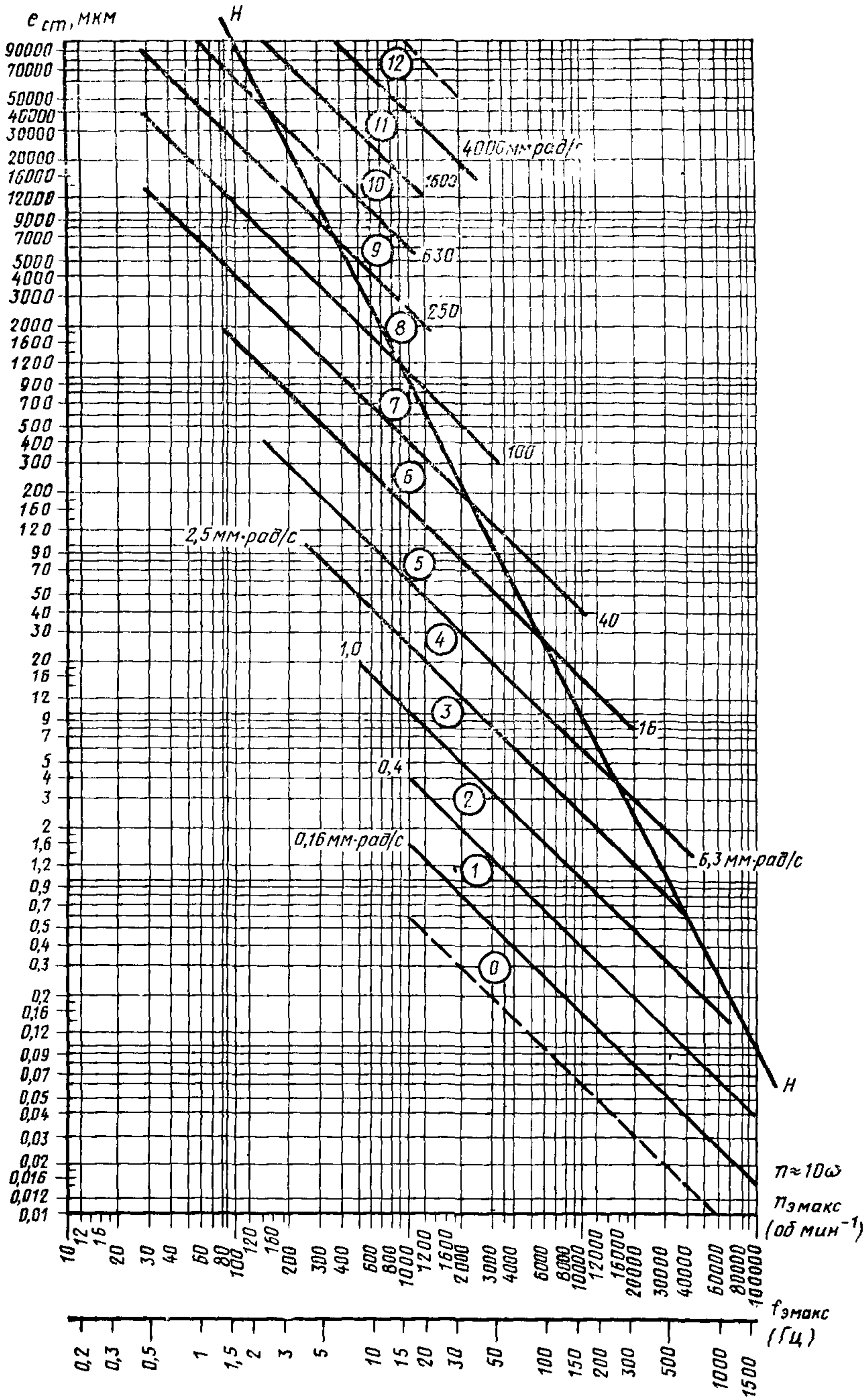
Черт. 1
