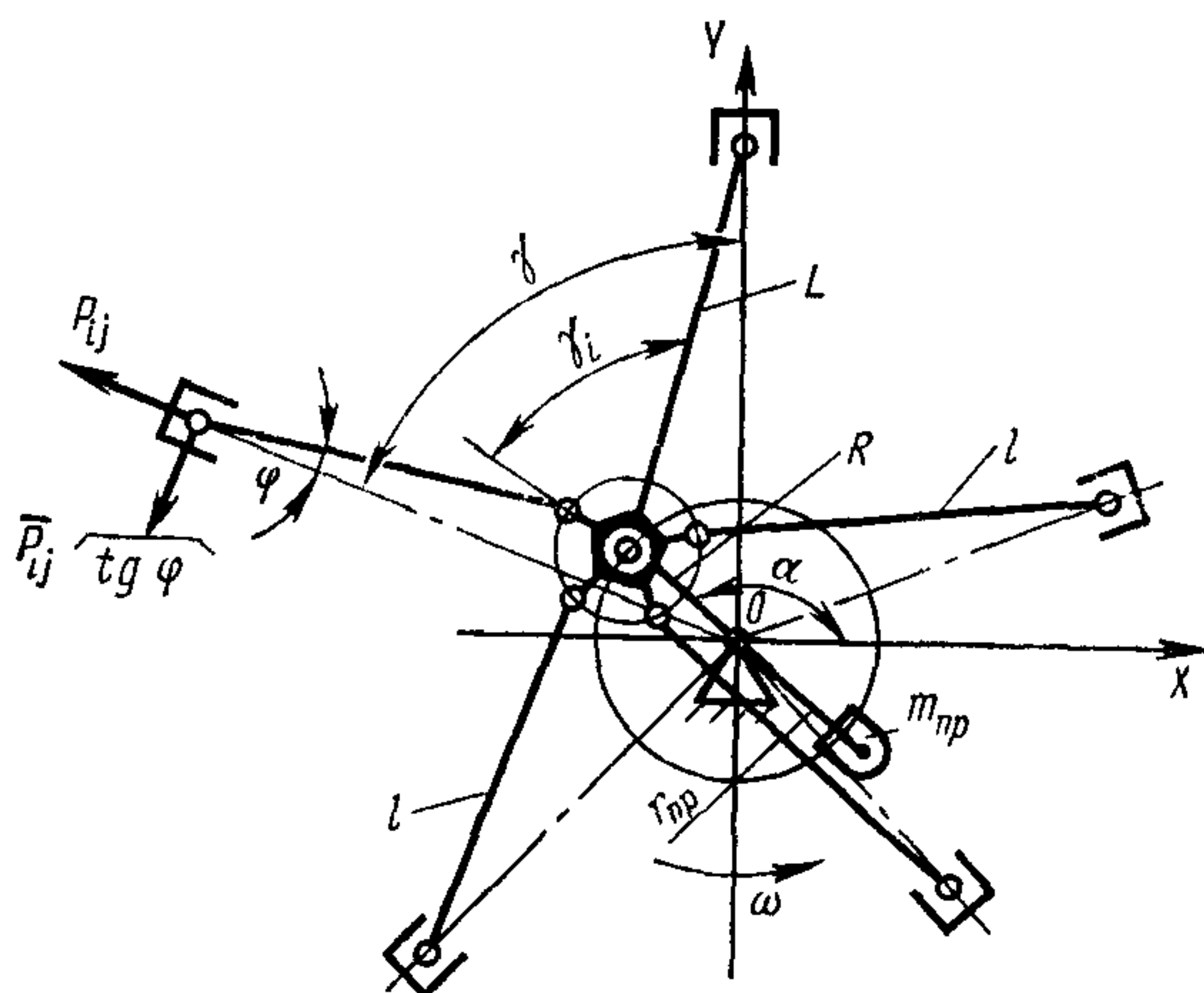
Черт. 21
