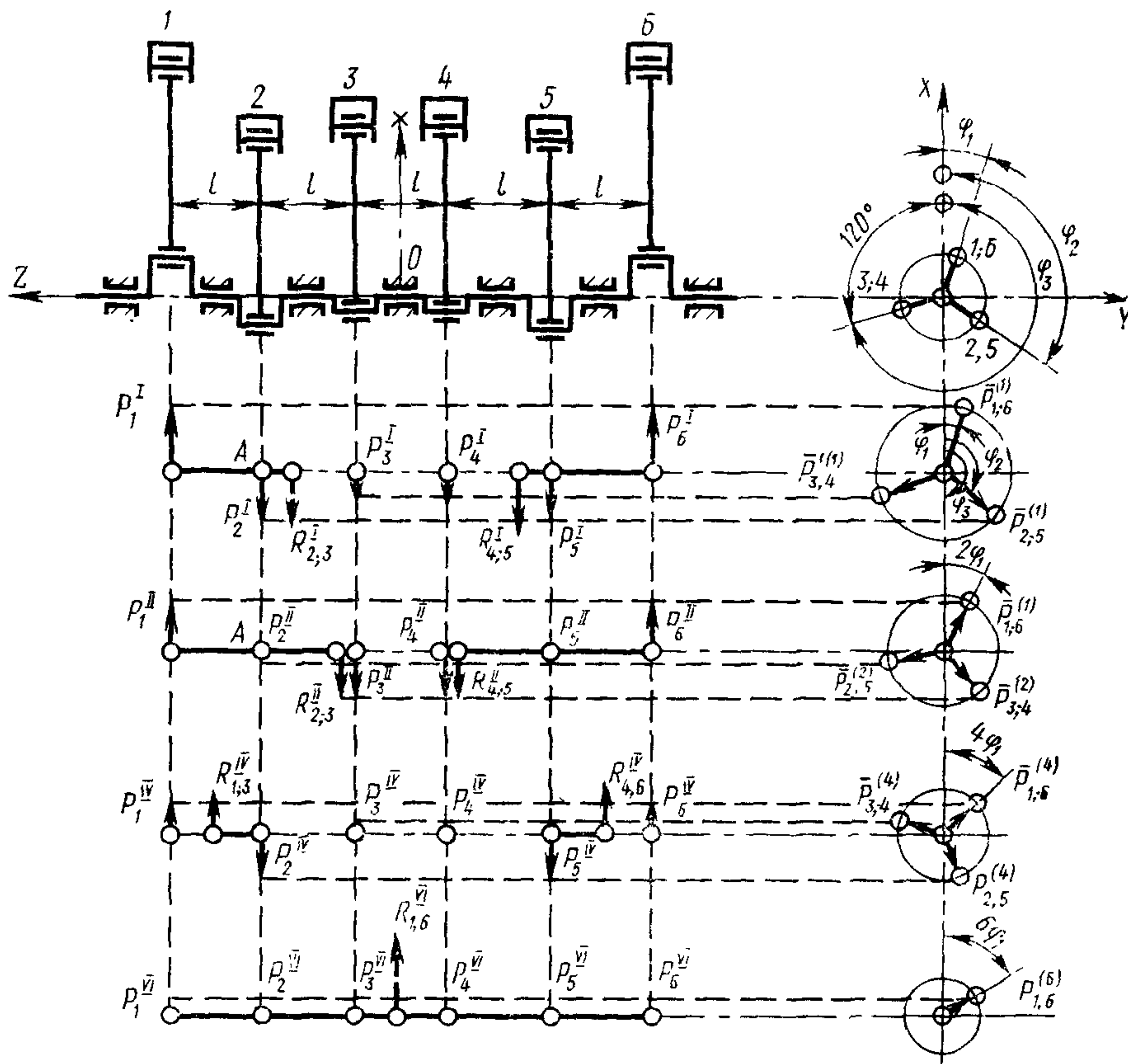
Черт. 20
