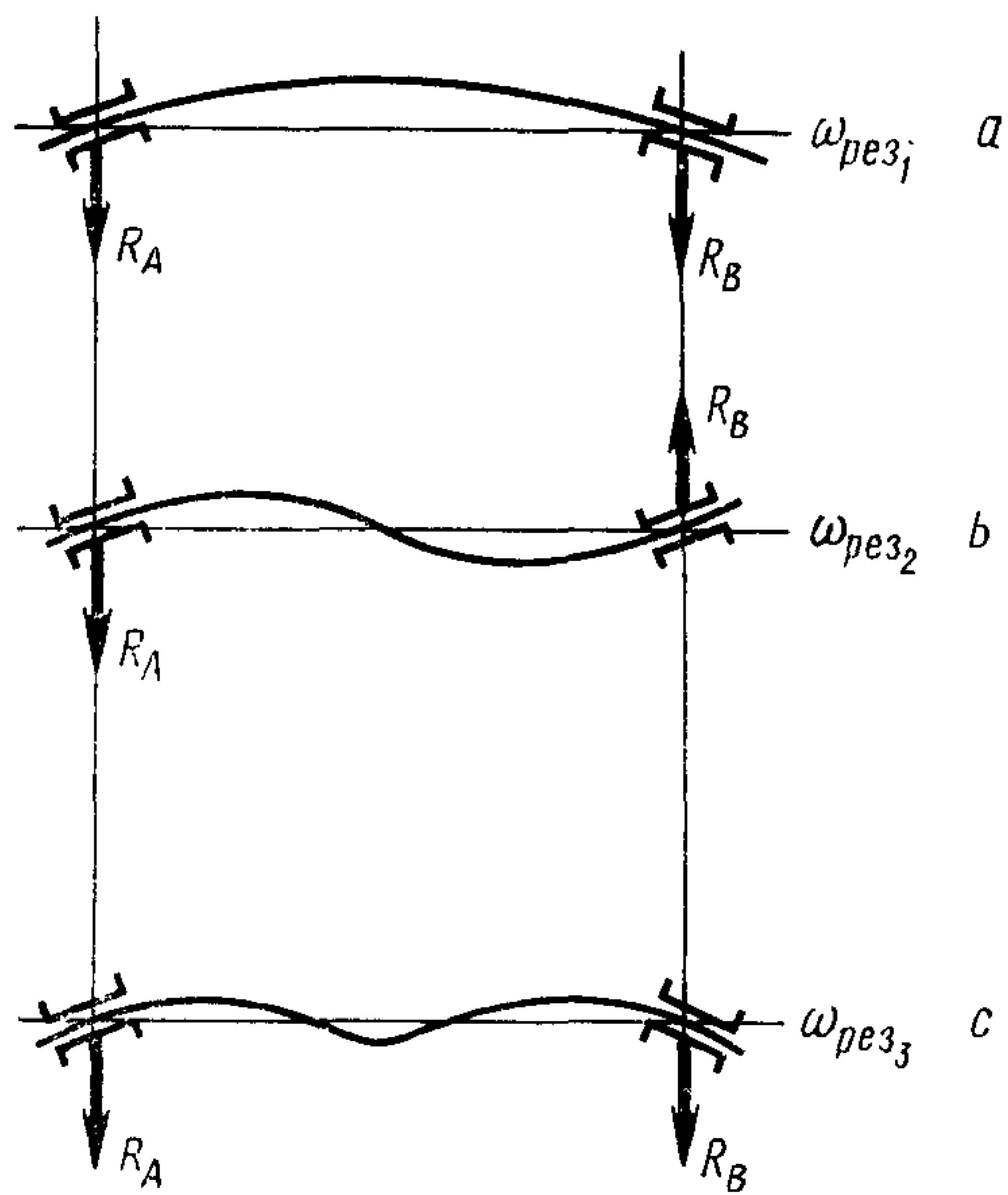
Черт. 29
