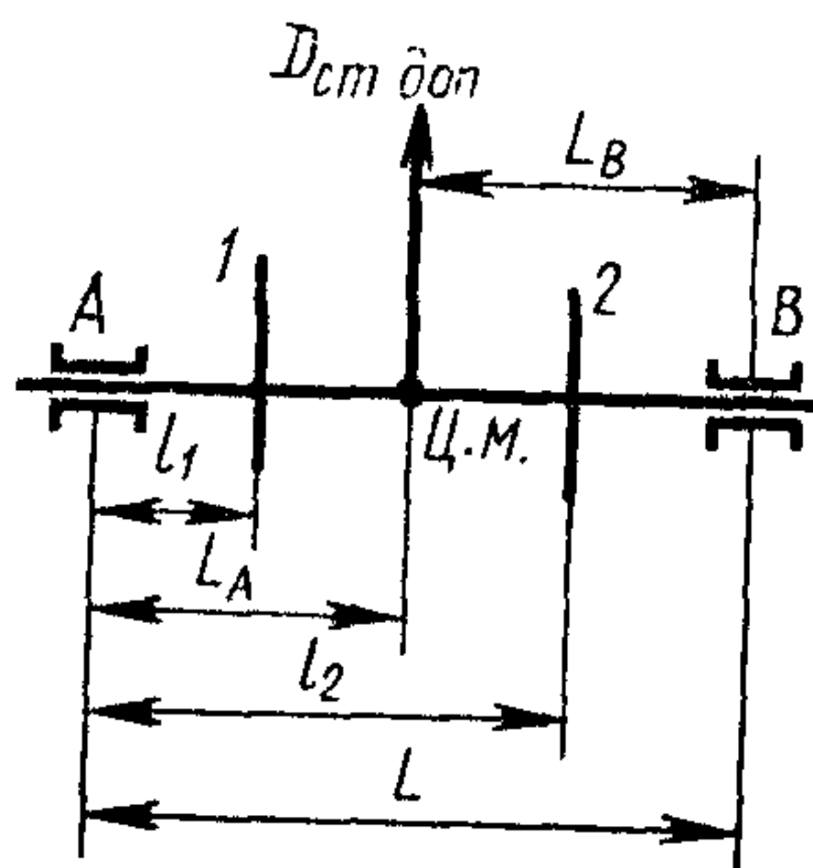
Черт. 2
