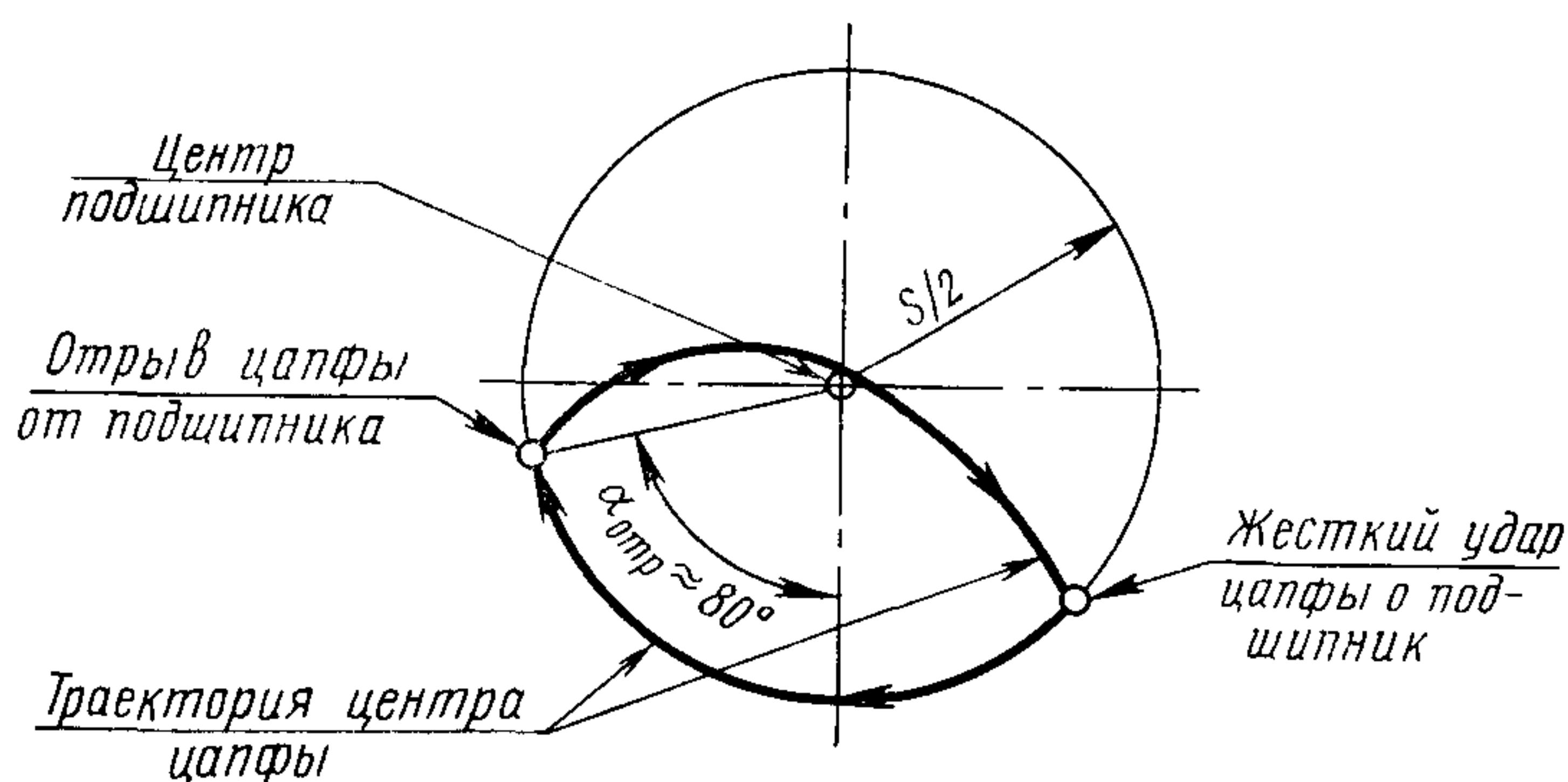
Черт. 13
