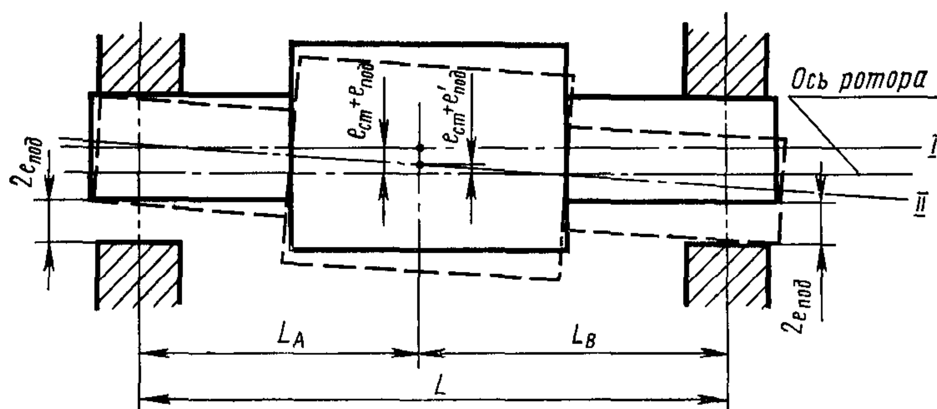
Черт. 51
