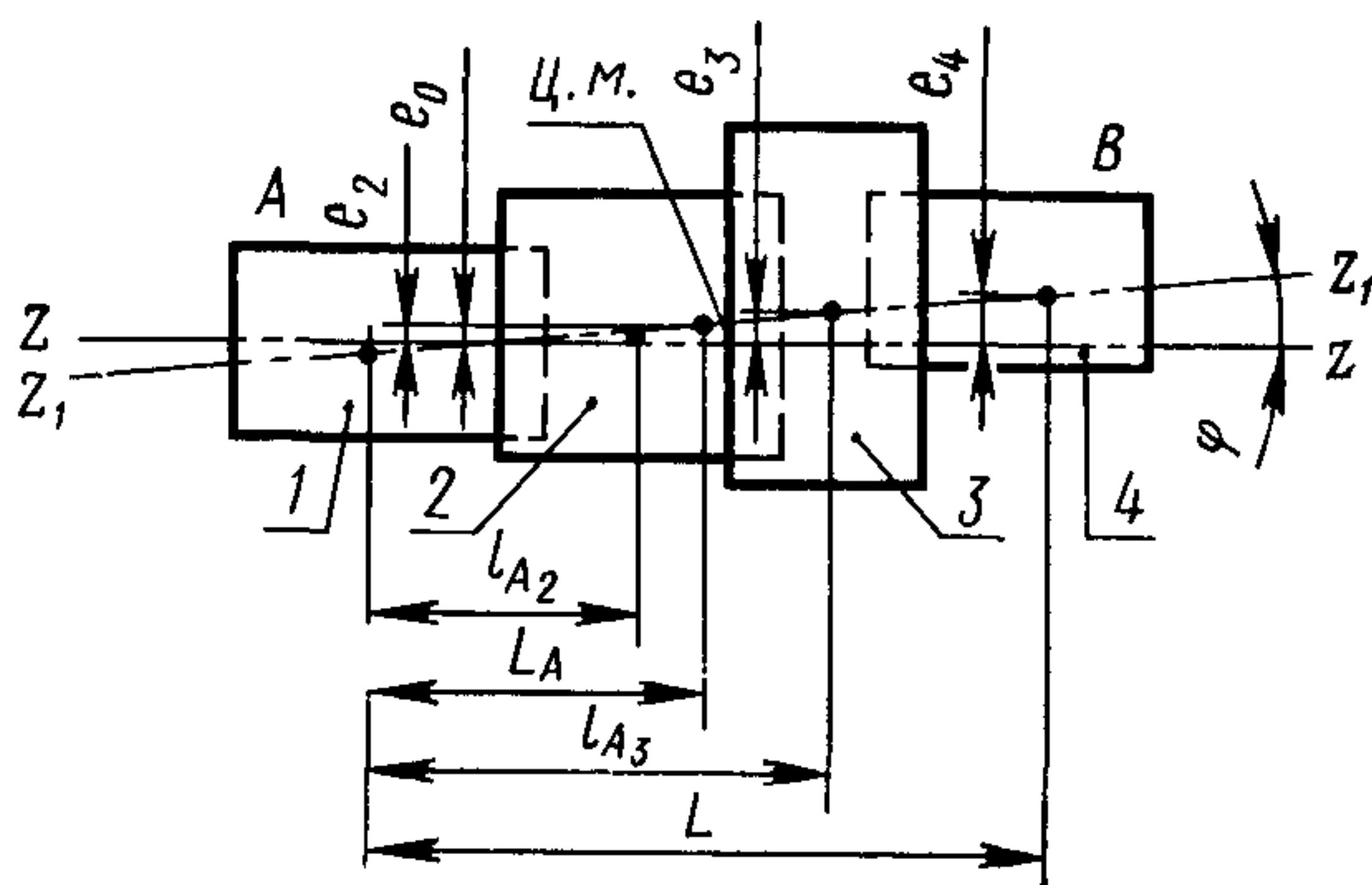
Черт. 45
