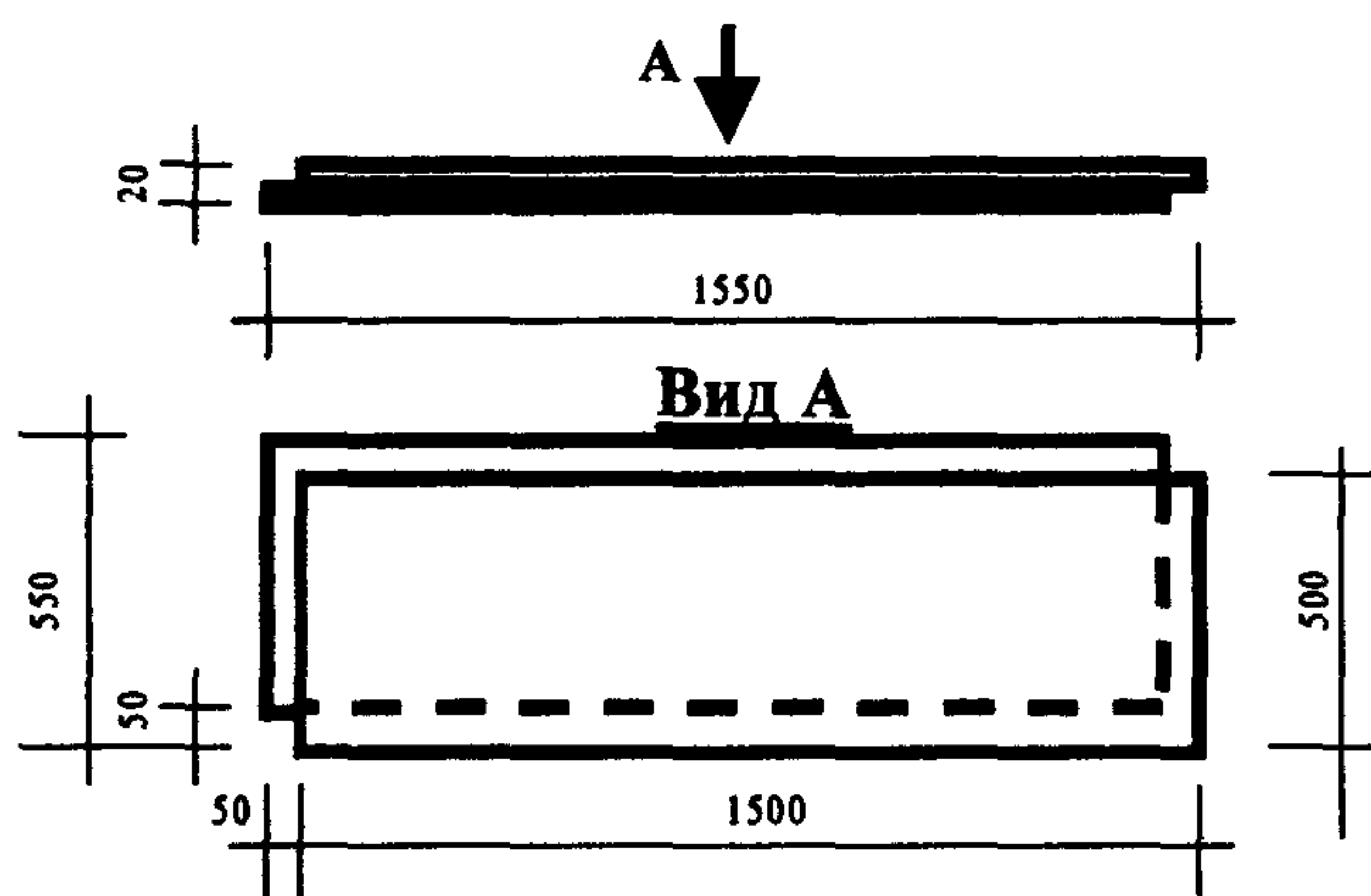
Рисунок 14 — Элемент сборного основания пола
