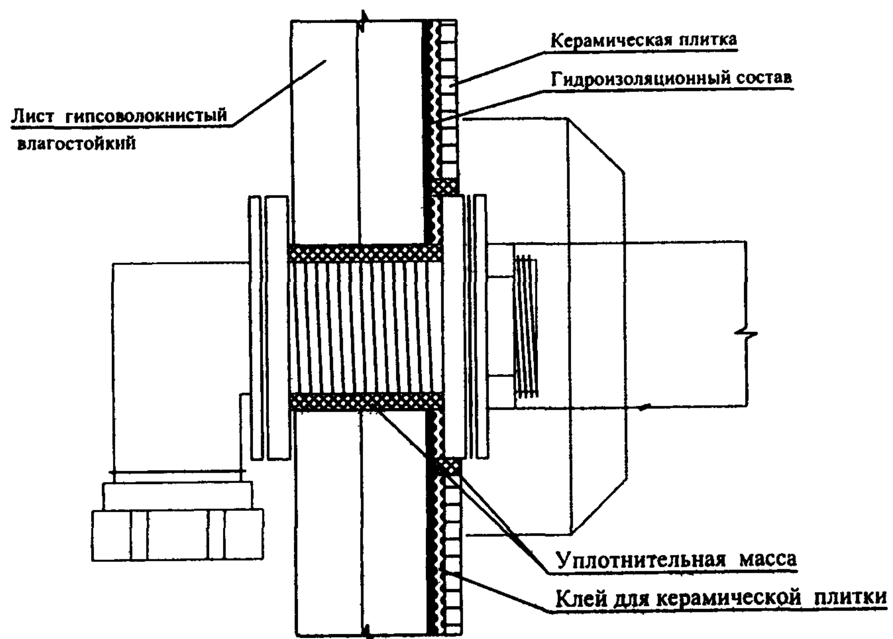
Рисунок 6 — Схема закрепления трубопровода к обшивке перегородки из гипсоволокнистых листов
