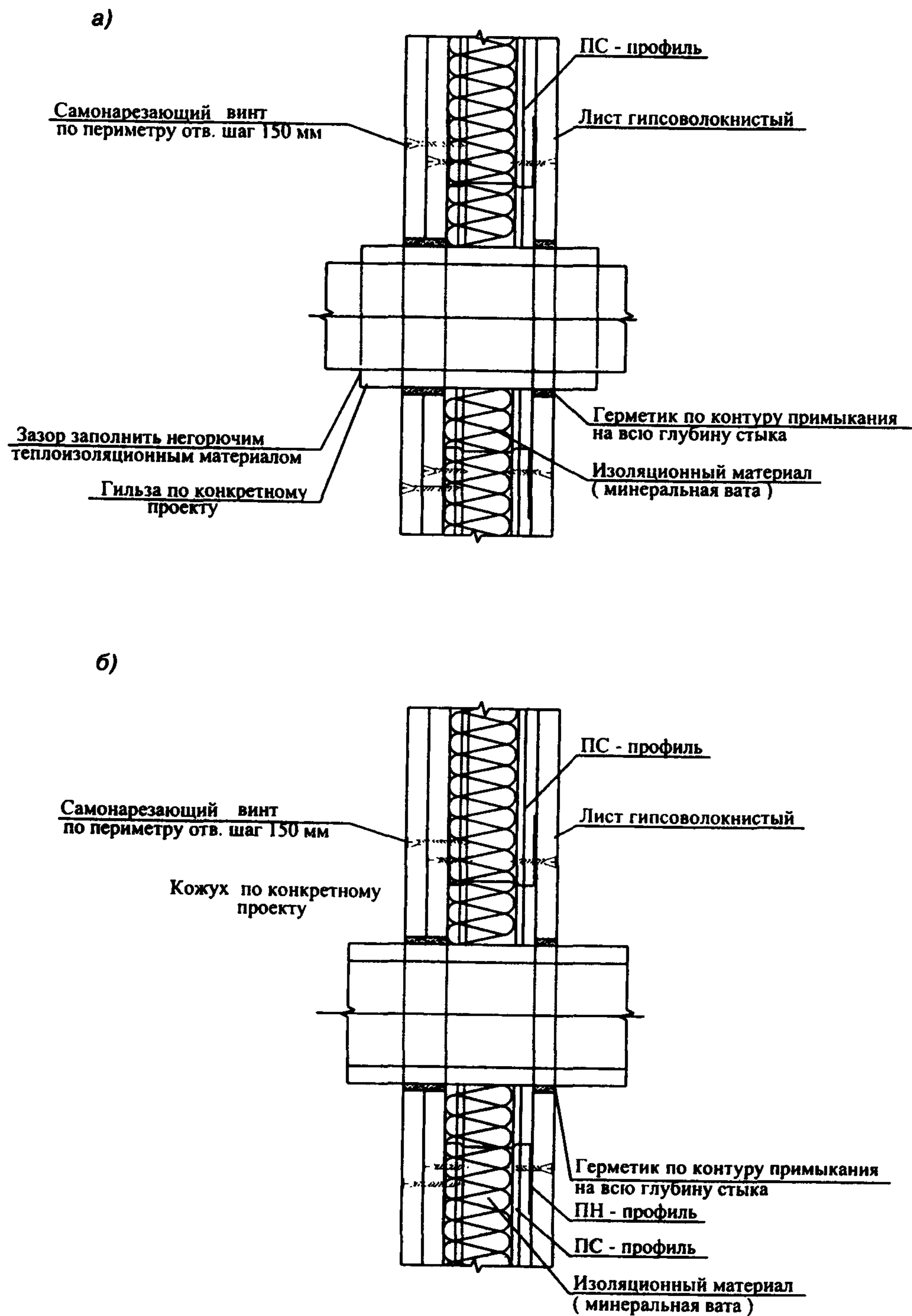
Рисунок 7 — Схема устройства гильзы (а) и кожуха (б) при сопряжении перегородки из гипсоволокнистых листов с трубопроводами
