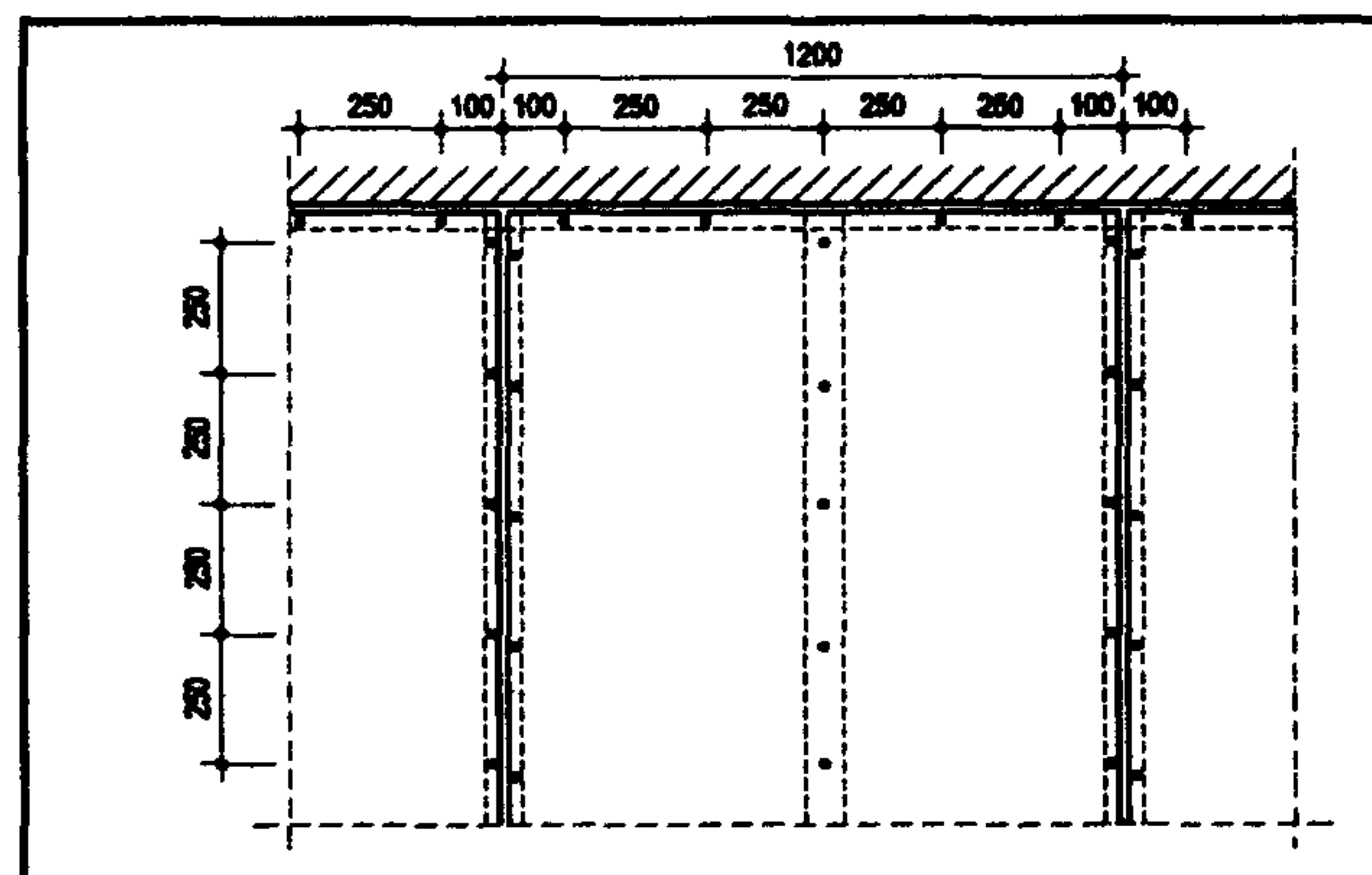
Рисунок 18 — Крепление гипсоволокнистых листов к каркасу
