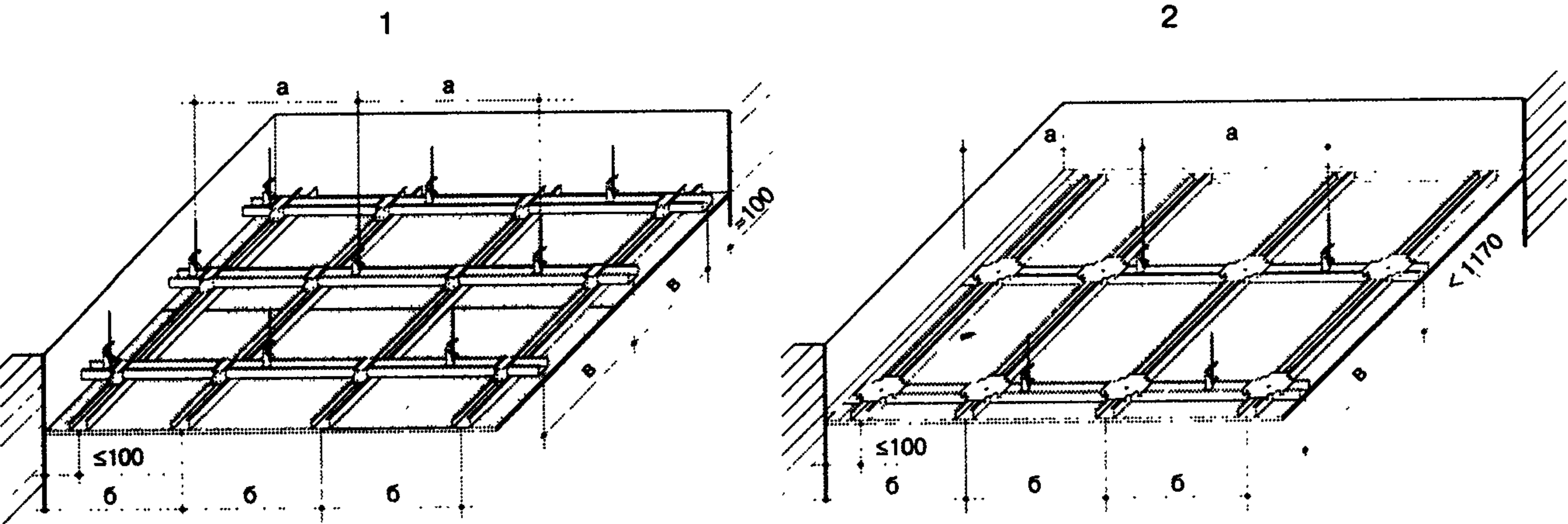
1 — конструкция двухуровневого потолка; 2 — конструкция одноуровневого потолка; а — расстояние между подвесами, б — расстояние между несущими профилями, в — расстояние между основными профилями
