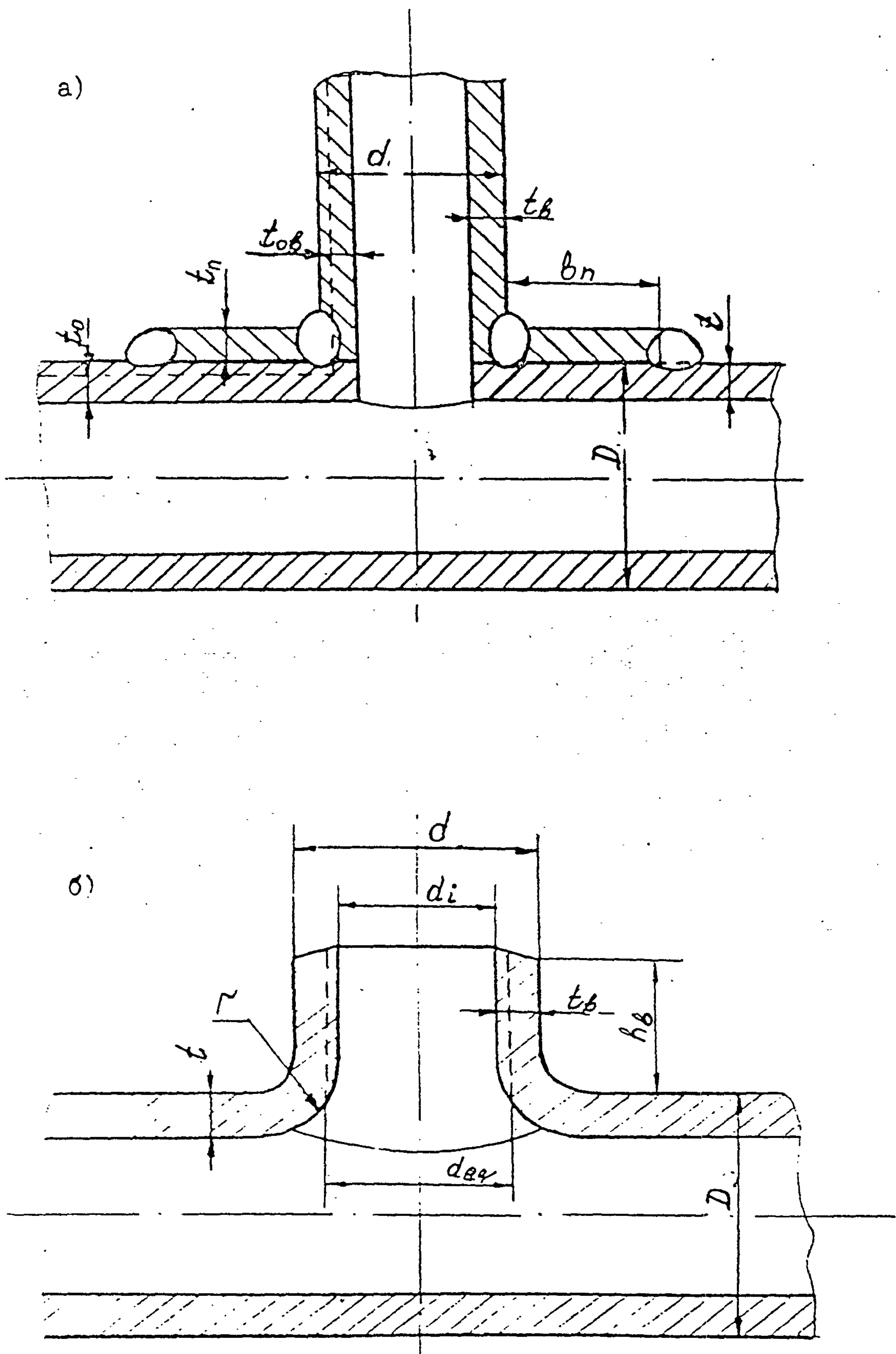
Черт. 5.3 Тройник
