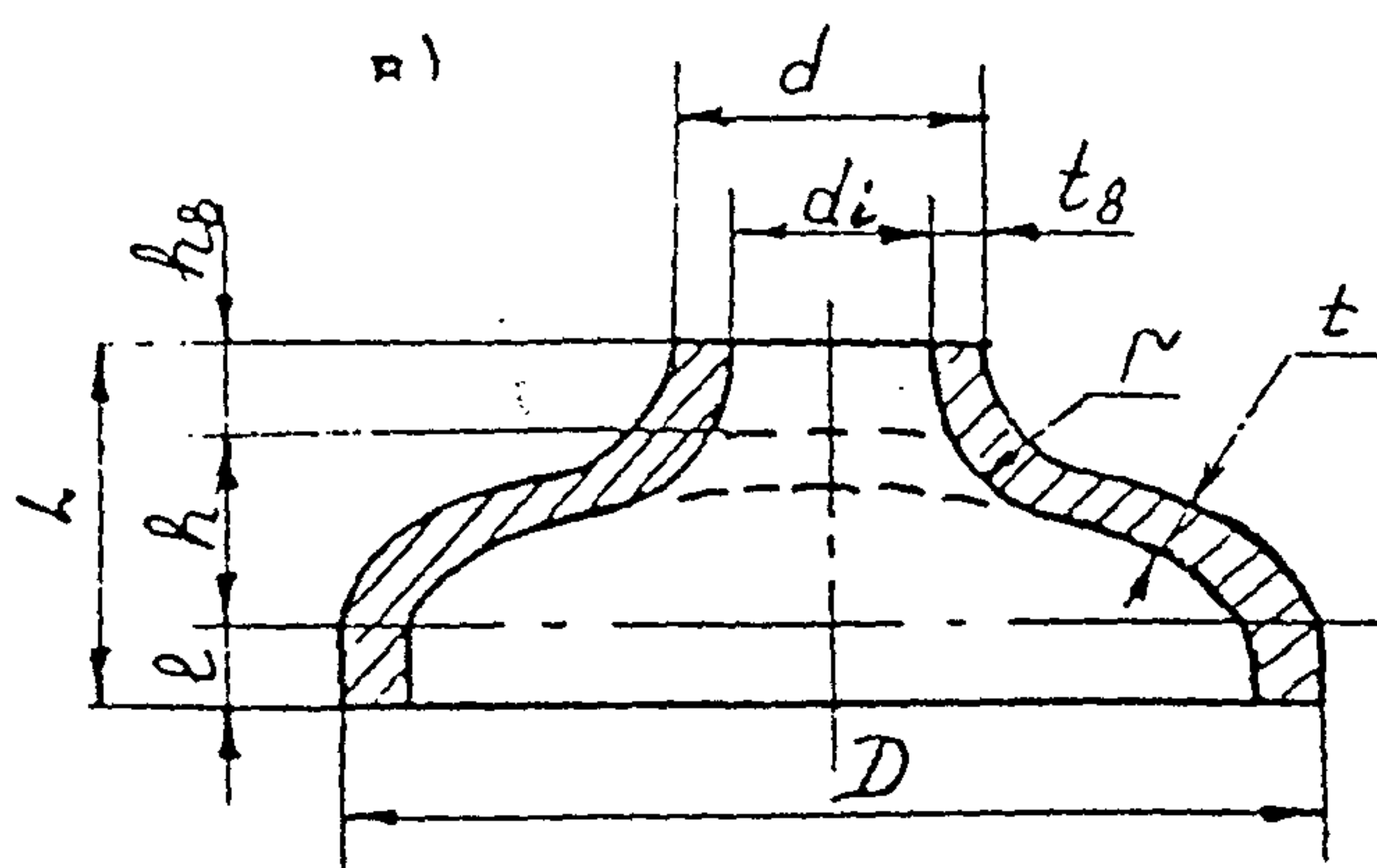
Черт. 27. Эллиптические заглушки со штуцером
