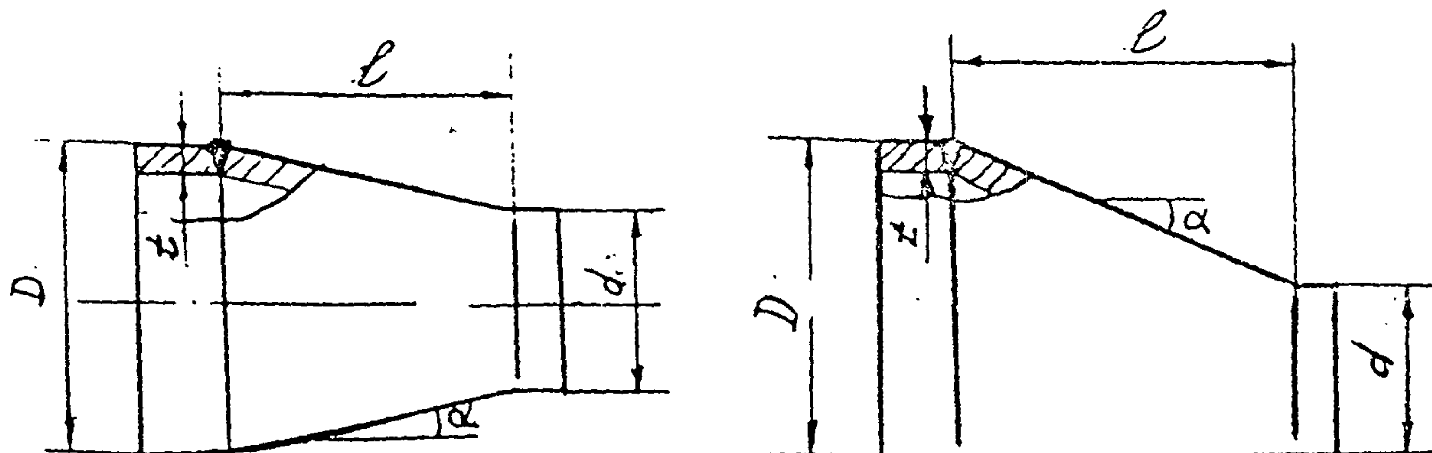
Черт. 5.2 Переходы
