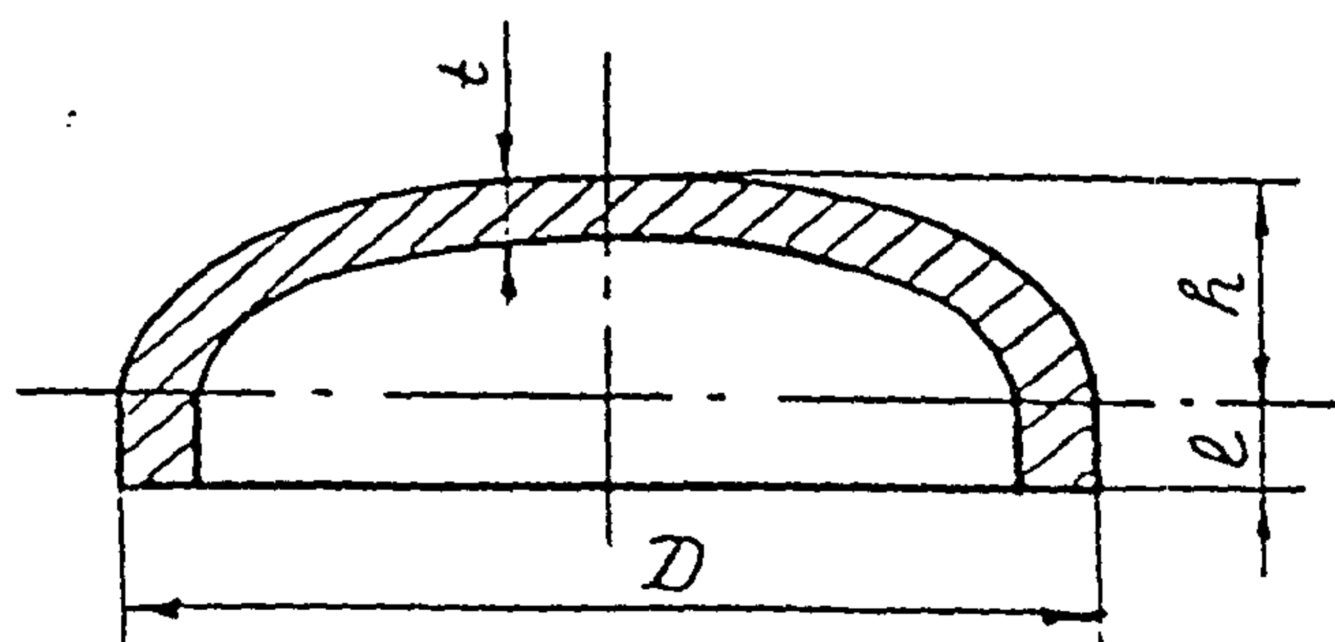
Черт. 26. Эллиптическая заглушка
