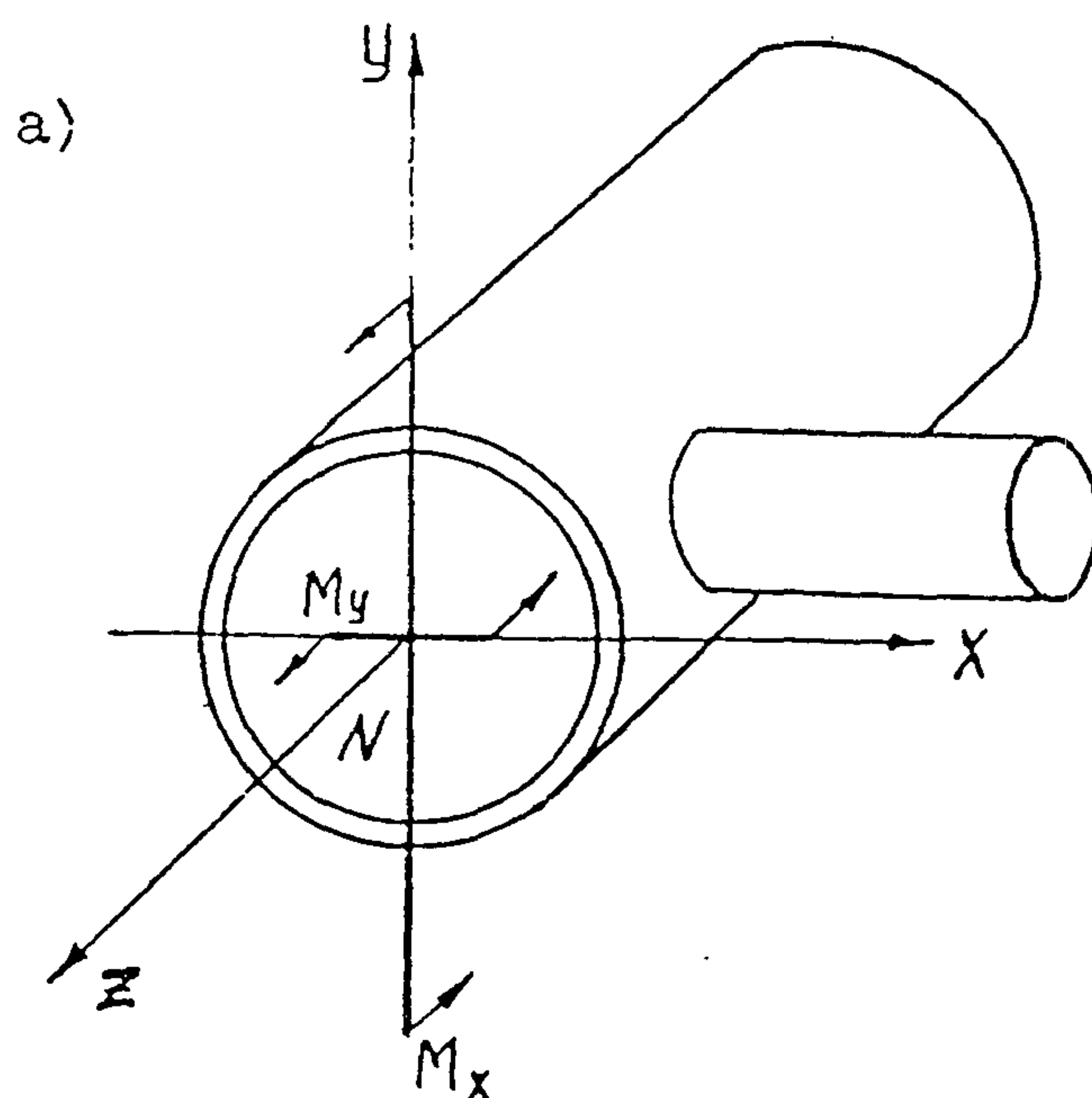
Черт. 7.2 Расчетная схема тройникового соединения
