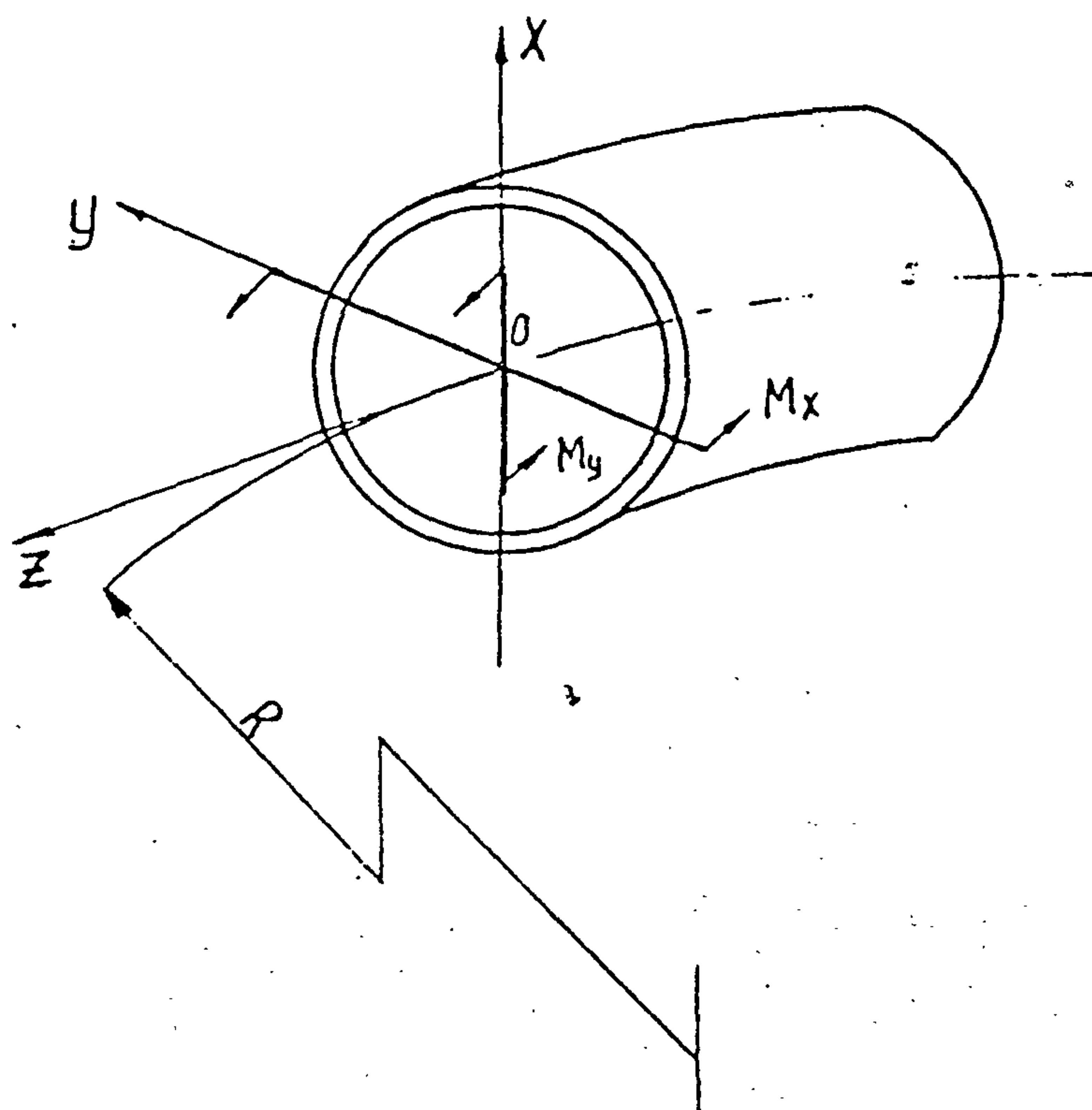
Черт. 7.1 Расчетная схема отвода
