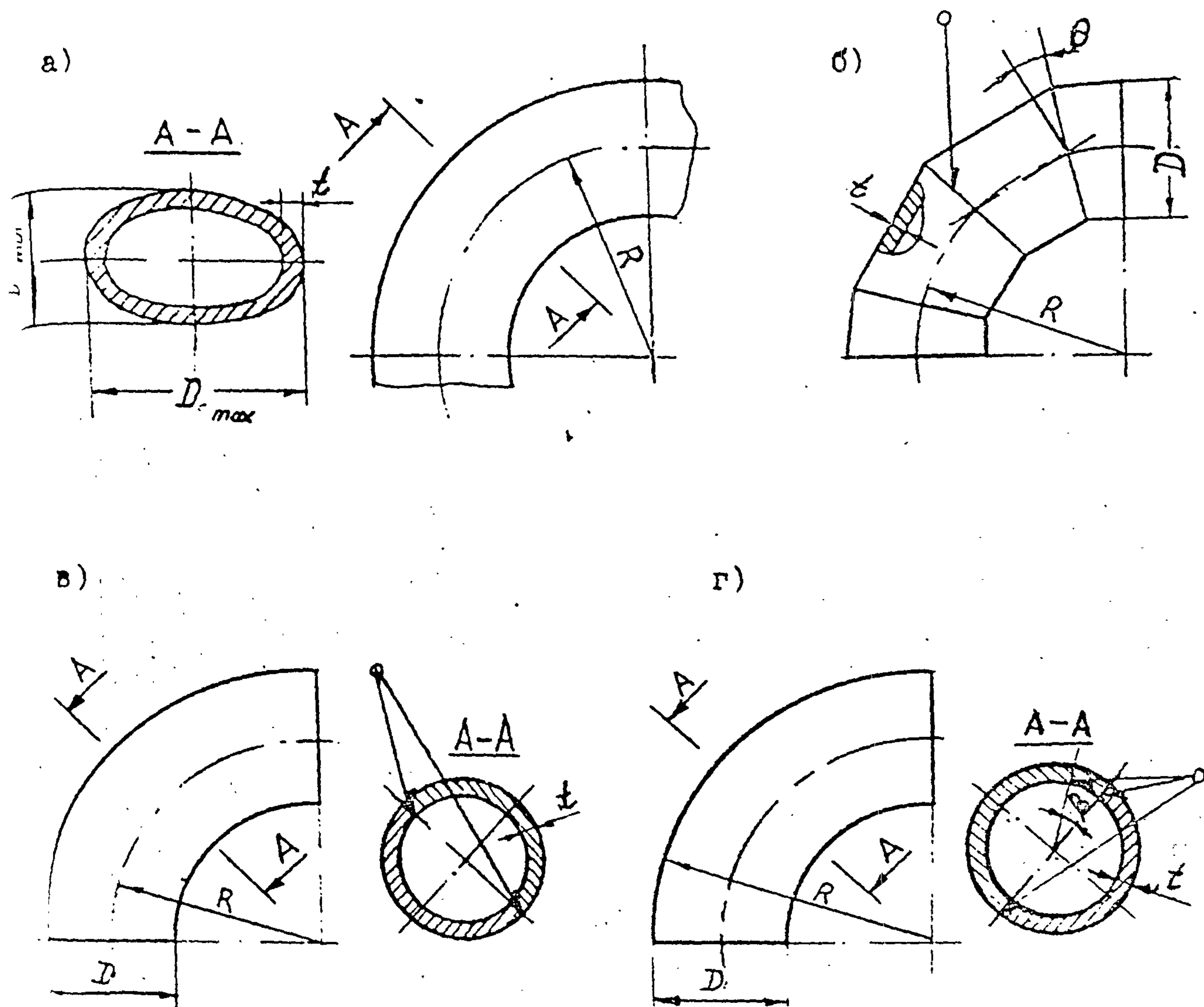
Черт. 5.1 Отводы
