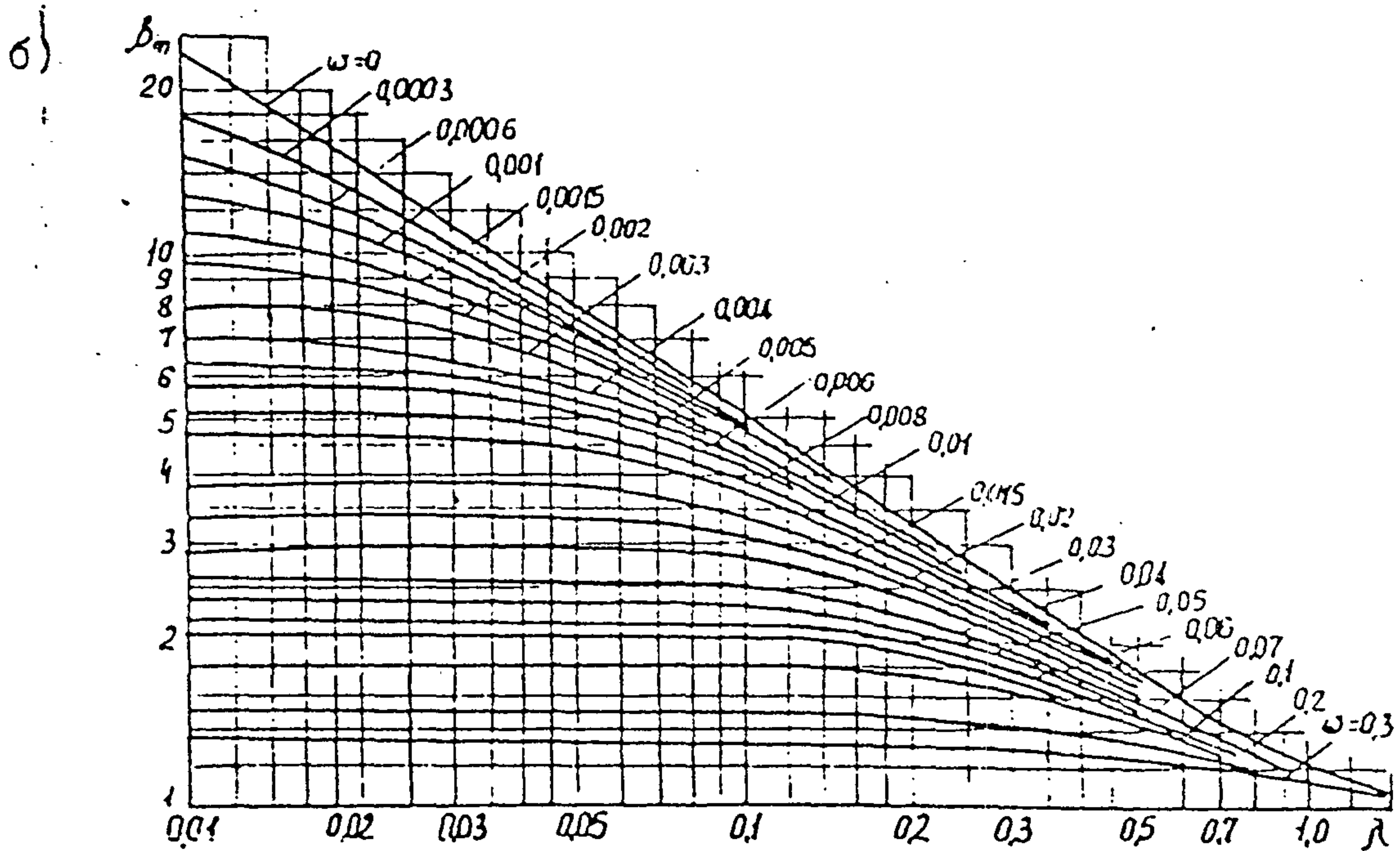
Черт. 7.3К определению коэффициентов \gamma_m (а) и \beta_m (б).
