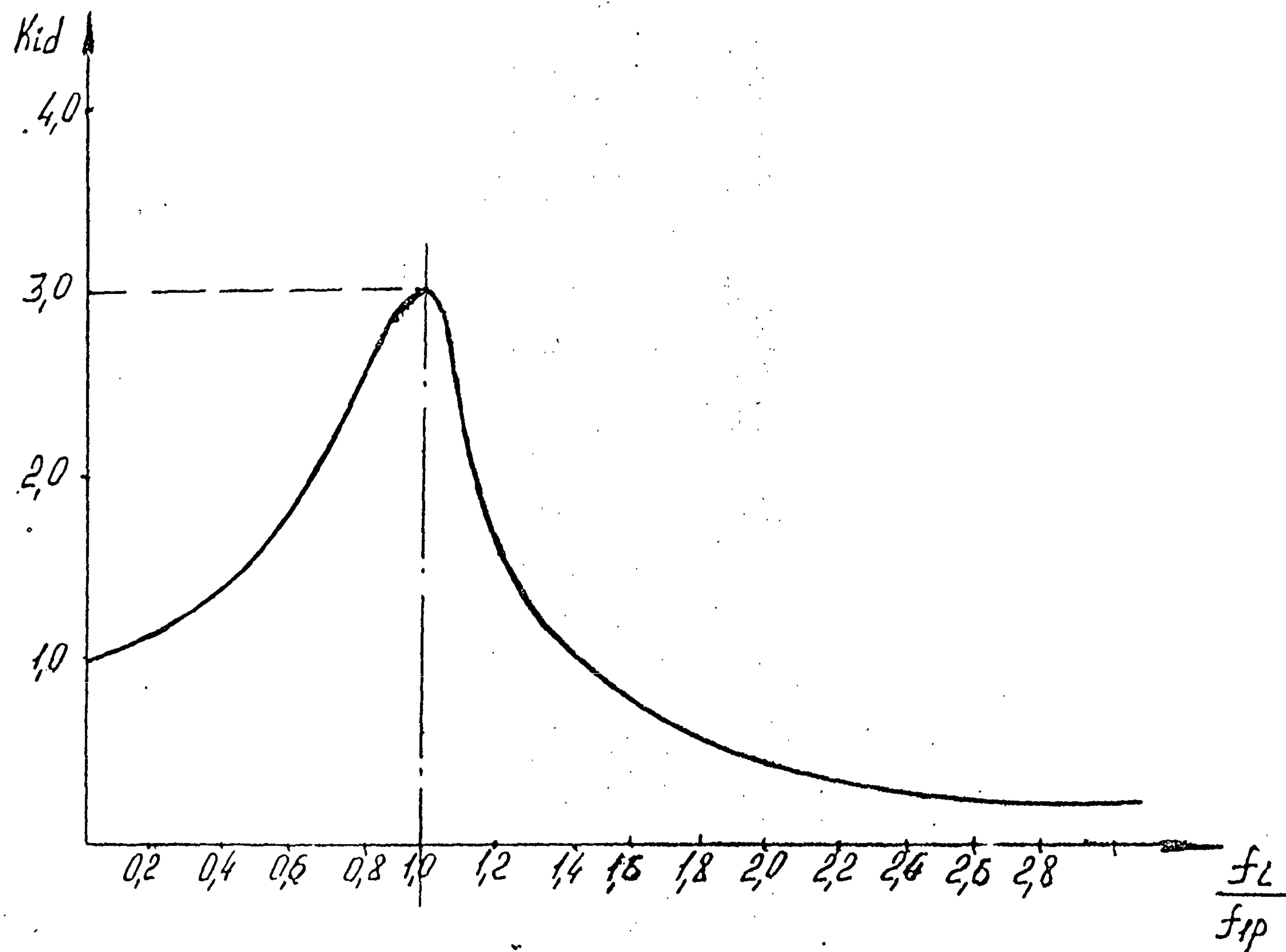
Черт. 8.1. Схема определения коэффициента K_{id} при K_{idmax} = 3.0
