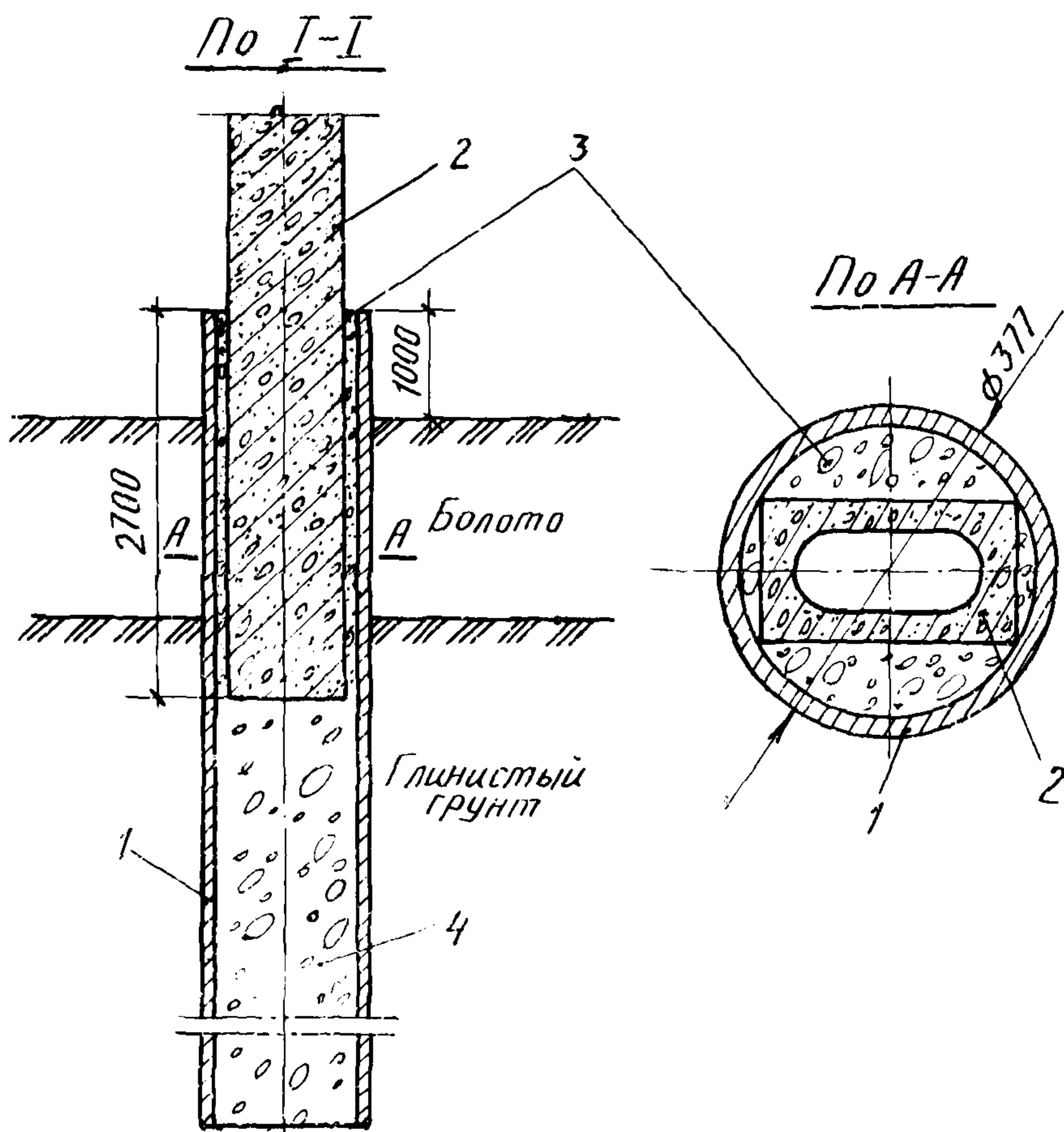
Рис.6. Закрепление промежуточных опор на болотах:
