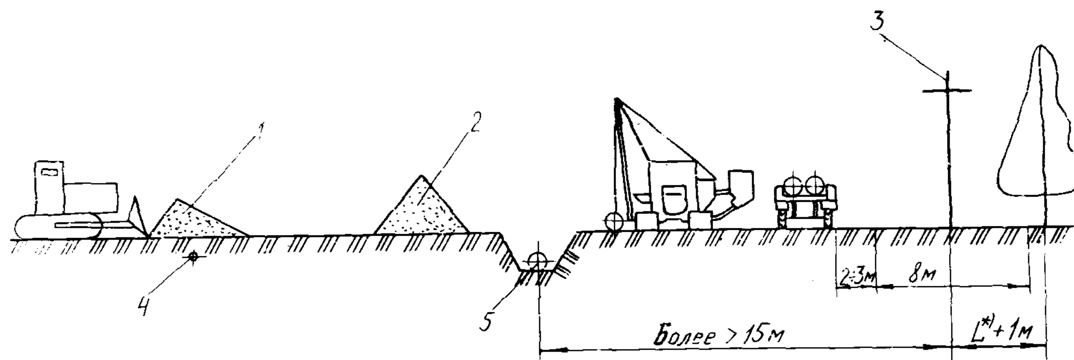
Рис. I. Схема расположения при совмещенном строительстве трубопровода вдольтрассовой ЛЭП 6-10 кВ и кабеля технологической связи:
