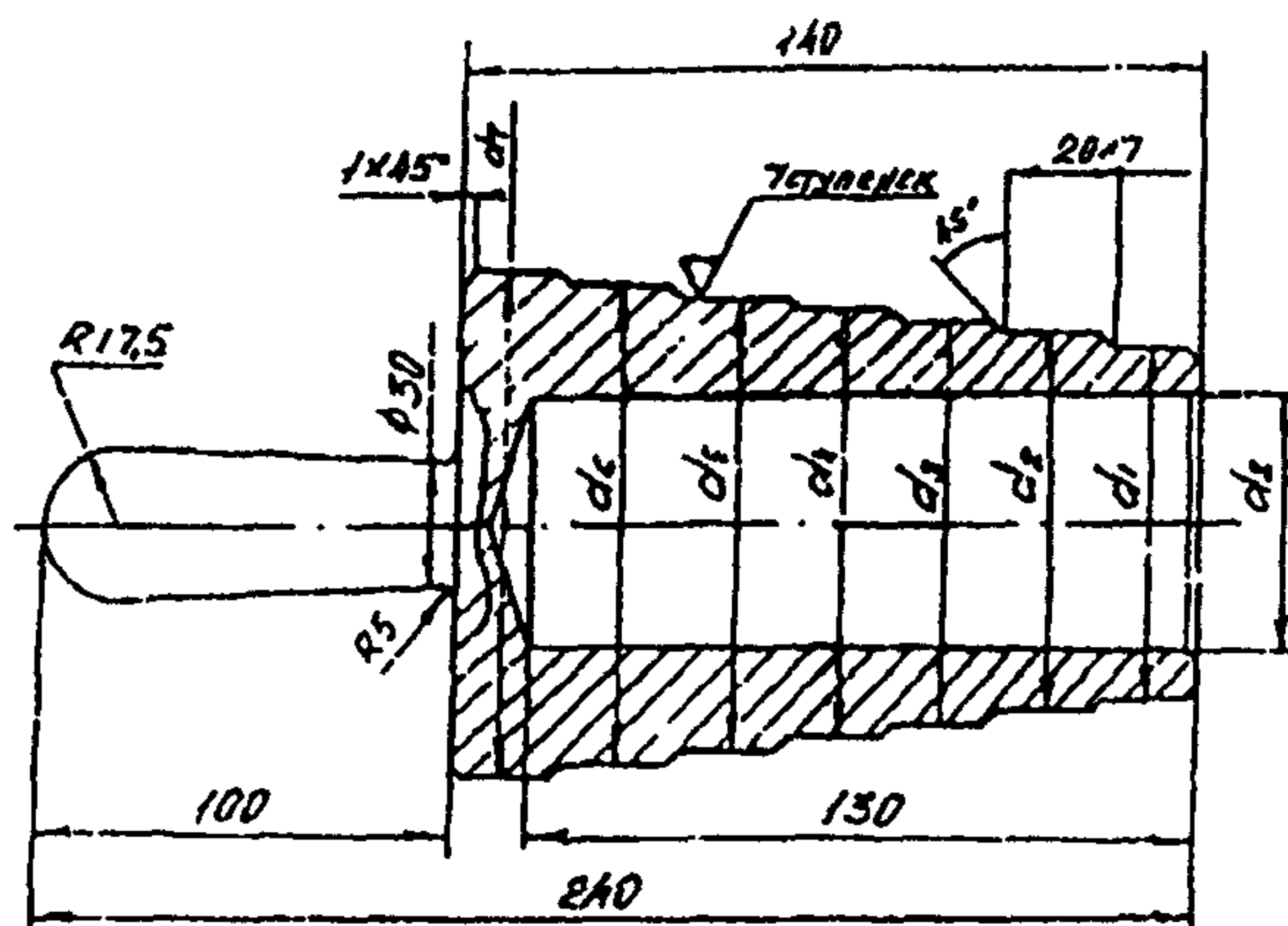
Рисунок 2. Ступенчатый калибр
