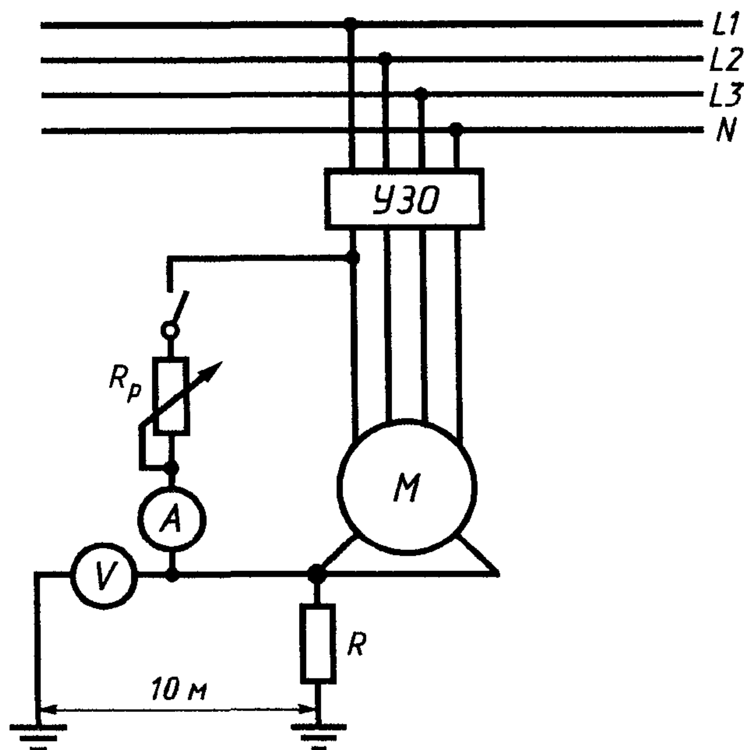
Рисунок В.3 — Схема проверки УЗО по методу 3
