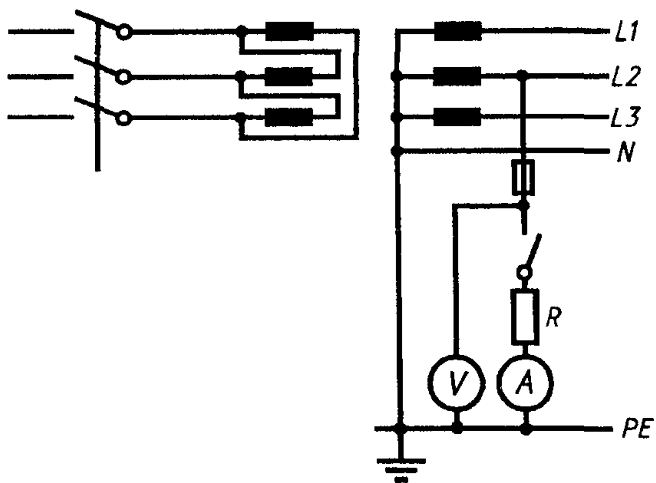
Рисунок D.1 — Схема измерения по методу 1
