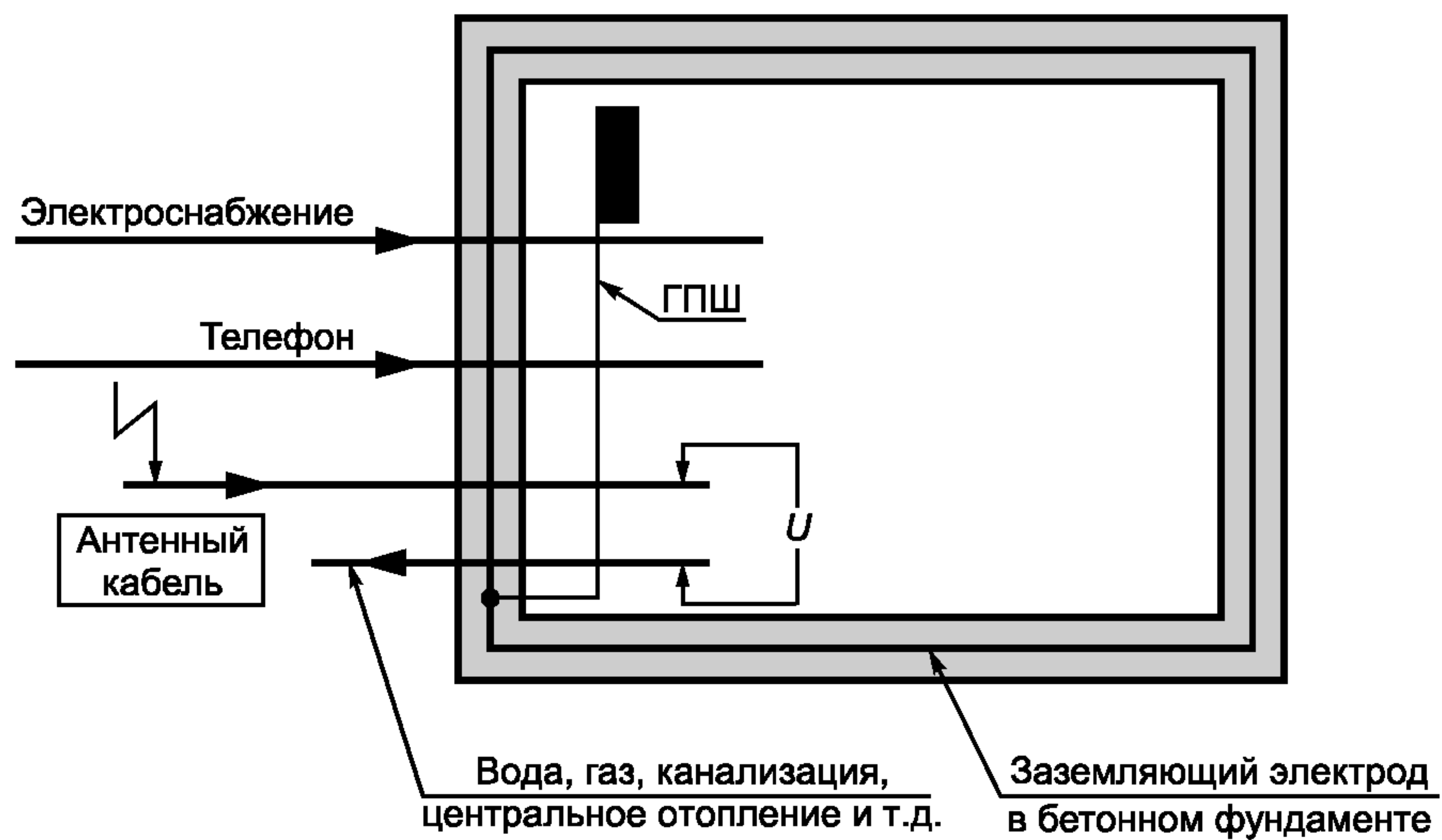
Рисунок 3а — Односторонний ввод (предпочтителен, \tilde{U} = 0 )
