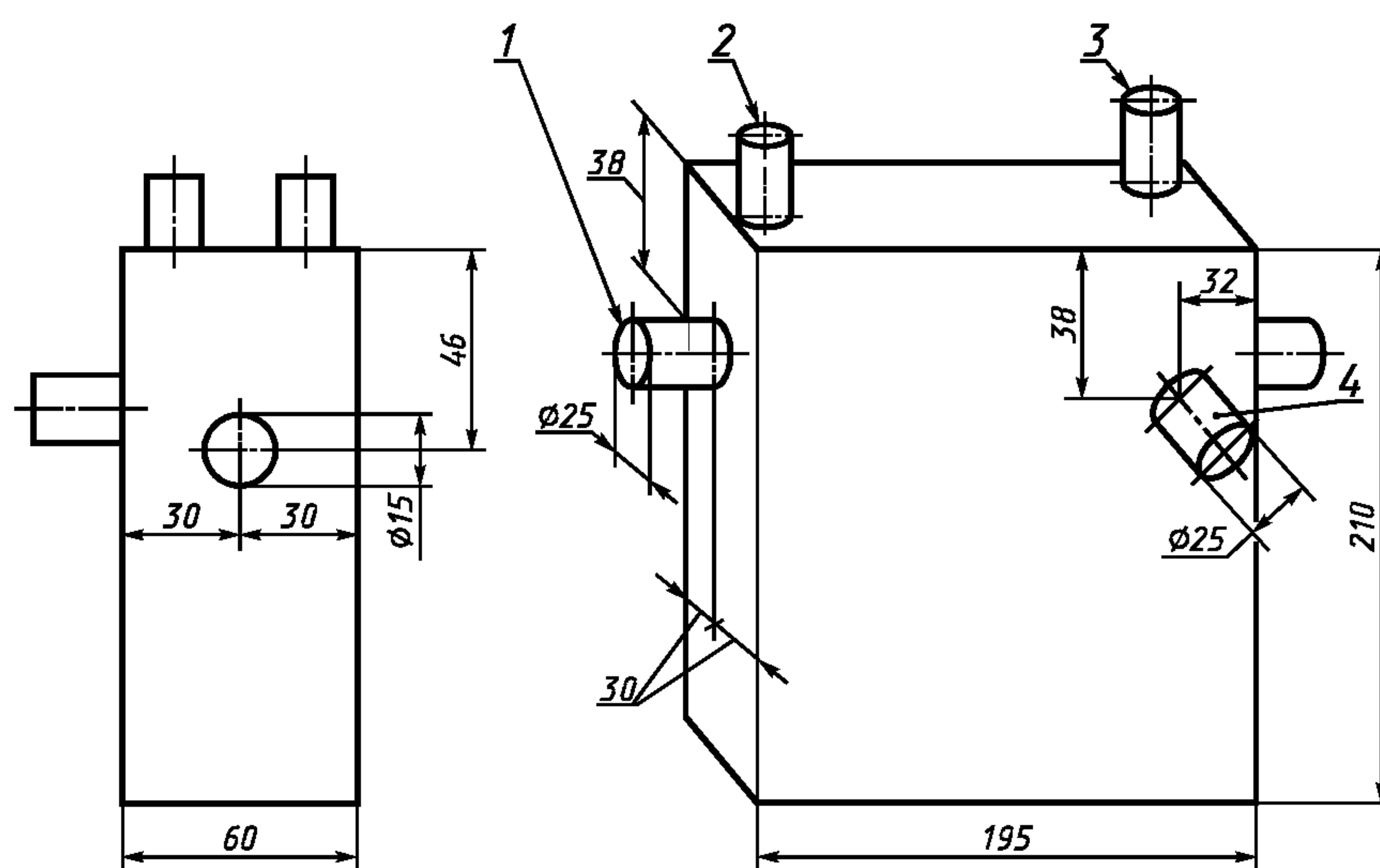
Рисунок А.2 — Схема термостата-увлажнителя
