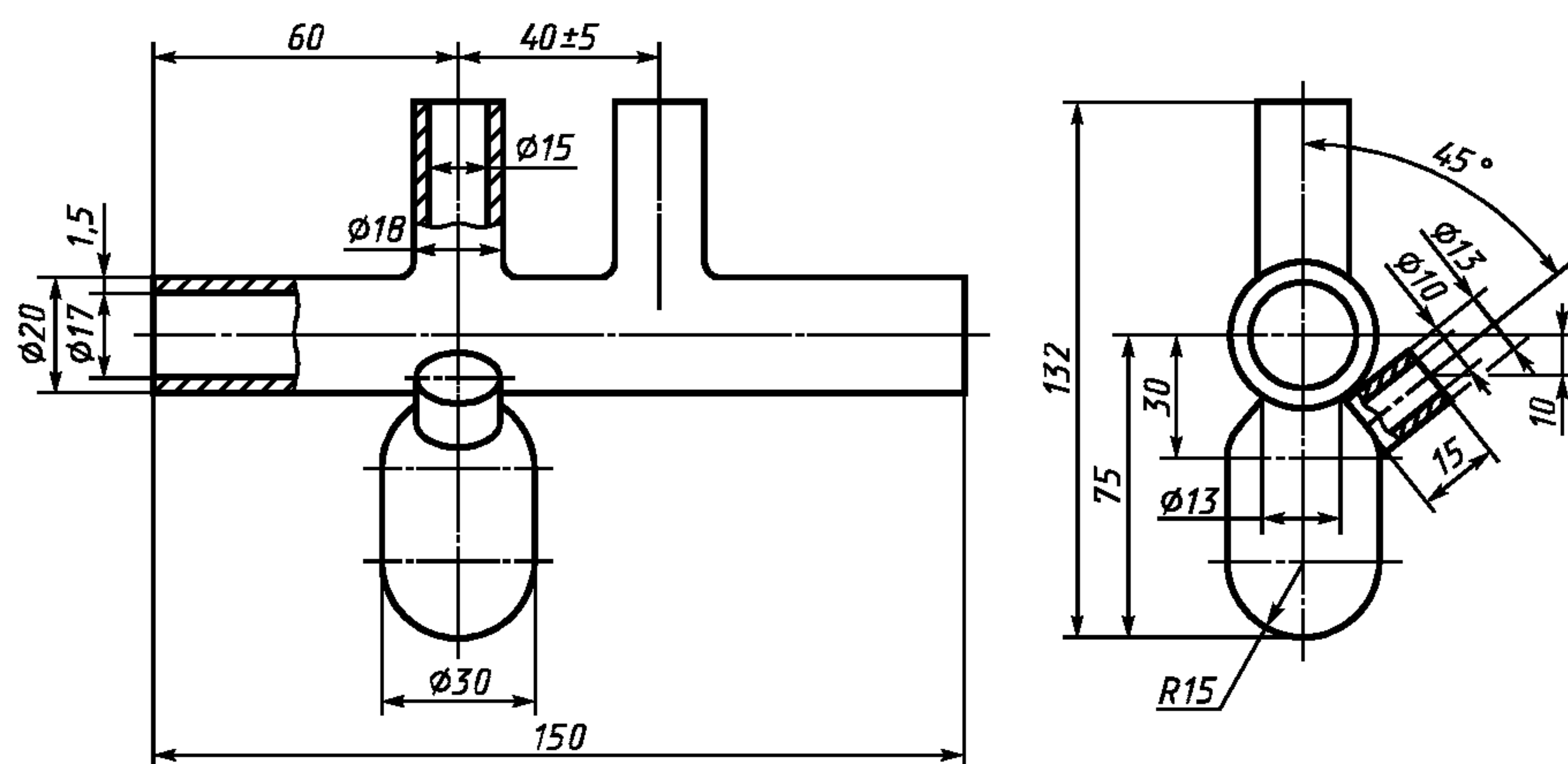
Рисунок Б.1 — Схема резервуара психрометра
