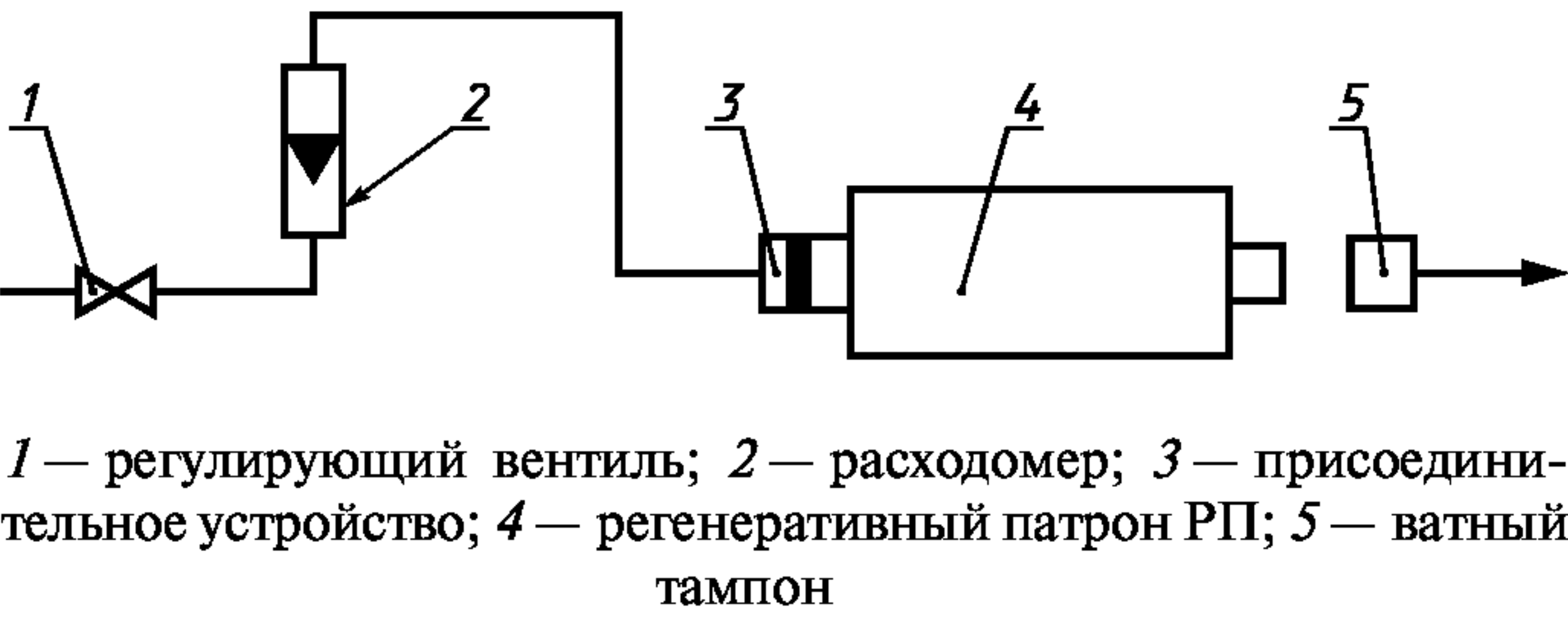
Рисунок 2 — Схема установки для определения наличия пыли регенеративного продукта
