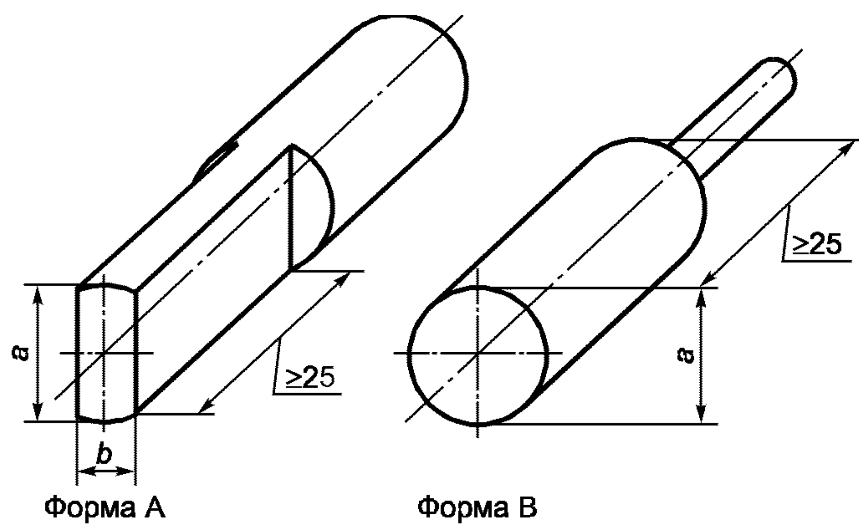
Рисунок 5 — Щупы (см. 9.2.4.5)
