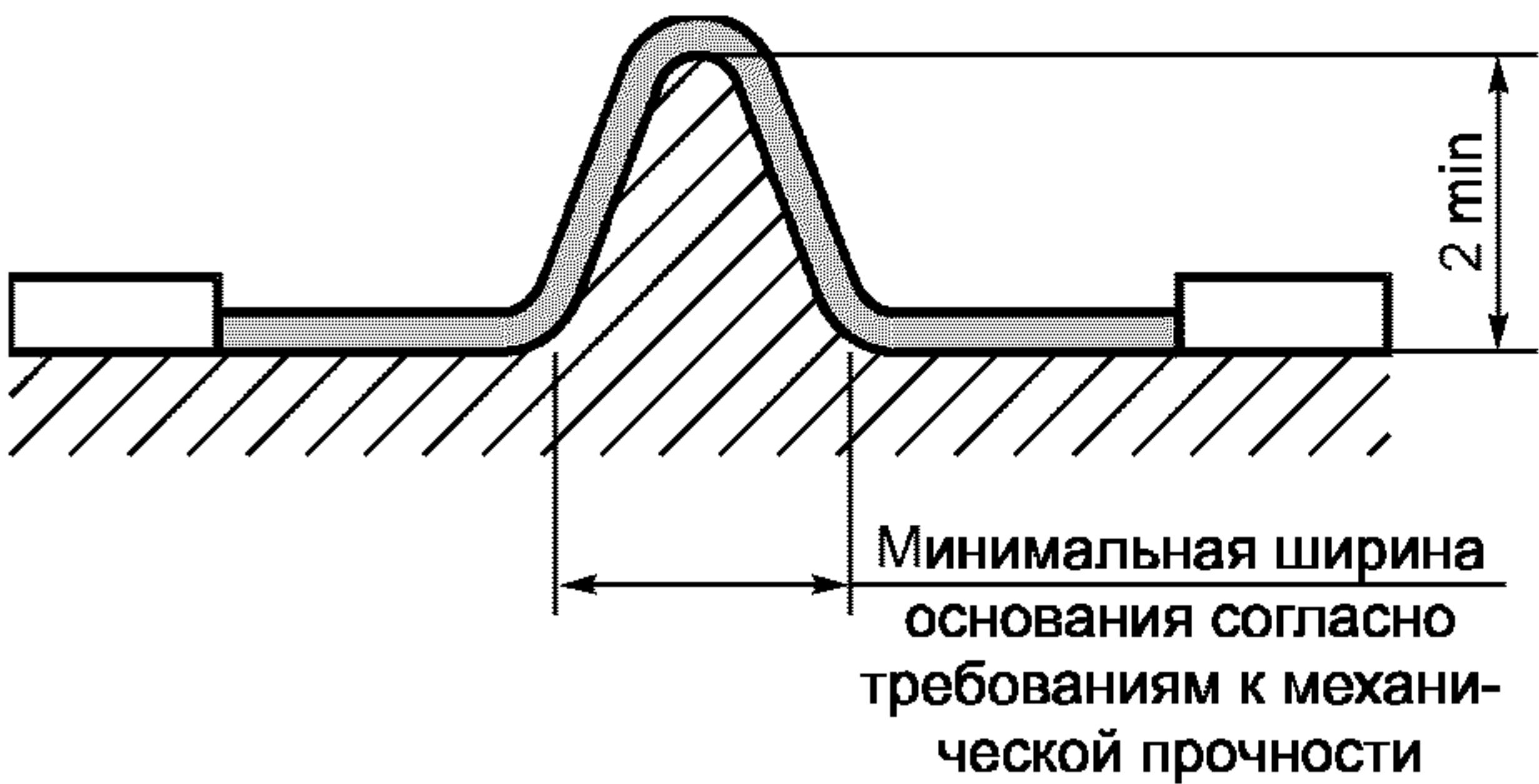
Рисунок Е.1 — Размеры ребер
