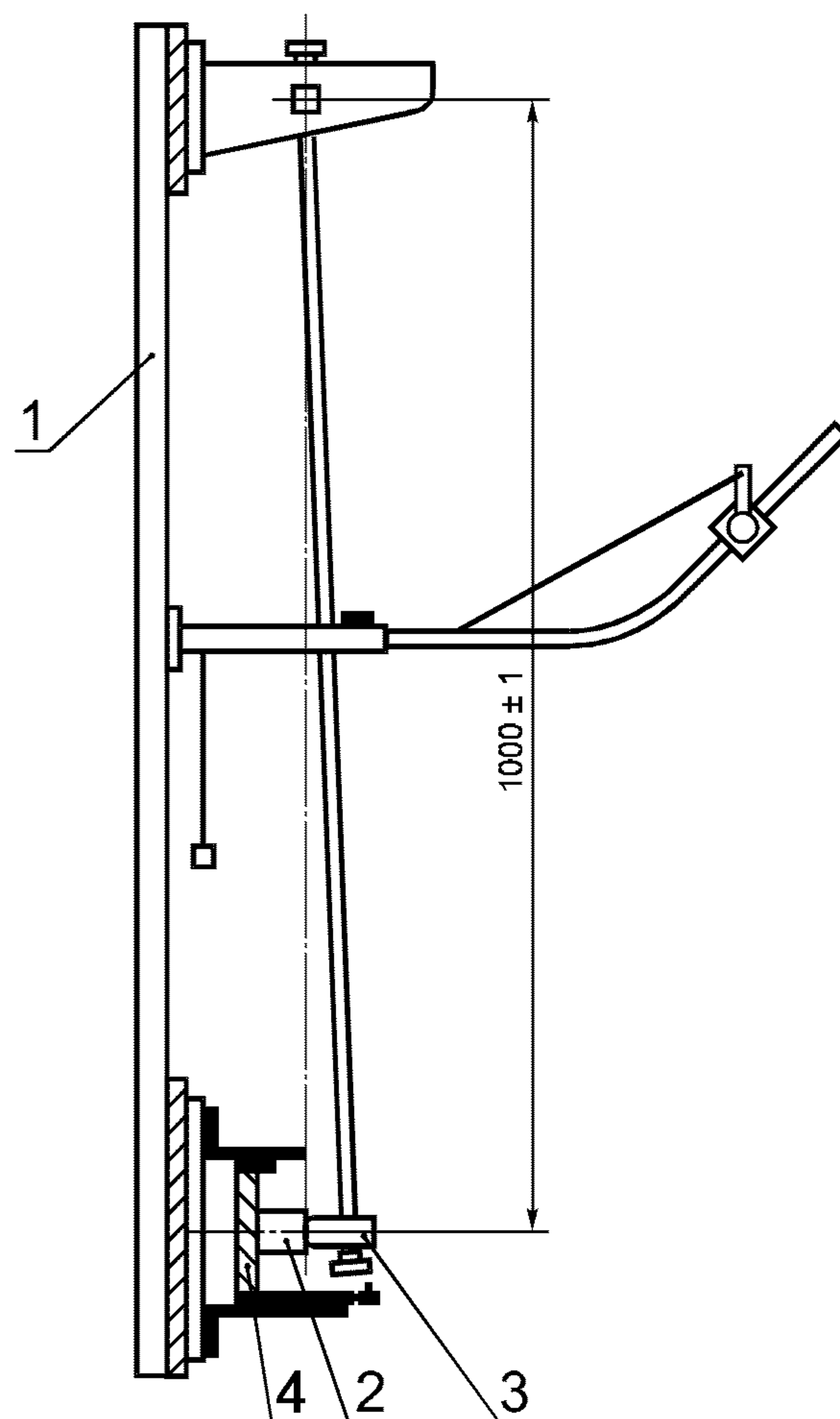
1 — опора; 2 — образец; 3 — ударный элемент; 4 — монтажная опора
