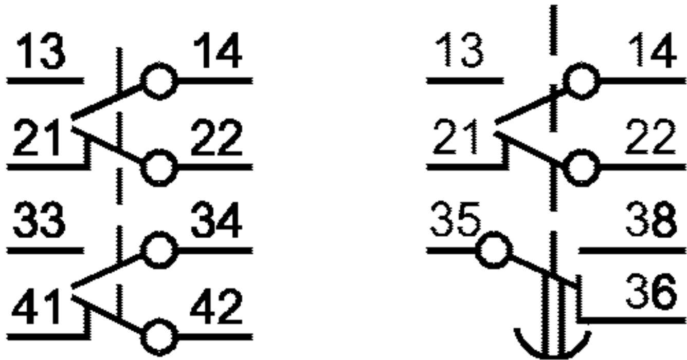
Четыре контактных элемента Три контактных элемента
