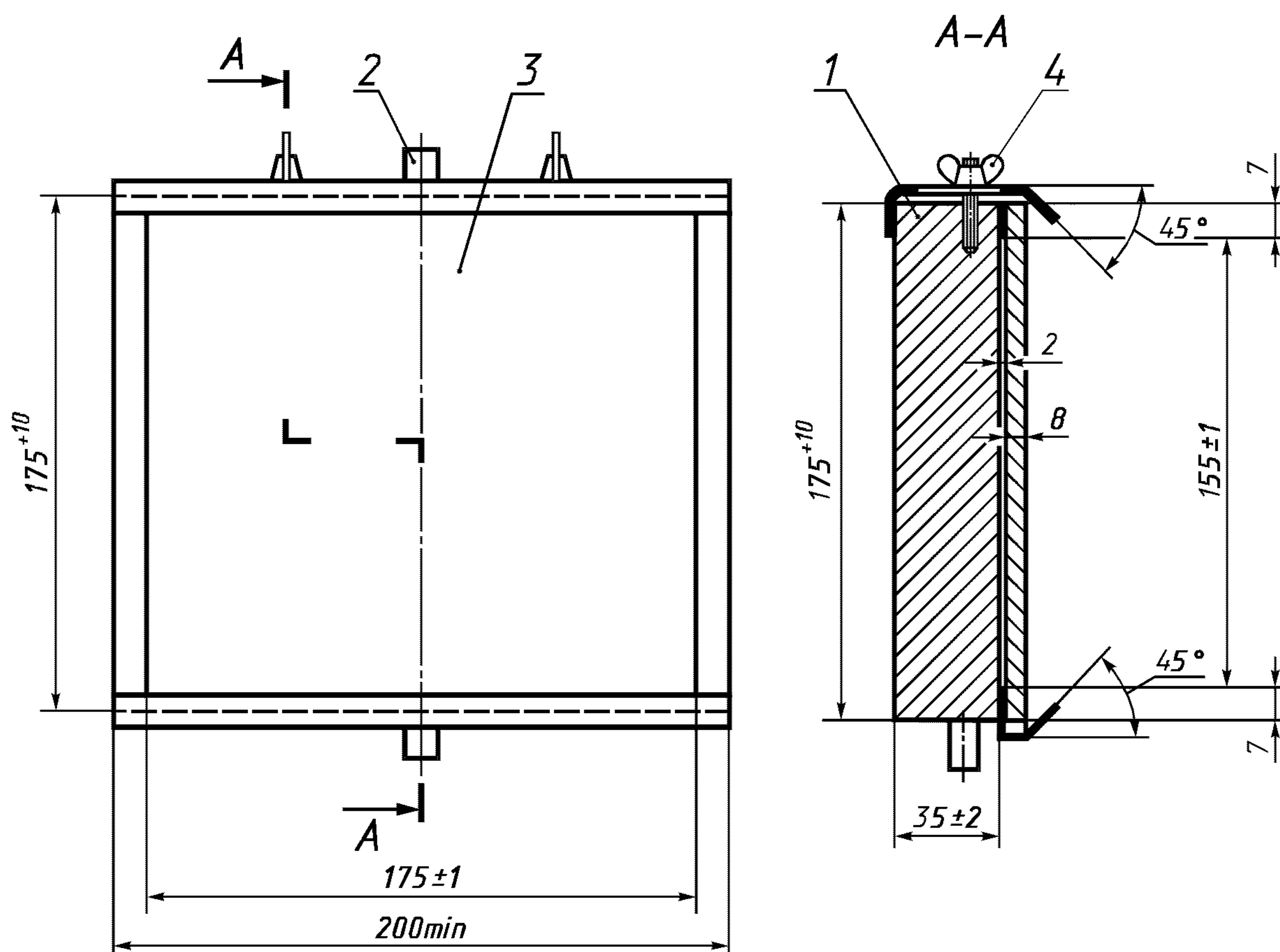
Рисунок 6 — Ударный элемент маятника для механических испытаний (см. 9.2.5.2.1)
