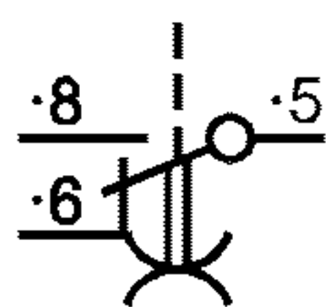
Переключающий контакт с замедлением в обоих направлениях
