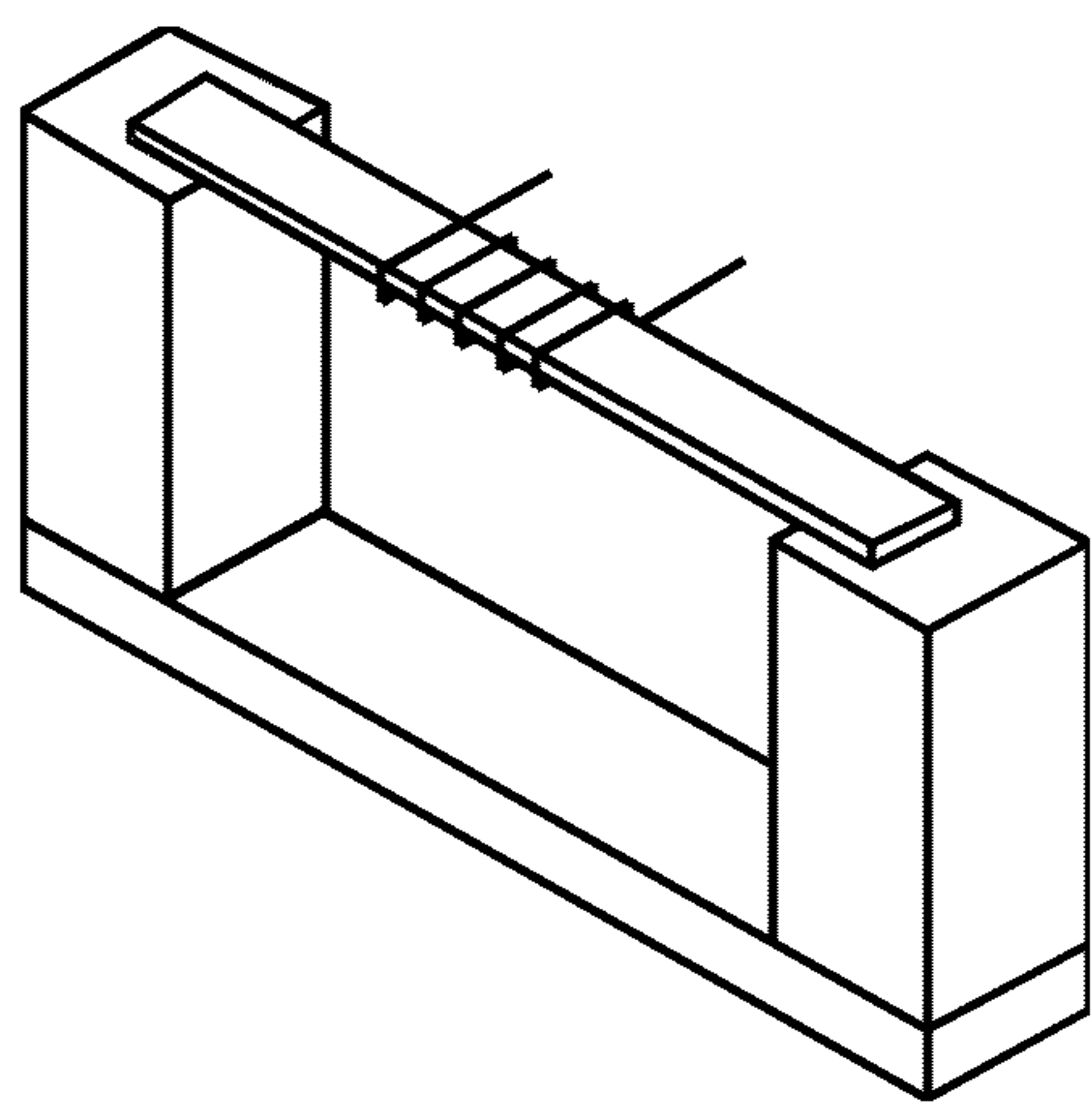
Рисунок G.1 — Приспособление для испытания нагретой проволокой
