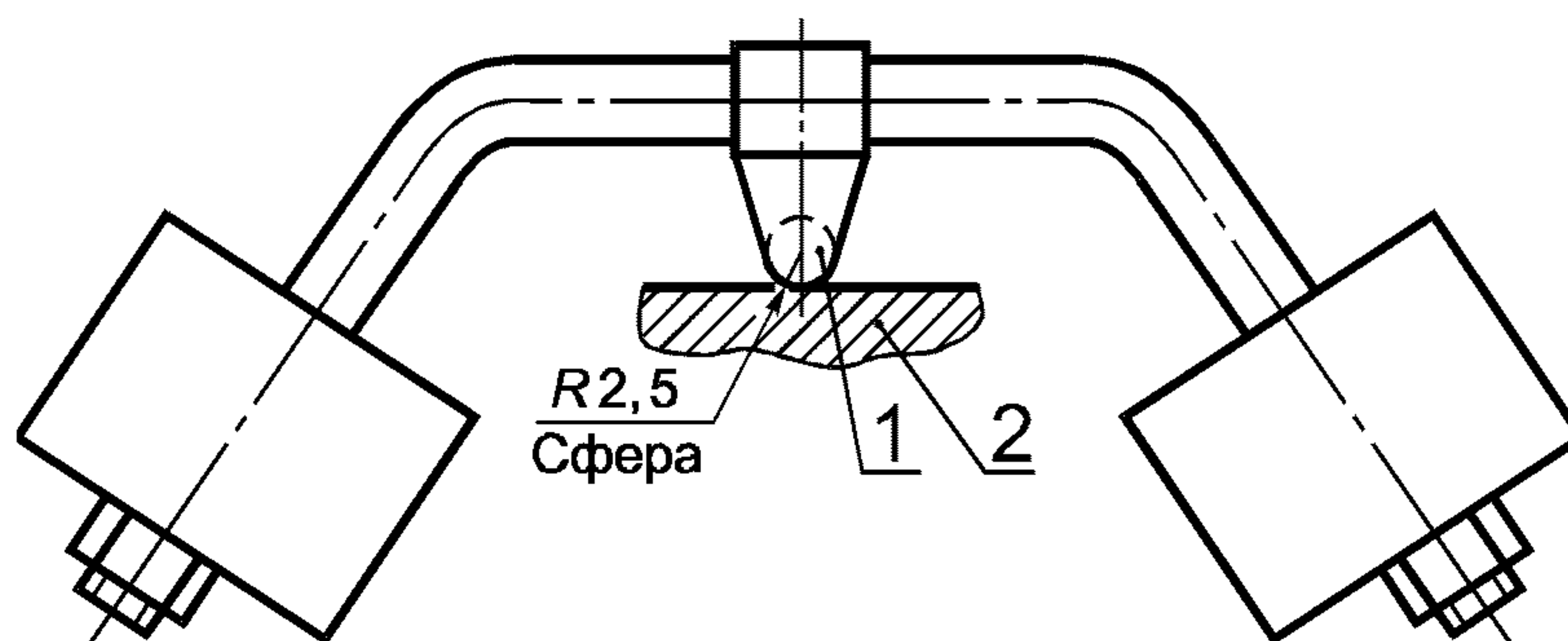
1 — стальной шарик; 2 — испытуемый образец
