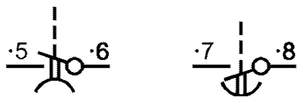
Размыкающий контакт с замедлением при замыкании
