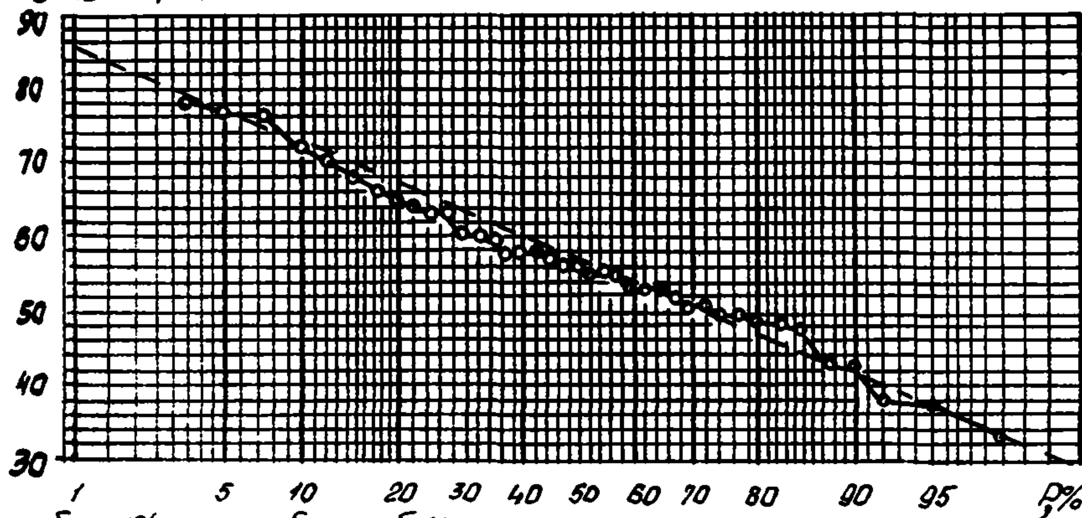
График для определения расчетной толщины льда
