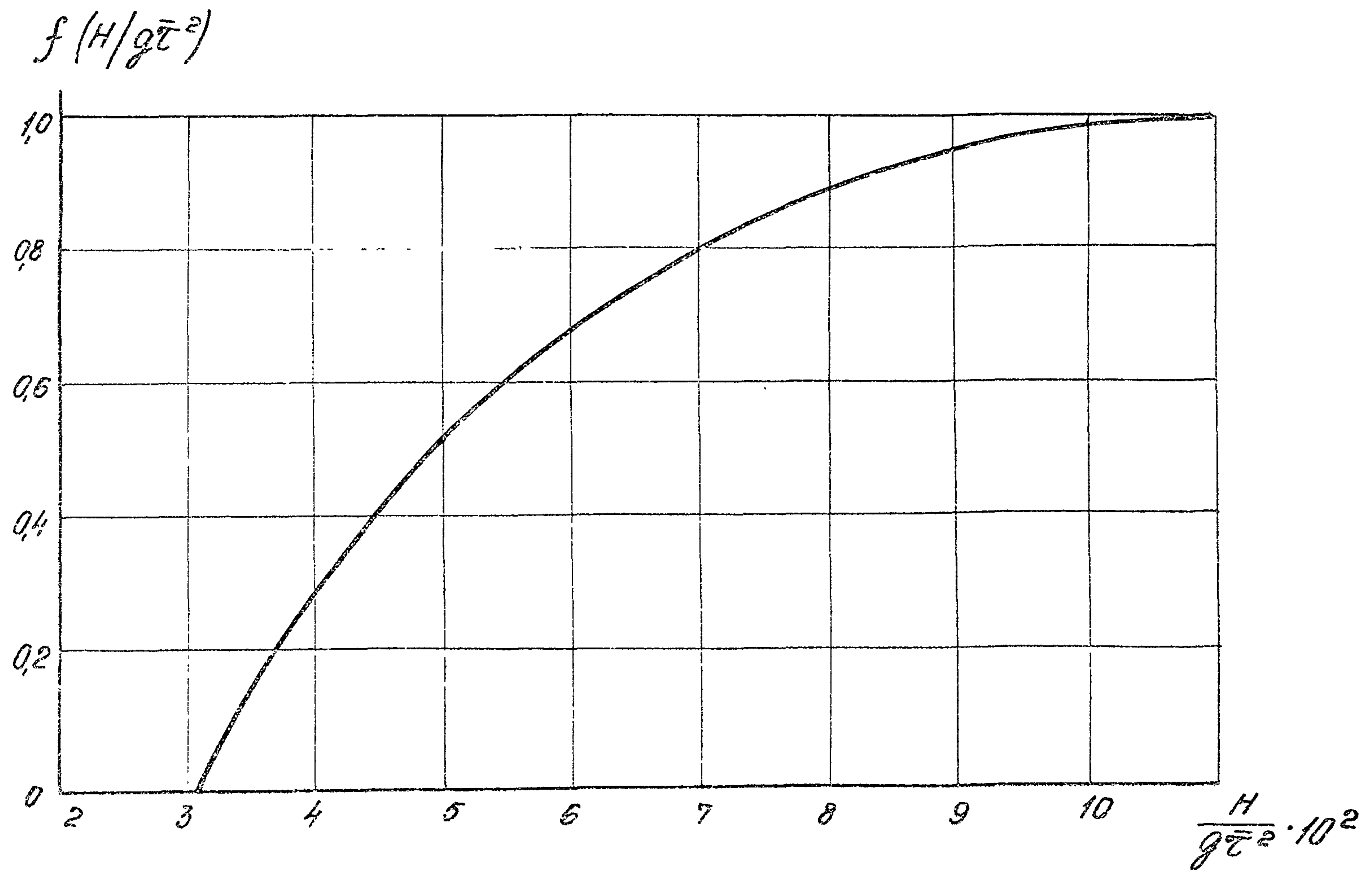
Рис. 4. 6. Зависимость функции f(H/q\tau^2) от параметра безразмерной глубины моря.
