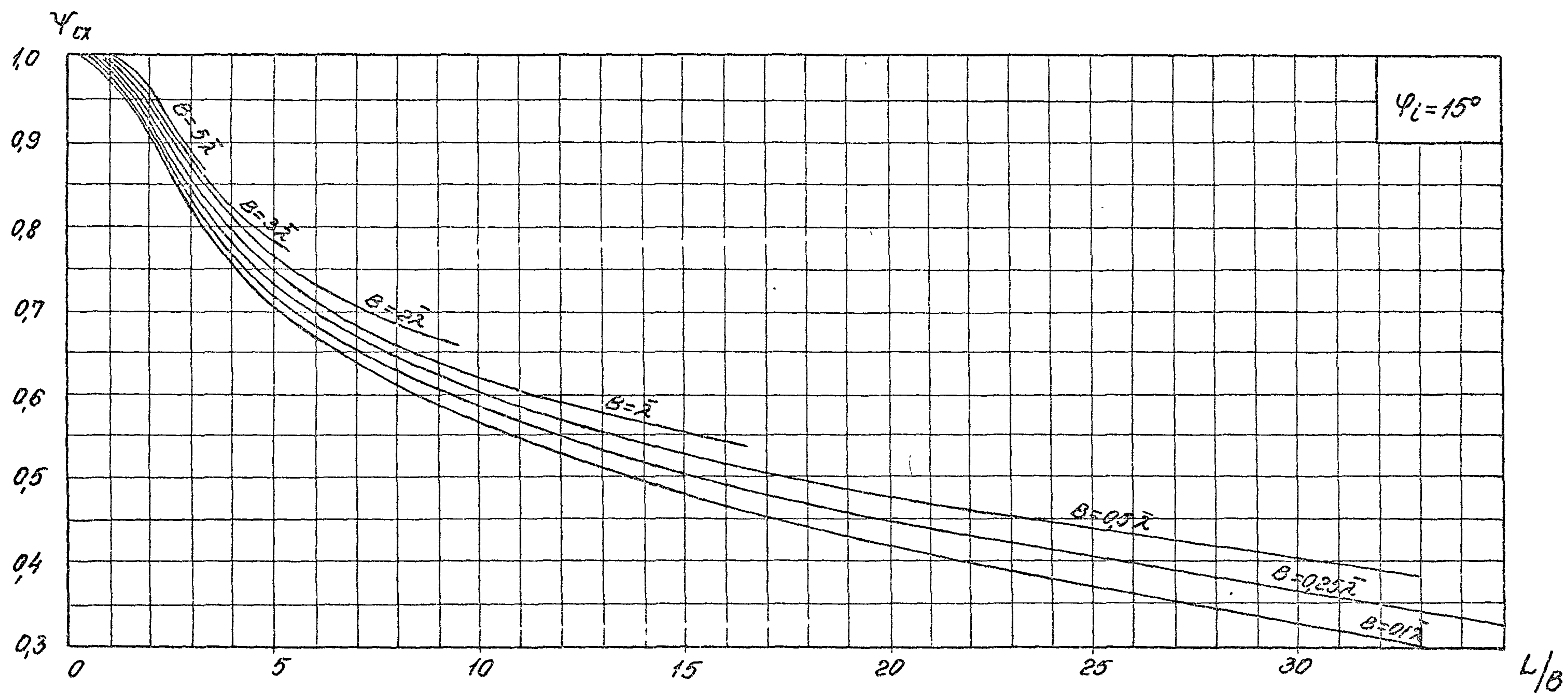
Рис. 12. Графики для определения \psi_{сх} при угле \psi_L = 15^\circ .
