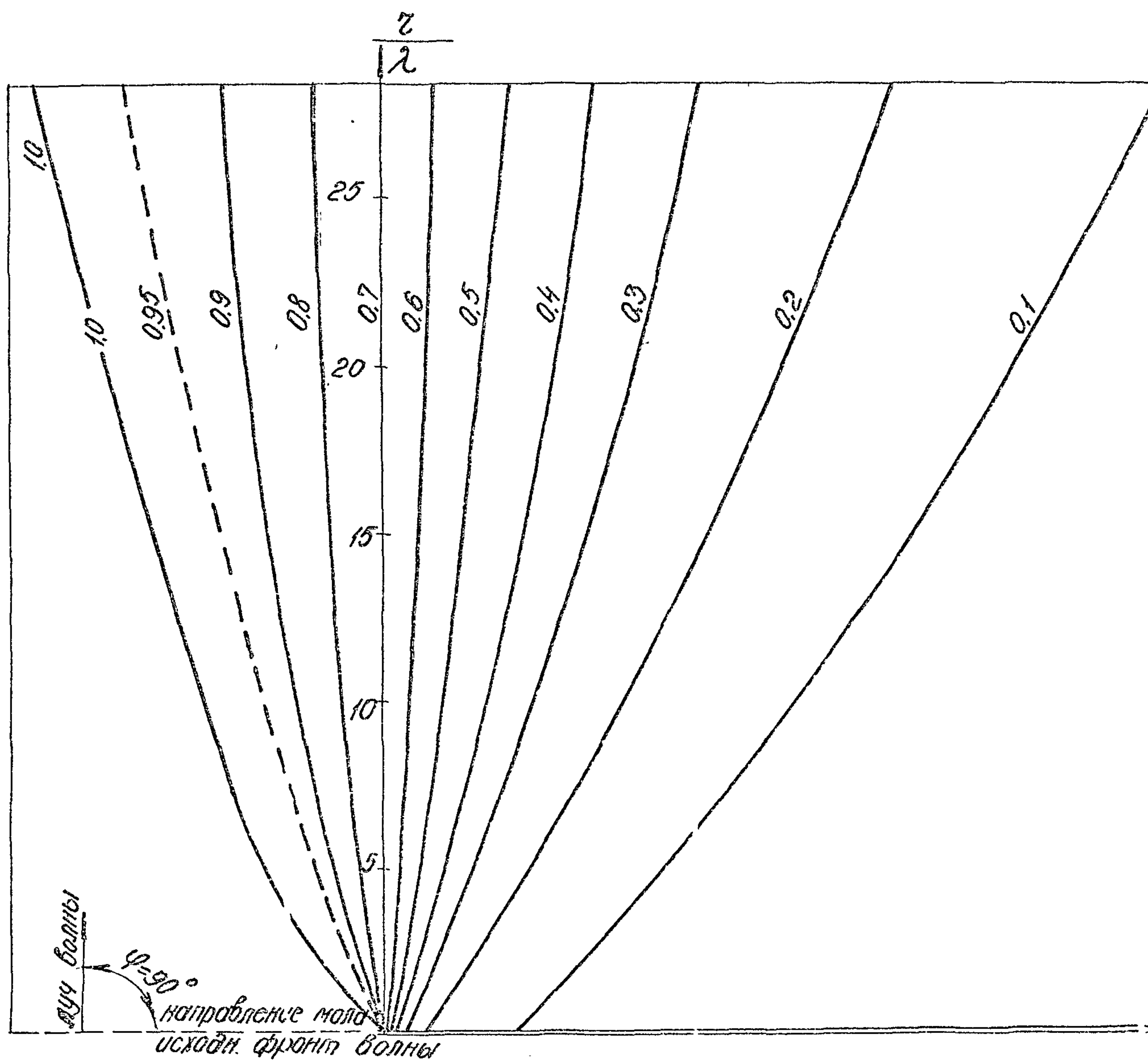
Рис. 9. График для определения коэффициента дифракции K_{d0} для угла \psi = 90^\circ .
