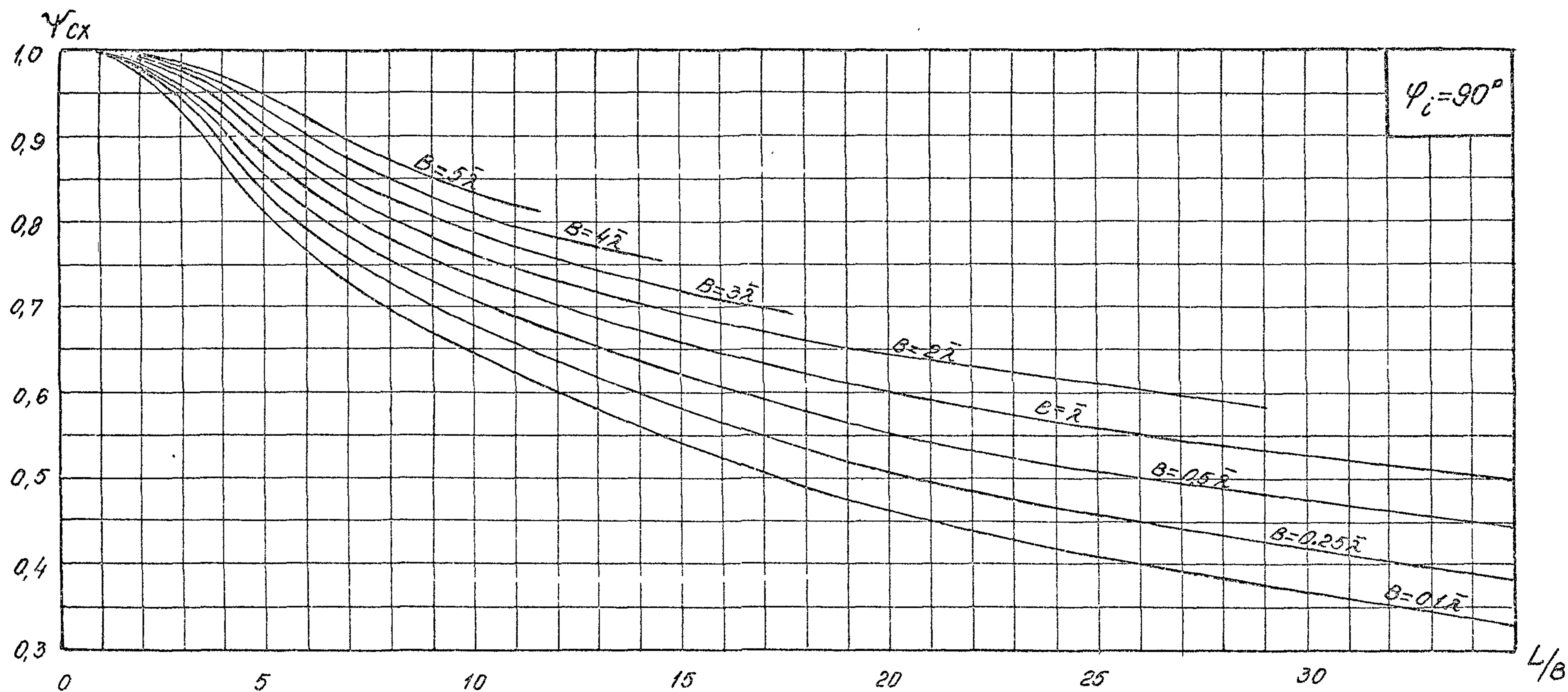
Рис.18. График для определения коэффициента \psi_{cx} при угле \varphi_i = 90^\circ .
