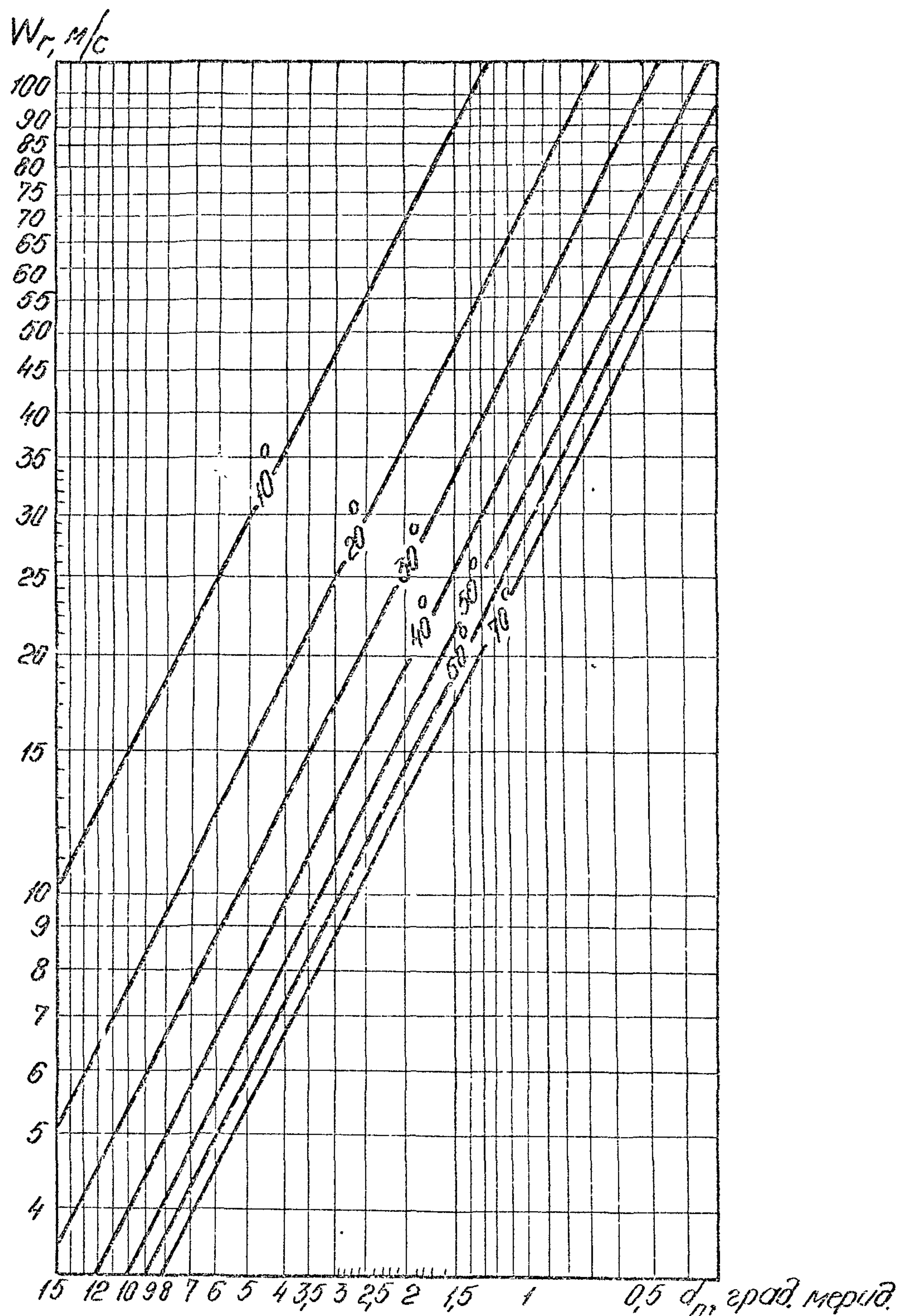
Рис. 2.2 График для определения скорости геострофического ветра W_r , м/с, по расстоянию между изобарами d_m , град. мерид., и широте места \varphi , град.
