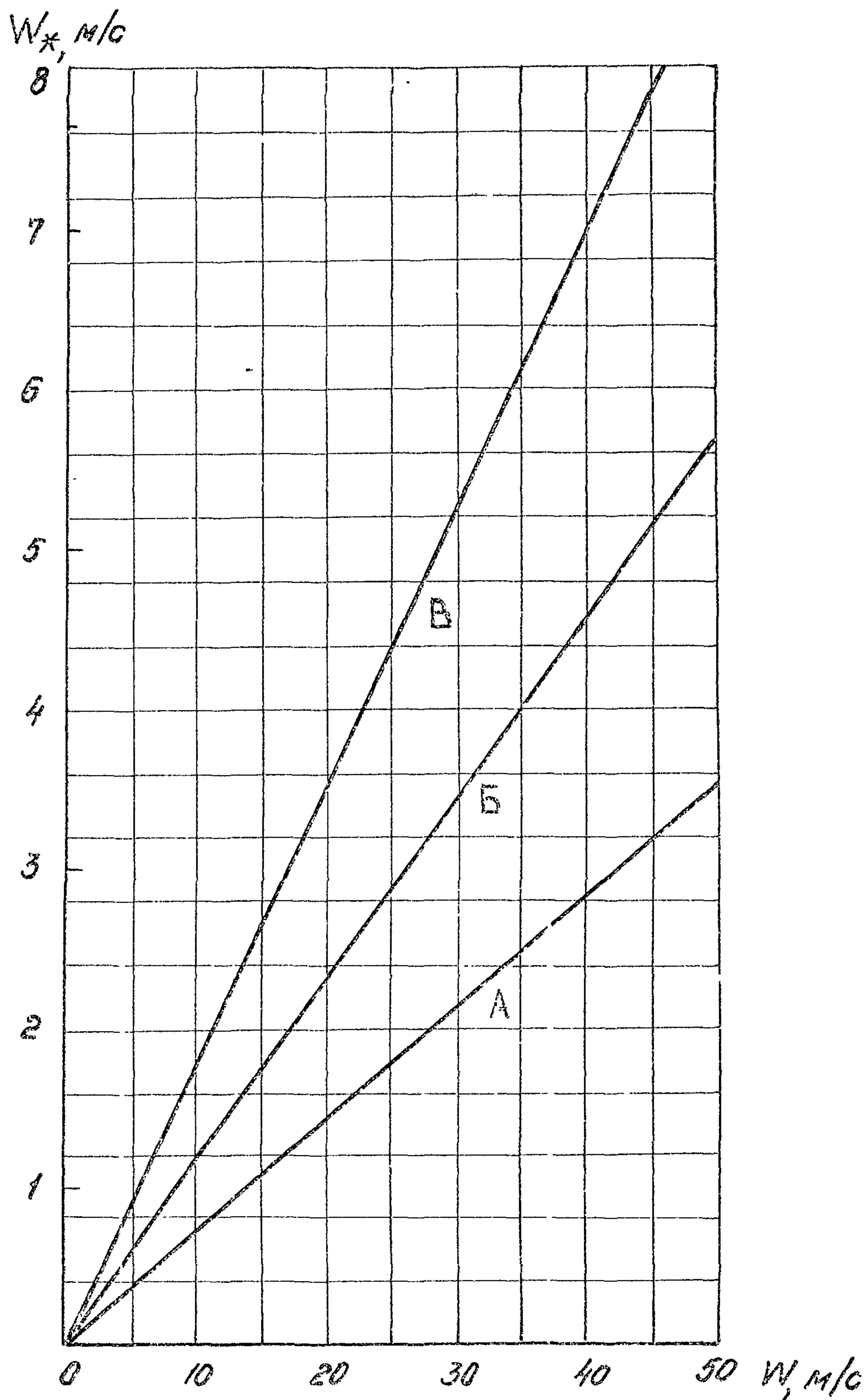
Рис. 2.6. График для определения динамической скорости W_* , м/с, по скорости ветра W , м/с, на горизонте 10 м для разных типов местности.
