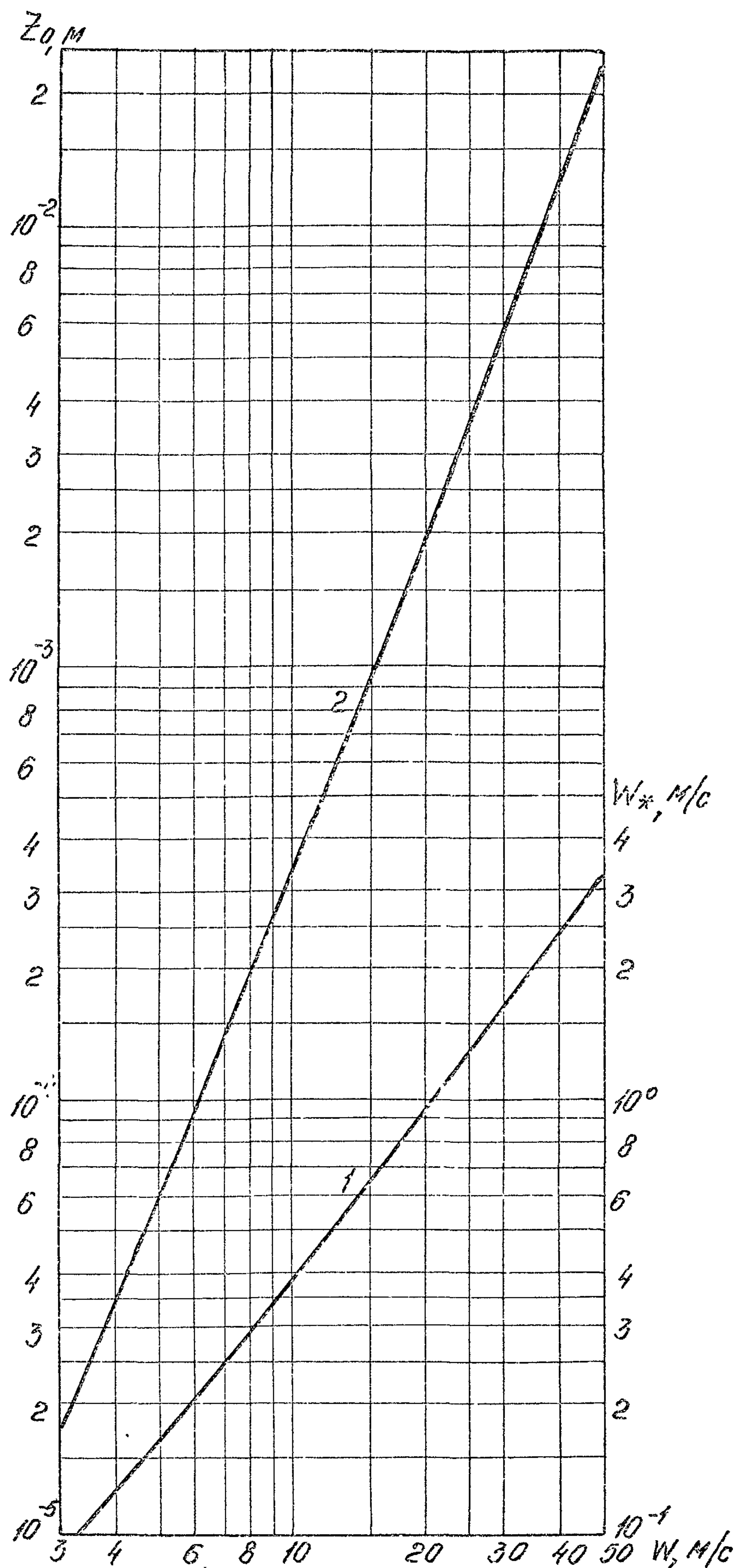
Рис.2.5 График для определения динамической скорости W_* , м/с, (линия 1) и параметра шероховатости Z_0 , м, (линия 2) по скорости ветра W , м/с, на горизонте 10 м.
