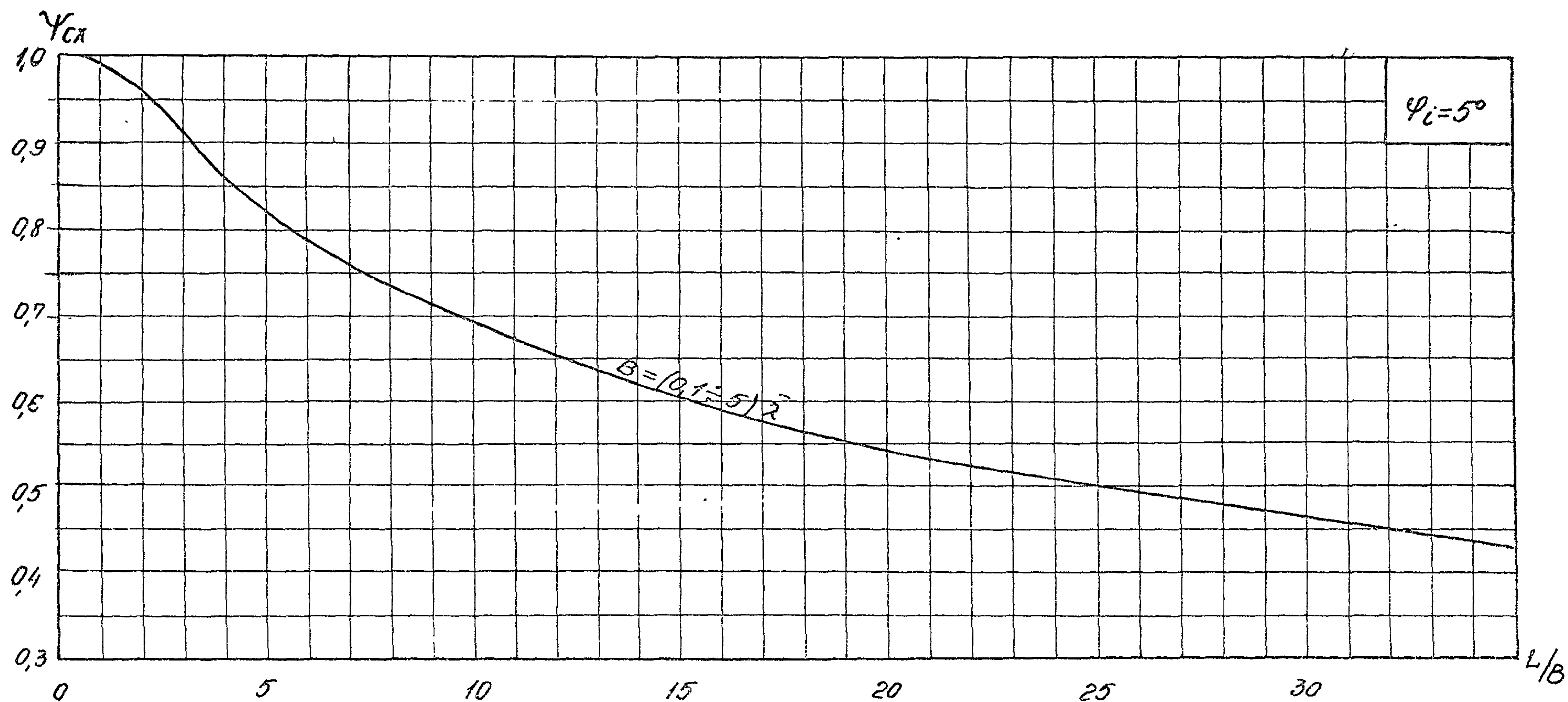
Рис. 10. График для определения коэффициента \Psi_{сх} при угле \varphi_i = 5^\circ .
