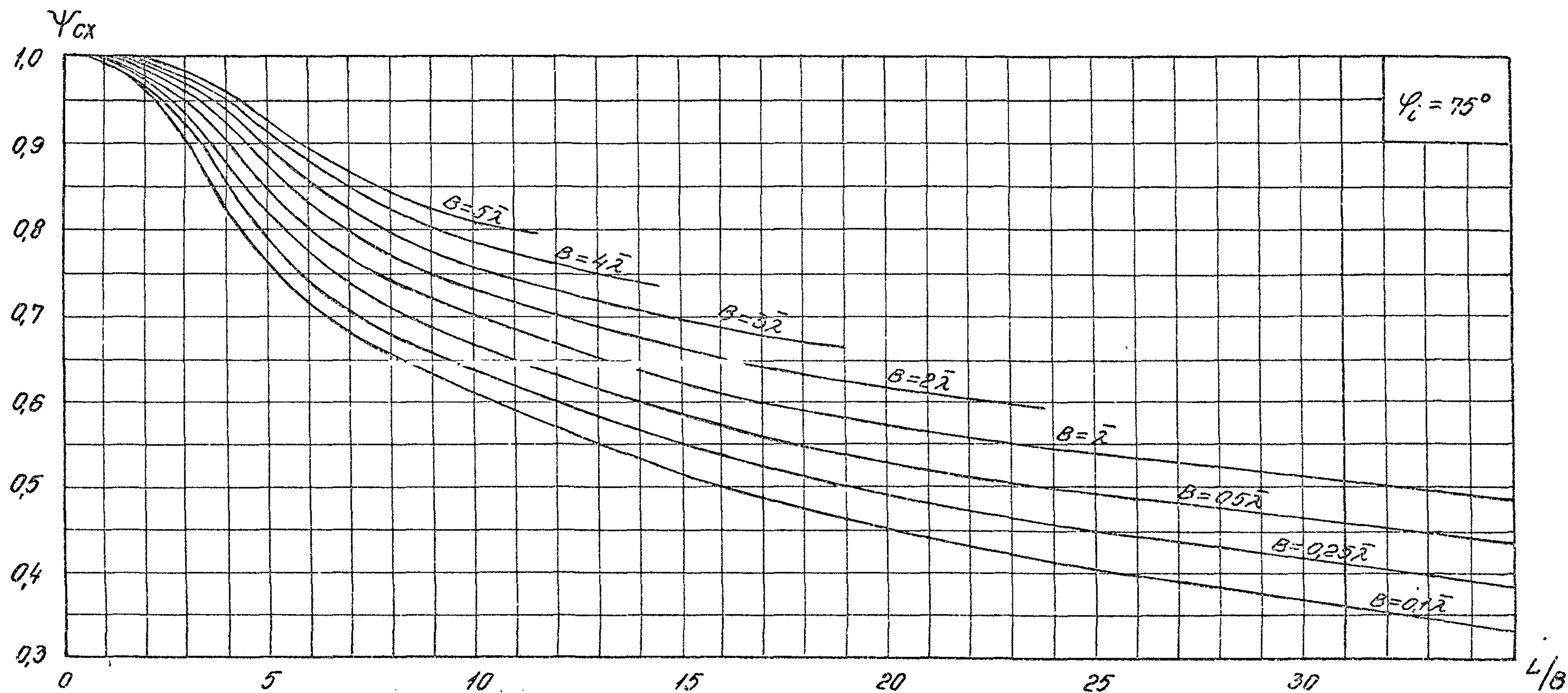
Рис. 17. График для определения коэффициента \psi_{cx} при угле \varphi_c = 75^\circ .
