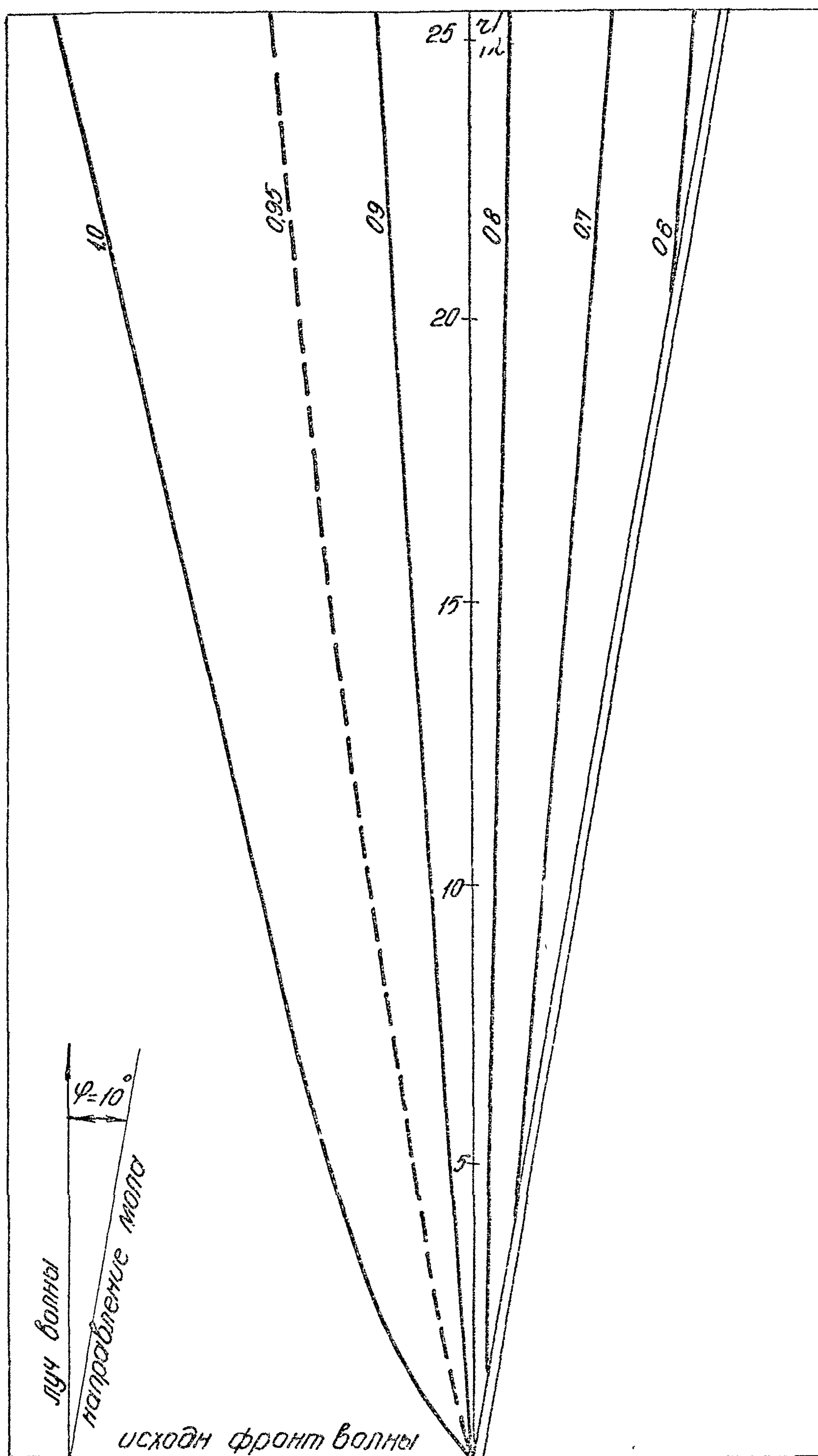
Рис. 2. График для определения коэффициента дифракции K_{d0} для угла \psi = 10^\circ .
