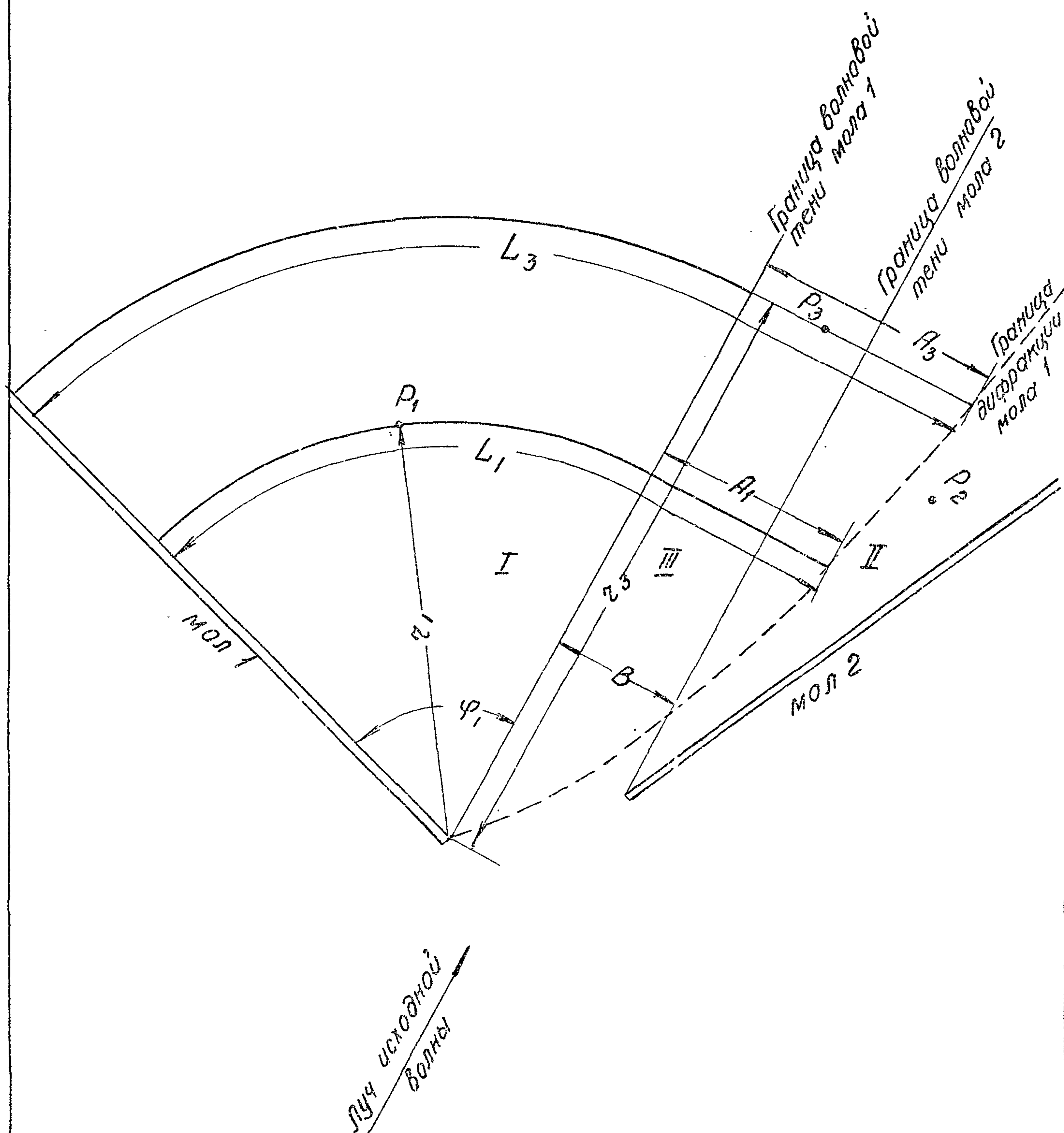
Рис. 4.4. Схема акватории порта, огражденного двумя сходящимися молами
