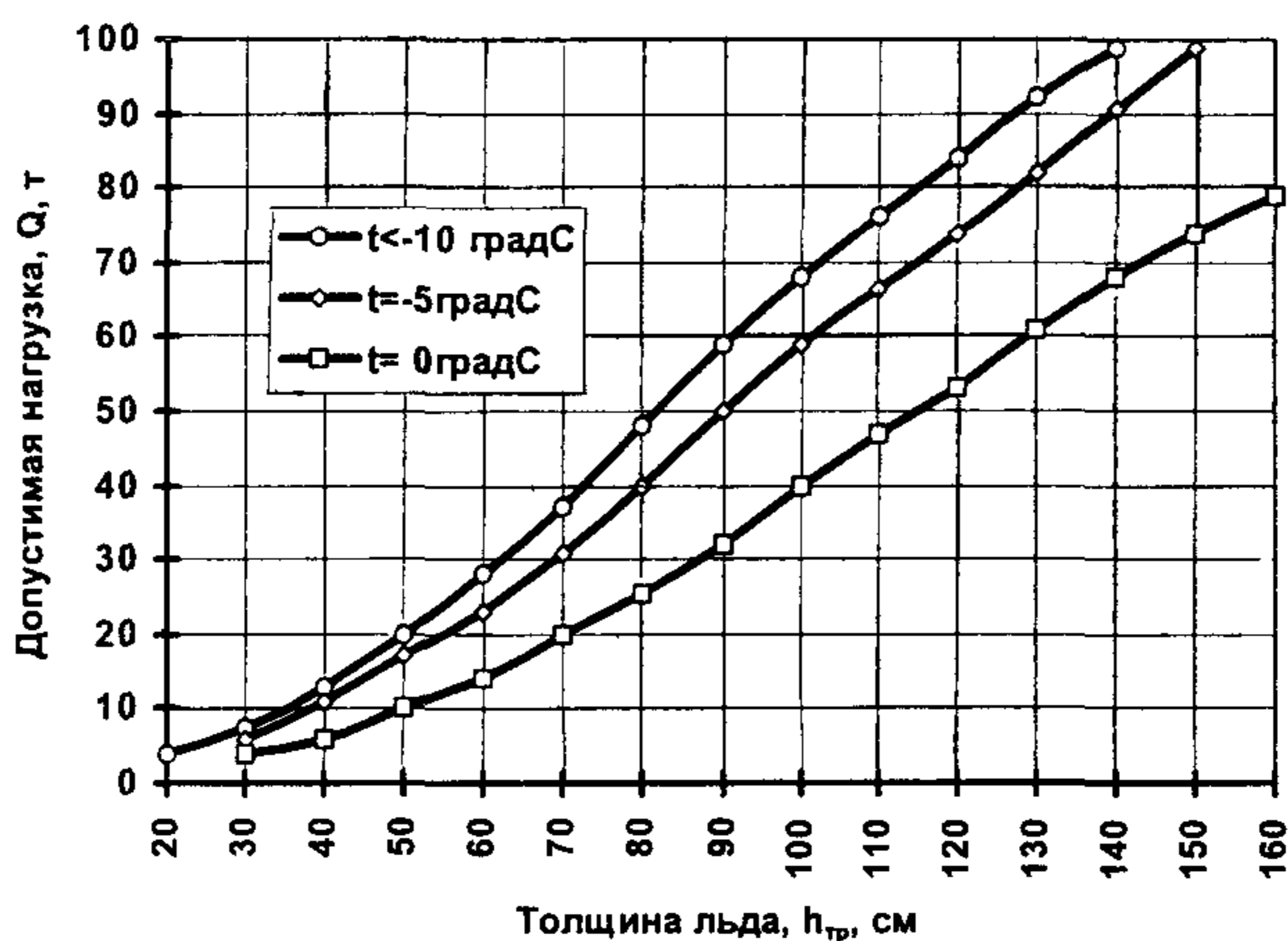
Рис.П.2.2. Допустимые нагрузки на ледяной покров при пропуске по нему колесных автомобилей
