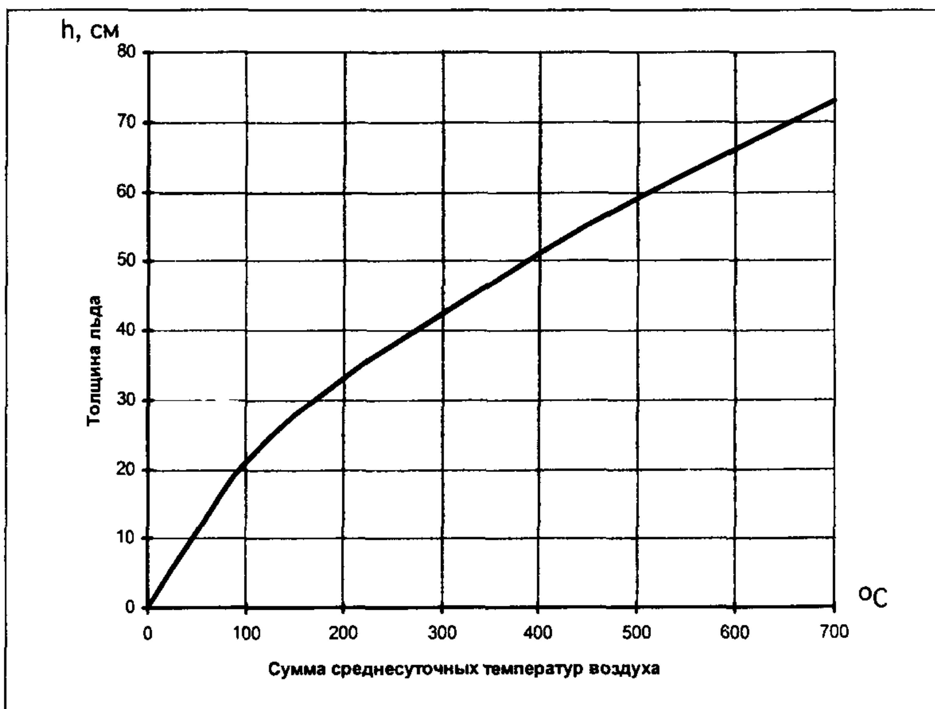
Рис.4.5. График нарастания толщины пресноводного льда, очищенного от снега, на водоемах без течения
