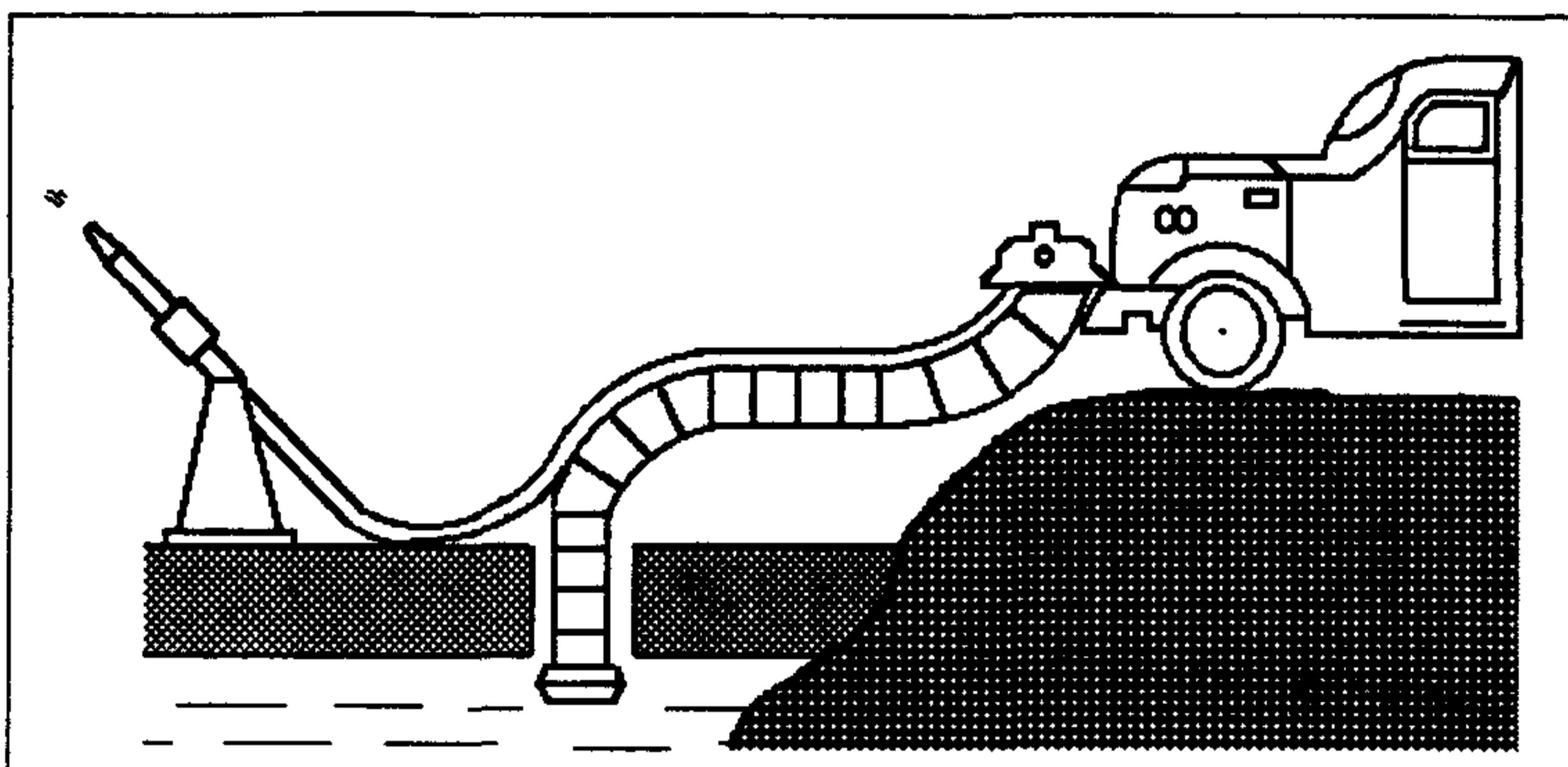
Рис.П.4.3. Намораживающий агрегат "Град-3"
