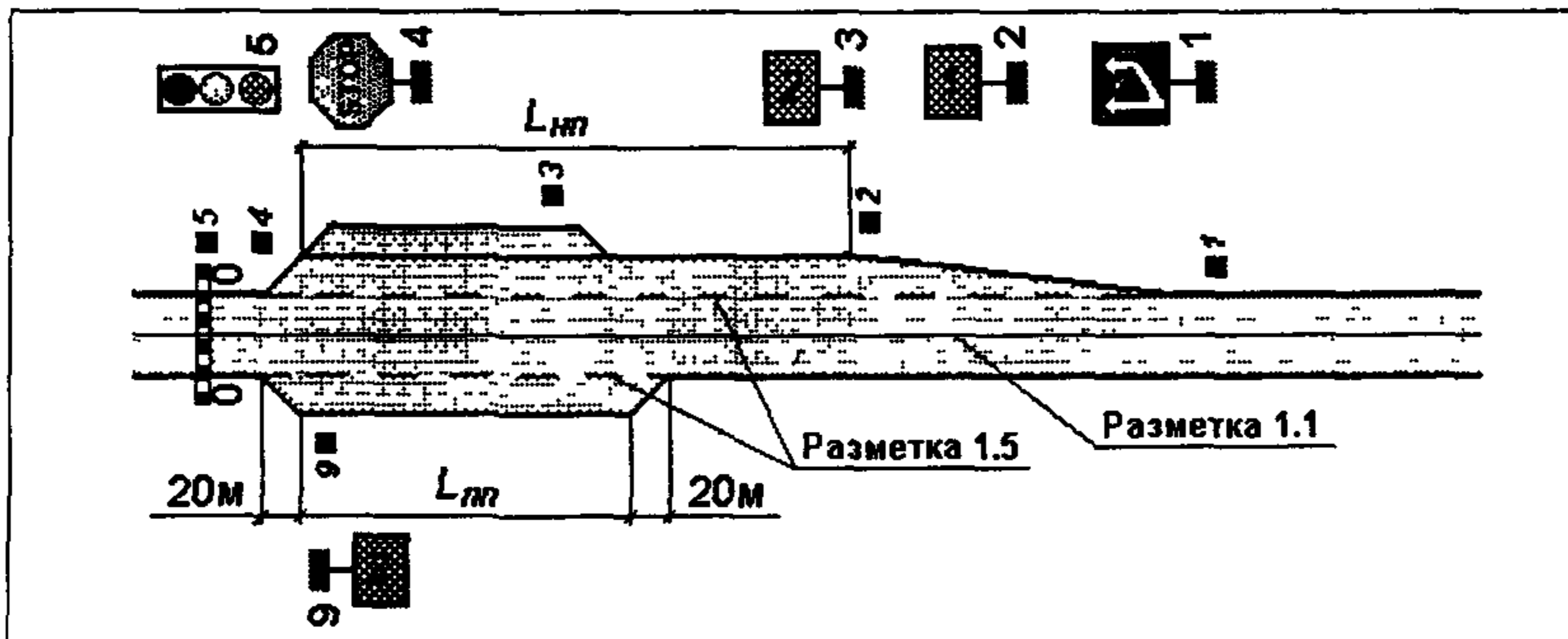
Рис.8.5. Принципиальная схема организации движения на подходах к ледовой переправе в зонах накопительных и посадочных полос 1 - транспарант "Левая полоса для приоритетного движения", 2 - транспарант "Место для высадки пассажиров", 3 - транспарант "Место для посадки пассажиров"
