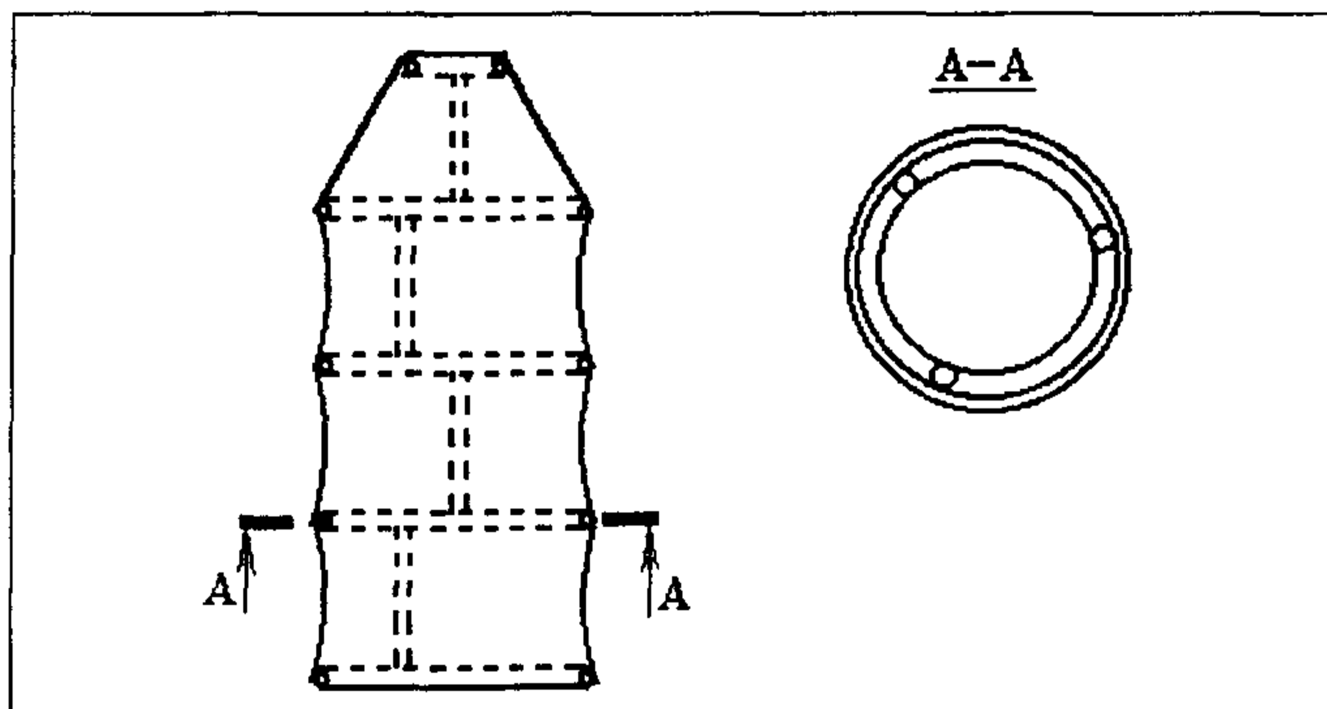
Рис.6.3. Объемный компенсатор
