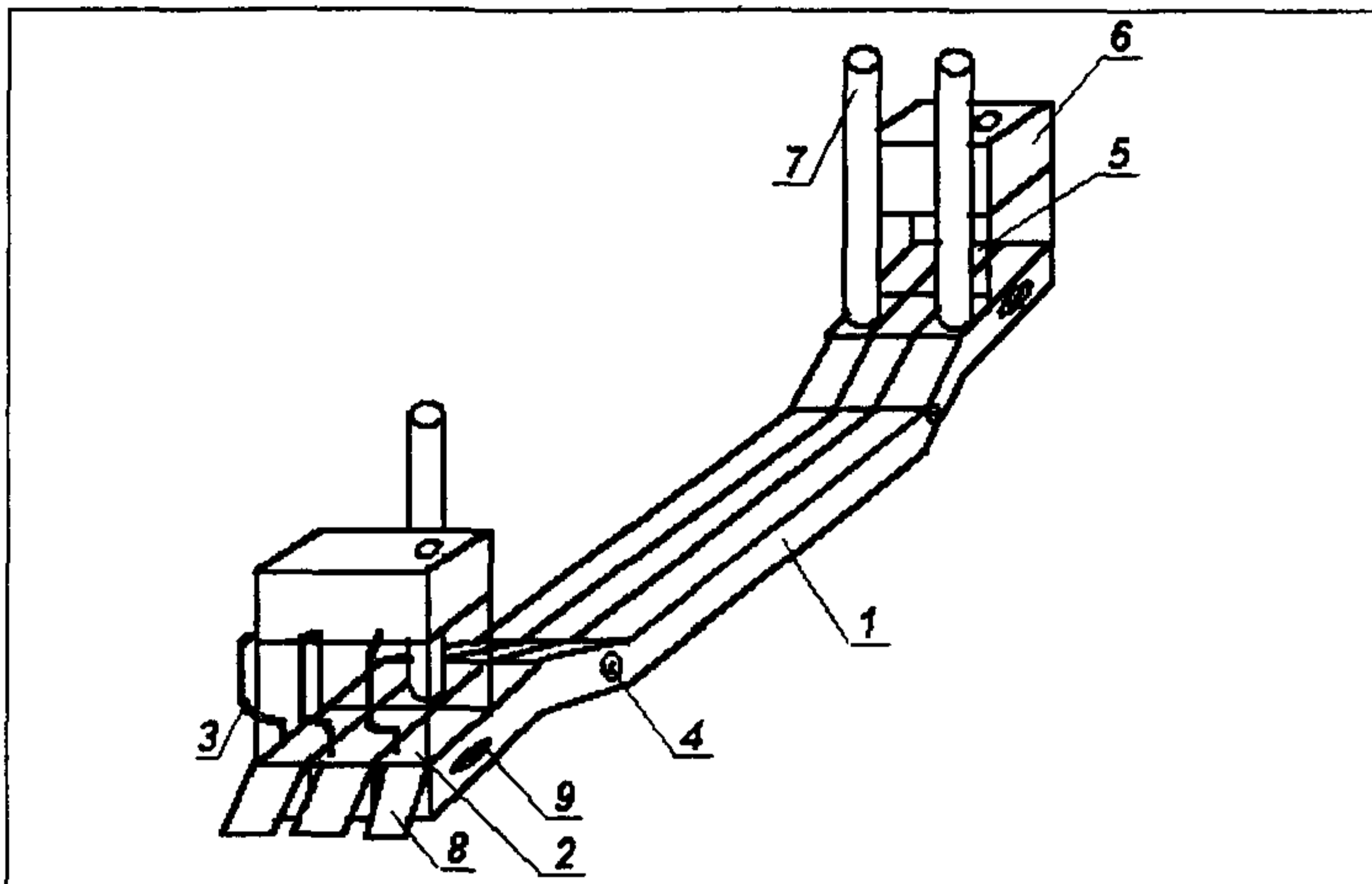
Рис.6.2. Общий вид термолыжи. 1 - полозья, 2 - основная топка, 3 - топливопровод, 4 - сцепное устройство, 5 - стартовая топка, 6 - топливный бак, 7 - дымовая труба, 8 - крышка топки, 9 - рым
