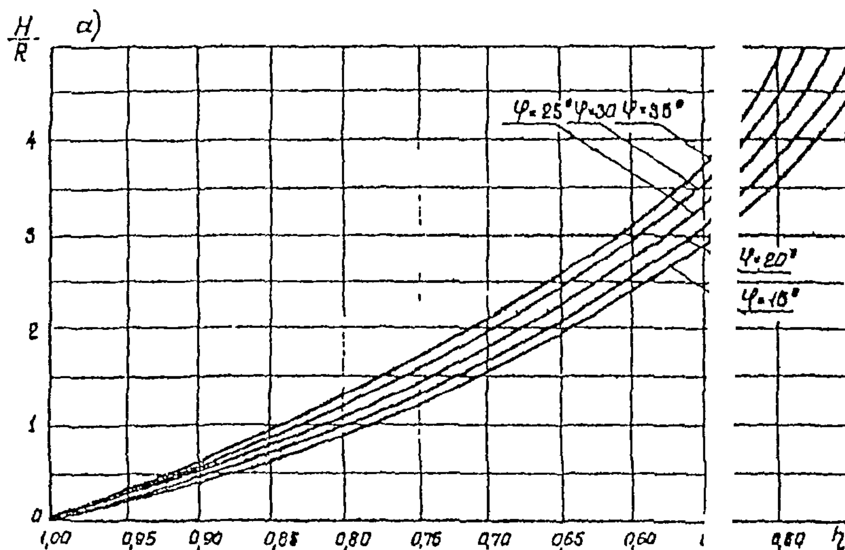
Черт. 11.2. График изменения коэффициента \eta
