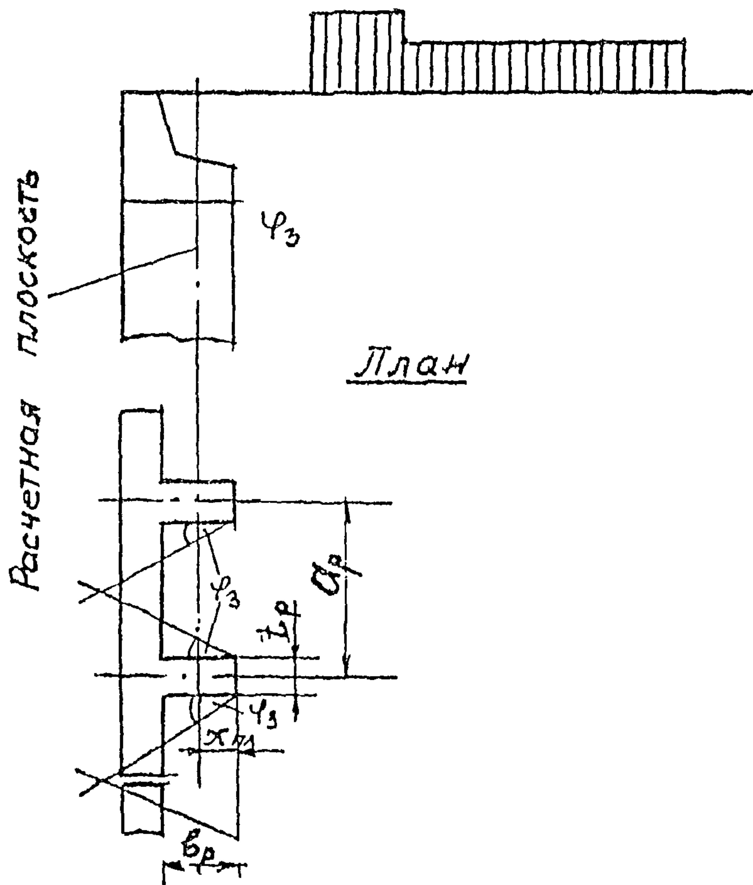
Черт. 7.12. Схема определения расчетной плоскости
