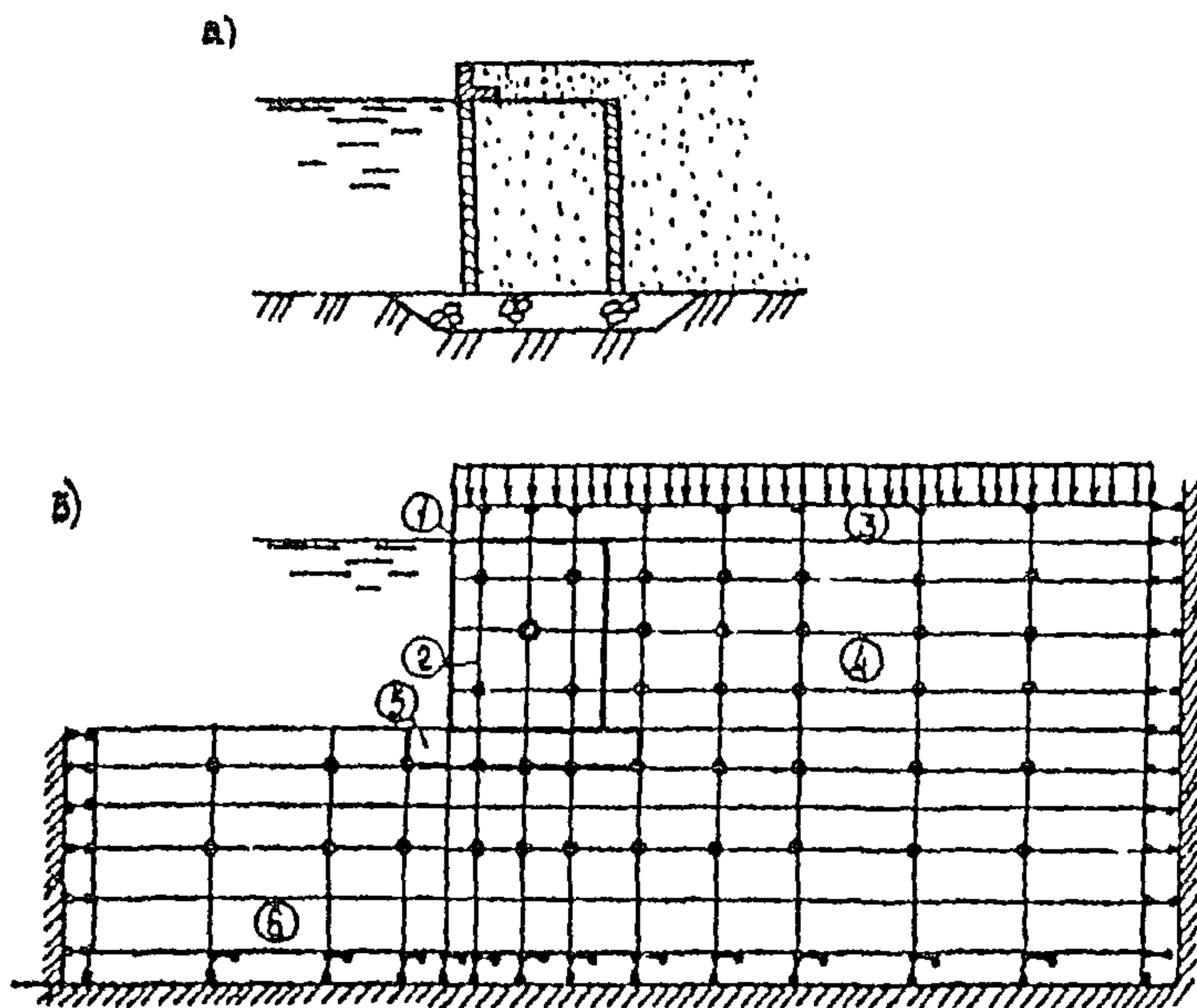
Черт. 3. Динамическая расчетная схема сооружения гравитационного типа
