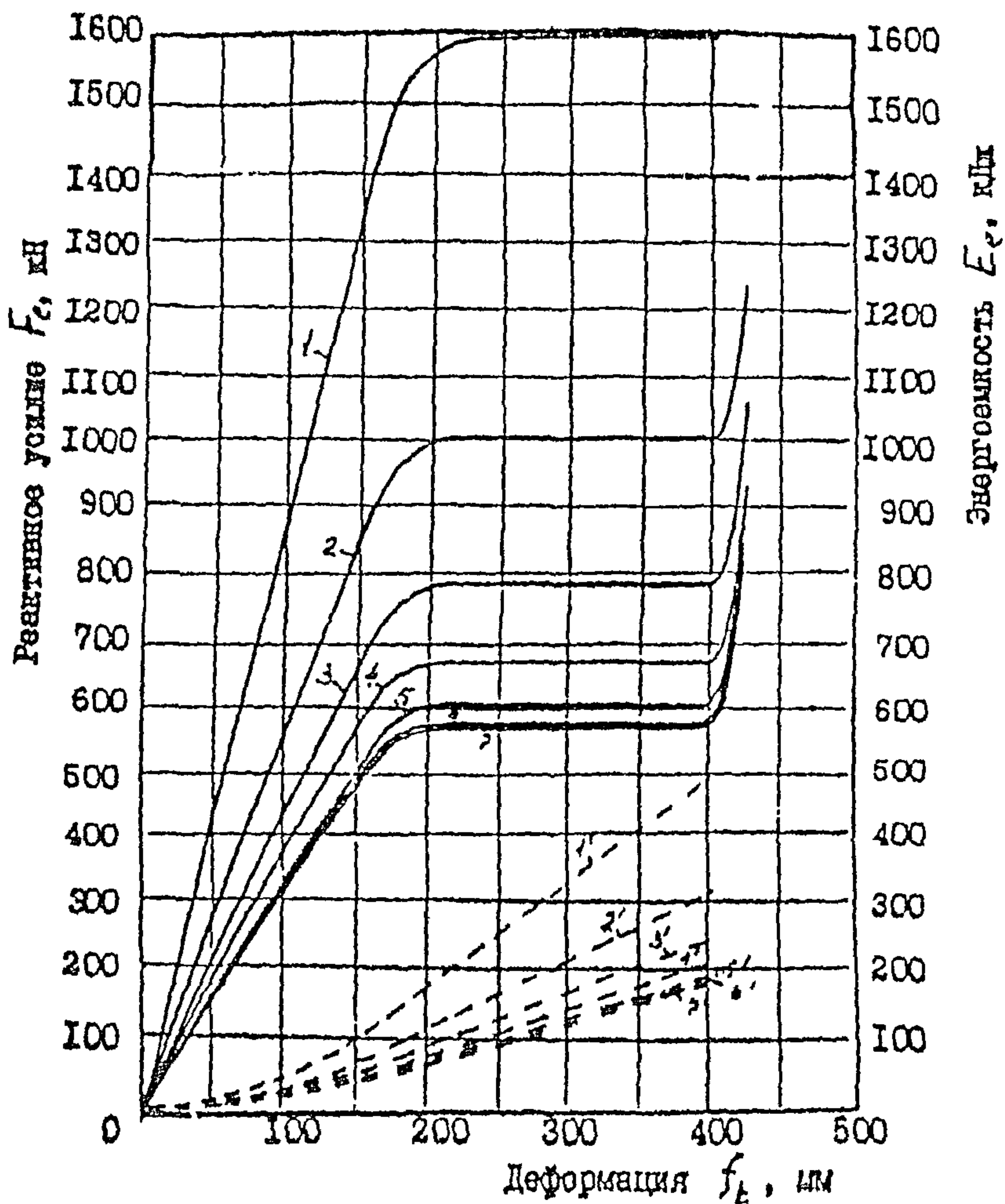
Черт. 3. Графики зависимости реактивного усилия F_r (сплошные линии) и энергоемкости E_r (штриховые линии) от деформации f_L амортизационного устройства РАТ-1000 при температурах: -40^{\circ}\text{C} - кривая 1; -30^{\circ}\text{C} - кривая 2; -20^{\circ}\text{C} - кривая 3; -10^{\circ}\text{C} - кривая 4; 0^{\circ}\text{C} - кривая 5; 10^{\circ}\text{C} - кривая 6; 25^{\circ}\text{C} - кривая 7
