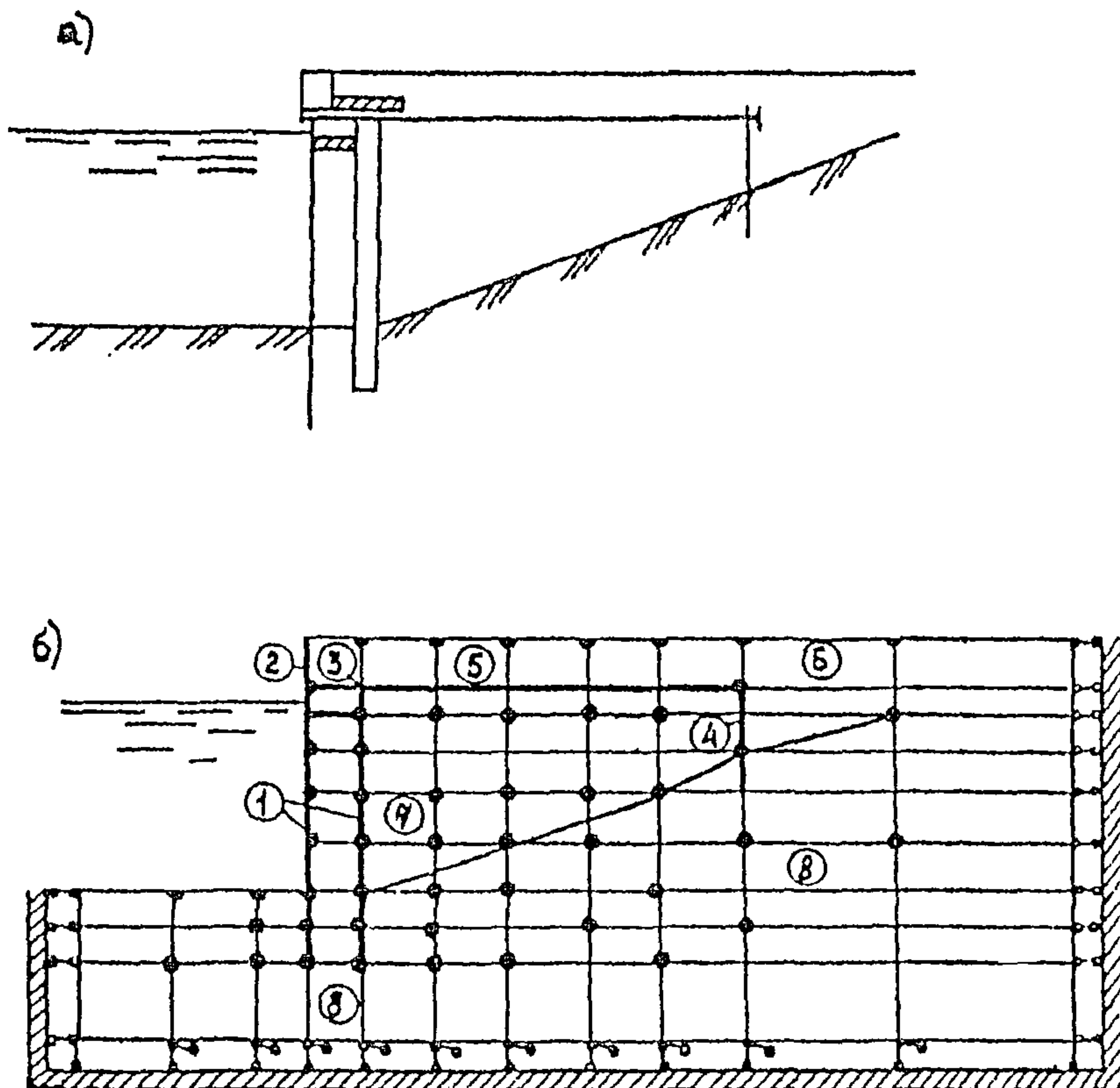
Черт. 5. Динамическая расчетная схема экранированного боль- верка
