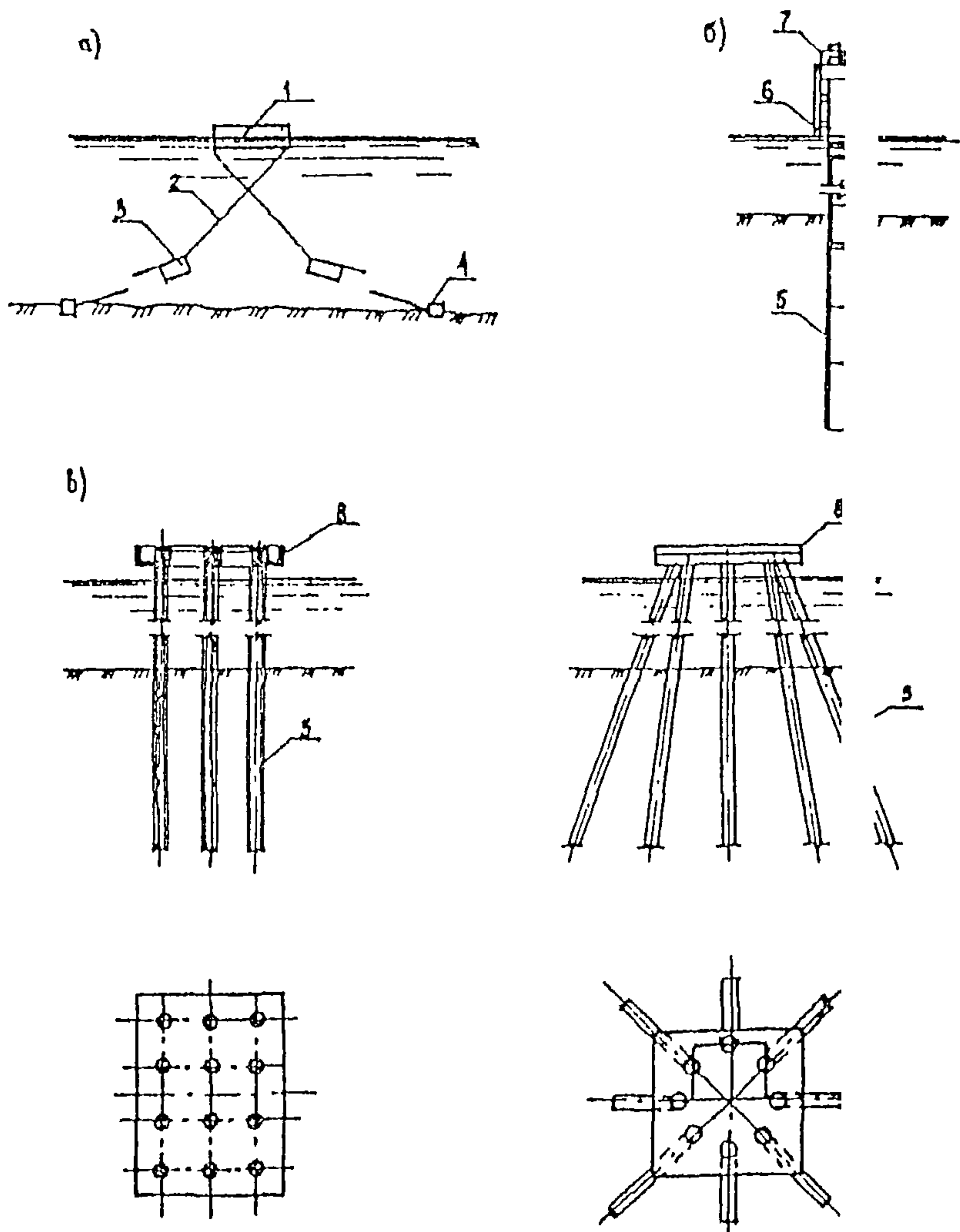
Черт. 2.4. Типы причальных сооружений
