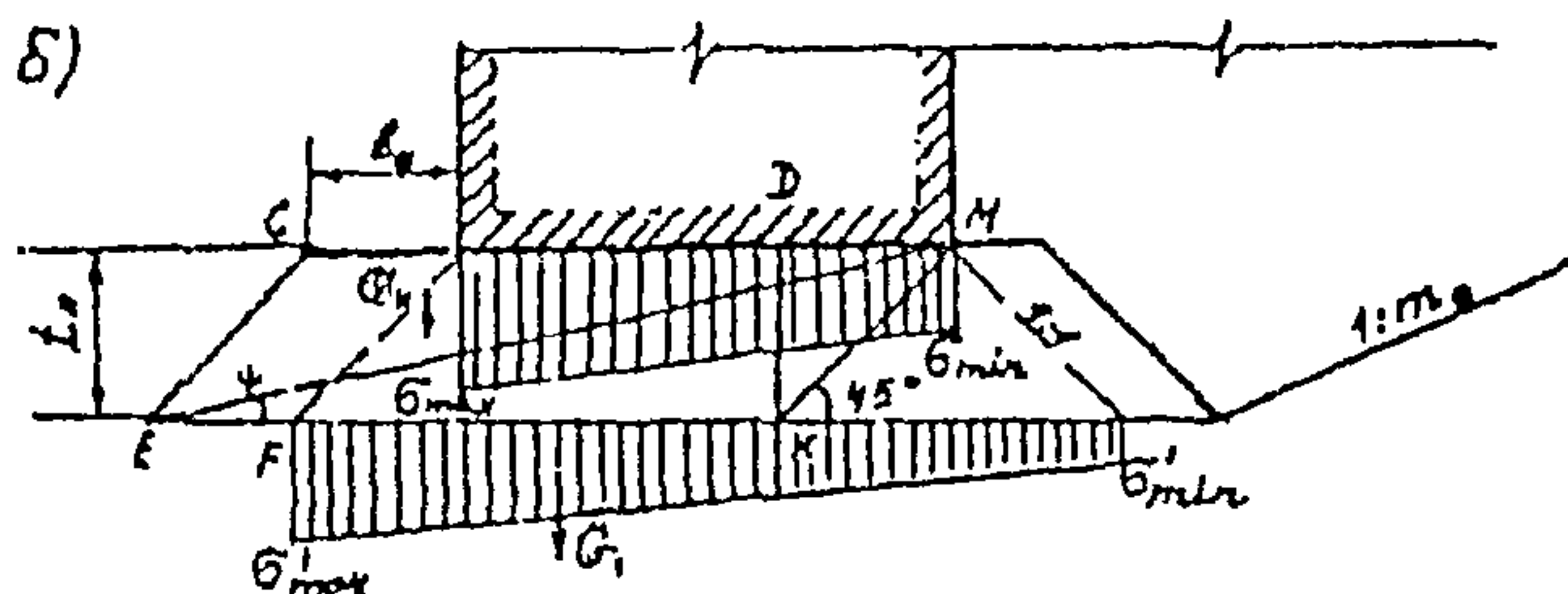
Черт. 7.3. Эпюры краевых напряжений по контакту каменной п стели и основания
