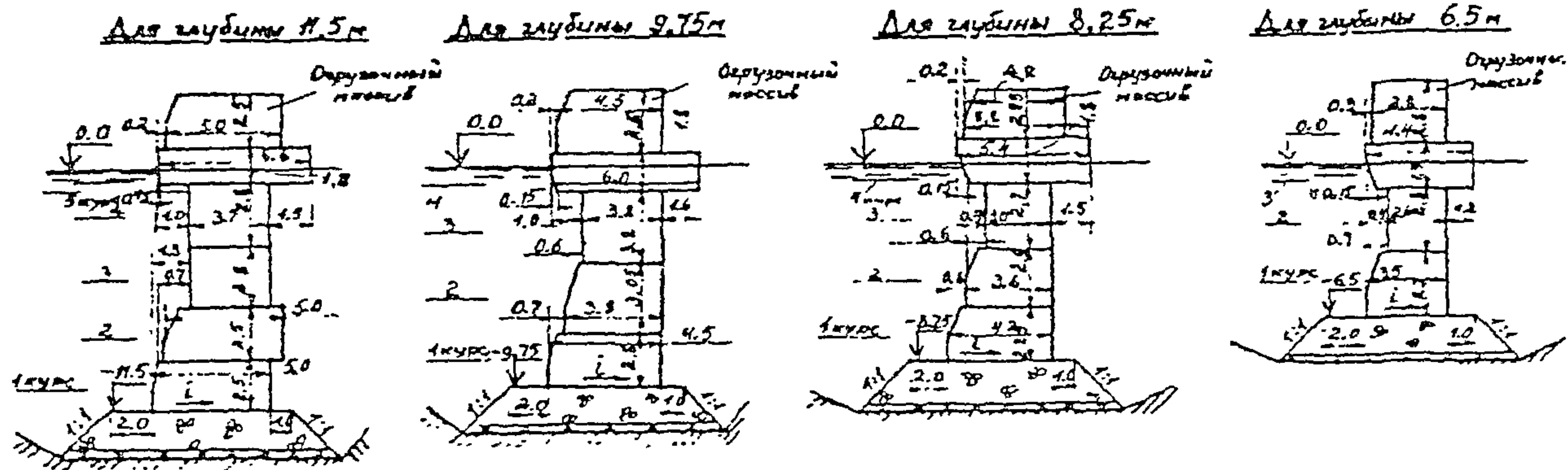
Черт. 1. Схемагрузки постели стенки из кладки обыкновенных массивов весом до 100 т с отметкой кордона +2,80 м и с глубинами у причала с 11,5 до 6,5 м
