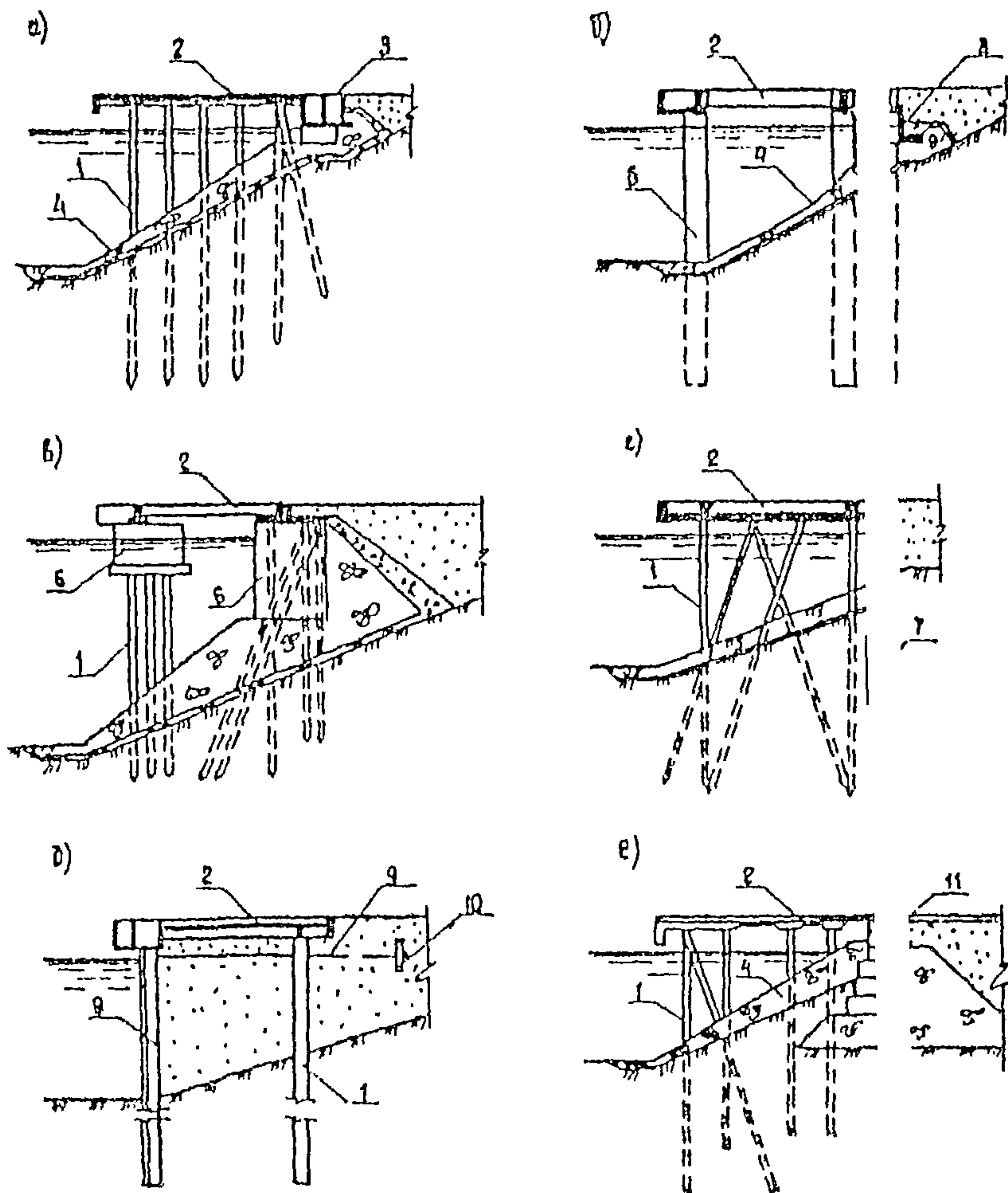
Черт. 2.2. Типы причальных сооружений
