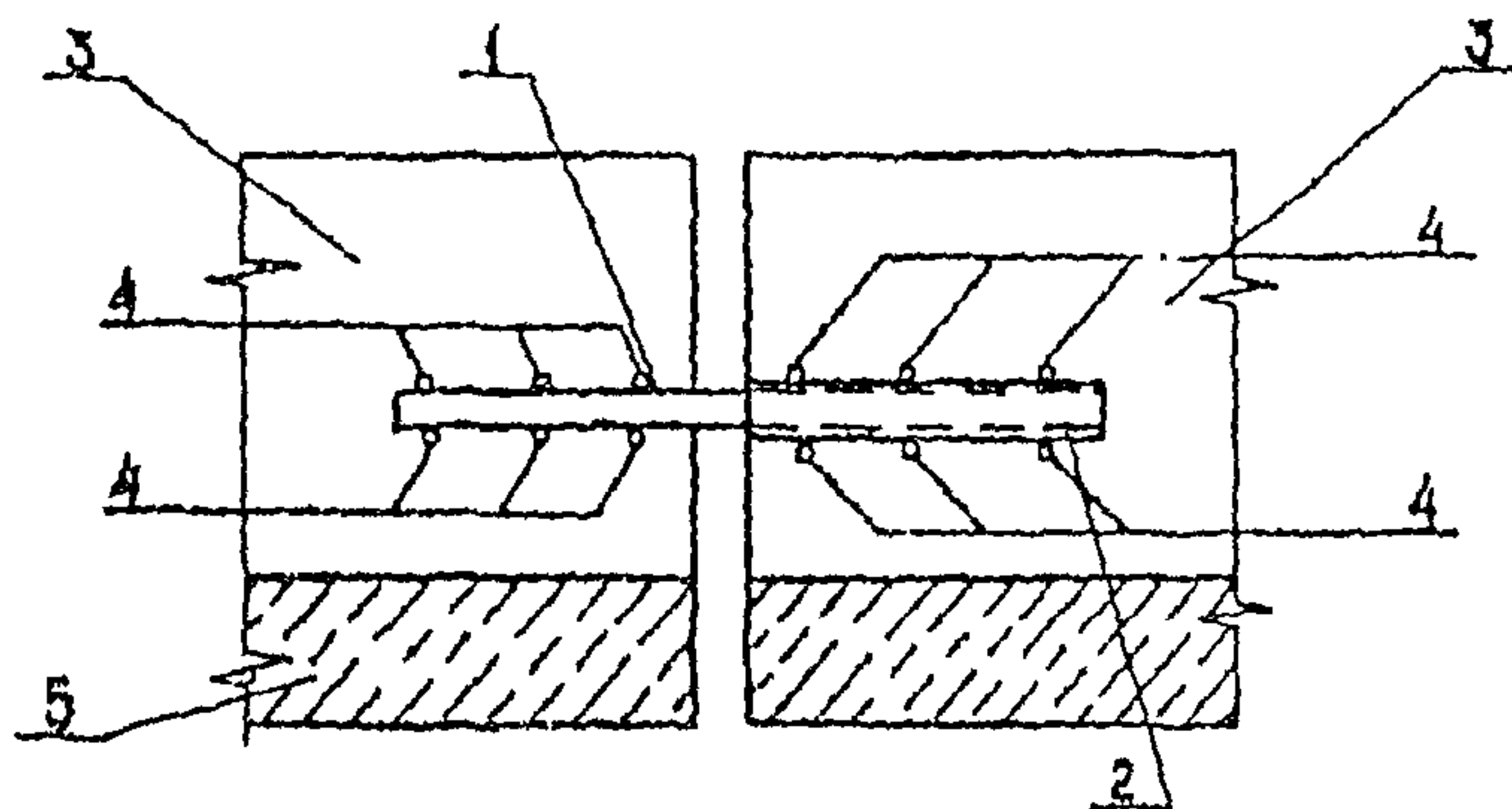
Черт. 14.2. Конструкция связи между секциями причала
