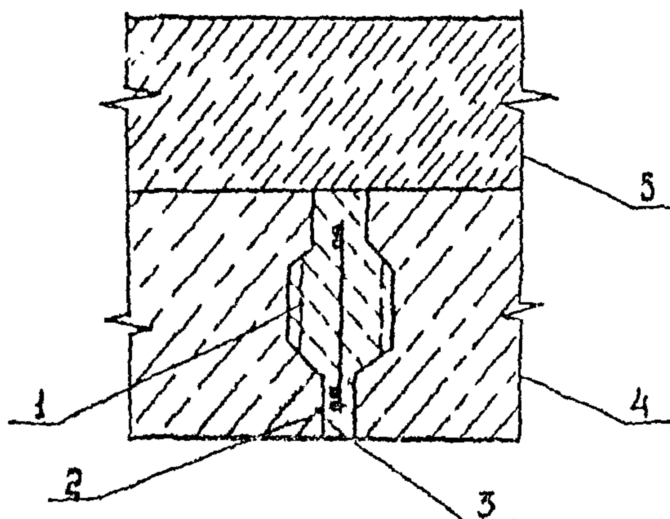
Черт. 14.1. Омоноличивание сборных плит покрытия
