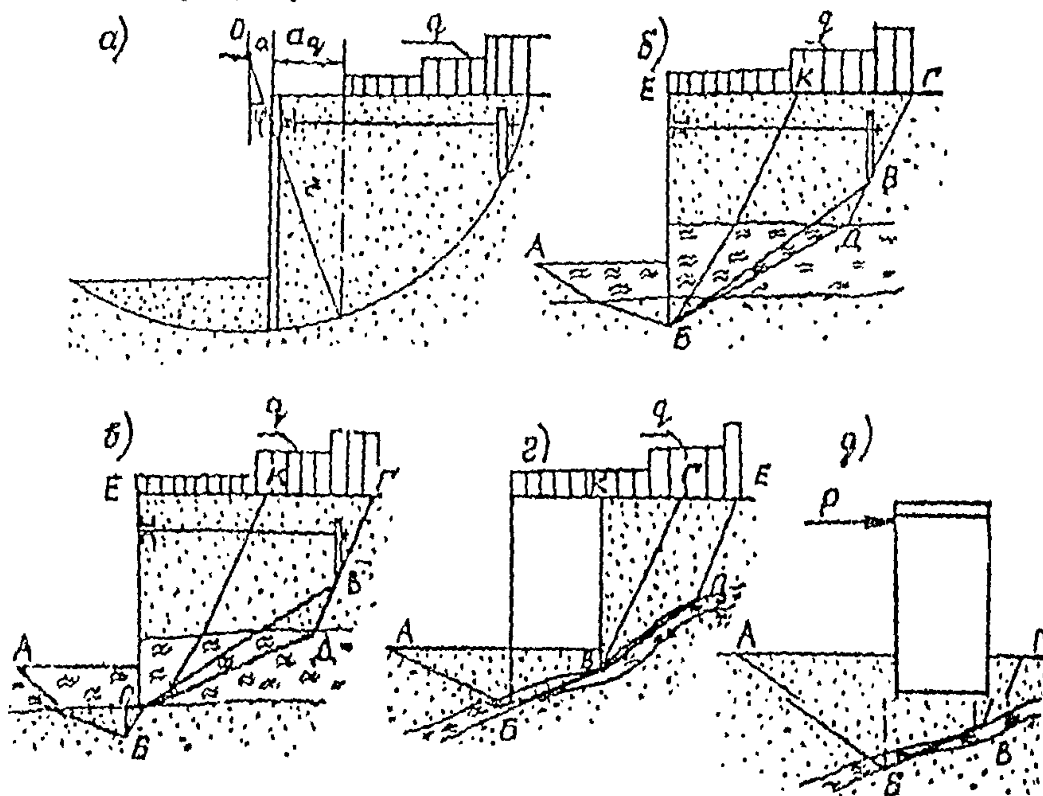
Черт. 6.3. Расположение поверхностей скольжения:
