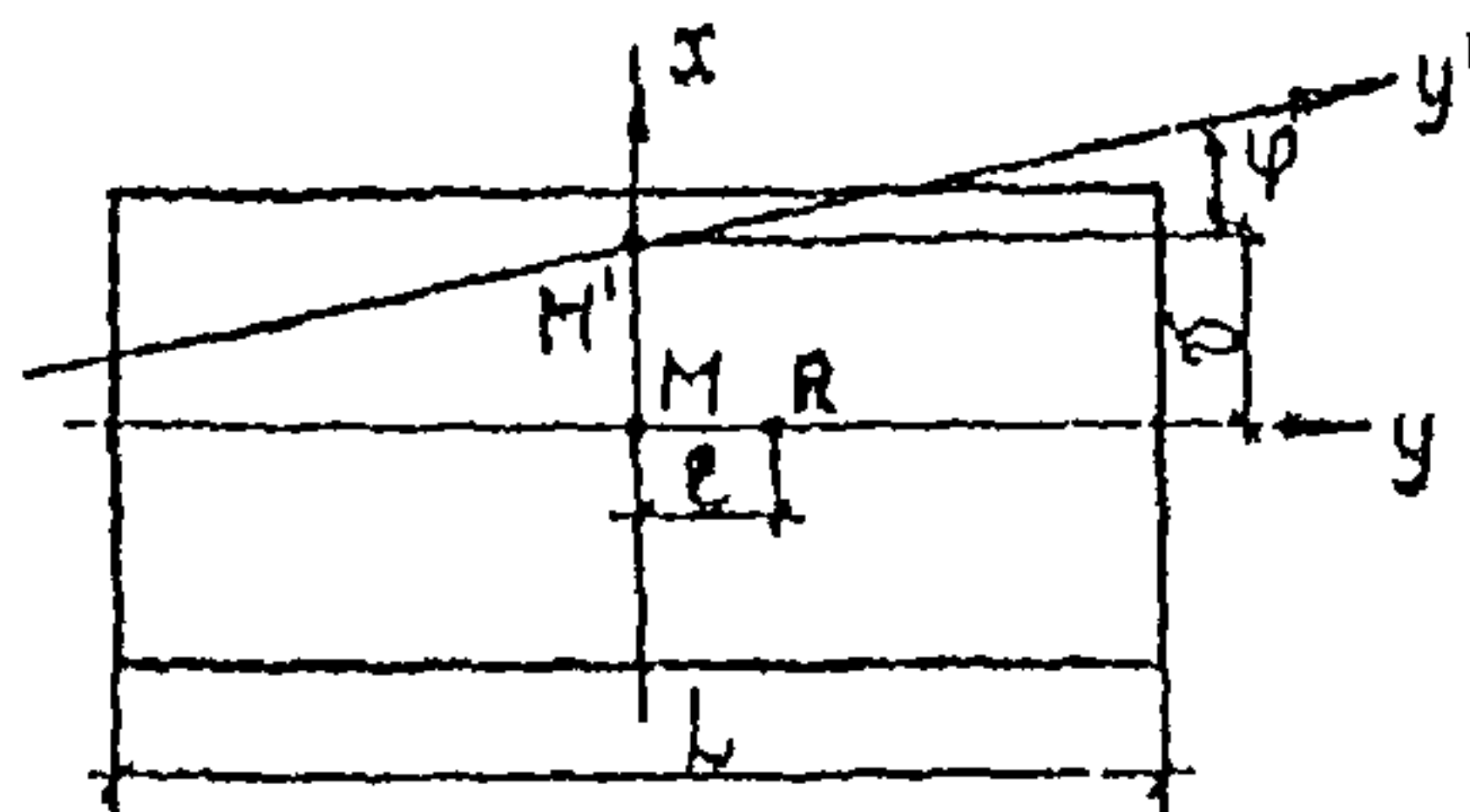
Черт. 9. Схема перемещений жесткой плиты ростверка
