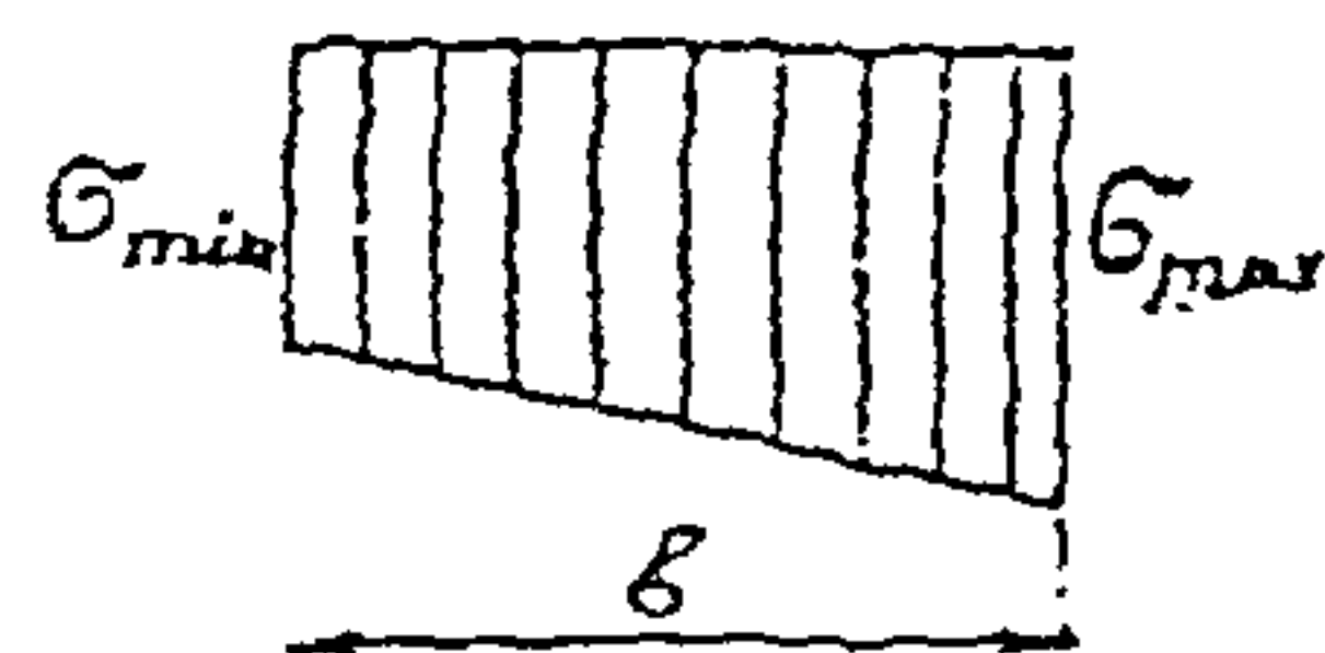
Эпюра напряжений по постели
