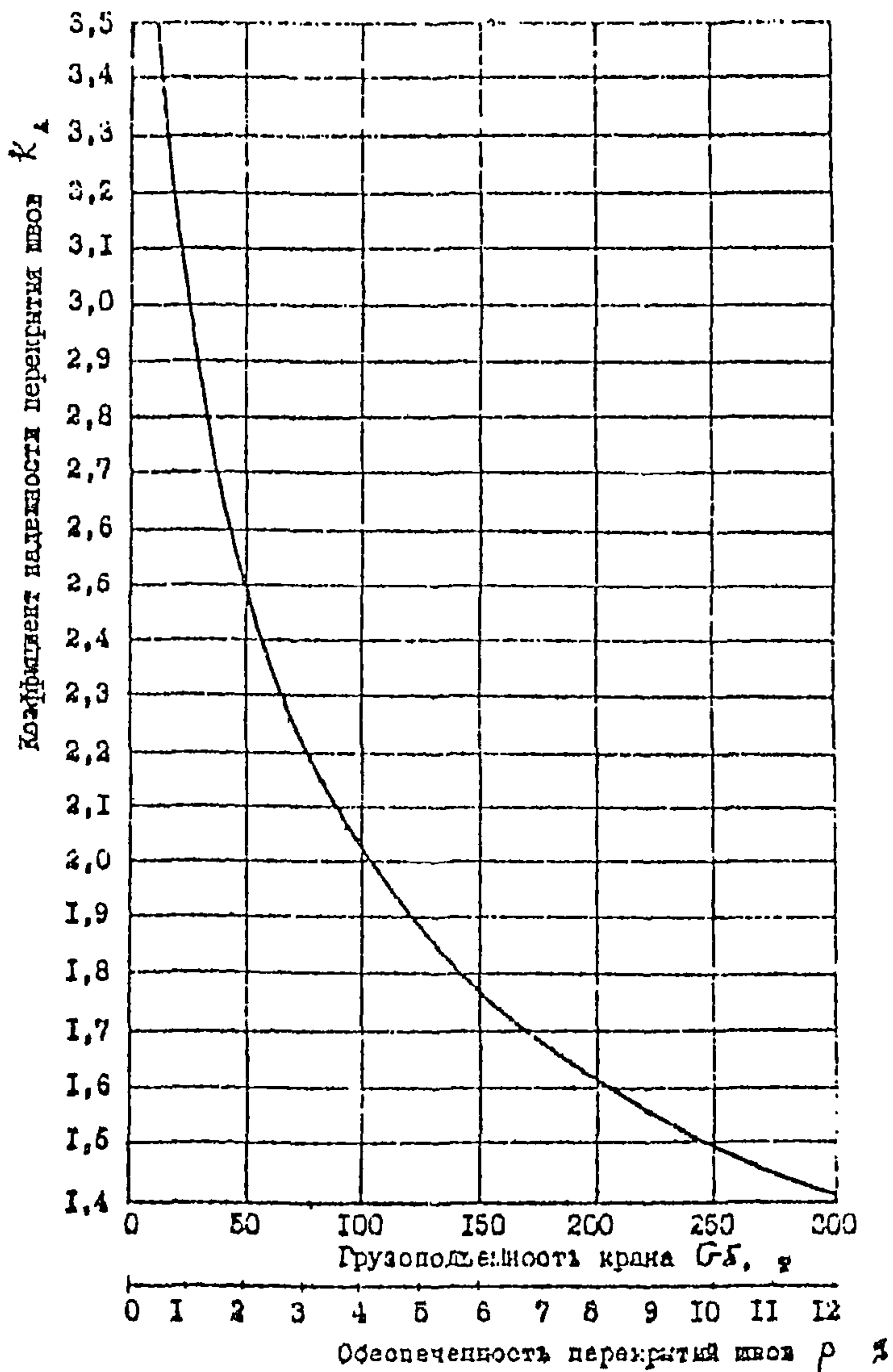
Черт. 2. График зависимости коэффициента надежности перекрытия швов k_d от грузоподъемности крана G_k
