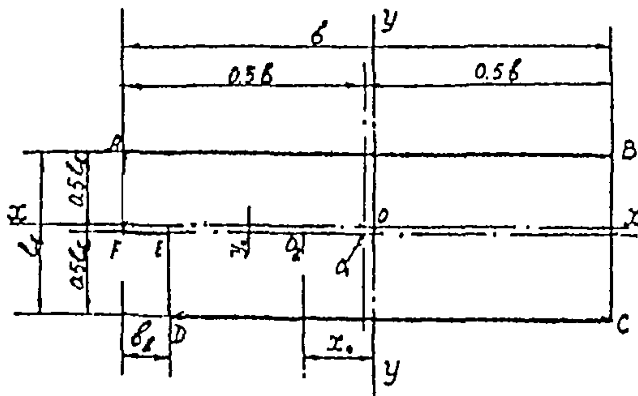
Черт. 7.9. Схема расчета фундаментной плиты с учетом неполноты контакта с основанием
