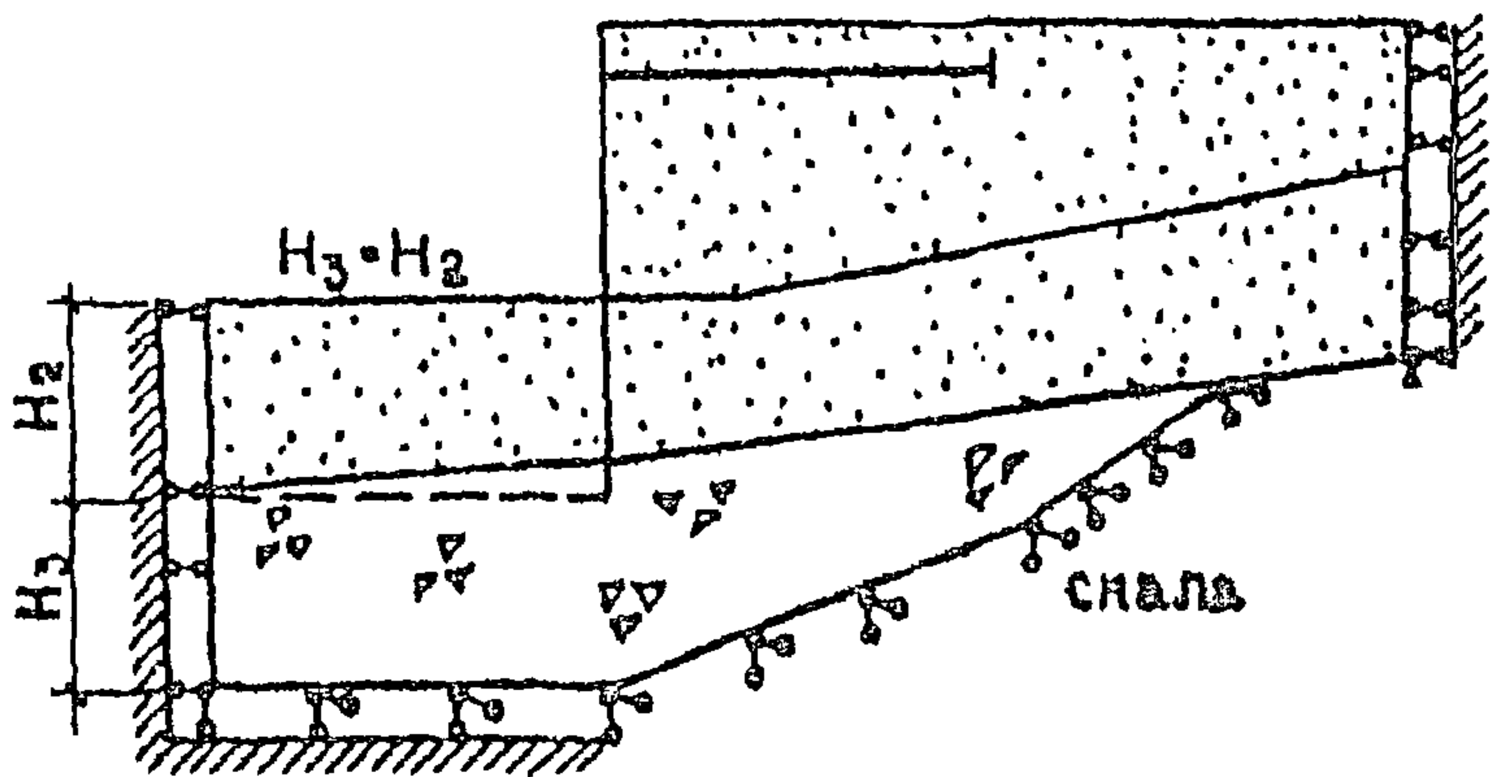
Черт. 2. Пример расчетной схемы на скальном основании
