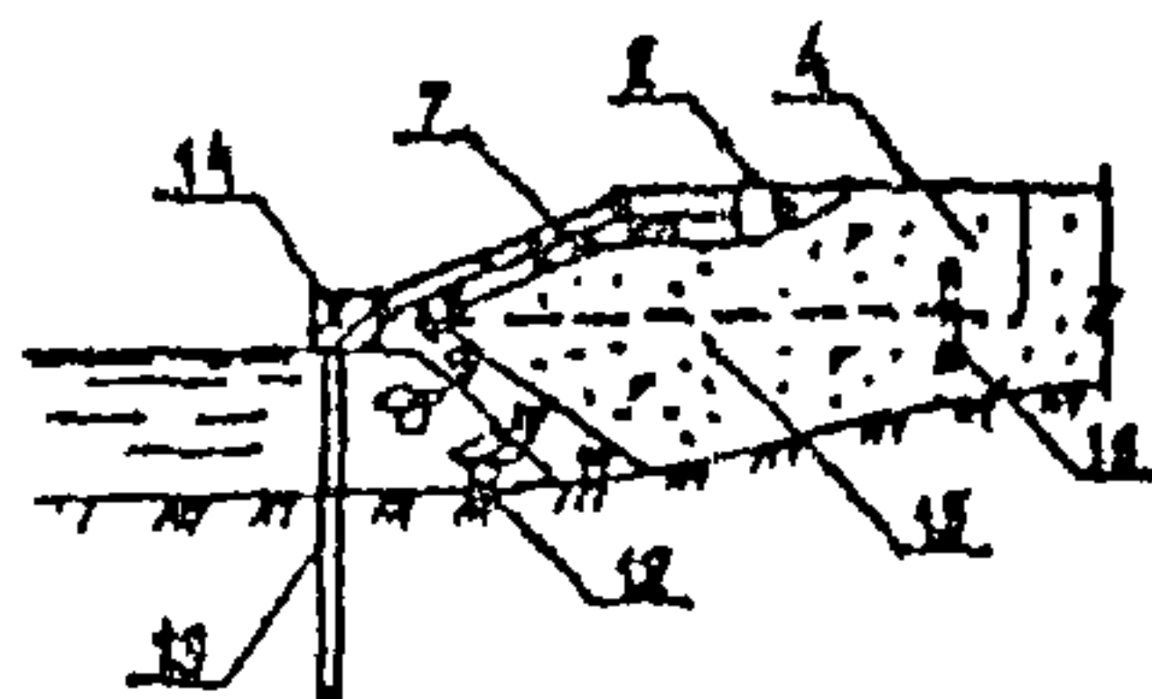
Черт. 13.1. Типы берегоукрепительных сооружений
