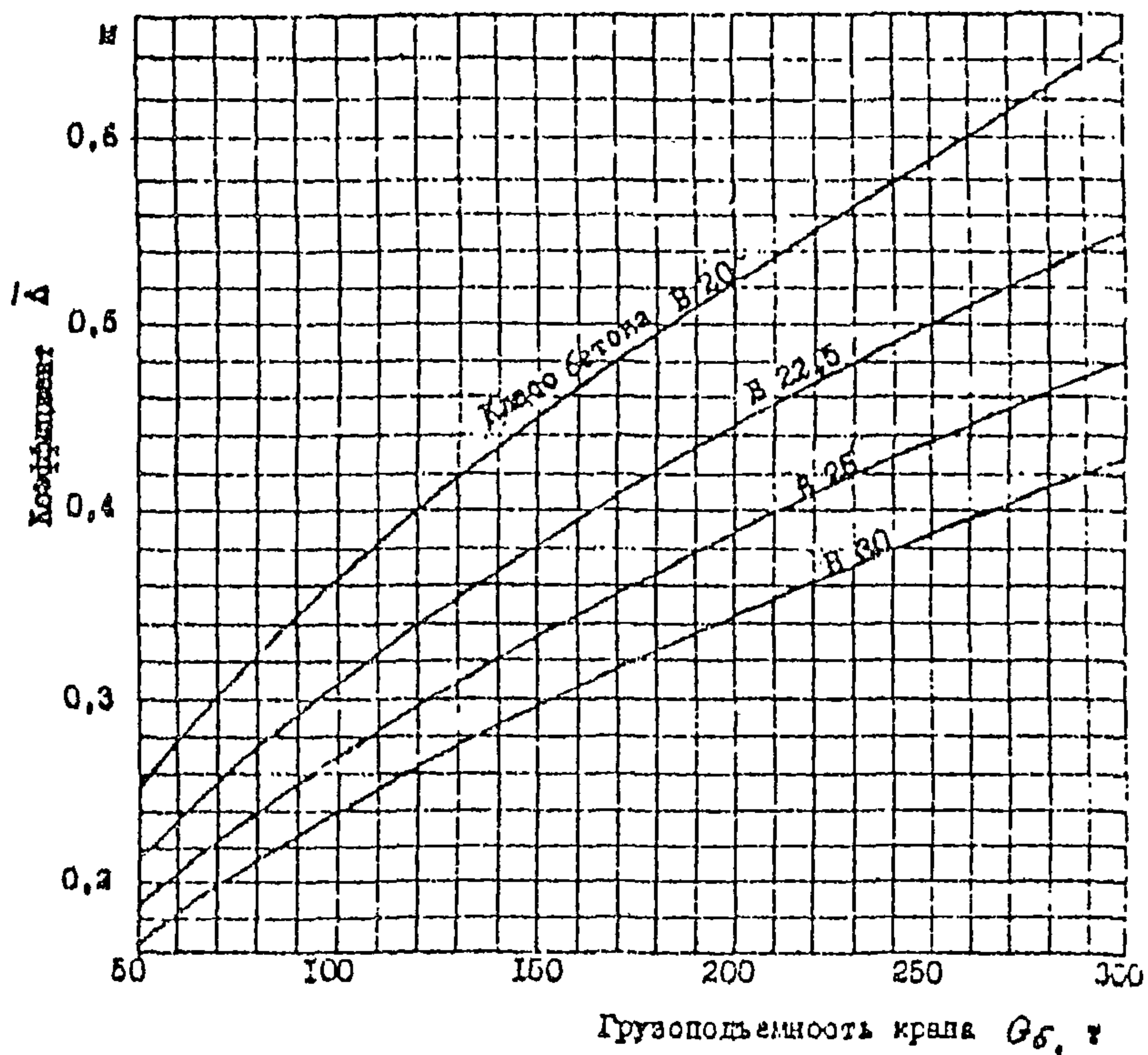
Черт. 1. Графики зависимости параметра \Delta от класса бетона и грузоподъемности крана G_{\delta}
