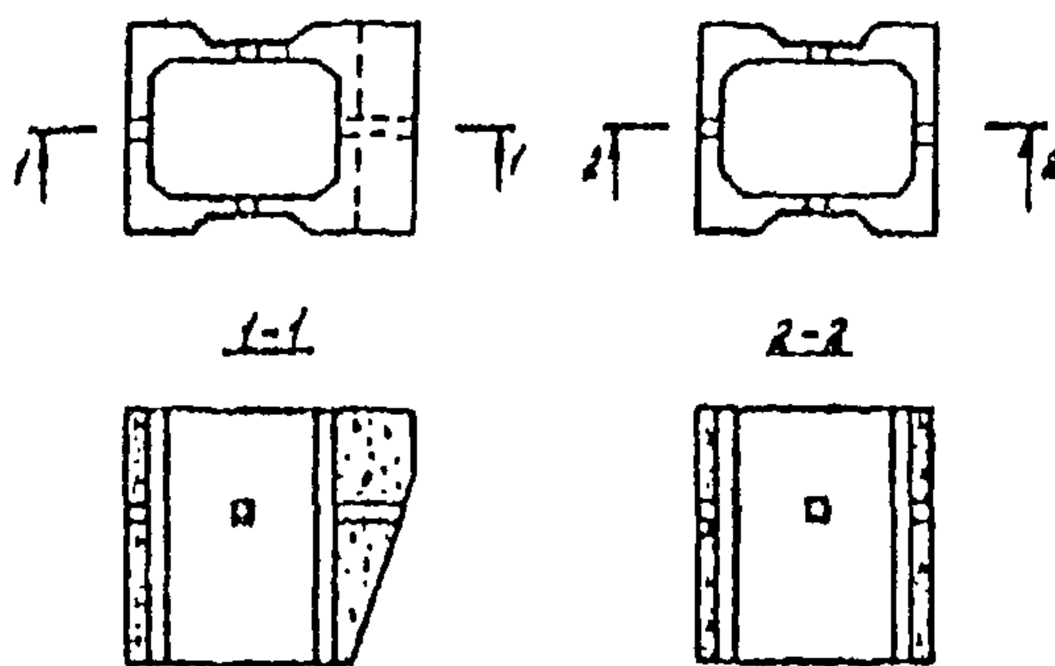
Черт. 7.1. Типы пустотелых массивов
