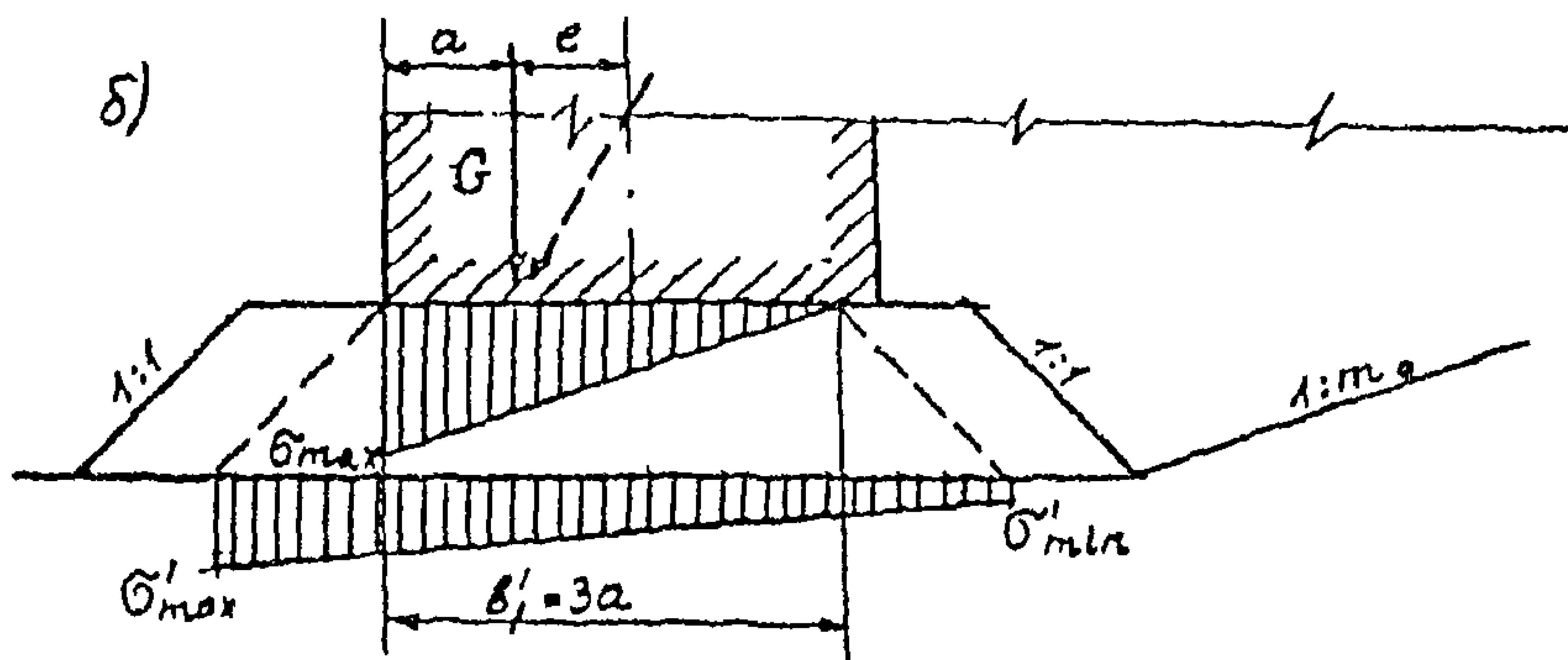
Черт. 7.2.Эпюры краевых напряжений по контакту основания сооружения и каменной постели
