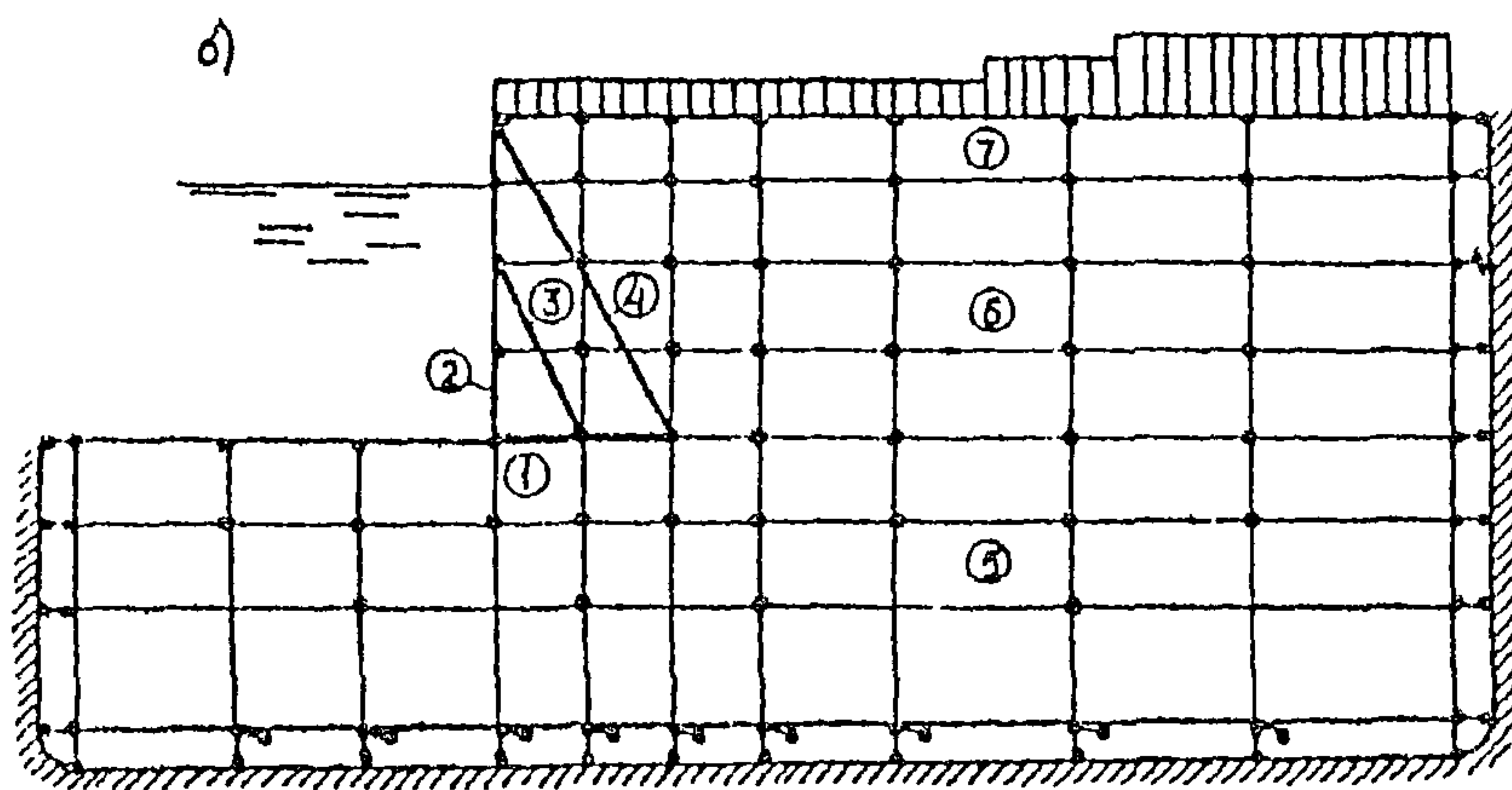
Черт. 4. Динамическая расчетная схема стенки углового типа с контрфорсом
