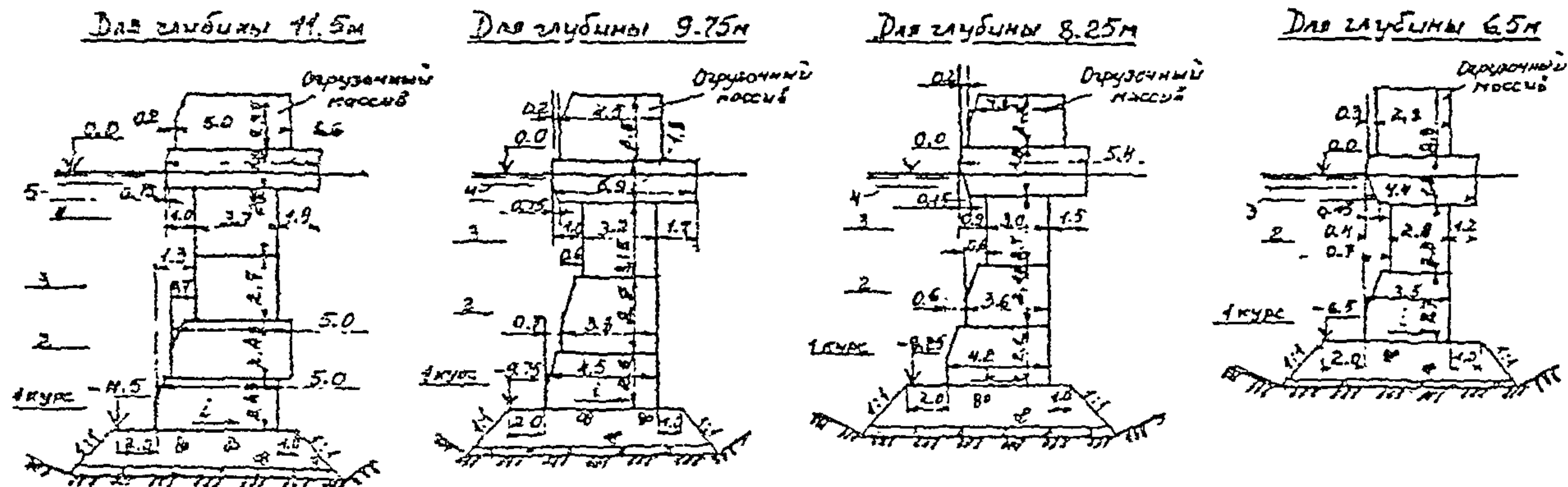
Черт. 2. Схема огрузки постели стенки из кладки обыкновенных массивов весом до 100 т с отметкой кордона +2,50 м и с глубинами у причала с 11,5 до 6,5 м
