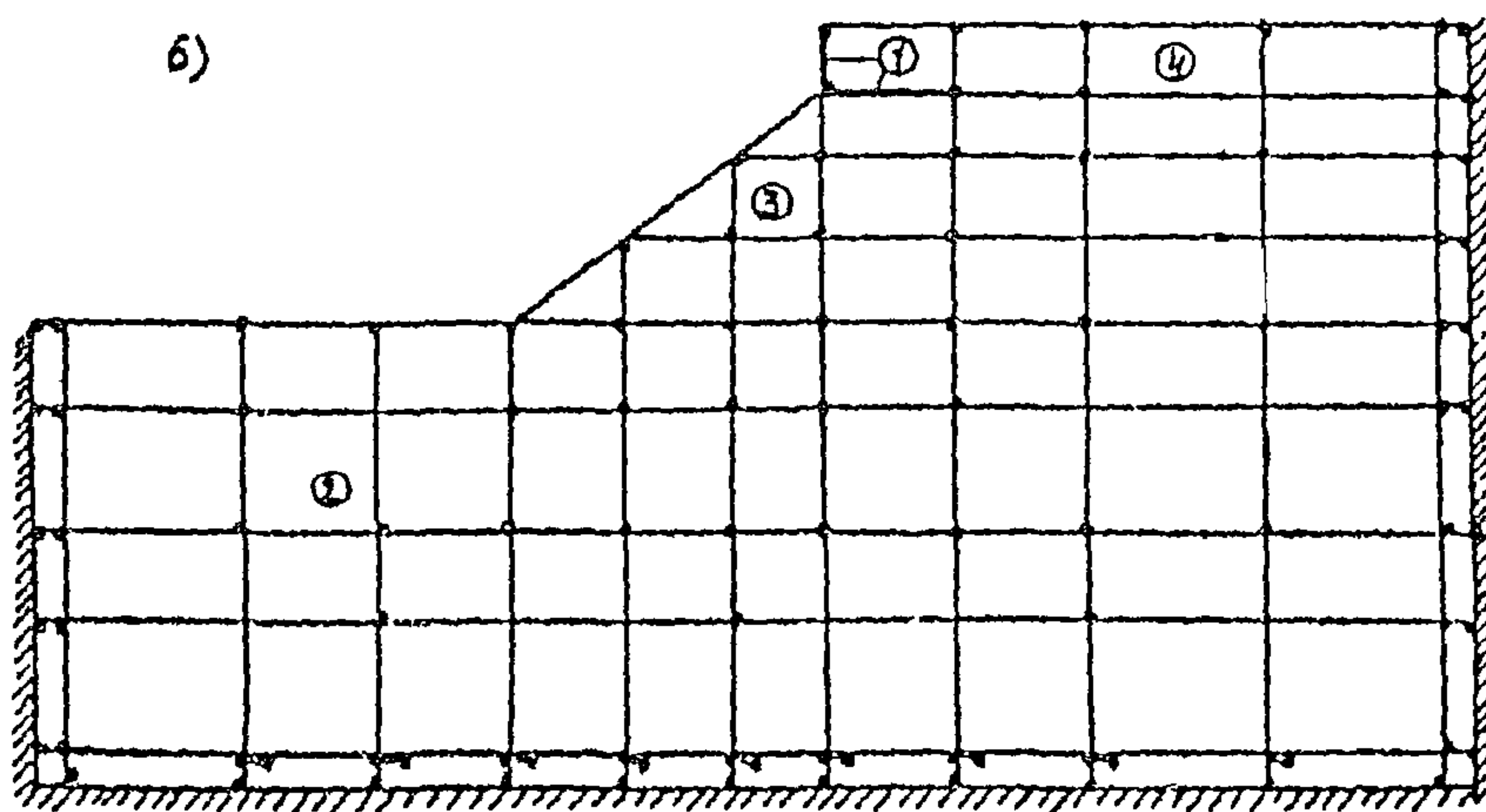
Черт. 11. Динамическая расчетная схема подпричального откоса набережной
