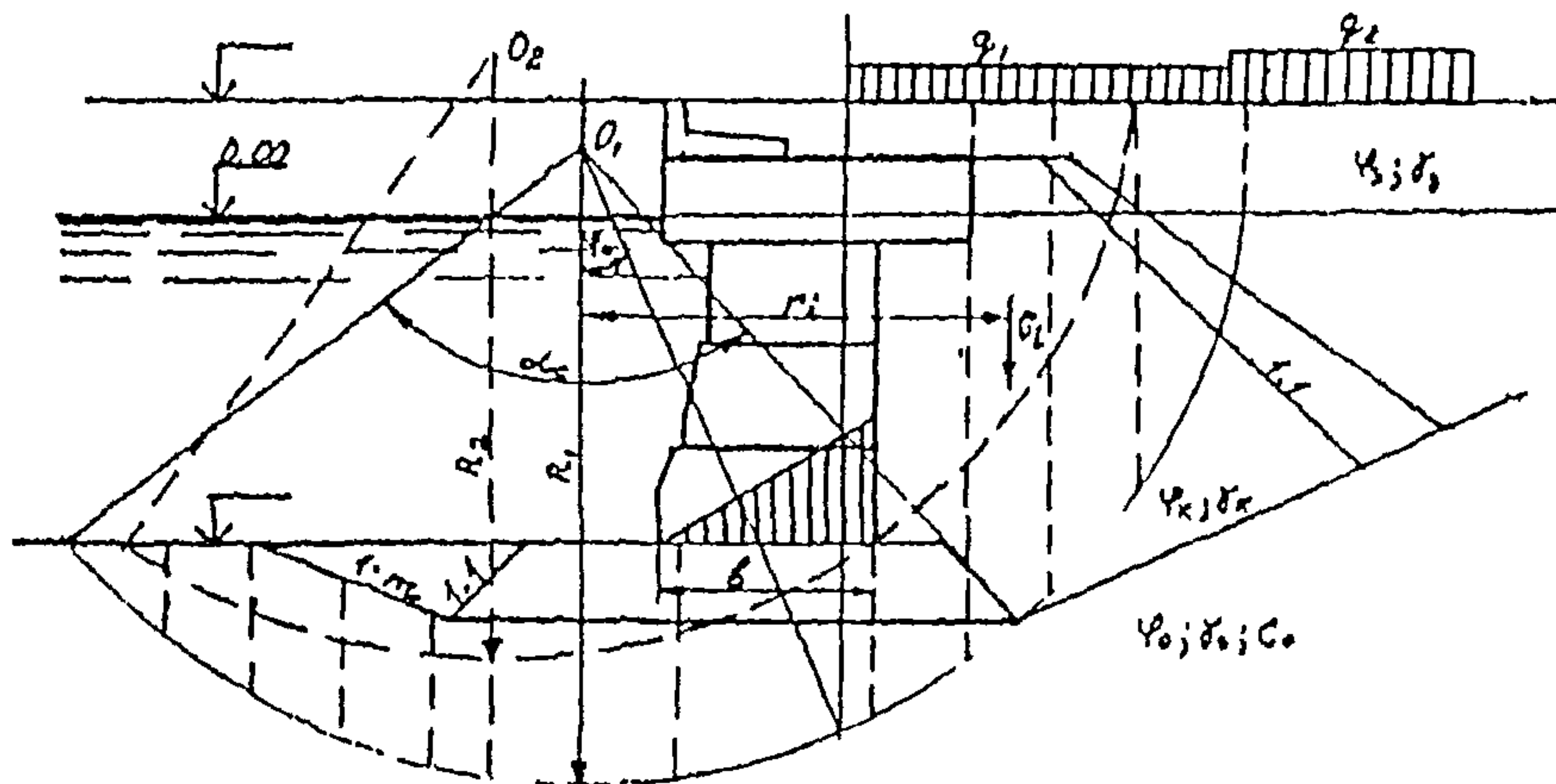
Черт. 7.5. Схема расположения эксплуатационных нагрузок
