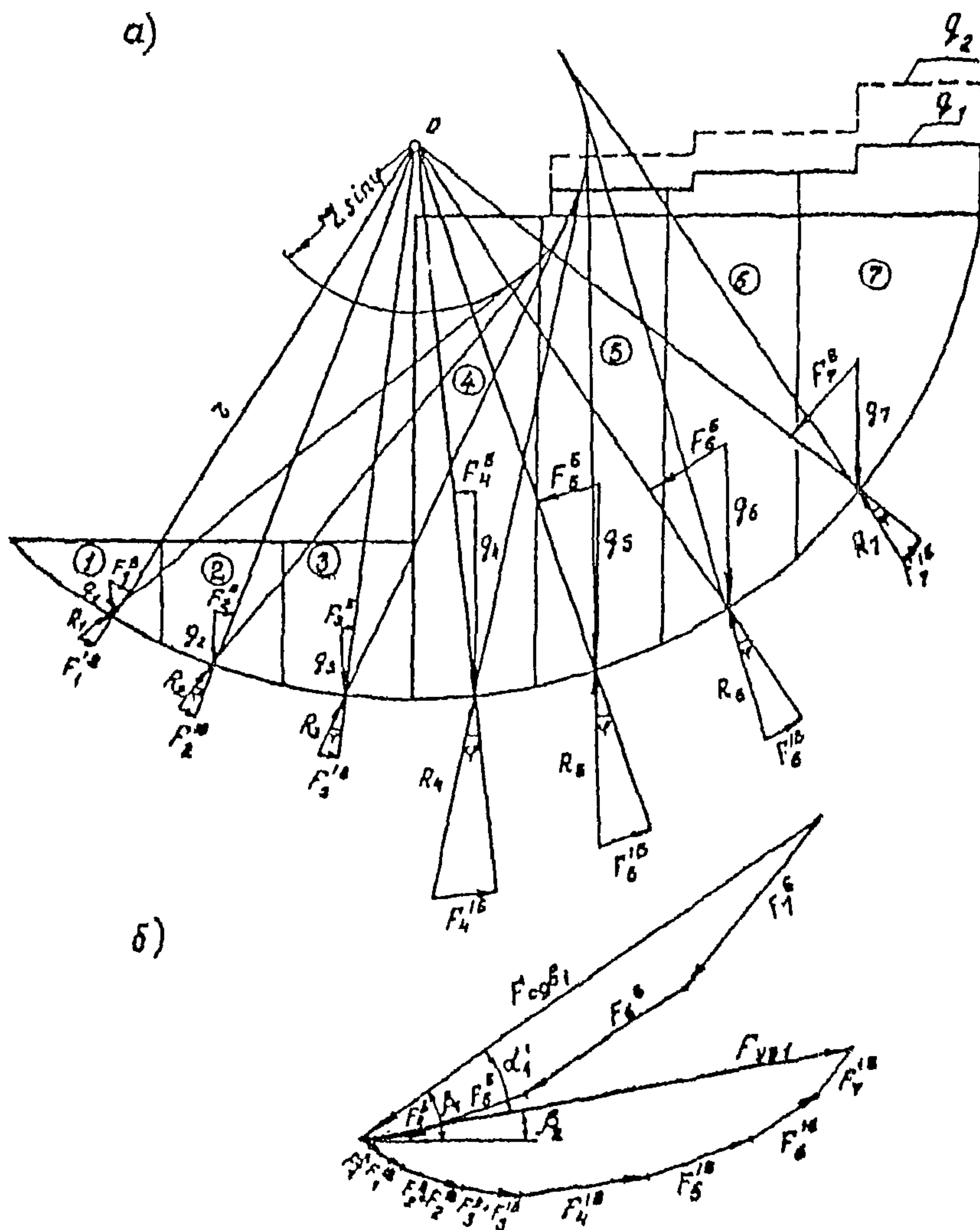
Черт. 6.1. Графическое выполнение расчета а - расчетная схема; б - силовые многоугольники
