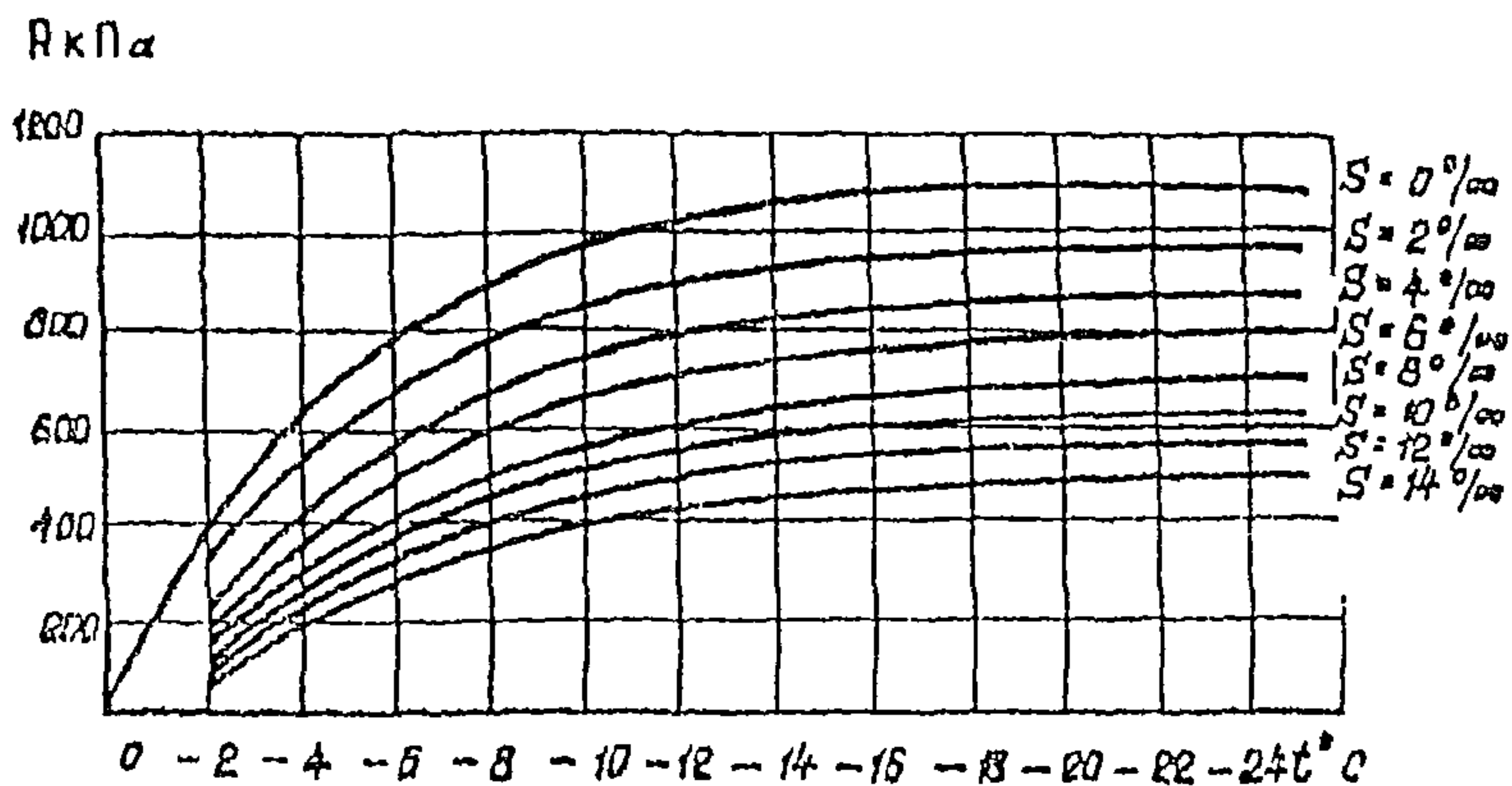
Черт. 3 Зависимость прочности льда на срез от его температуры и солености
