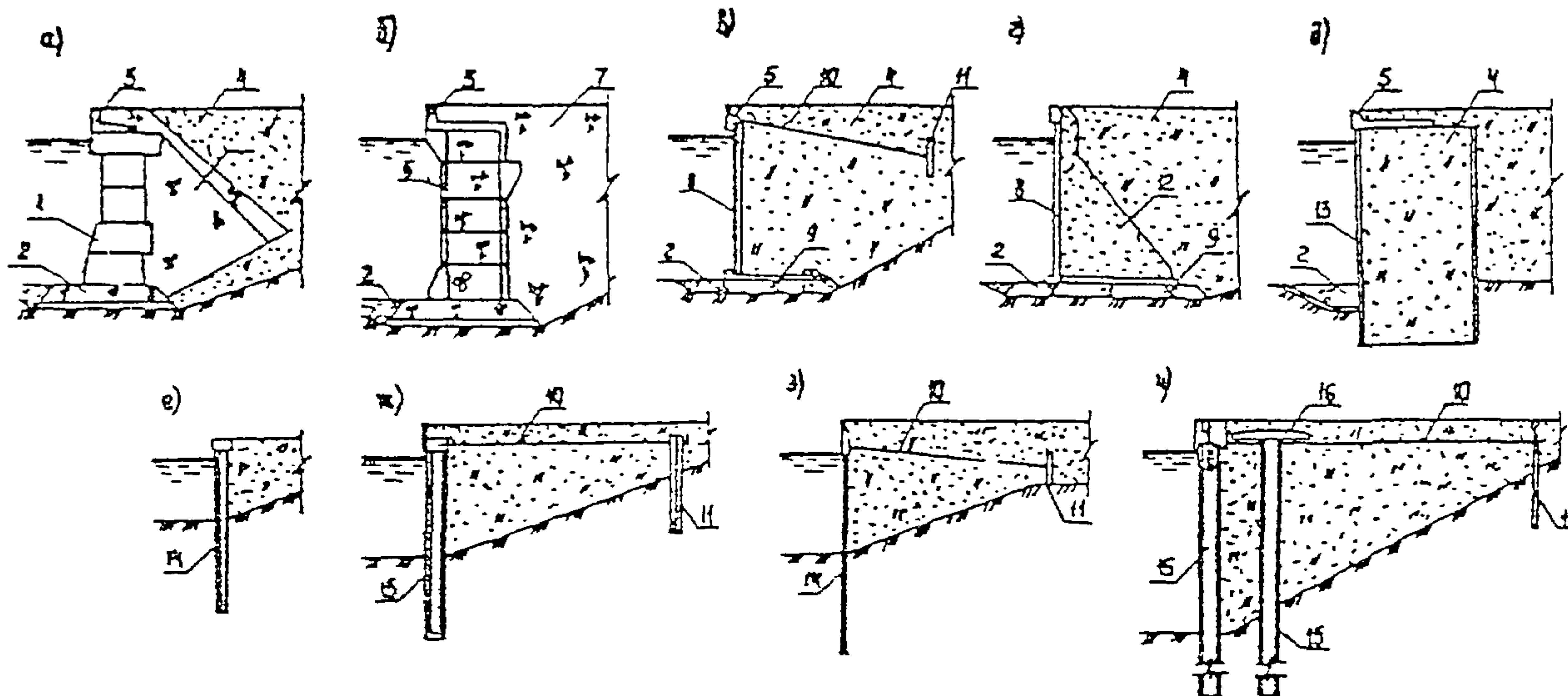
Черт. 2.1. Типы причальных сооружений
