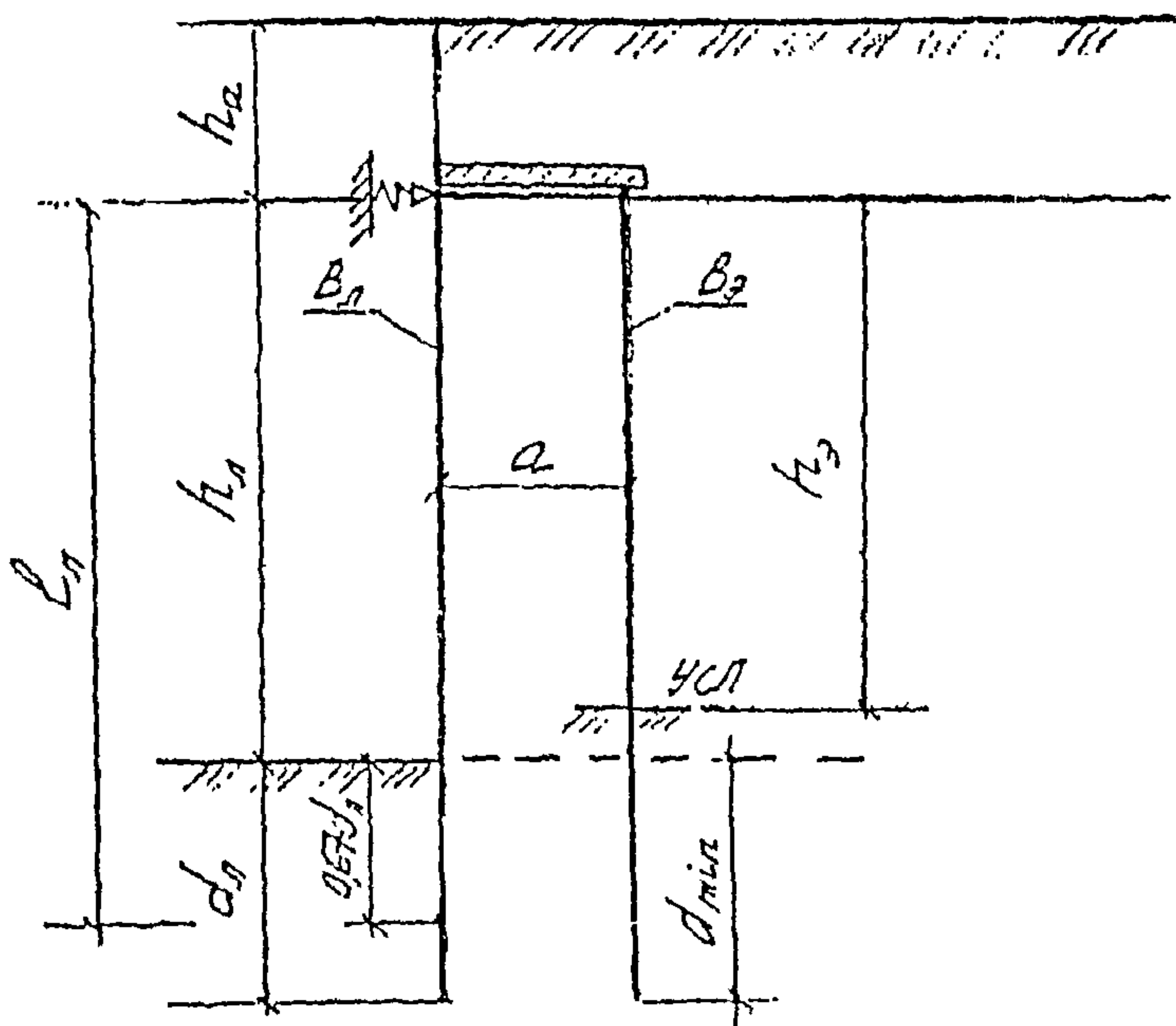
Черт. 8.2. Схема к определению положения уровня УСП.
