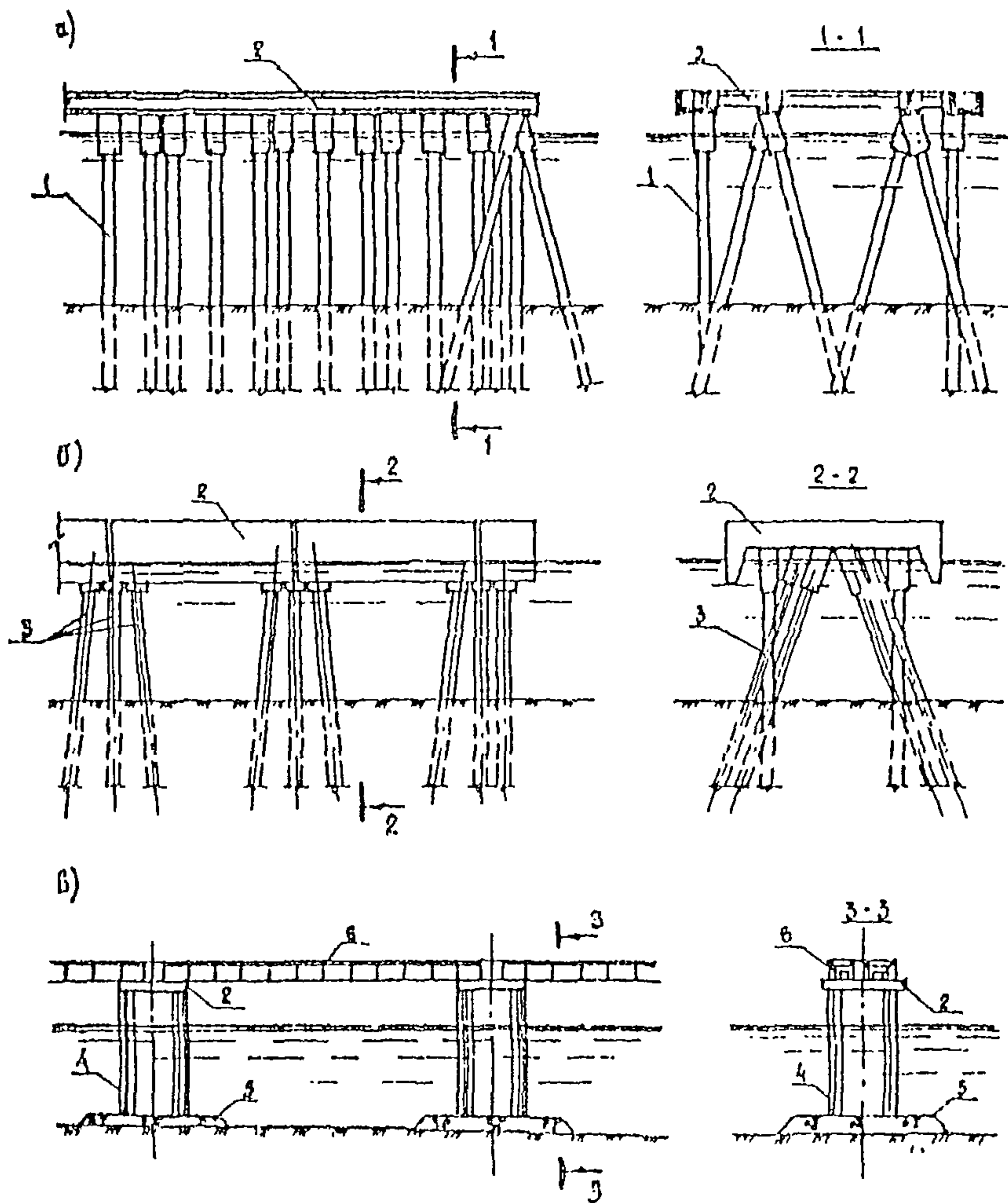
Черт. 2.3. Типы причальных сооружений
