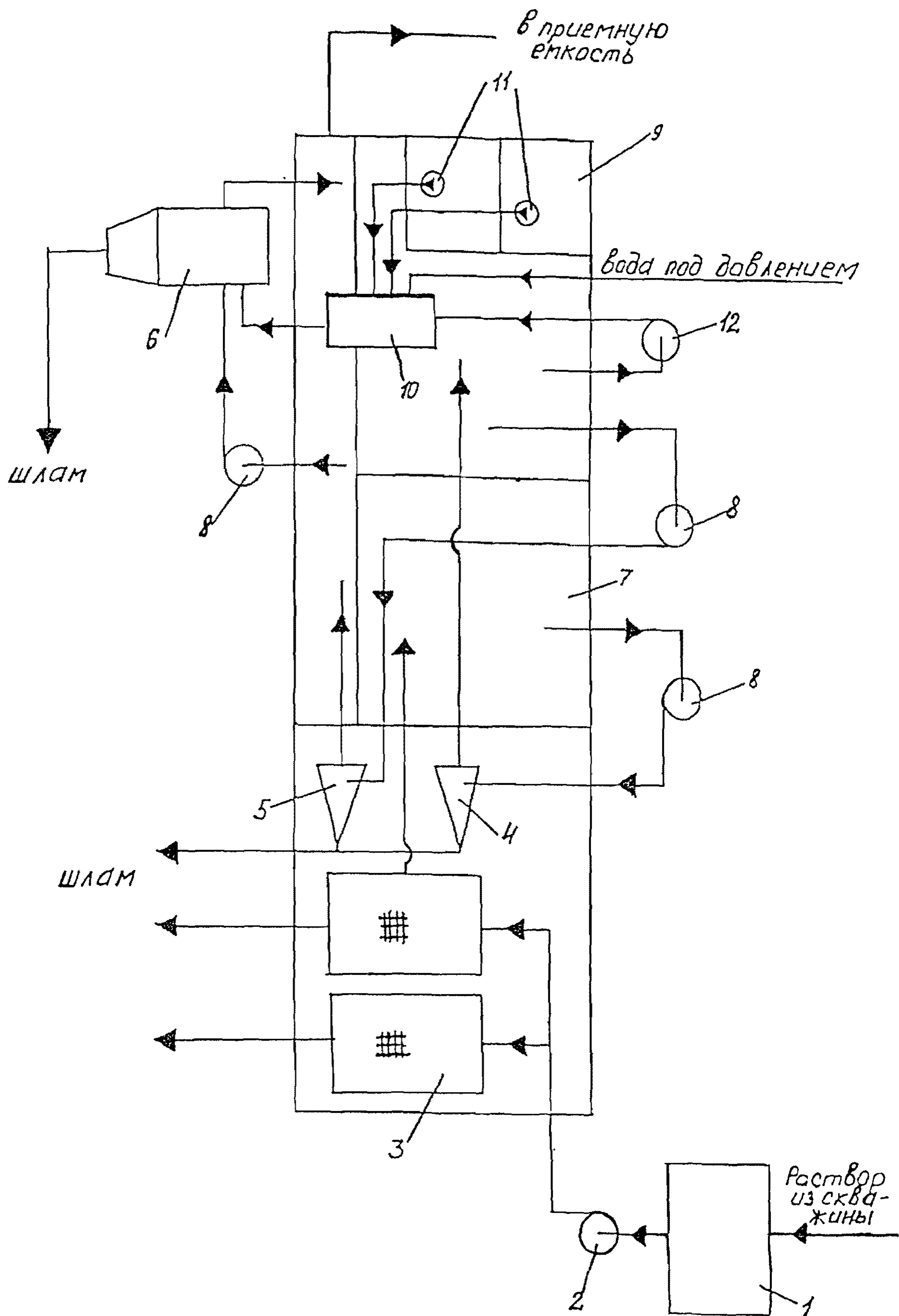
Рис.2 Технологическая схема блока очистки бурового раствора
