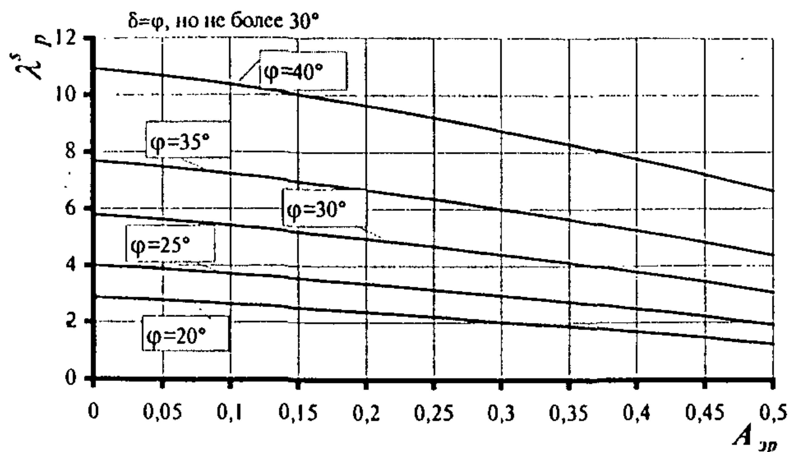
Рис.Д.2 – График зависимости коэффициента горизонтальной составляющей пассивного остаточного давления \lambda_p^s от эффективного коэффициента сейсмичности A_{эп}
