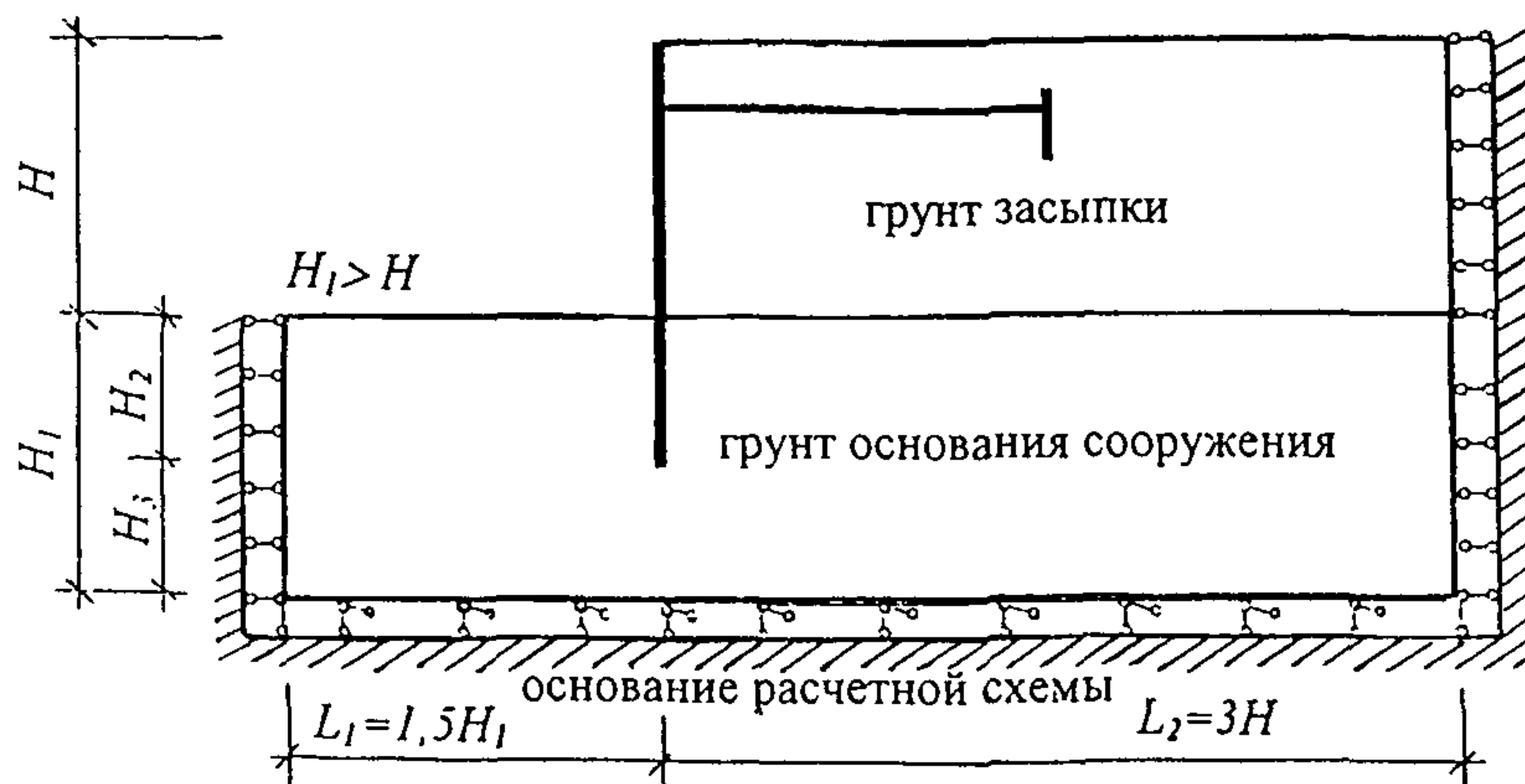
Рисунок 5.1 - Положение границ и граничные условия в расчетной схеме больверка
