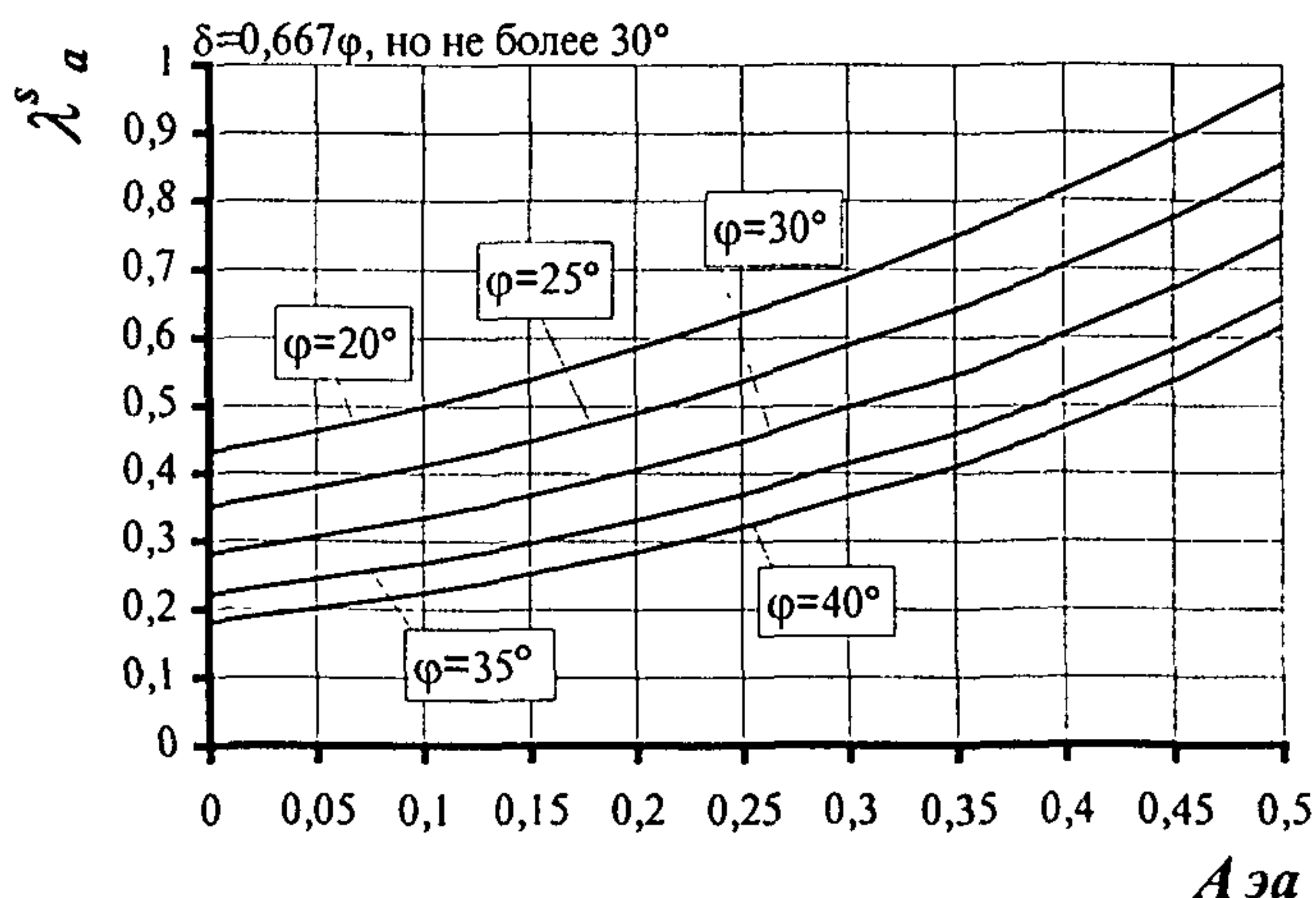
Рис.Д.1 – График зависимости коэффициента горизонтальной составляющей активного остаточного давления \lambda^s_a от эффективного коэффициента сейсмичности A_{эа}
