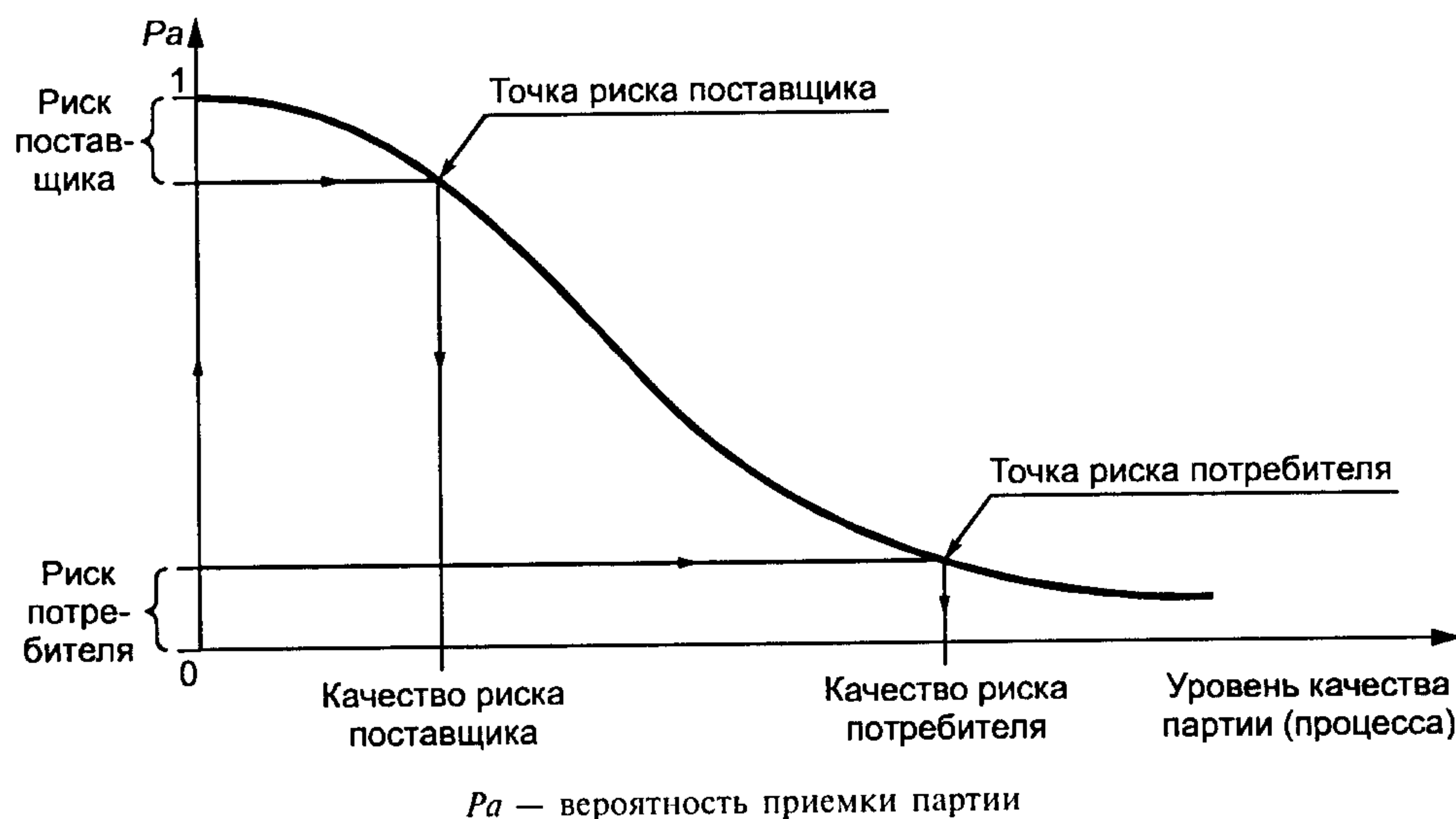
Рисунок 1 — Кривая оперативной характеристики для качества риска потребителя и риска поставщика
