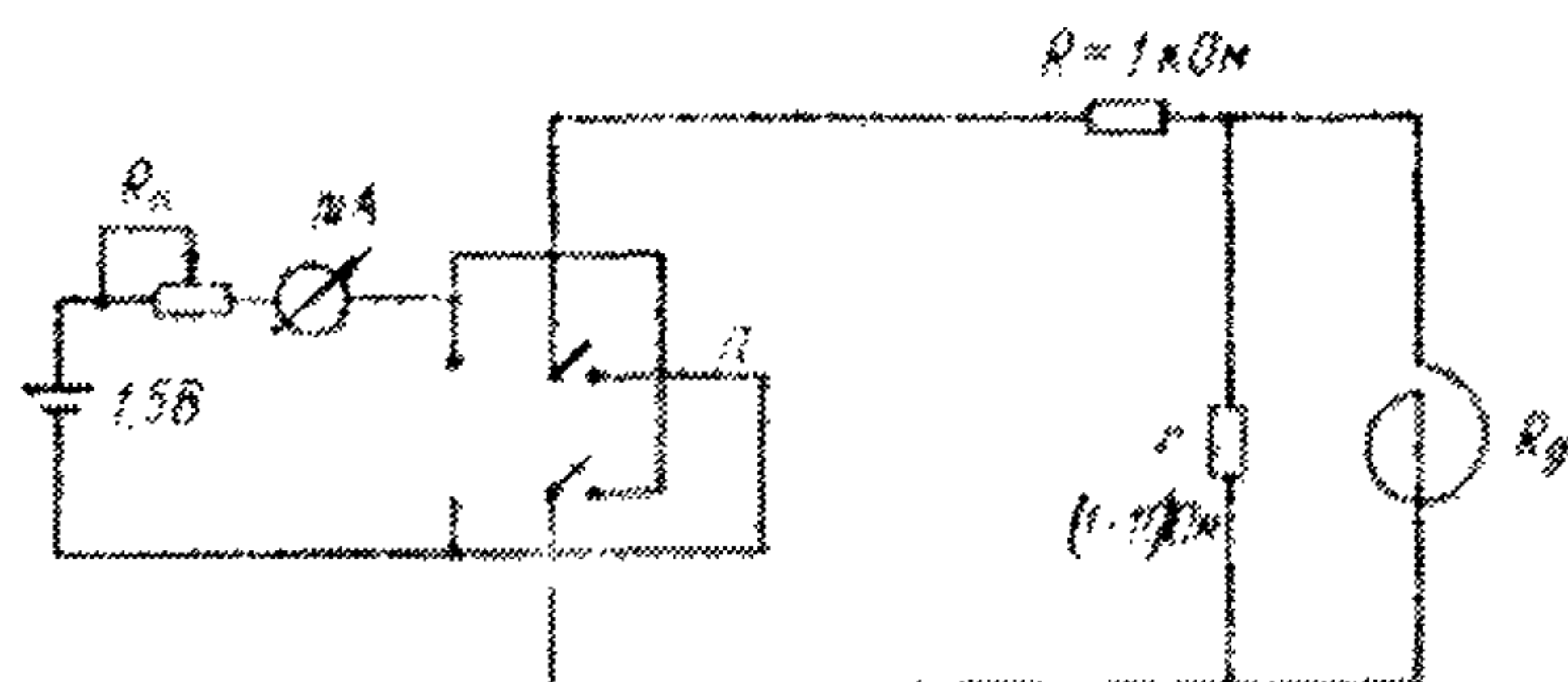
Рис. 17. Электрическая схема для определения чувствительности гальванометра
