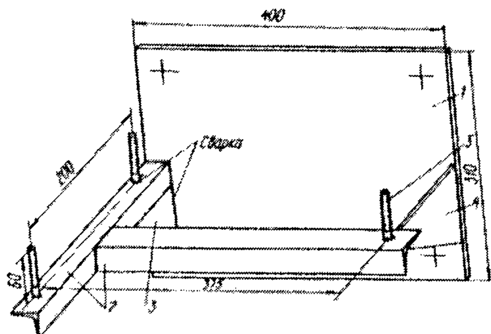
Рис.14. Переходный кронштейн для крепления С-5-С к стене
