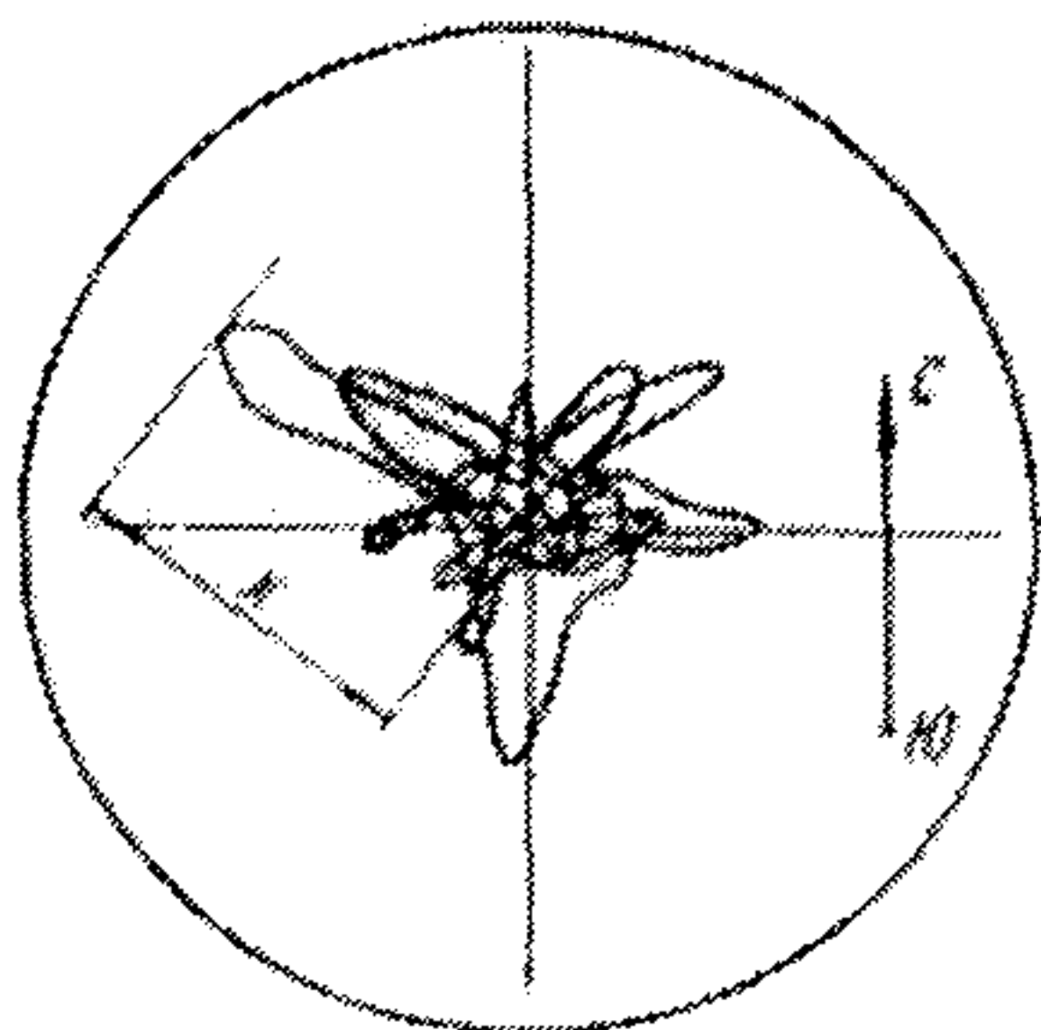
Рис.11. Пример определения максимального смещения по записи сейсмокопиров СБМ
