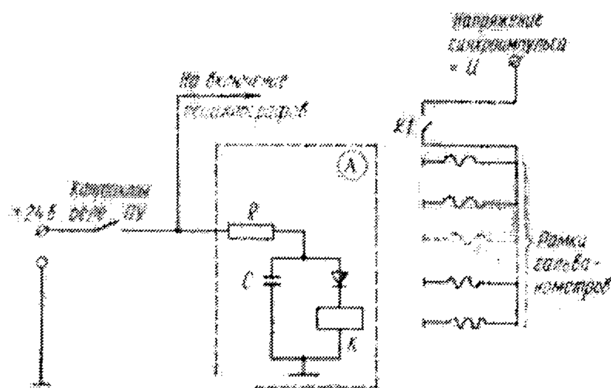
Рис.5. Схема выработки синхронимпульса по всем каналам ИСС (Блок А рассчитывается из условия выработки временного импульса через \sim 0,2 с после включения осциллографов)
