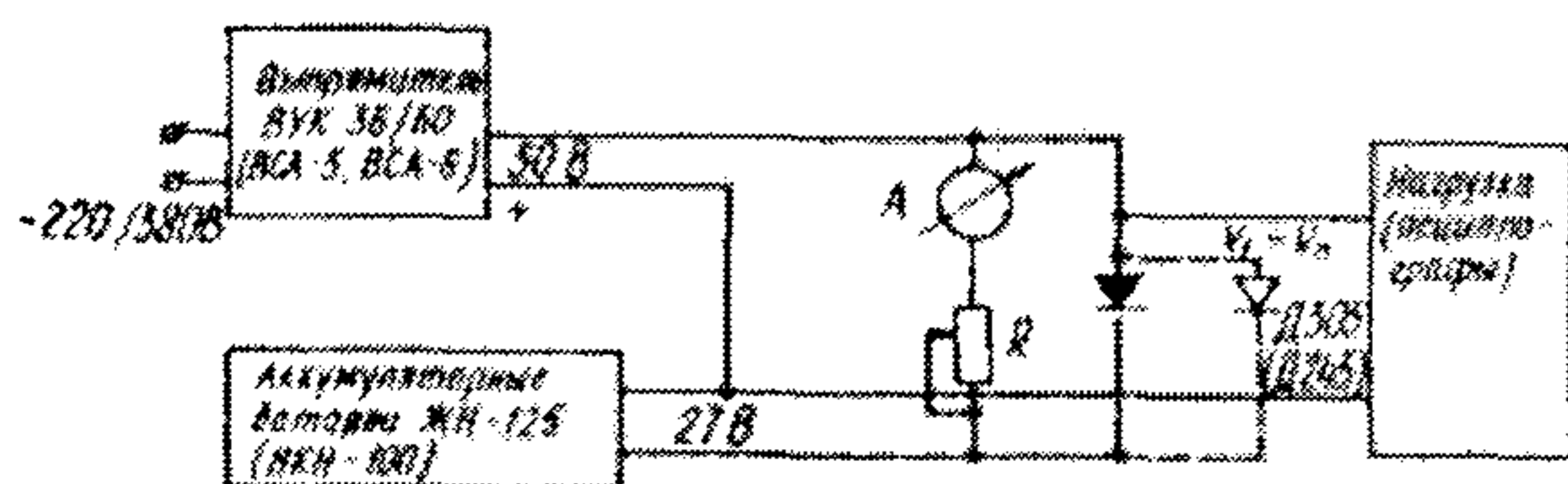
Рис.10. Схема блока питания станции ИСС
