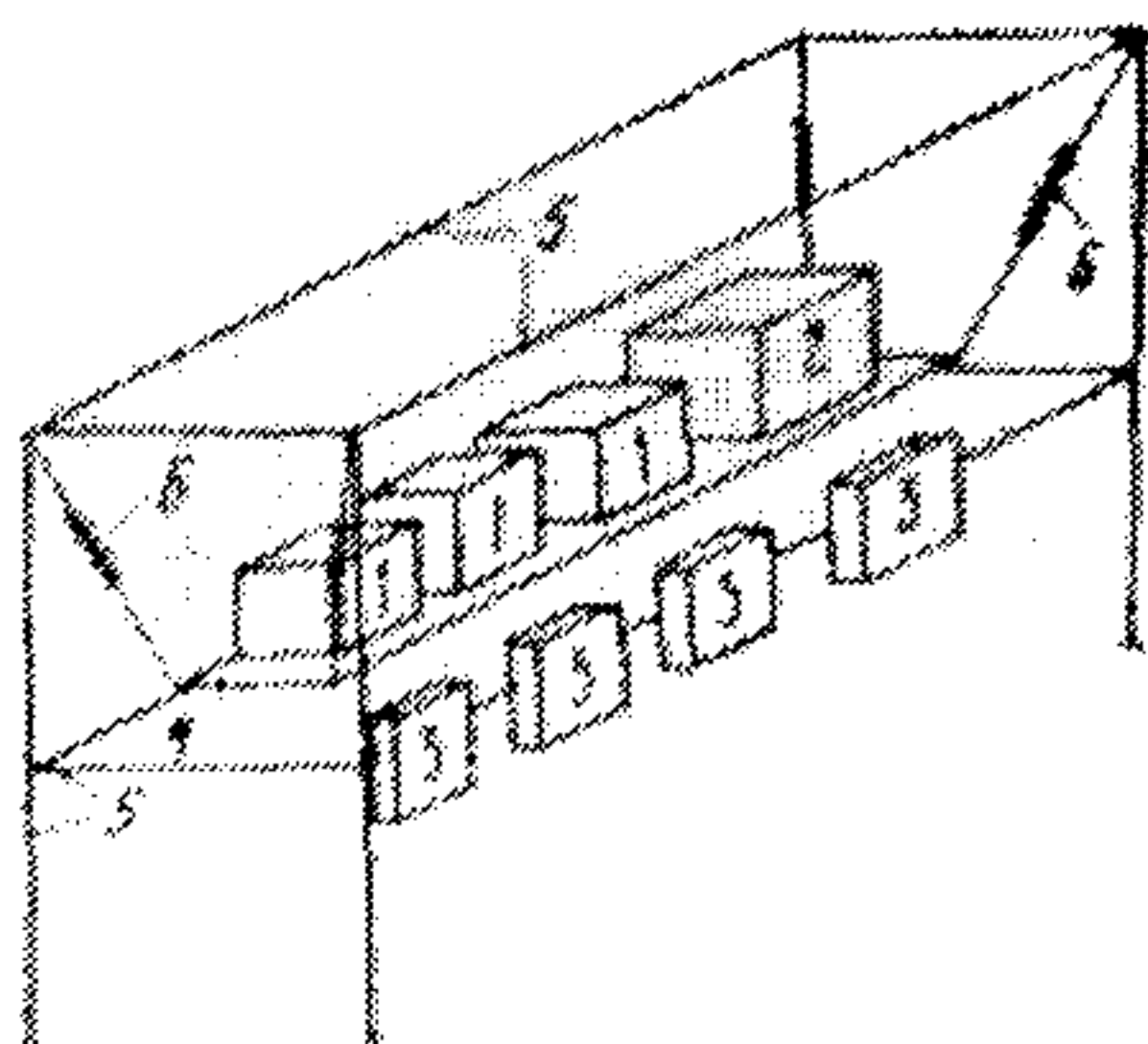
Рис.7. Схема рамы для гибкой подвески регистрирующей аппаратуры
