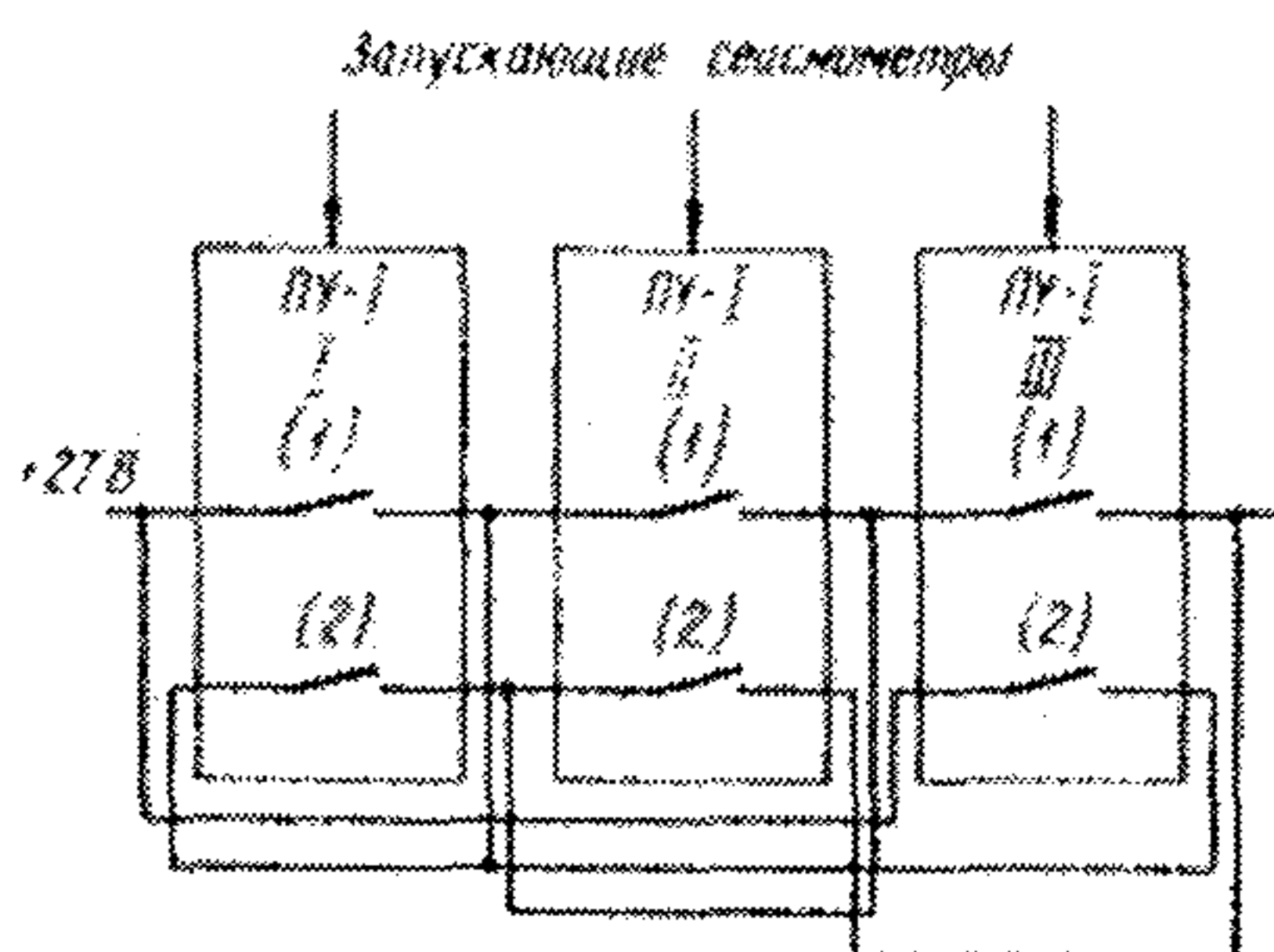
Рис.4. Логическая схема соединения трех параллельных пусковых устройств ПУ-1 (I, II, III – пусковые устройства); (1), (2) – контакты реле
