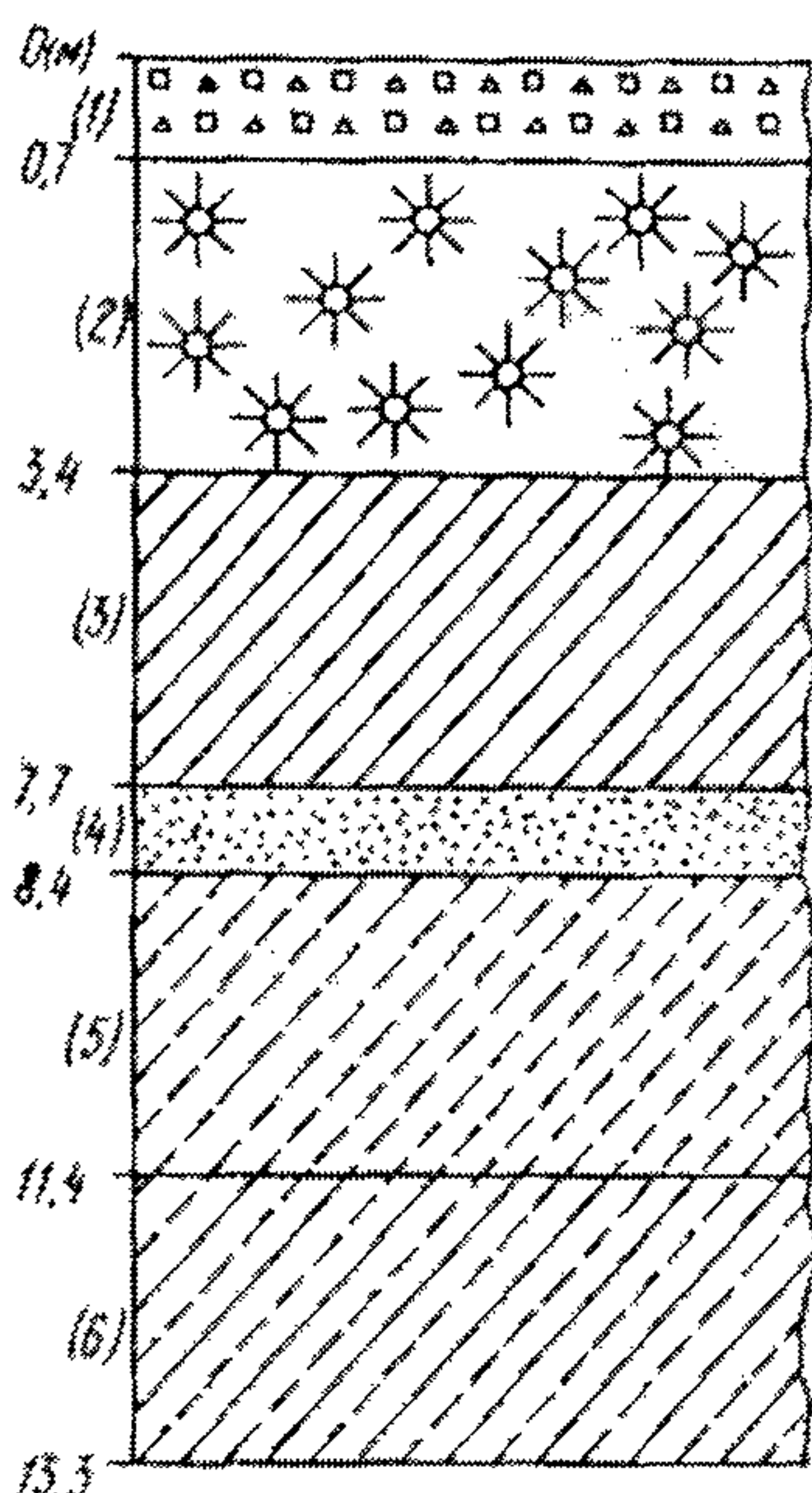
Рис.24. Геолого-литологическое строение площадки строительства
