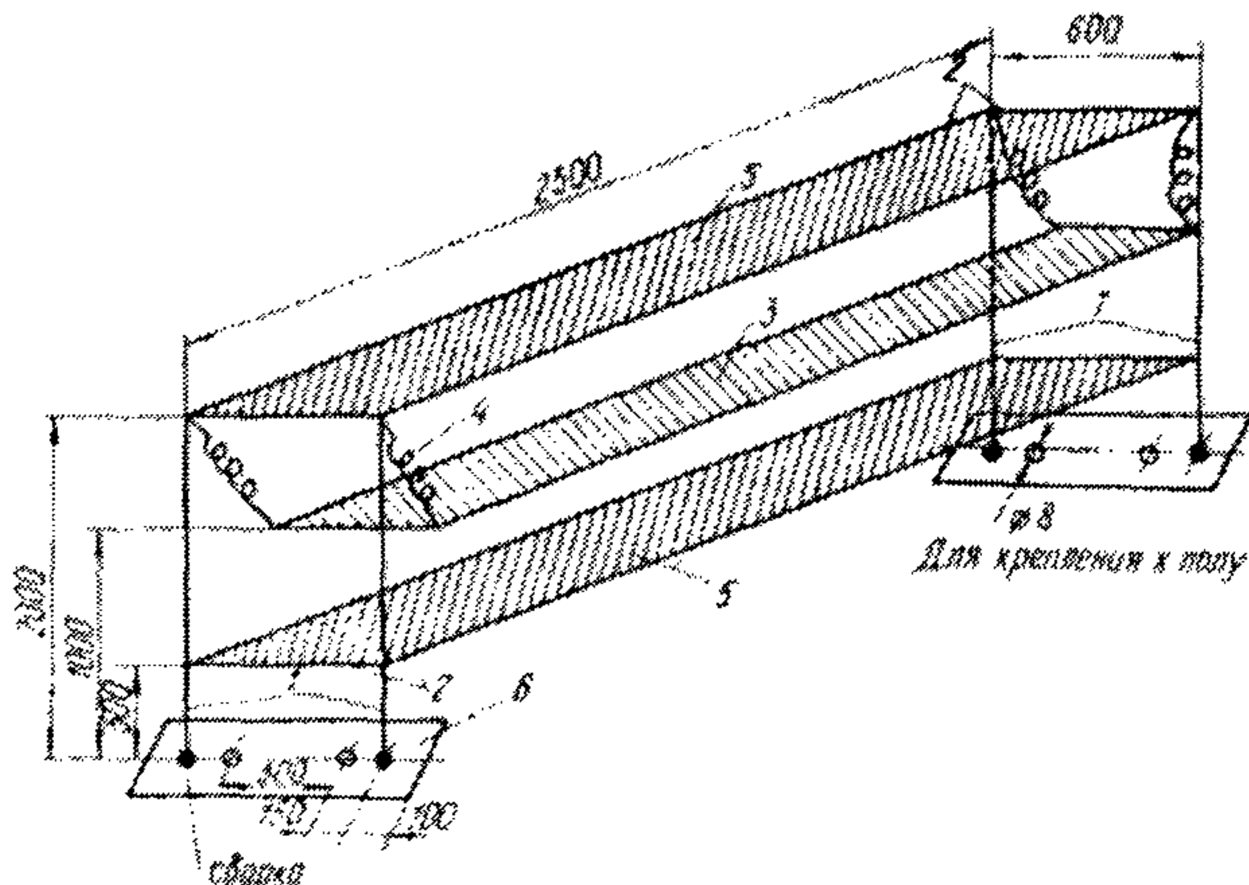
Рис. 26. Устройство защиты осциллографов от сейсмических воздействий
