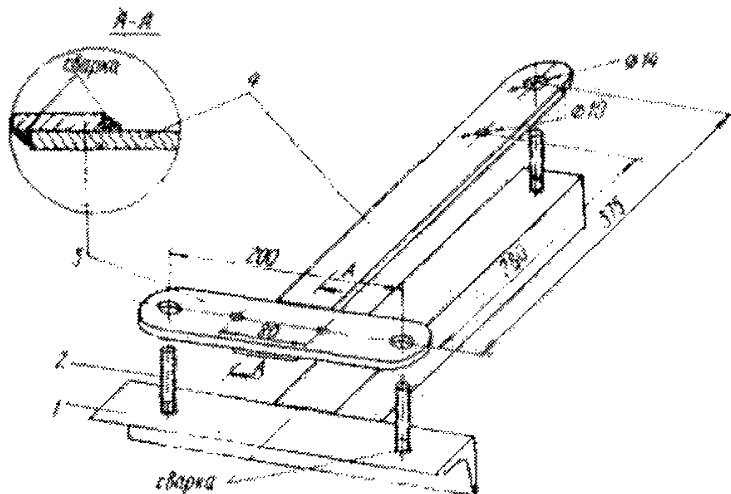
Рис.13. Переходный кронштейн для крепления С-5-С к постаменту
