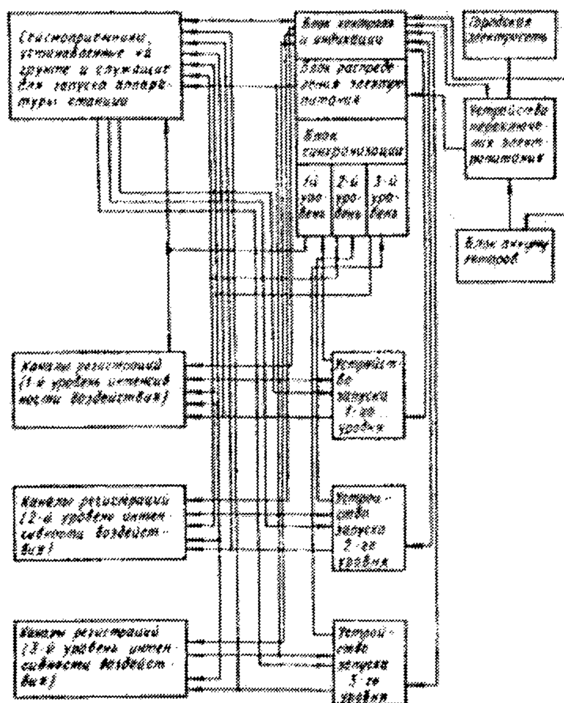
Рис.1. Структурная схема инженерно-сейсмометрической станции
