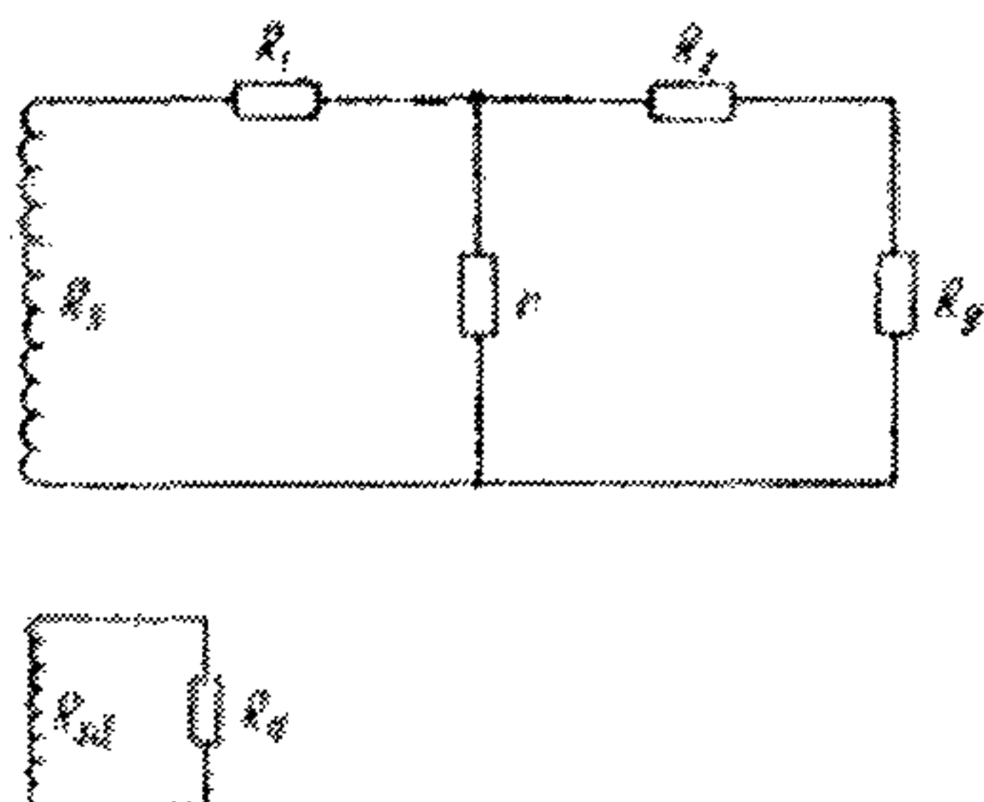
Рис. 16. Электрическая схема соединения сейсмометра и гальванометра в регистрационном канале станции ИСС
