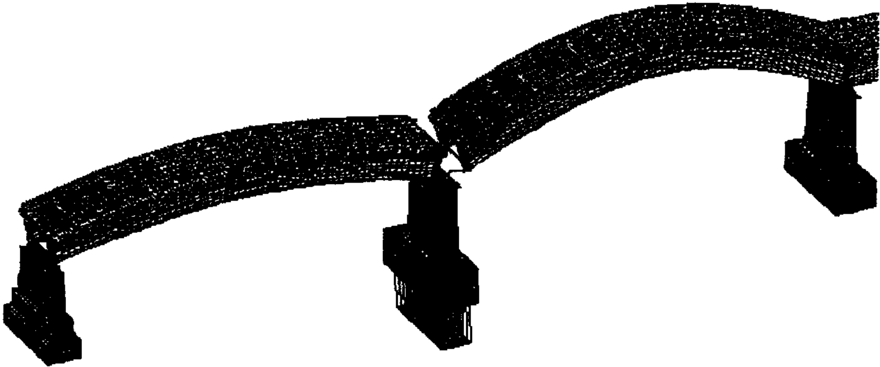
Форма колебаний МКЭ-модели на частоте 2.2 Гц
