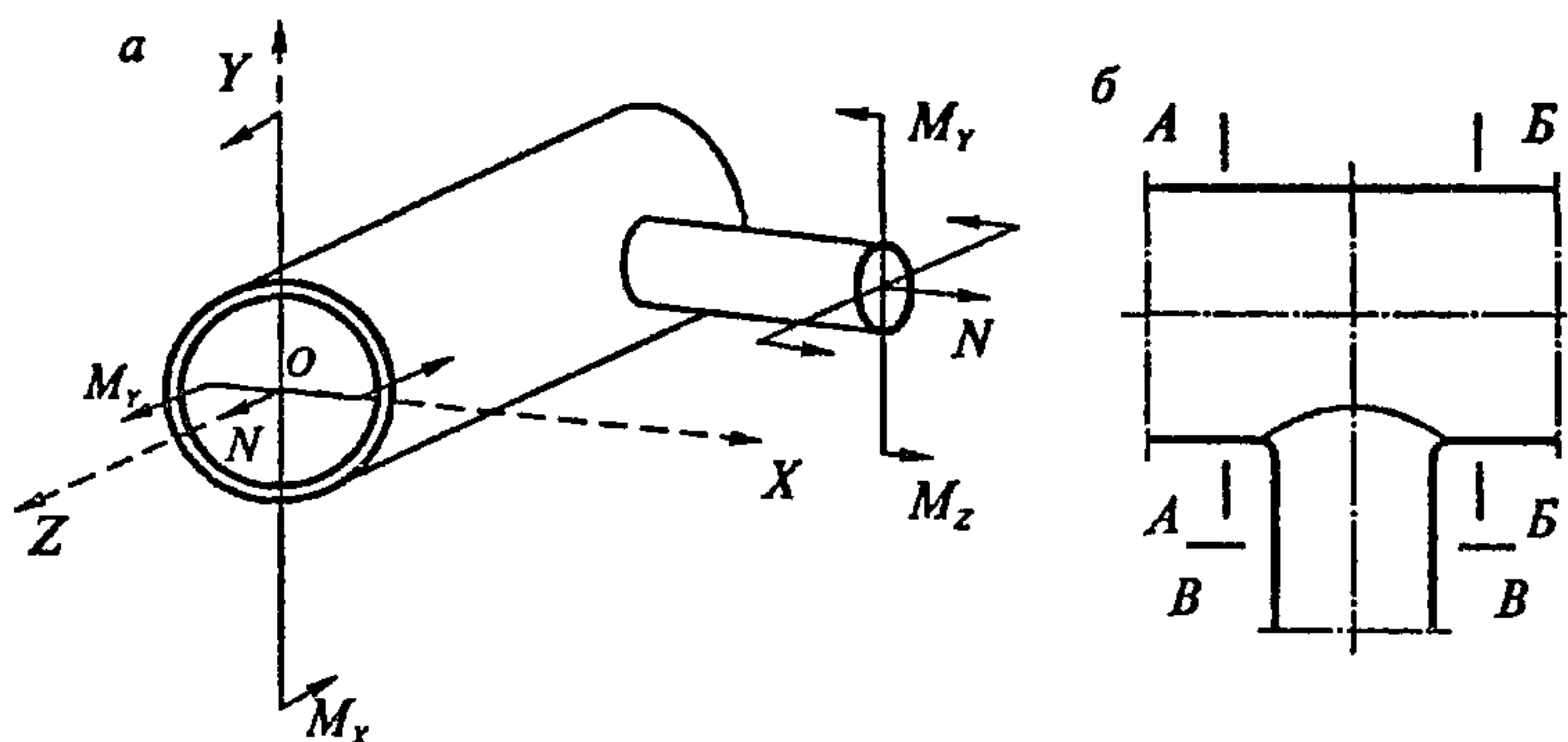
Рис. 5.4. Расчетная схема тройникового соединения: a – схема нагружения; б – расчетные сечения
