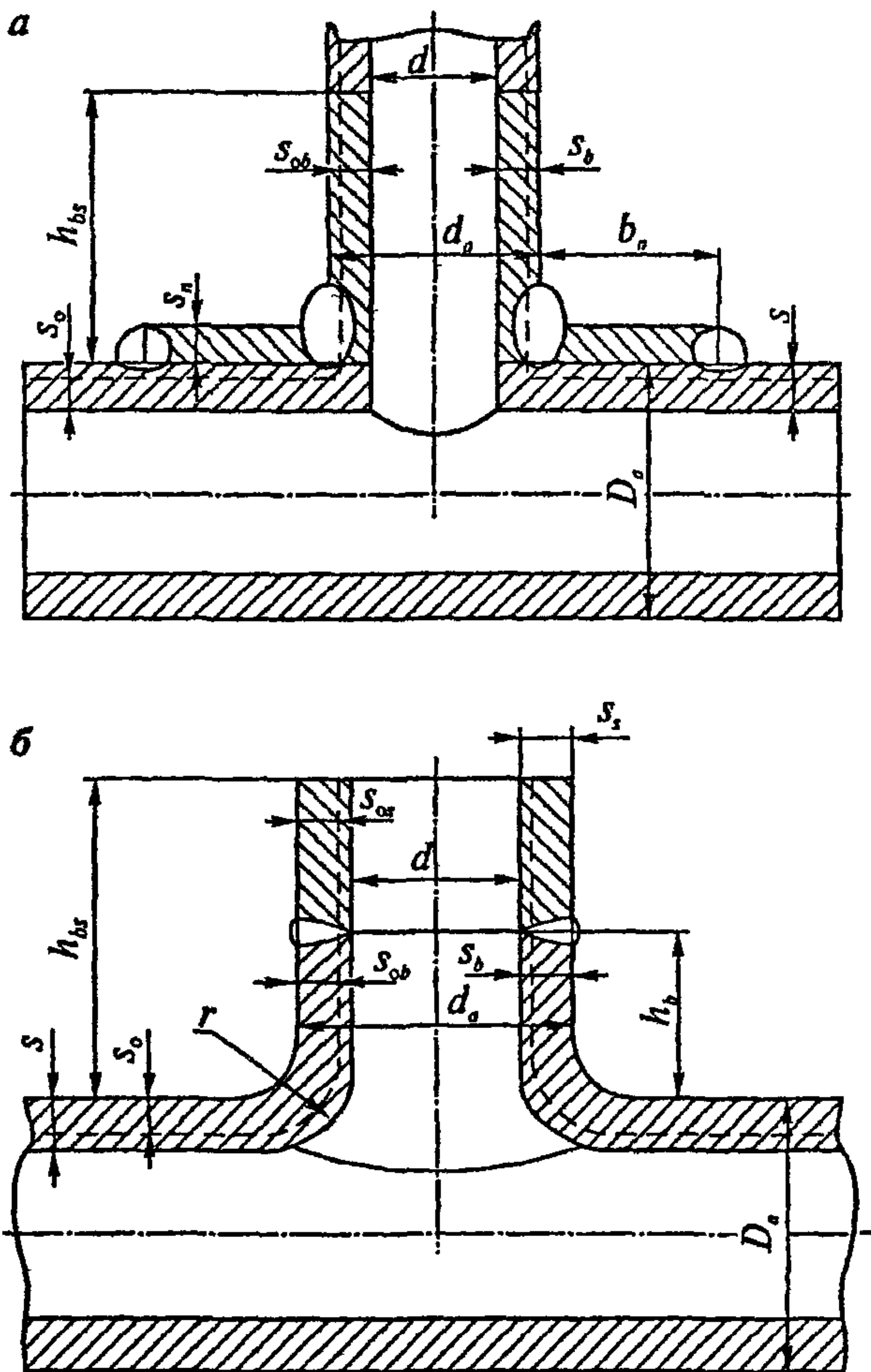
Рис. 4.3. Тройник: а – сварной; б – штампованный
