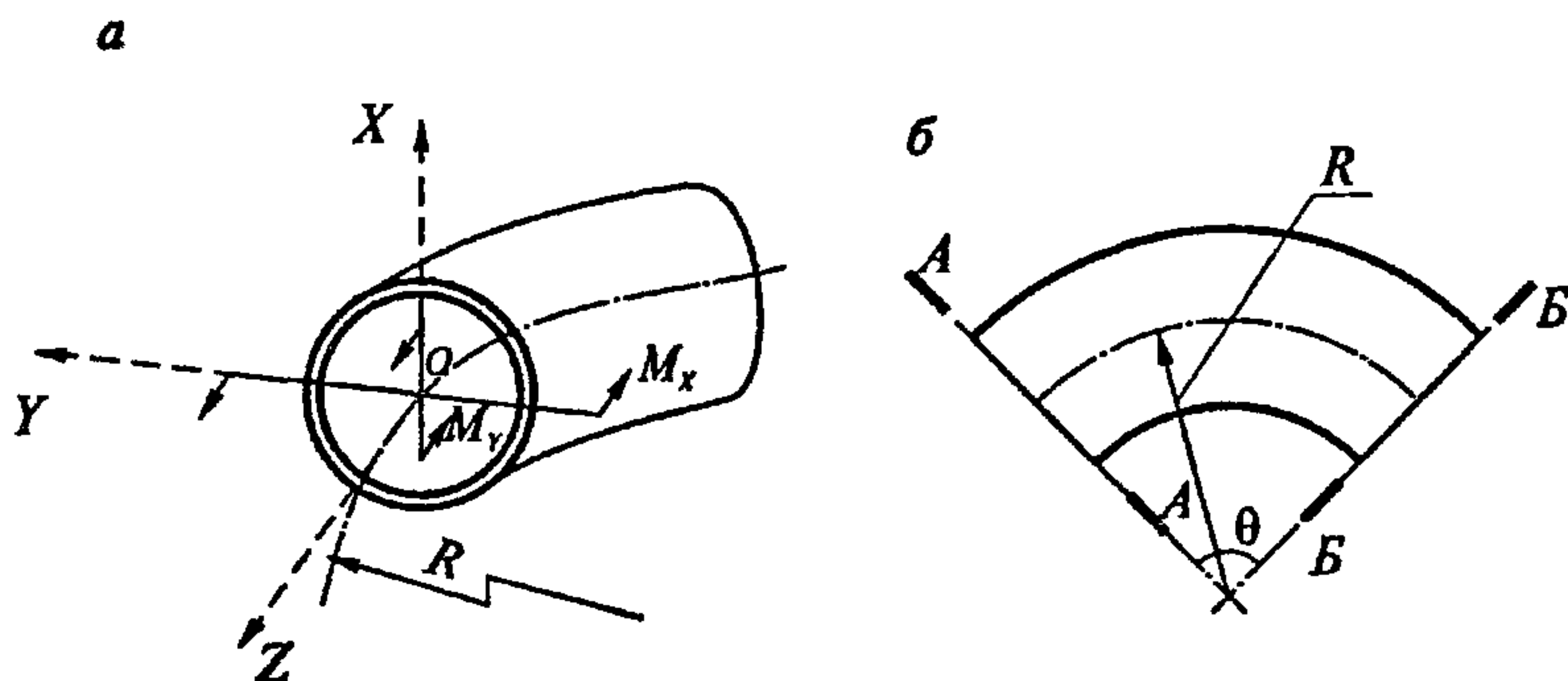
Рис. 5.3. Расчетная схема отвода: a – схема нагружения, б – расчетные сечения
