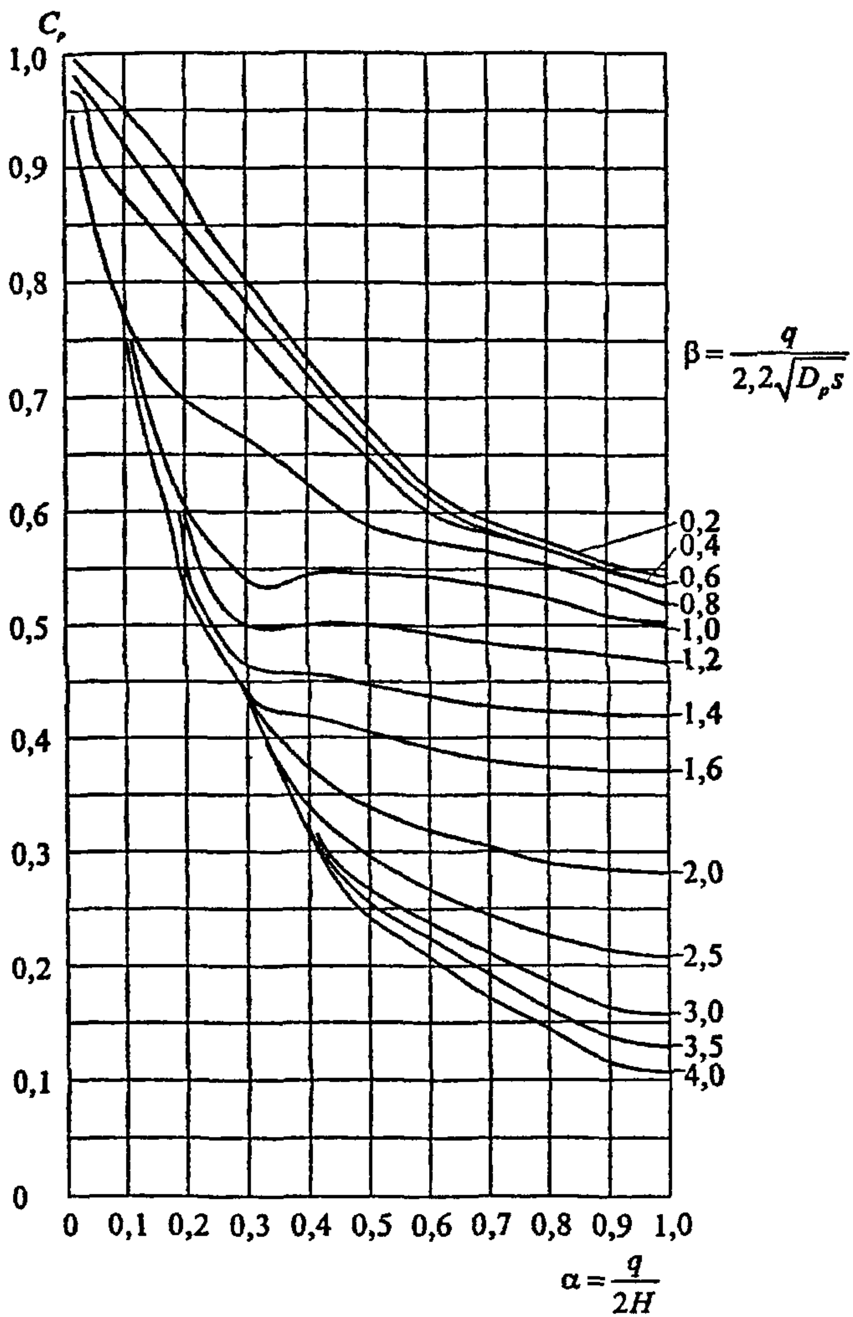
Рис. 5.9. Графики для определения коэффициента C_p
