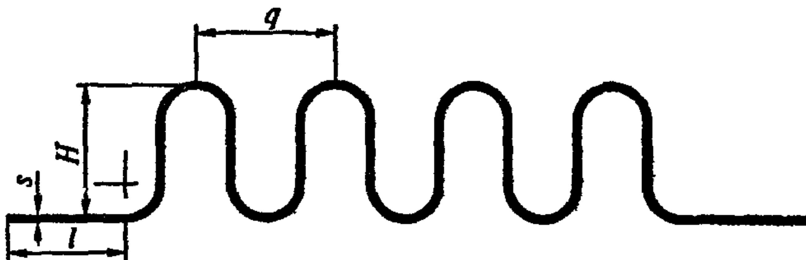
Рис. 5.5. Гибкий элемент компенсатора
