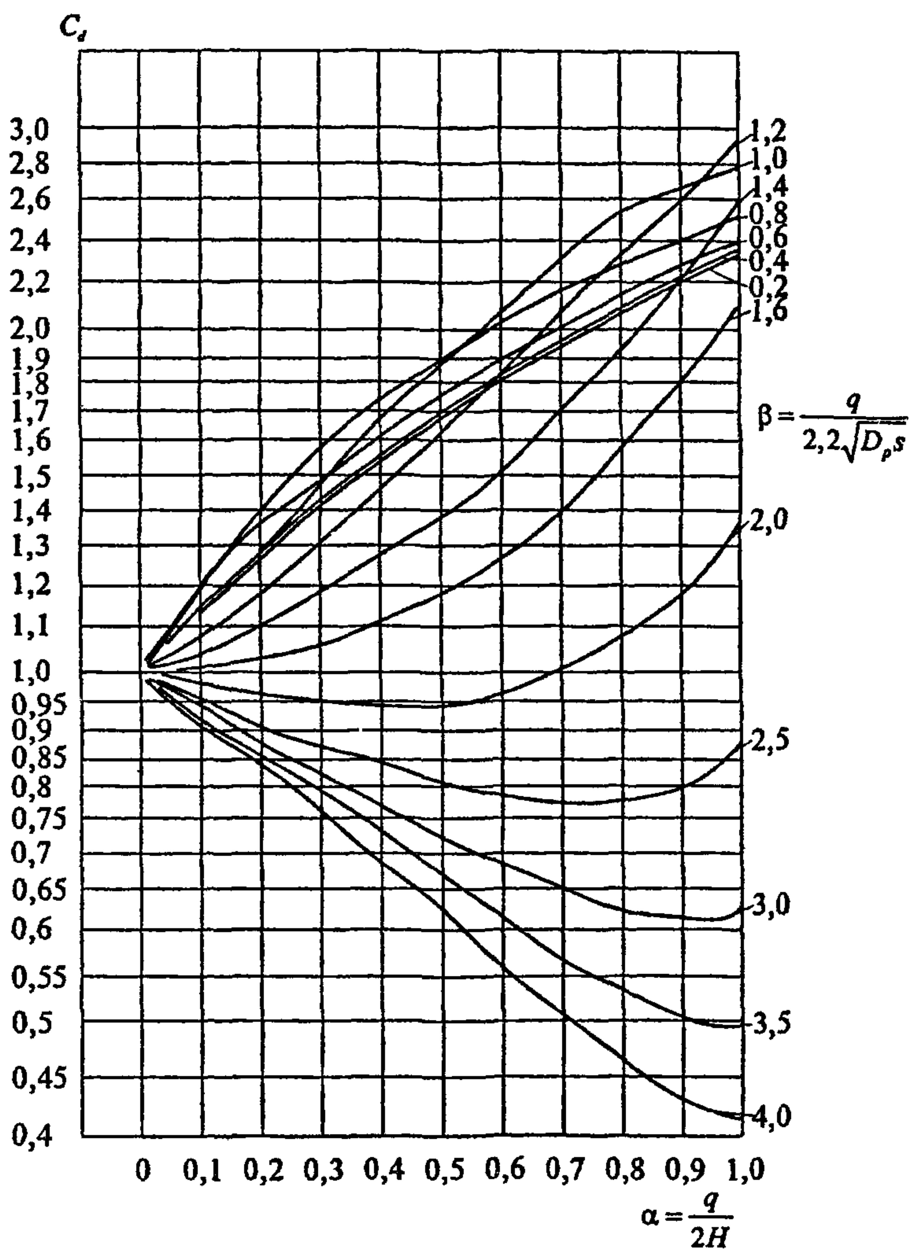
Рис. 5.10. Графики для определения коэффициента C_d
