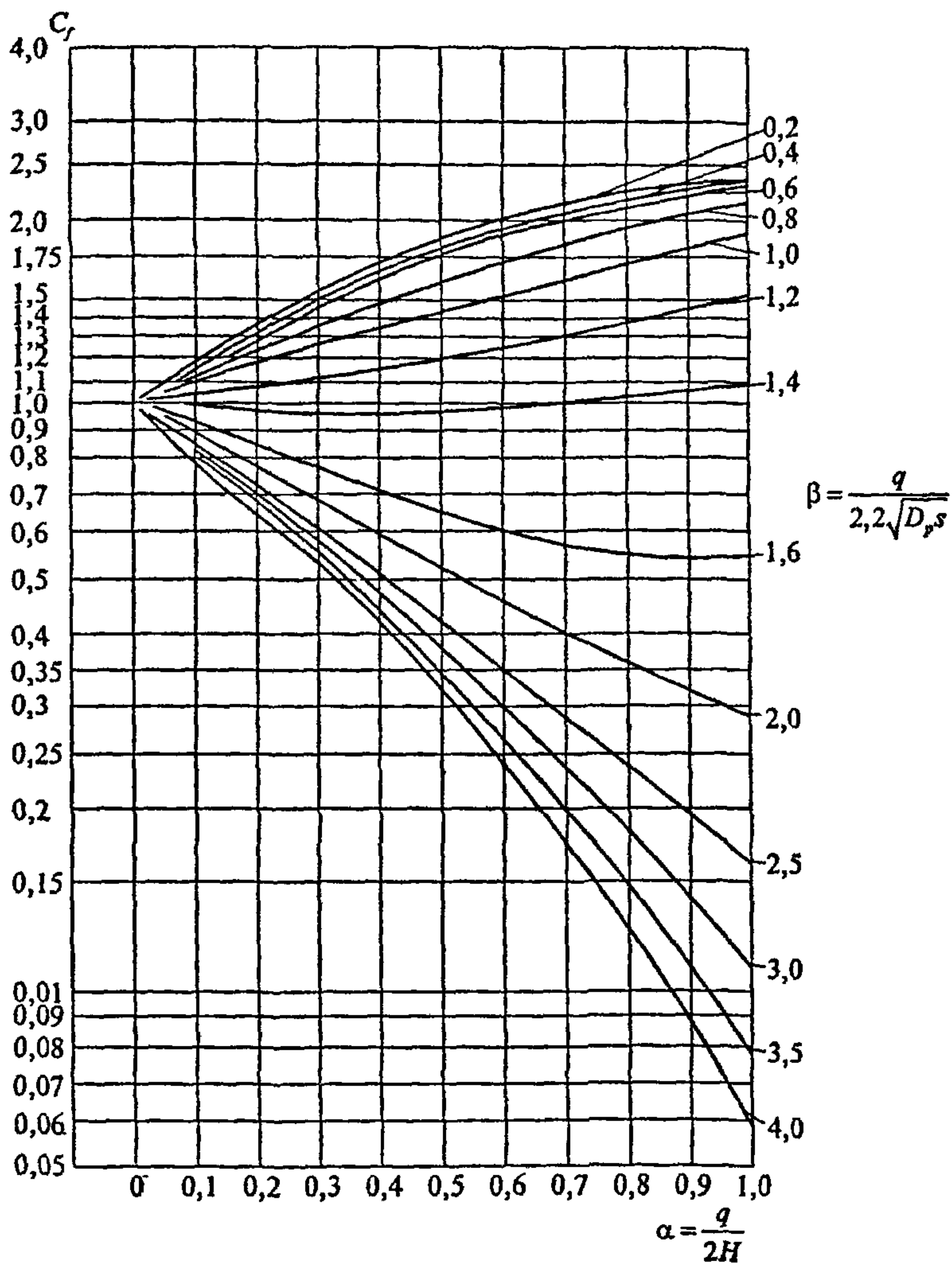
Рис. 5.8. Графики для определения коэффициента C_f
