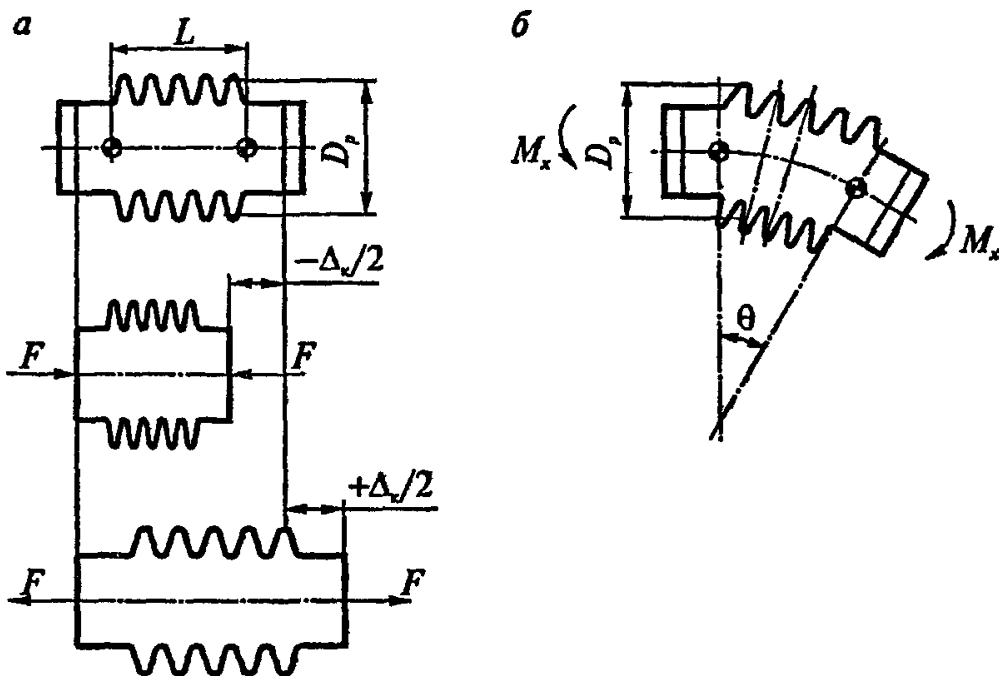
Рис. 5.6. Схема работы компенсатора: а – осевого; б – углового
