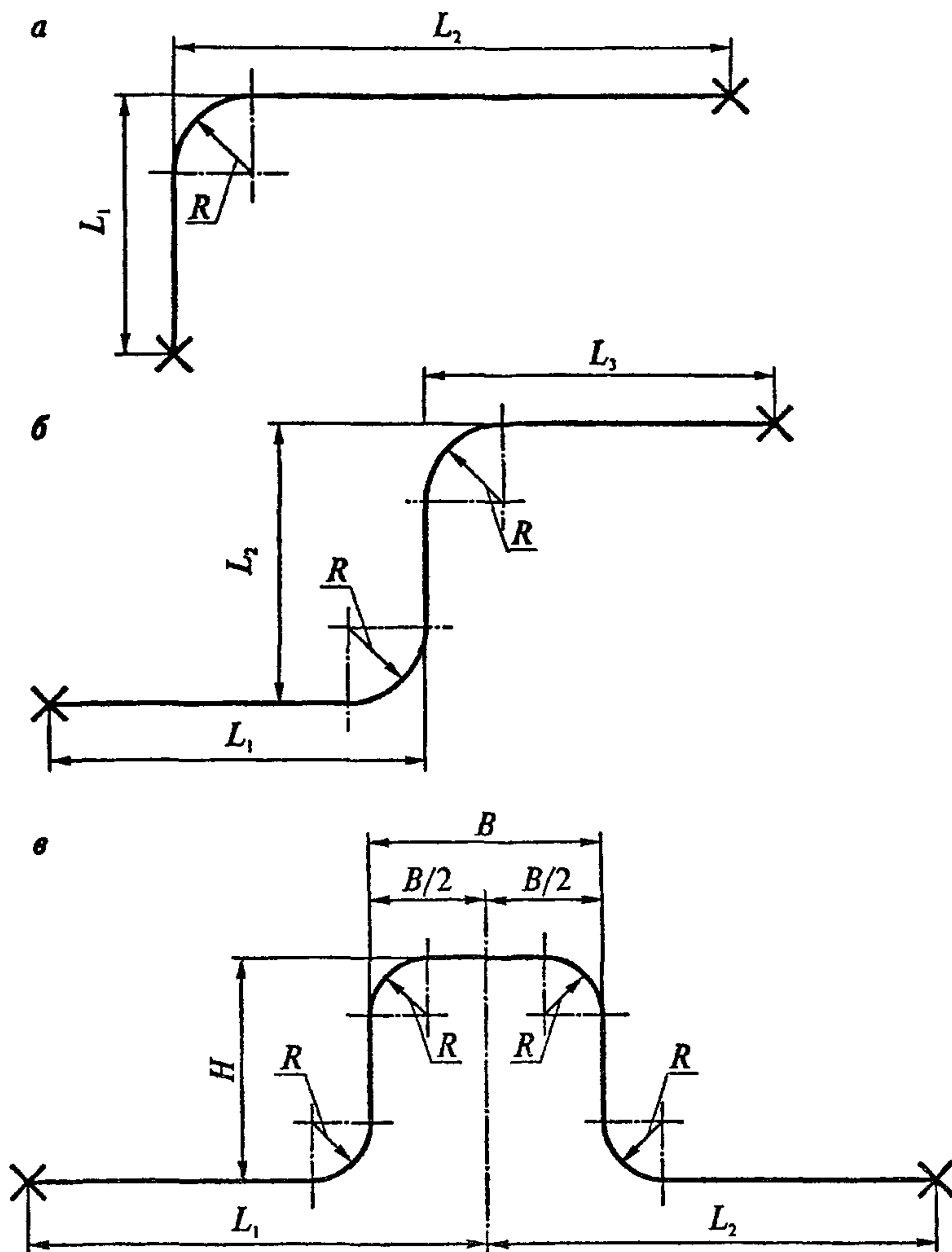
Рис. п. 3.1. Схемы участков трубопроводов с прямыми углами: a – Г-образной формы; б – Z-образной формы; в – П-образной формы
