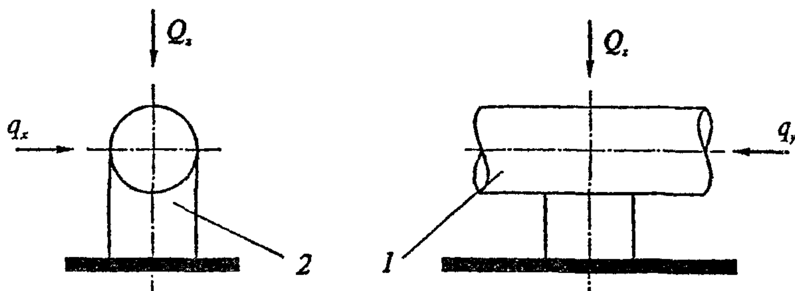
Рис. 5.1. Схема нагрузок на опору: 1 – труба; 2 – подвижная опора
