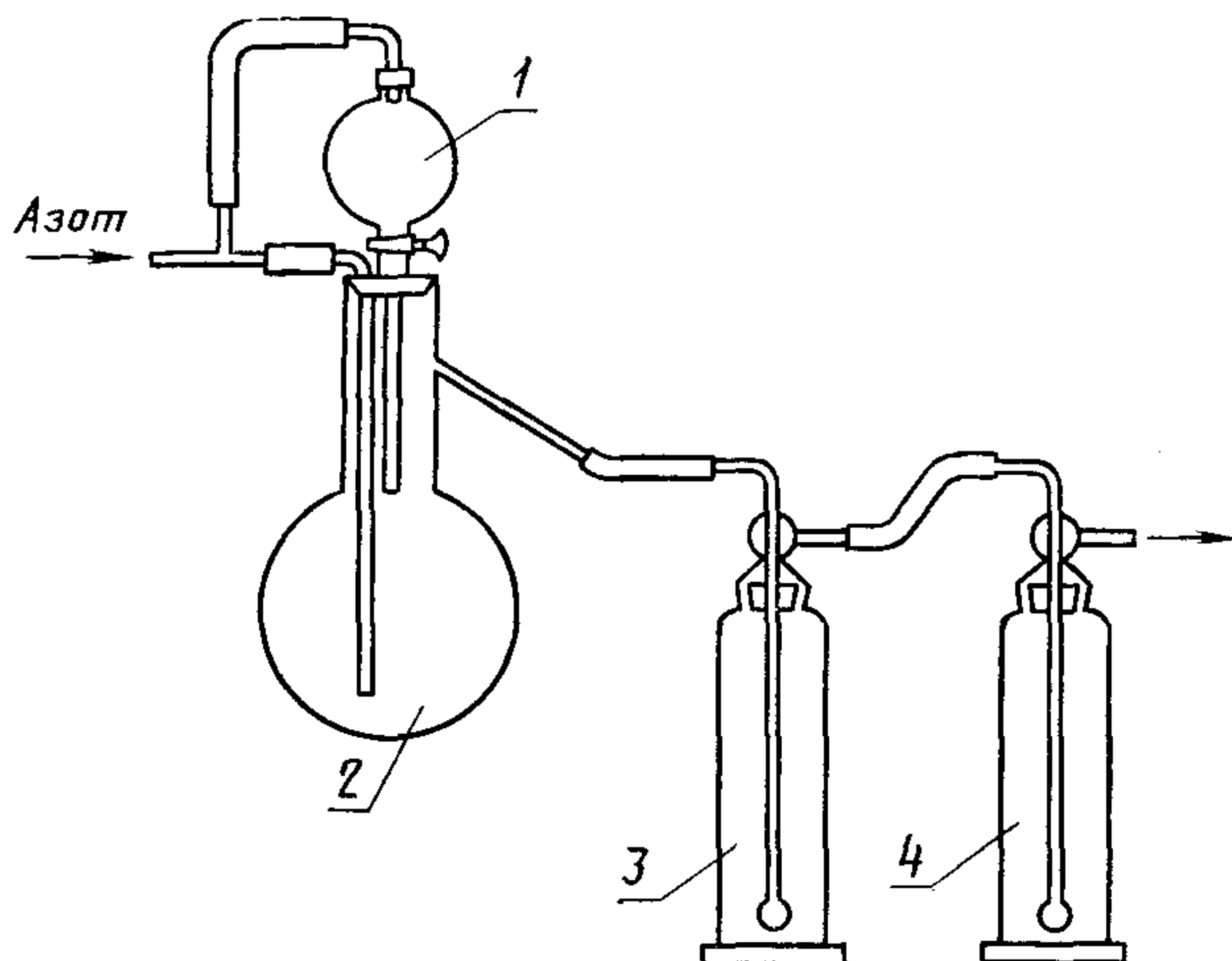
Прибор для выделения сульфидной серы
