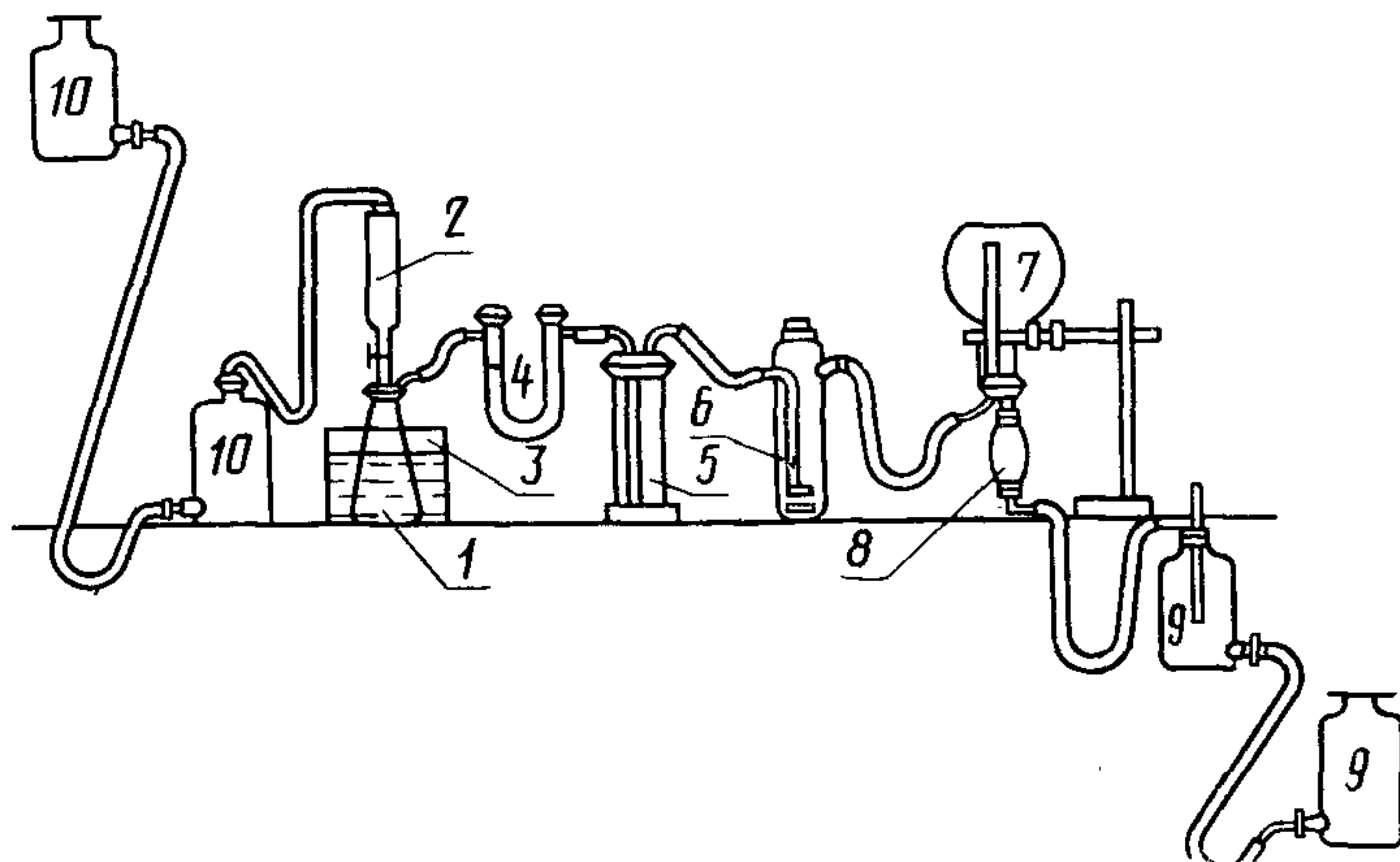
1—коническая колба; 2, 8—капельные воронки; 3—ванна для охлаждения колбы; 4—U-образная трубка; 5—склянка для промывания газа; 6—склянка для промывания газа со стеклянным пористым фильтром; 7—плоскодонная колба; 9—большой аспиратор; 10—малый аспиратор
