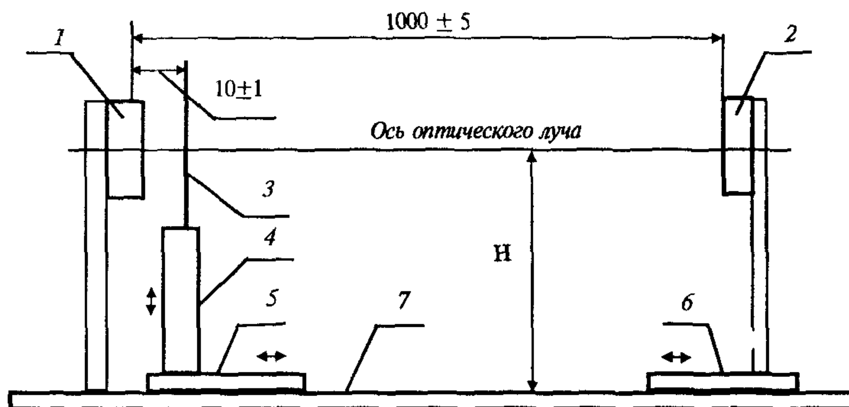
Рис. 1. Схема расположения элементов ИПДЛ и аттенюатора (вариант 1 - передатчик и приемник):
