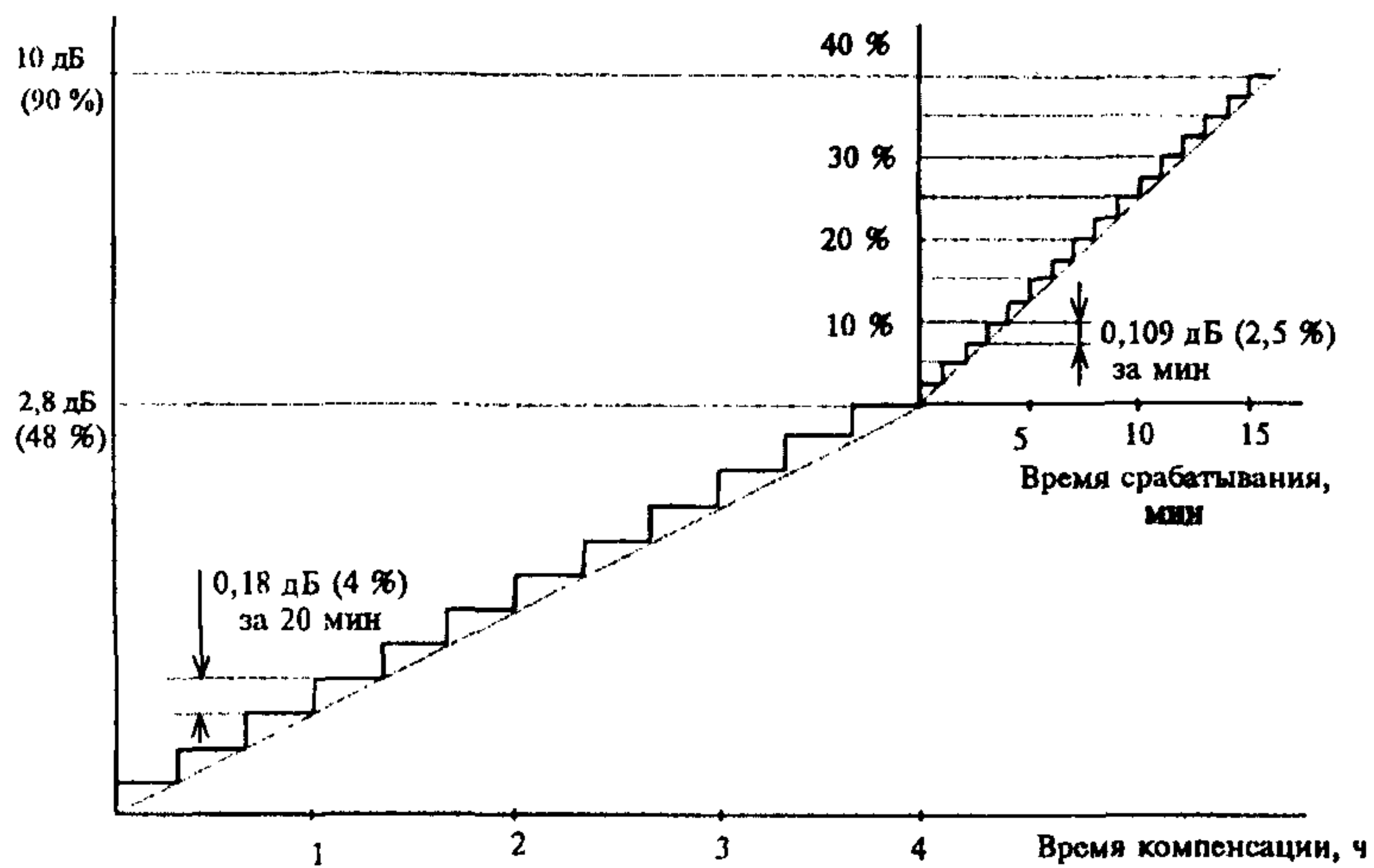
График зависимости изменения оптической плотности среды от времени
