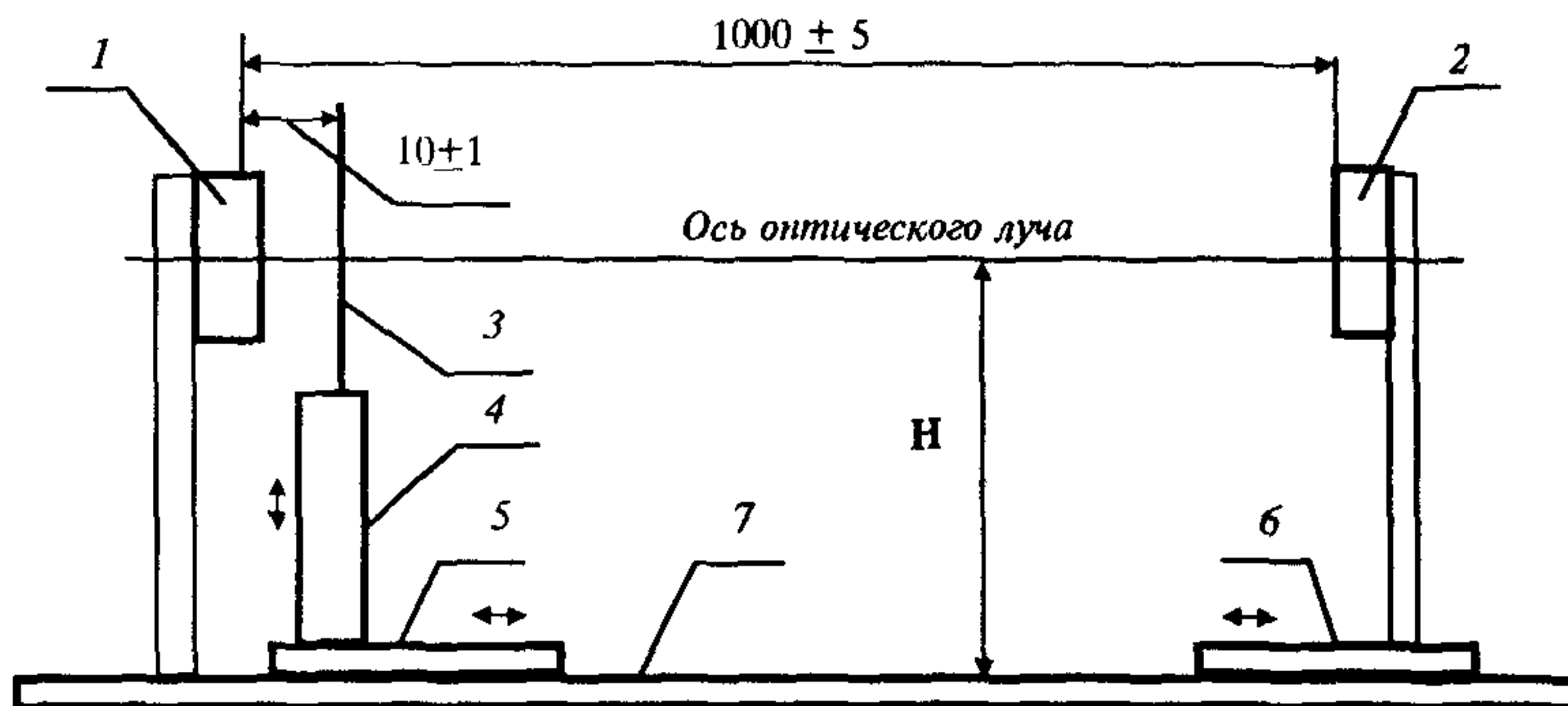
Рис. 2. Схема расположения элементов ИПДЛ и аттенюатора (вариант 2 - приемопередатчик и отражатель):
