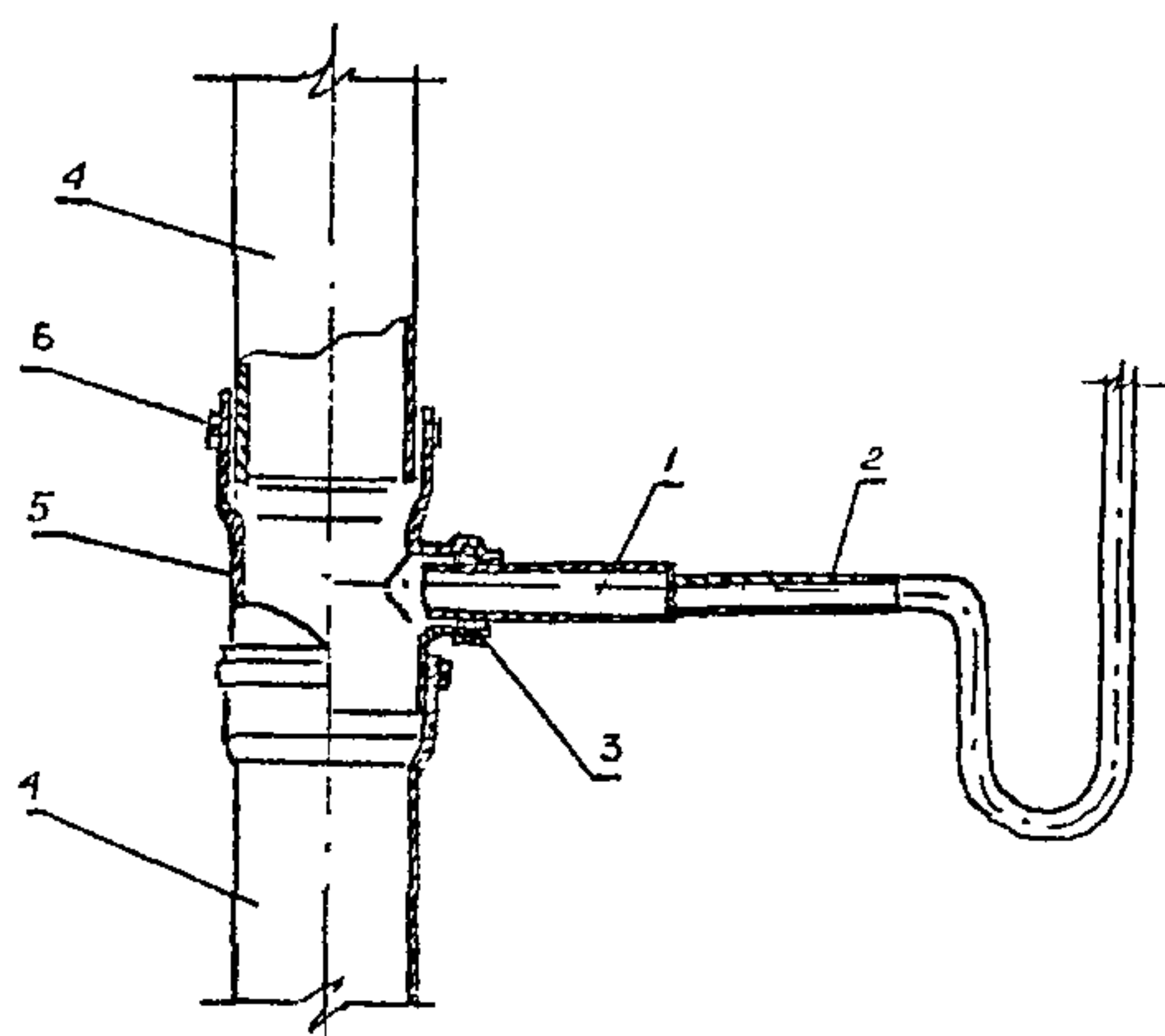
Рис. 9. Узел перепуска стоков:
