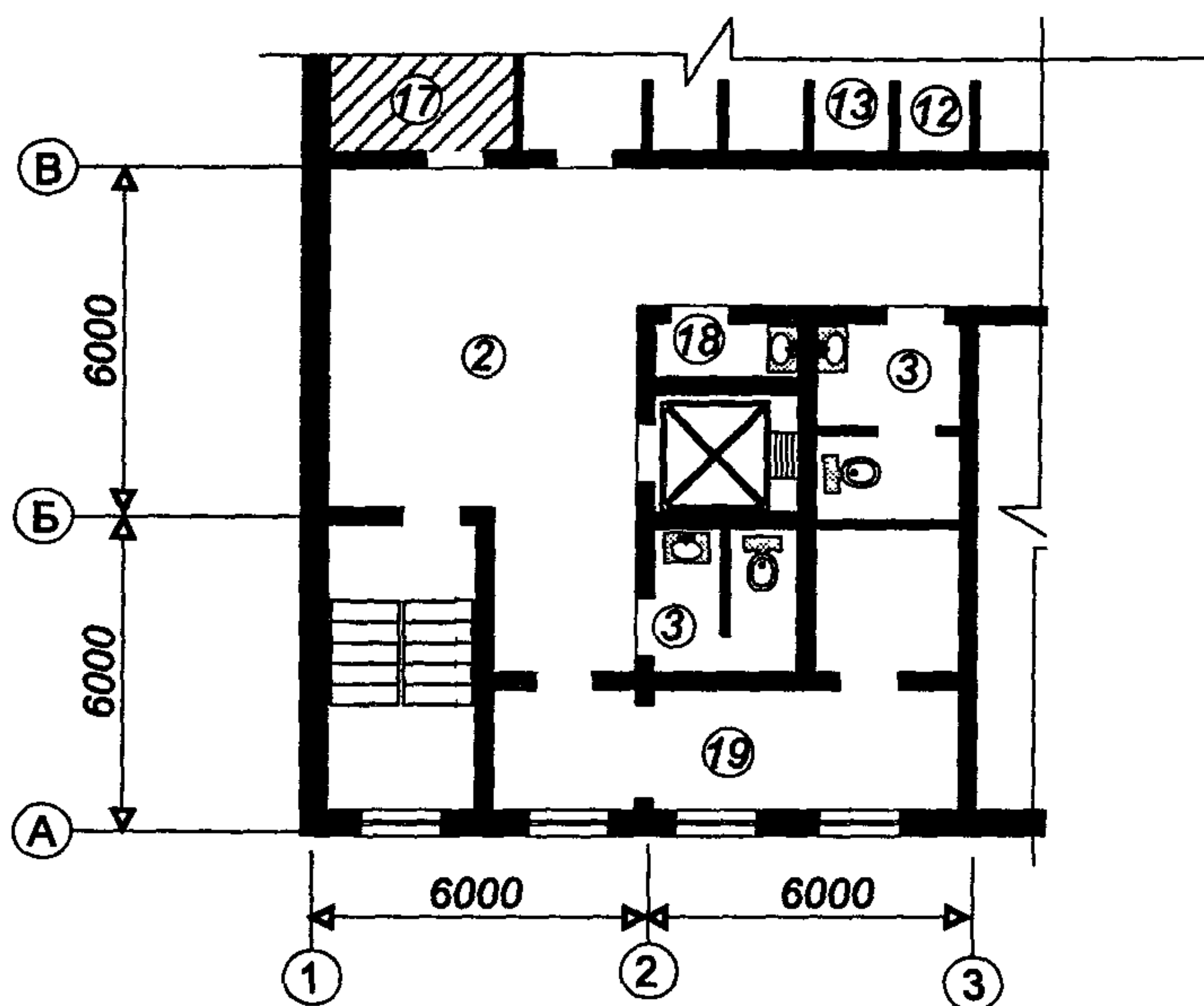
Фрагмент плана на отм. 4.800
