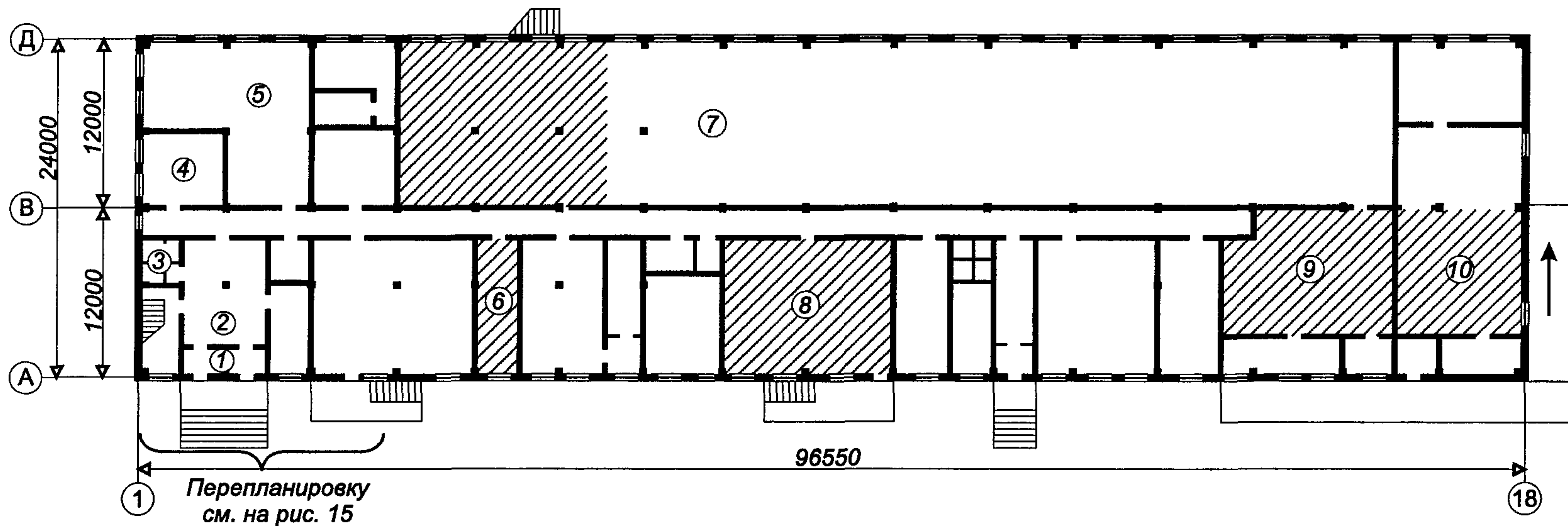
План на отм. 4.800
