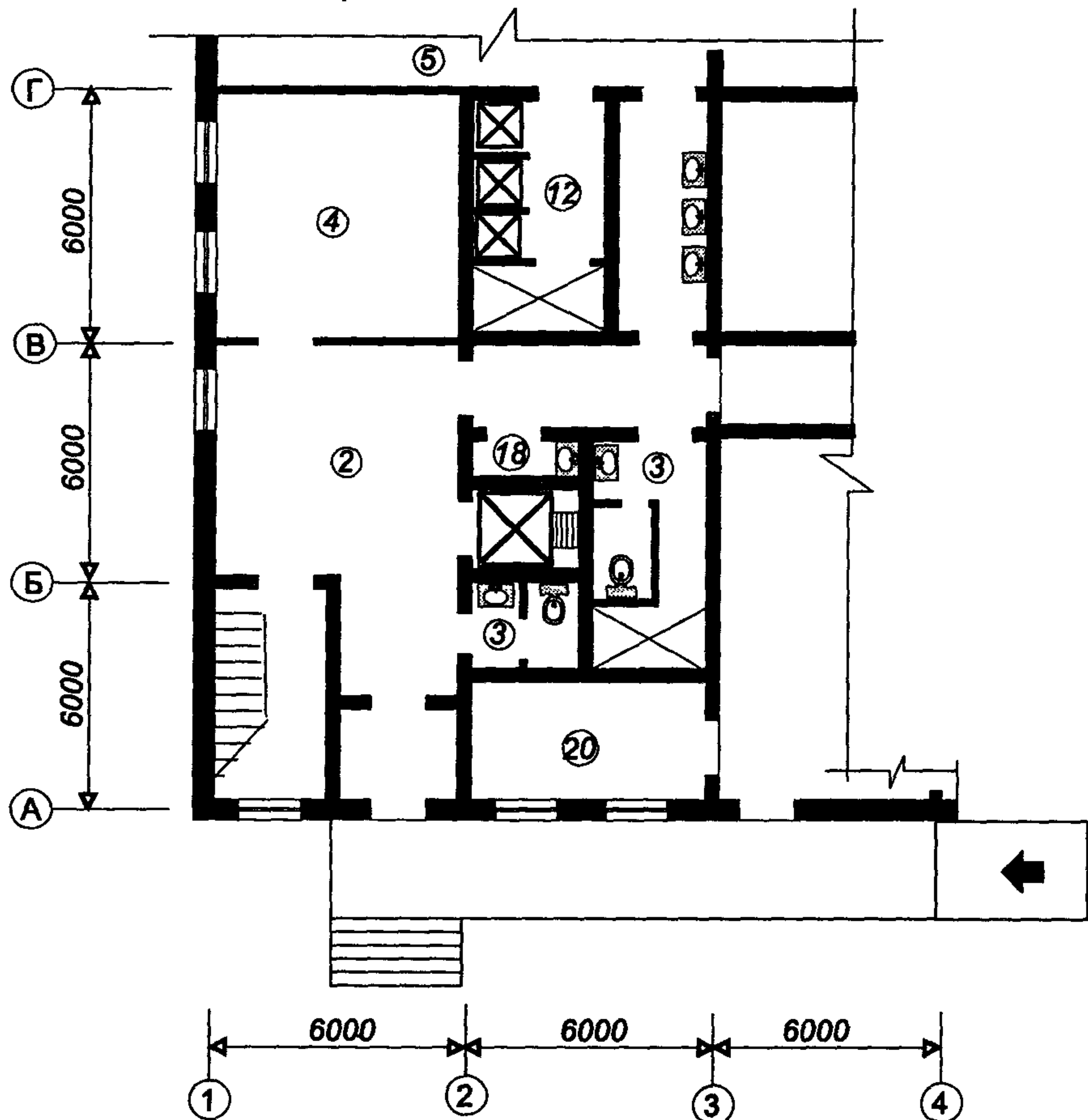
Фрагмент плана на отм. 0.000
