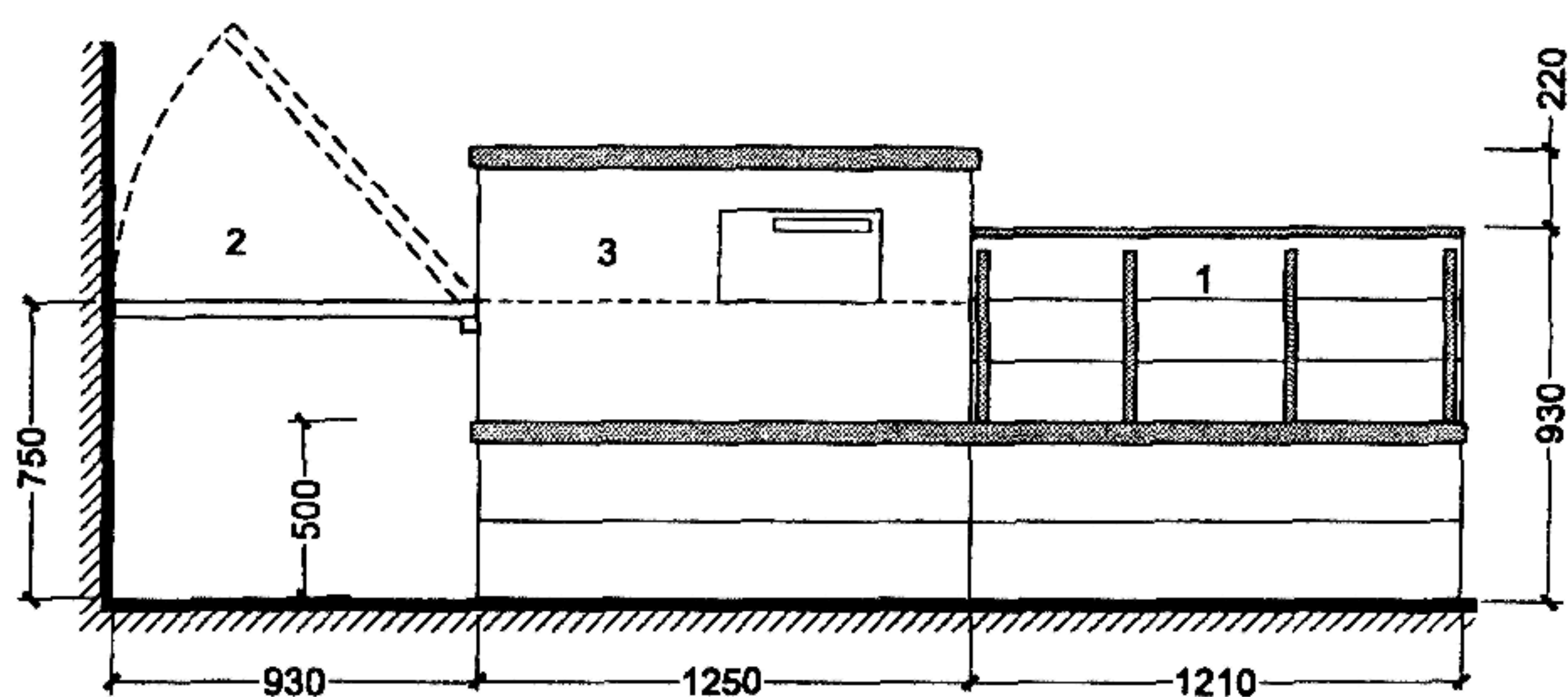
Вид спереди
