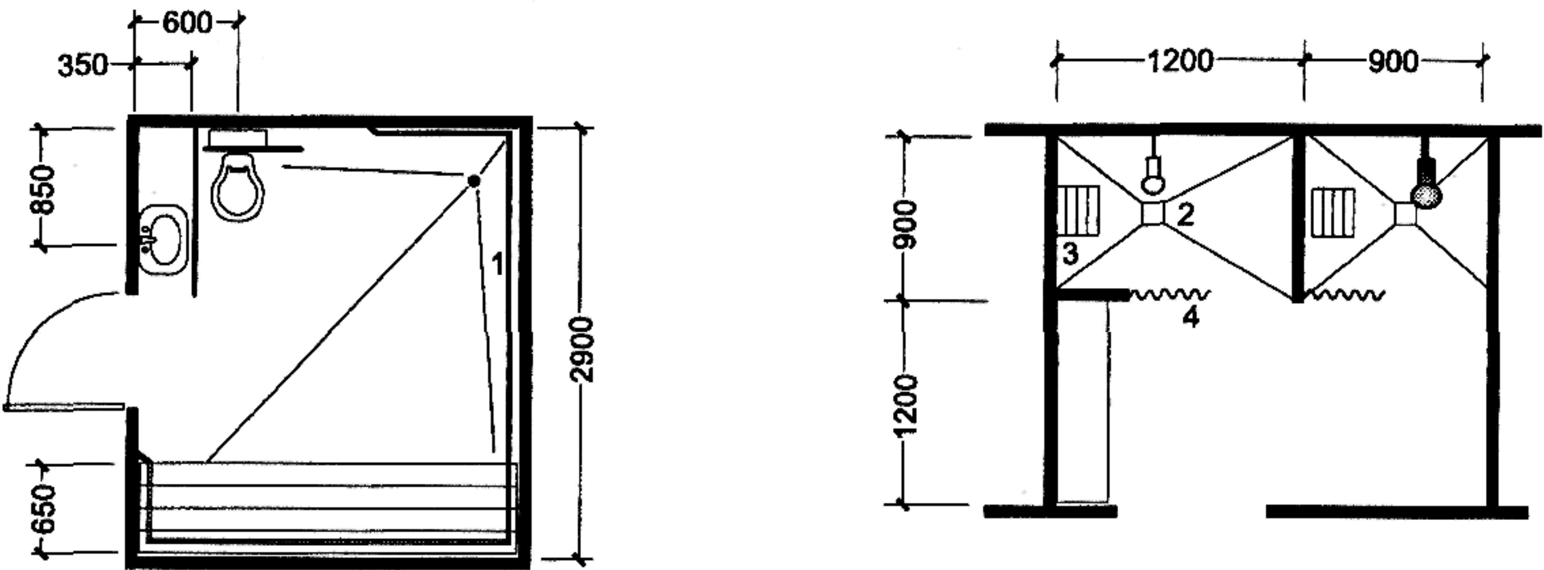
1 — поручень; 2 — душевая сетка; 3 — откидное или стационарное сиденье; 4 — занавес или раздвижная дверь
