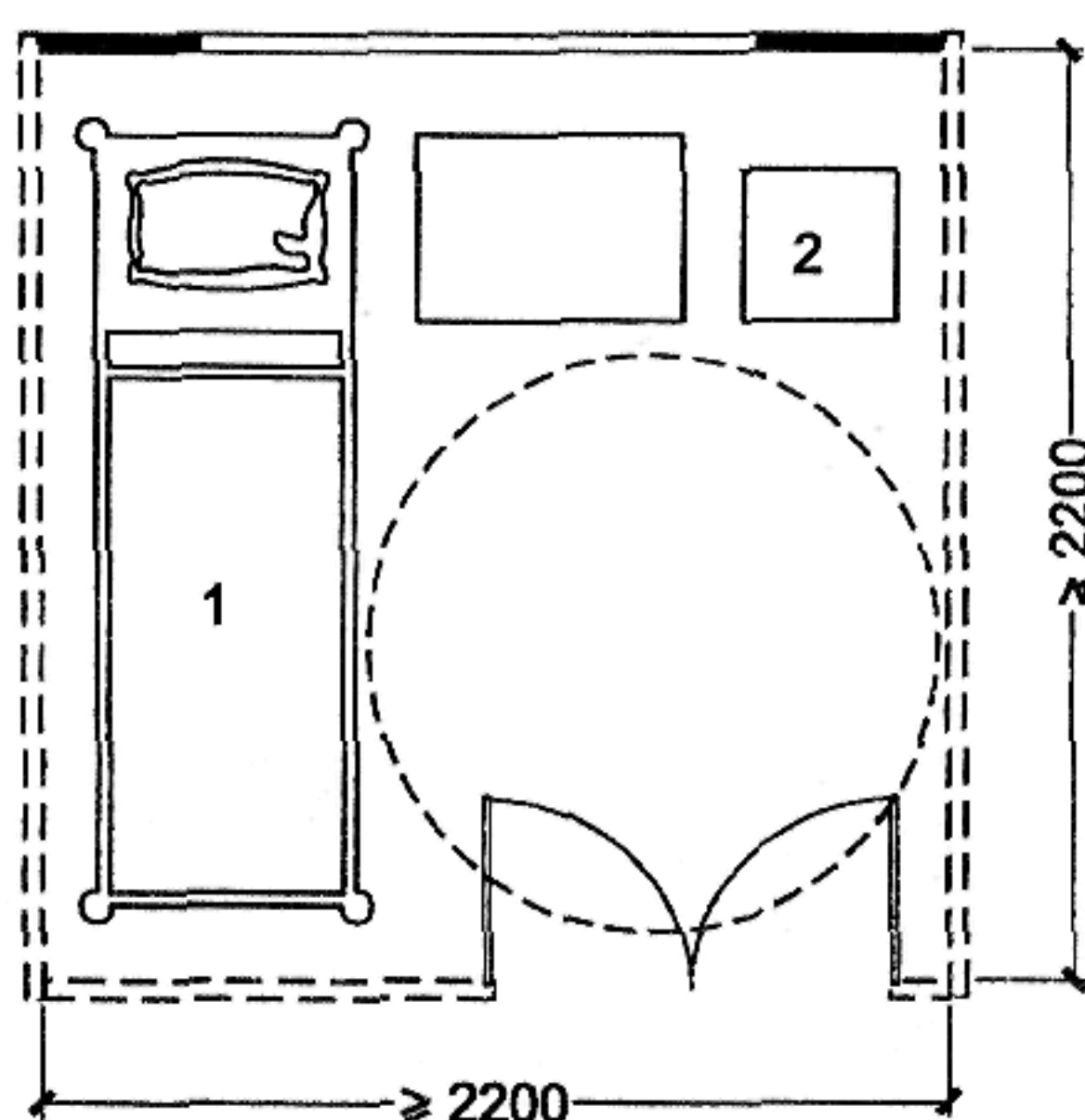
Кабинет светолечения 1 — кушетка; 2 — стол для аппаратуры
